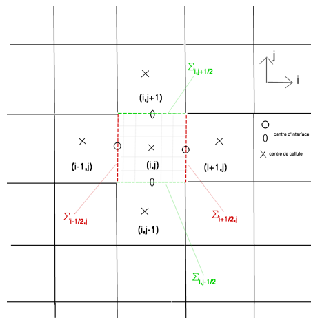
FIGURE 4.4 – Stencil pour le calcul de gradients aux centres des cellules
