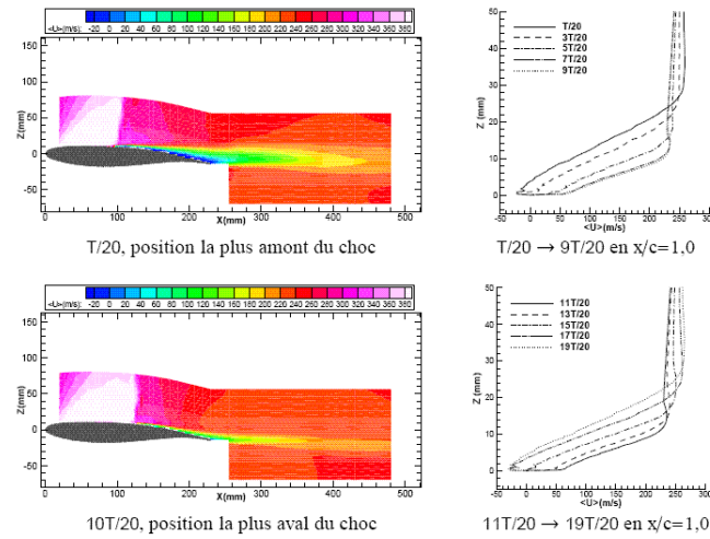
FIGURE 3.7 – Visualisations de la vitesse longitudinale moyenne (position la plus amont et aval du choc). M_\infty = 0.73 , Re = 3 \times 10^6 et \alpha = 3.5 .
