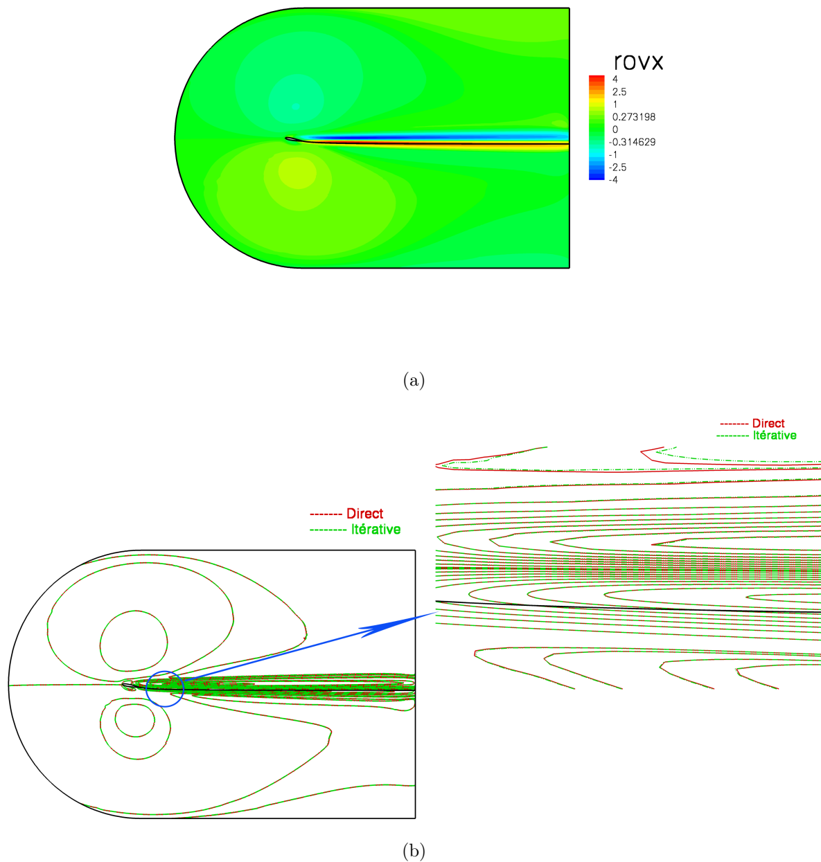
FIGURE 7.3 – Cas d'un écoulement laminaire compressible pour un profil NACA0012 avec incidence \alpha = 10 , M = 0.5 et Re = 689 : Superposition des lignes d'isovaleurs de la variable (\rho) calculées par deux méthodes d'inversions (elsA et MUMPS)
