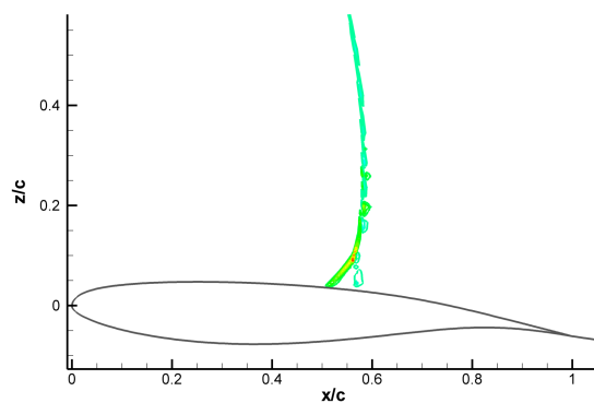
(b) \widehat{\rho w} : vue globale du choc
