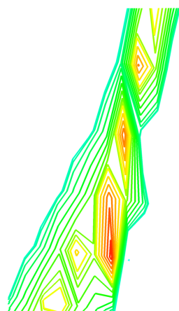
(c) \widehat{\rho w} : vue partiel du choc
