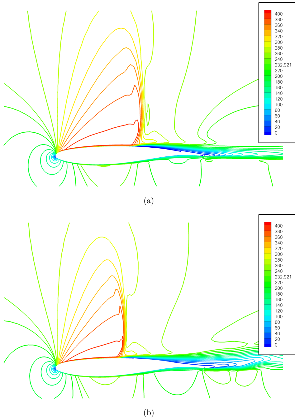
FIGURE 5.13 – Lignes des isovaleurs de la vitesse : (a) la position la plus avale et (b) la position la plus amont du choc ; calcul URANS avec le modèle (k - \omega) de Wilcox. M = 0.73 , \alpha = 3.5 et Re = 3.10^6
