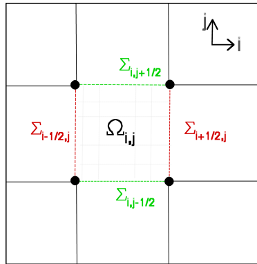
FIGURE 6.7 – Présentation d'une cellule de discrétisation \Omega_{i,j} et de ses interfaces pour un maillage bidimensionnel.
