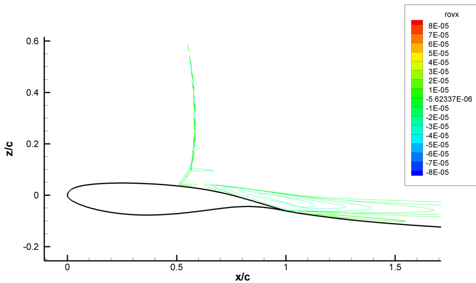
(b) \widehat{\rho u} : vue globale du choc
