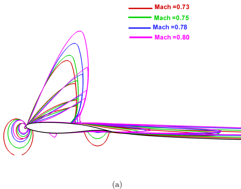
FIGURE 8.14 – Les contours des nombres de Mach pour un calcul RANS d'un écoulement compressible avec modèle de turbulence ( k - \omega ) de Wilcox sur un profil OAT15A, avec Re = 3.10^6 et \alpha = 3.5 .
