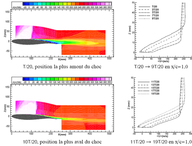
FIGURE 3.7 – Visualisations de la vitesse longitudinale moyenne (position la plus amont et aval du choc). M_\infty = 0.73 , Re = 3 \times 10^6 et \alpha = 3.5 .
