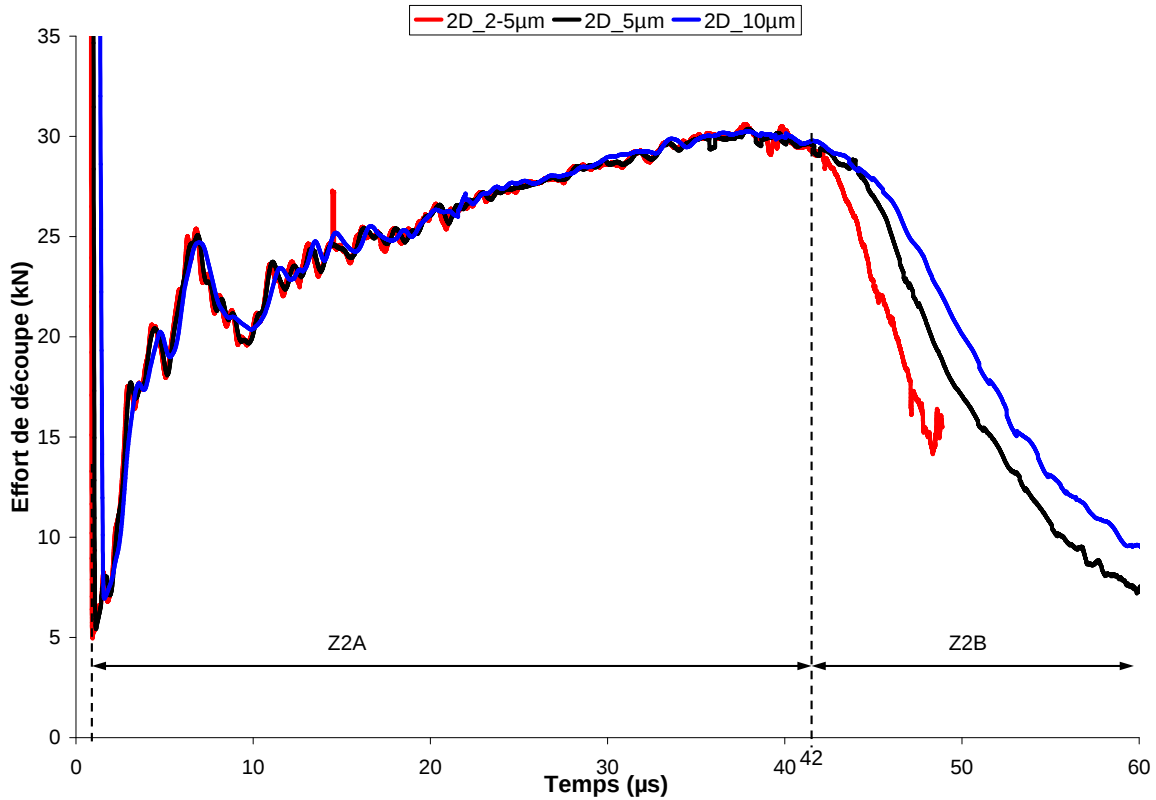
FIG. 4.11 – Effort en fonction du temps pour une simulation numérique en 2D avec une vitesse de poinçon de 15\text{ m/s} , un congé de 50\text{ }\mu\text{m} et une distance entre nœuds de 2 , 5 , 5 et 10\text{ }\mu\text{m}
