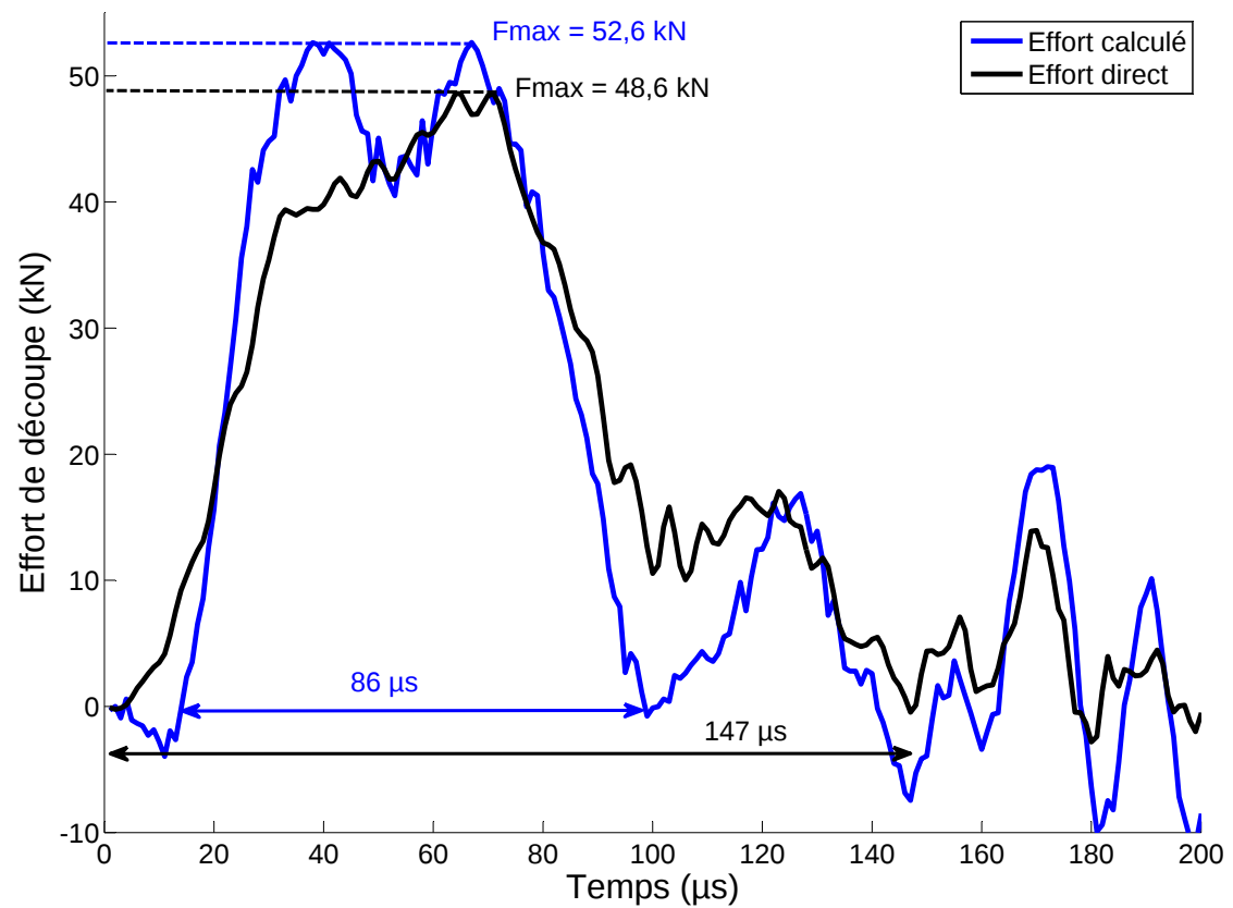
FIG. 3.20 – Evolution de l'effort calculé avec méthode par recomposition (en bleu) et méthode directe (en noir) pour une vitesse de poinçon égale à 18,1 \text{ m/s} et un jeu de 0,05 \text{ mm}
