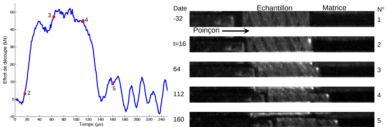
FIG. 5.25 – Evolution de l'effort de découpe et photos de la découpe à grande vitesse pour un échantillon de 3 mm d'épaisseur et une vitesse de poinçon égale à 10,7 m/s (Durée de découpe = 181 \mu s )
