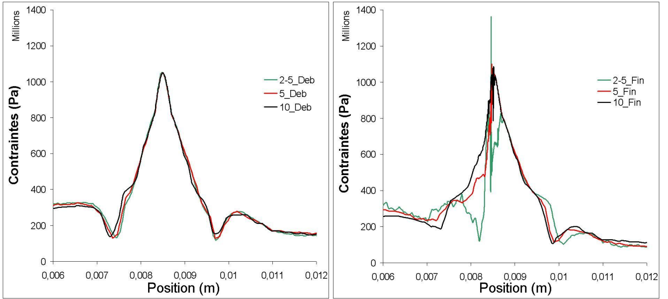
FIG. 4.14 – Contrainte en fonction de la position (en m) obtenue pour des simulations numériques en 2D avec une vitesse de poinçon de 15\text{ m/s} , un congé de 50\mu\text{m} et des distances entre les cellules égales à 2, 5, 5 et 10\mu\text{m}
