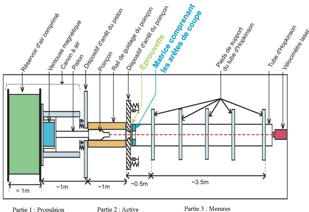
FIG. 2.5 – Représentation schématique du banc de découpe : vue de dessus
