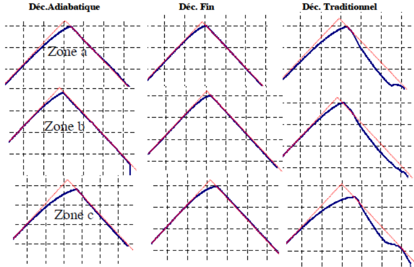
FIG. 1.12 – Profils du bord découpé obtenus avec les 3 procédés de découpage. Cas de la nuance S355MC. (Maillard, 2005)
