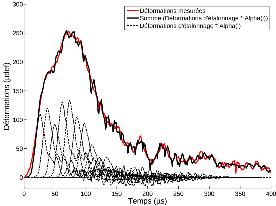
FIG. 3.10 – Déformations mesurées, construites et élémentaires dans le cas d'une découpe d'un échantillon de 2 mm avec une vitesse de 9,88 m/s et un jeu de 0,05 mm (essai 2C23)
