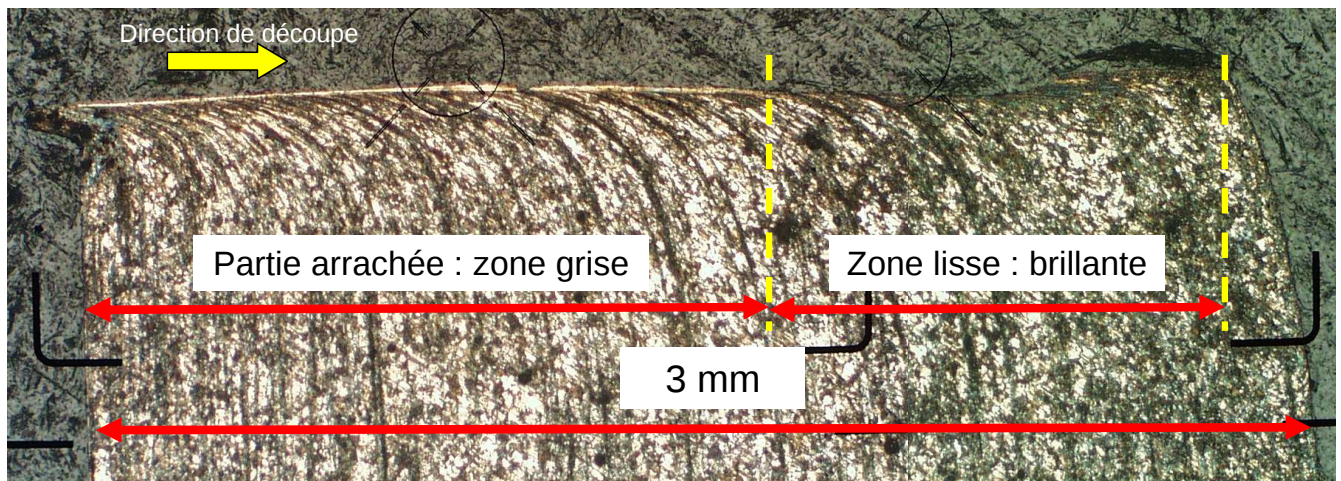
FIG. 5.18 – Photo au microscope optique d'un échantillon d'acier de 3 mm d'épaisseur, vitesse du poinçon = 16,2 m/s et jeu poinçon/matrice = 0,05 mm : présence d'une BCA
