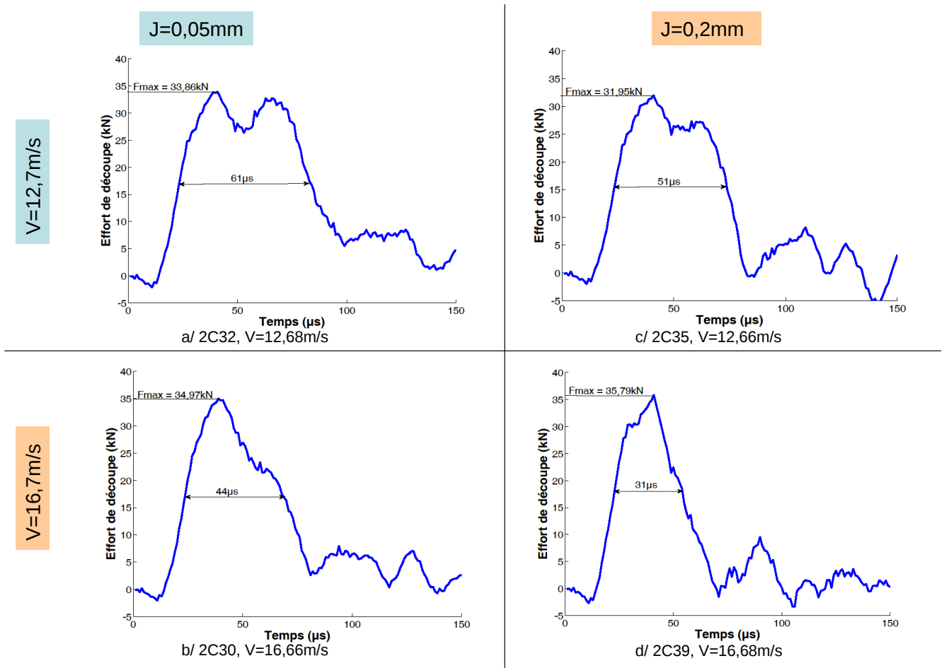
FIG. 5.2 – Evolution de l'effort en fonction du temps pour des vitesses de poinçon égale à 12,7 m/s et 16,7 m/s et un jeu poinçon matrice égal à 0,05 mm ou 0,2 mm, pour des échantillons de 2 mm d'épaisseur
