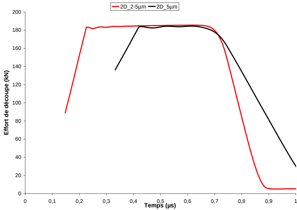
FIG. 4.16 – Effort de découpe en fonction du temps pour une simulation numérique en 2D avec une vitesse de poinçon de 15m/s , un congé de 50\mu m et une distance entre nœuds de 2,5 et de 5\mu m : zoom sur la zone Z1
