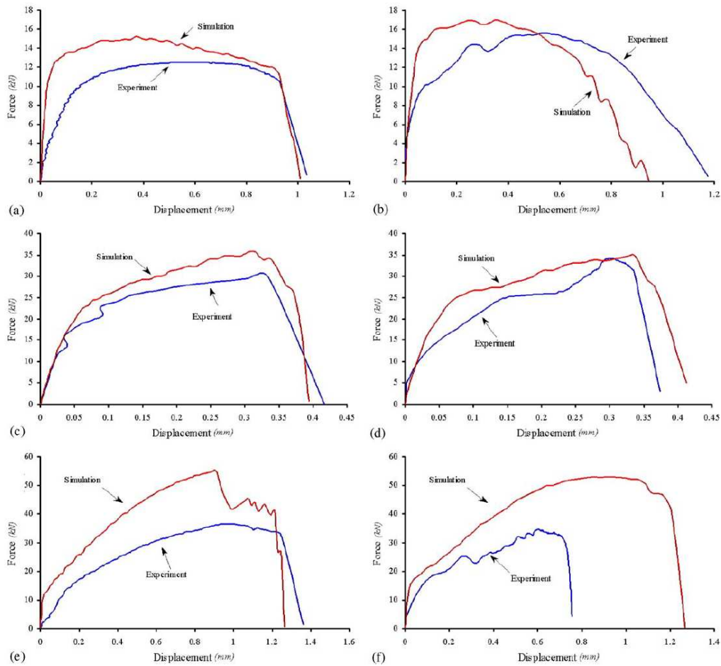
FIG. 1.15 – Courbes comparatives de l'effort de découpe en fonction du déplacement du poinçon pour : l'aluminium en quasi-statique (a) et en dynamique (b) ; le titane en quasi-statique (c) et en dynamique (d) ; et l'acier "nitronic" en quasi-statique (e) et en dynamique (f). (Dabboussi et Nemes, 2004)
