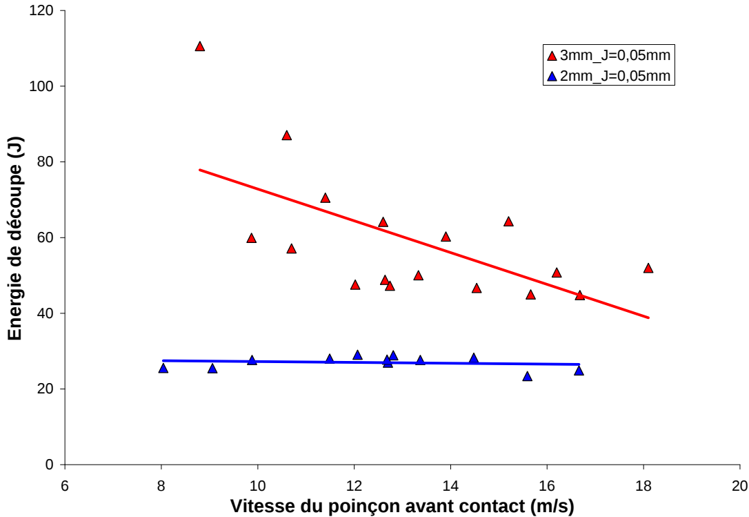
FIG. 5.7 – Evolution de l'énergie consommée par la découpe en fonction de la vitesse du poinçon pour des échantillons de 2 et 3\text{ mm} avec un jeu de 0,05\text{ mm}
