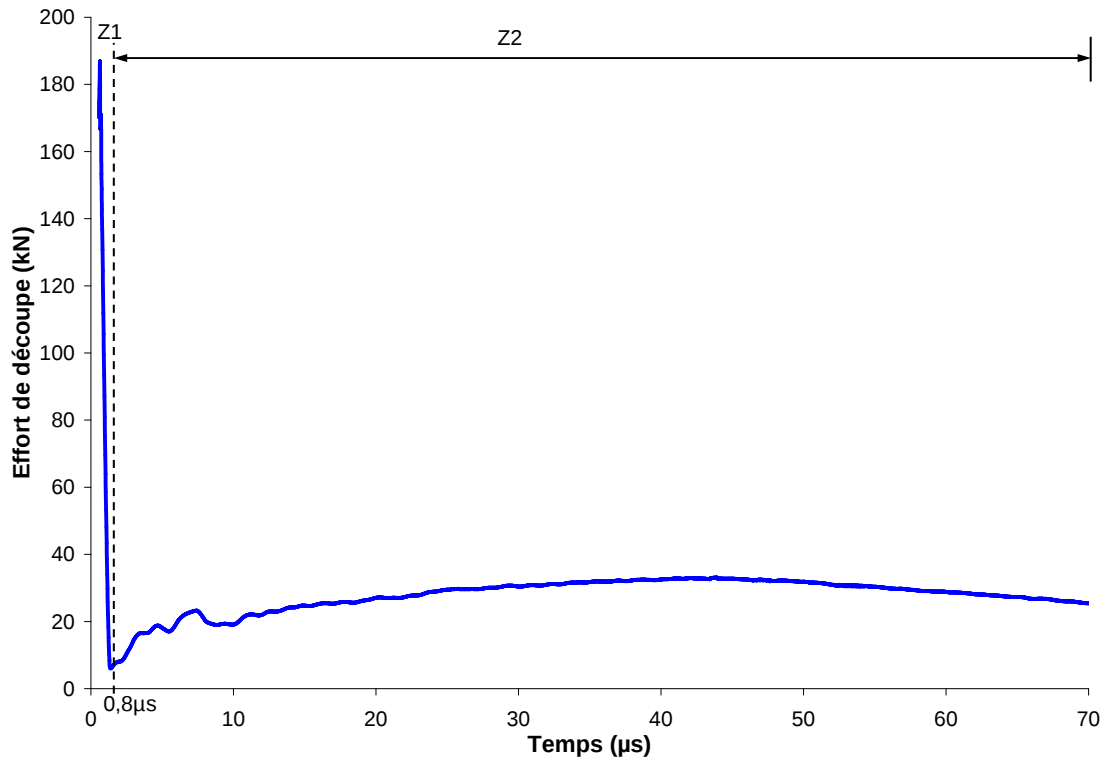
FIG. 4.10 – Effort en fonction du temps pour une simulation numérique en 2D avec une vitesse de poinçon de 15\text{ m/s} , un congé de 200\text{ }\mu\text{m} et une distance entre nœuds de 50\text{ }\mu\text{m}
