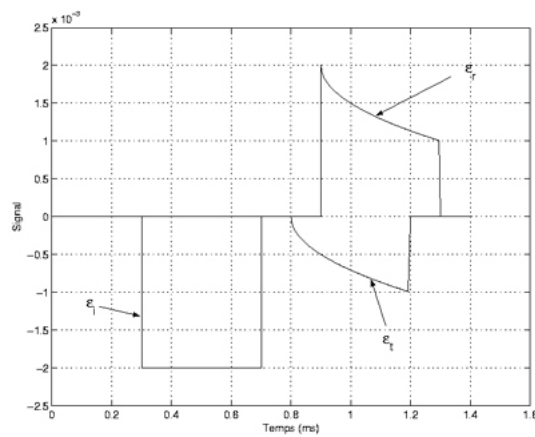
FIG. A.4 – Représentation schématisique des ondes incidente, transmise et réfléchie.
