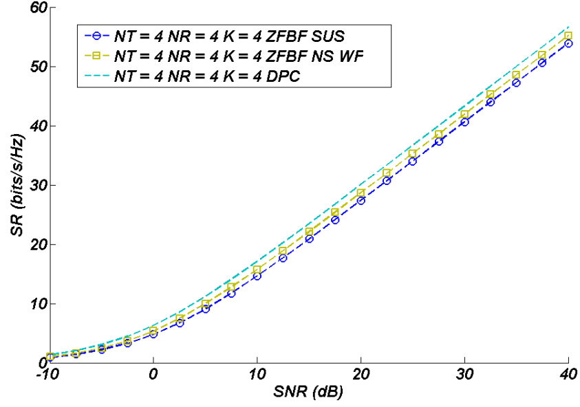
Figure 1.29: Débit total en fonction du SNR pour algorithme avec DPC.
