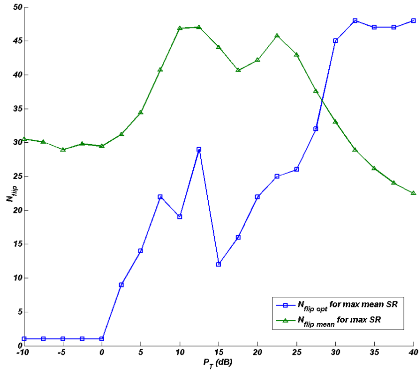
Figure 1.9: N_{flip} optimal en fonction of the SNR pour deux critères pour N_T=N_R=K=4 .
