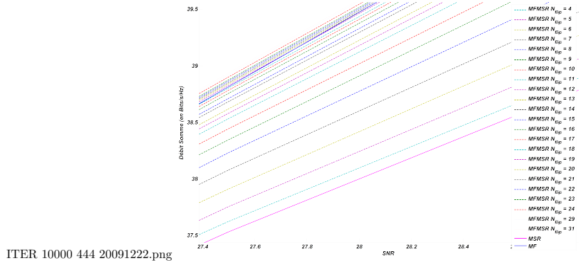
Figure 1.7: Débit total en fonction de SNR et de N_{flip} pour N_T=N_R=K=4 .
