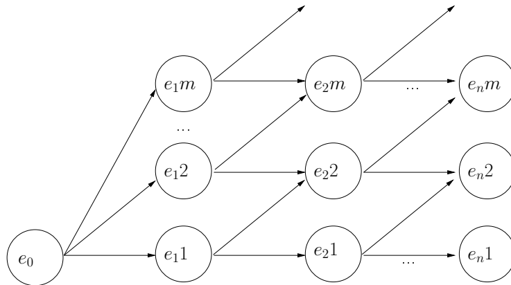
FIGURE 3.16 – Programmation dynamique.
