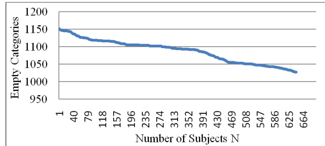
Figure 2. Nombre moyen de categories vides en fonction de N (Feret)
