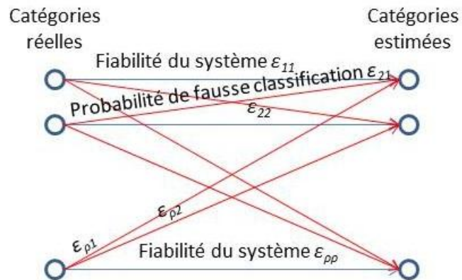
Figure 4. Paramètres de confusion \{\varepsilon_{ij}\}
