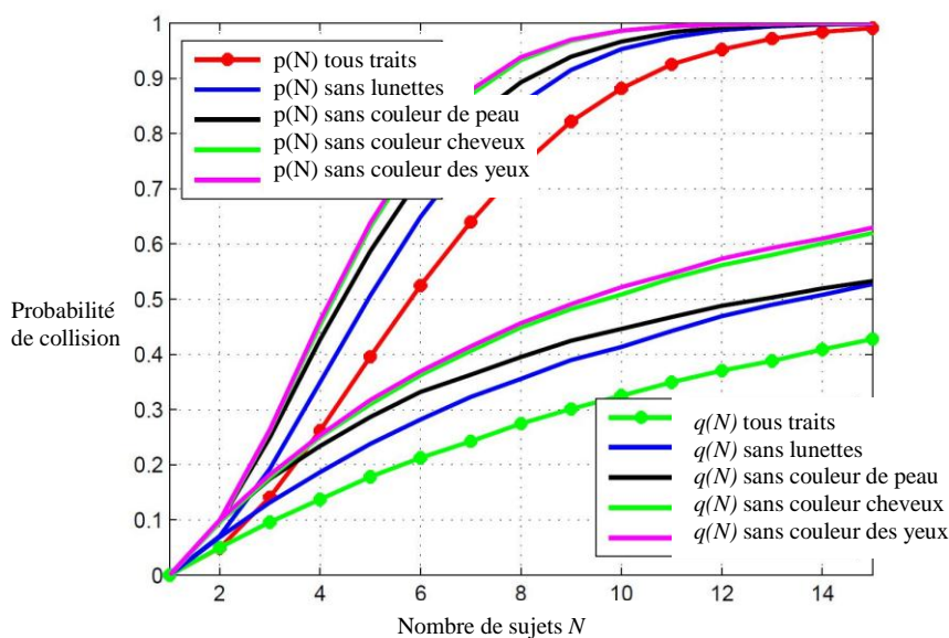
Figure 3. q(N) et p(N) pour une distribution réelle et uniforme
