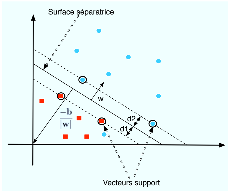
FIG. C.1 – Un cas simple de SVM pour des données presque séparables linéairement
