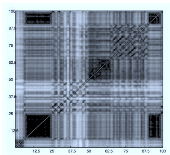
FIG. 3.2 – Un exemple de matrice de similarité. Les deux axes représentent le temps. Les distances entre les trames sont représentées par des niveaux de gris. En l’occurrence les grandes distances sont affectées à un niveau sombre et les faibles distances à un niveau clair.
