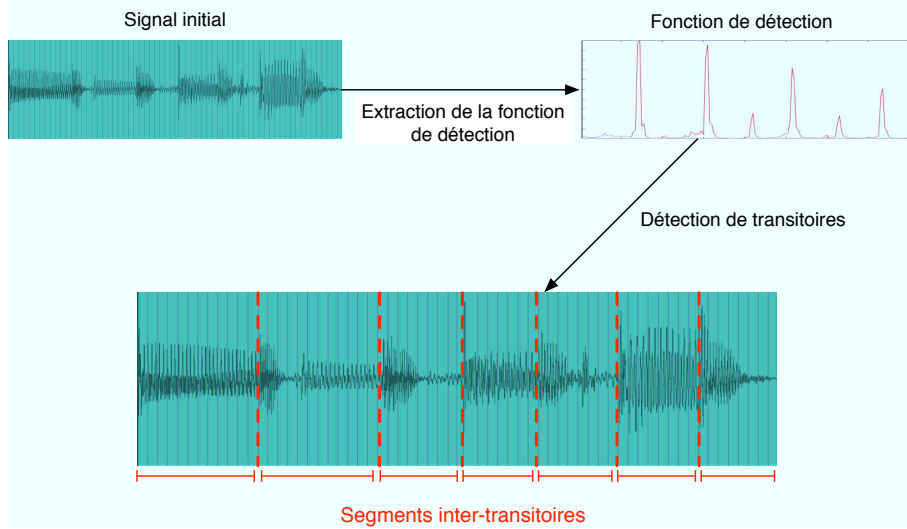
FIG. 3.7 – Détection de transitoires
