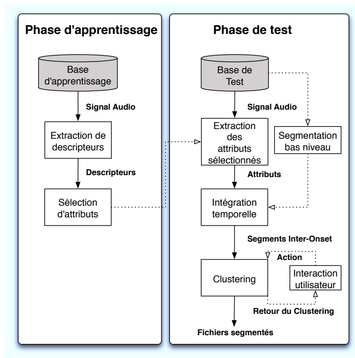
FIG. 3.3 – Architecture du système de segmentation interactif
