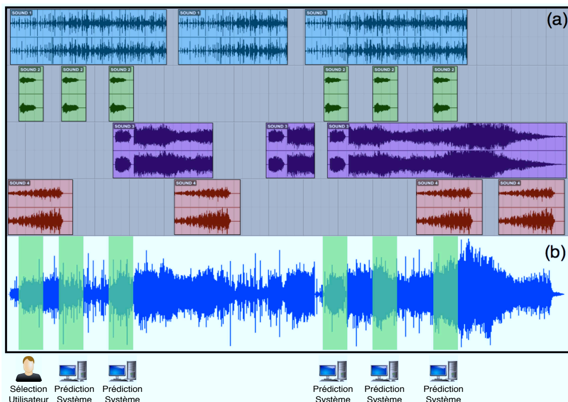
FIG. 2.10 – La figure (a), représente la superposition de diverses sources sonores dans une pièce musicale (un son différent par ligne/couleur), comme c'est le cas dans une pièce électroacoustique polyphonique. La figure (b) est le mixage résultant de toutes les sources sonores, lors de l'analyse nous n'avons accès qu'à ce mélange de sources. Le système doit pouvoir prédire les différentes instances d'un objet donné (en l'occurrence le son vert) à partir de l'instance de la sélection utilisateur.
