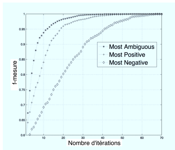
FIG. 4.7 – f - mesure en fonction du nombre d'itérations pour 3 stratégies d'échantillonnage
