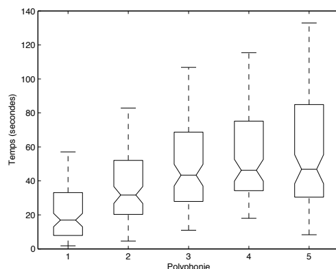
FIG. 4.12 – Temps d’attente total pour l’annotation d’un fichier avec la méthode PU2 en fonction du niveau de polyphonie
