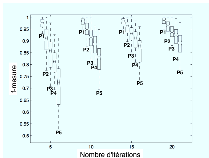
FIG. 4.9 – Score de f-mesure pour l’annotation d’une classe en fonction du nombre d’itérations pour une approche par passages multiples sur les 5 niveaux de polyphonie
