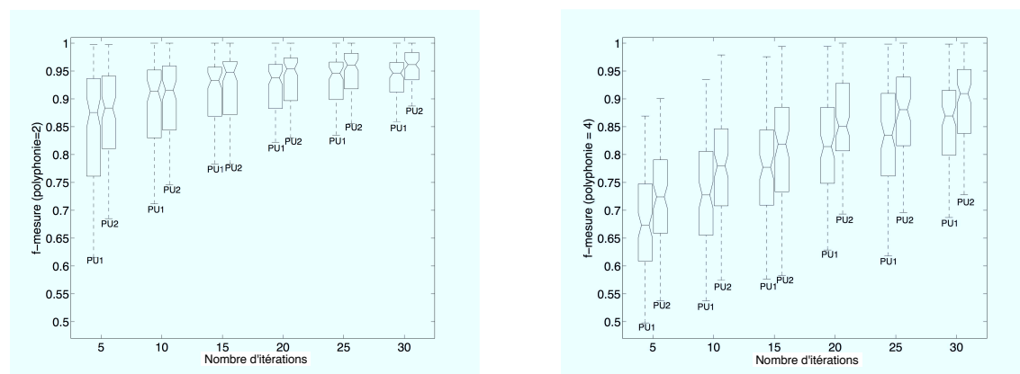
FIG. 4.10 – Score de f-mesure pour l'annotation d'une pièce complète en fonction du nombre d'itérations pour les deux méthodes par passage unique (la figure de gauche présente les résultats pour un degré de polyphonie de 2 et celle de droite pour un degré de polyphonie de 4).
