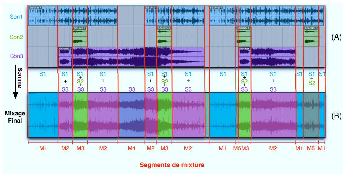
FIG. 3.1 – Segmentation d'un mixage sonore en segments de mixture
