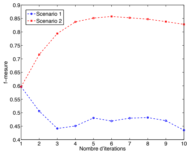
FIG. 3.12 – Comparaison de performances pour deux scénarios d'interaction
