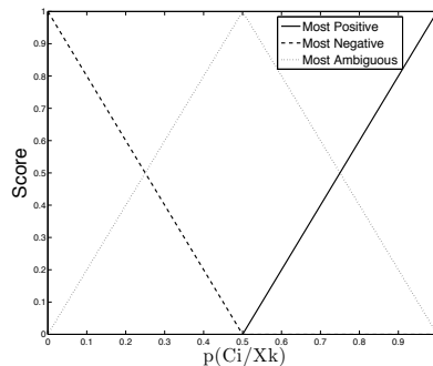
FIG. 4.6 – Courbes de calcul des scores d'utilités pour différentes stratégies
