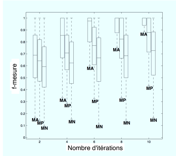
FIG. 4.8 – Comparaison de performances détaillées pour les premières itérations
