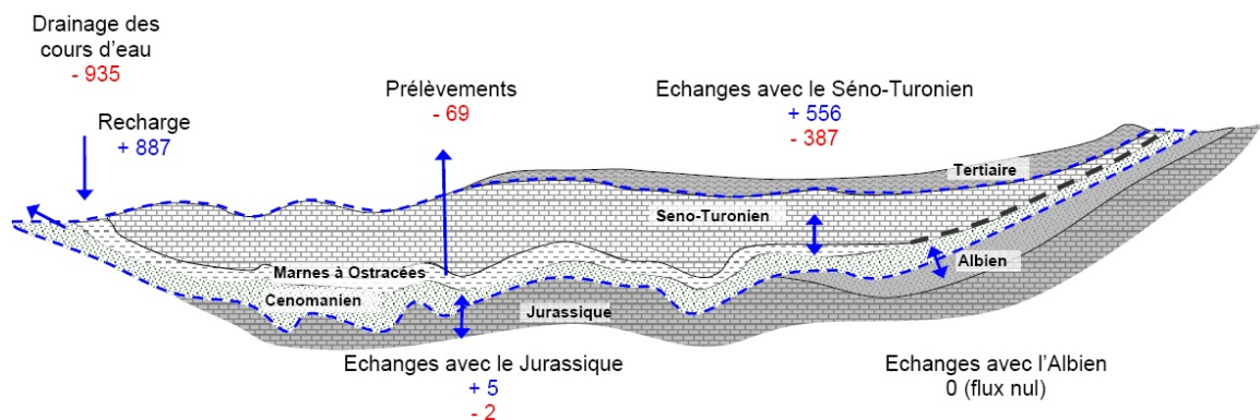
FIGURE 2.11 – Bilans des volumes échangés par le système aquifère du Cénomaniens en régime permanent, en Mm 3 .an -1 (Sogreah, 2006b)
