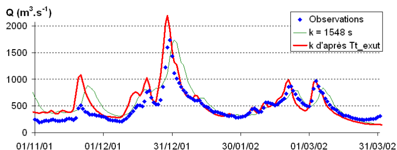
FIGURE 5.4 – Exemple de l'influence de k sur le débit simulé à Gien.
