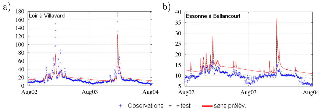
FIGURE 9.12 – Exemples de débits simulés pour une simulation ne prenant pas en compte les prélèvements en nappe (en \text{m}^3 \cdot \text{s}^{-1} ) : a) le Loir à Villavard, b) l'Essonne à Ballancourt. Les stations sont localisées à la figure 6.10a (p. 81).
