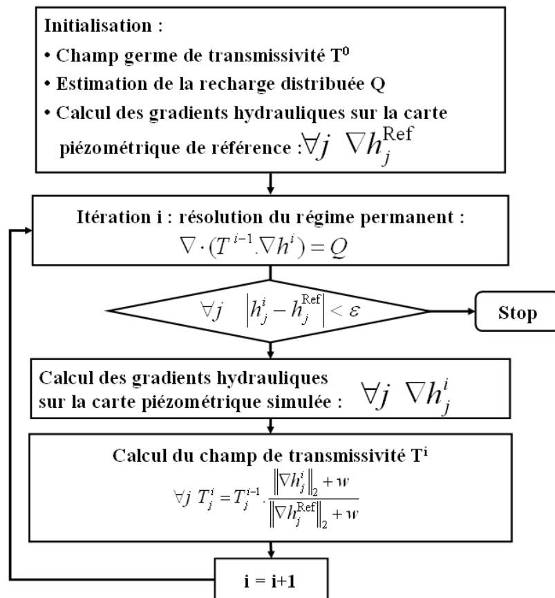
FIGURE 6.6 – Algorithme de l'inversion (Pasquier, 2005) : h^{Ref} correspond à la piézométrie de référence, h^i à la piézométrie à l'itération i , T^i est le champ de transmissivités de l'itération i , T_j^i : la valeur de la transmissivité de la maille j et w un paramètre d'amortissement.
