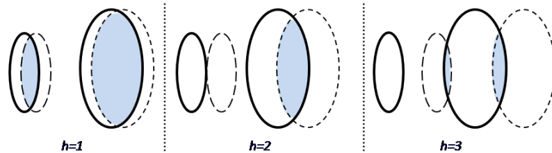
Figure 22 : Principe de calcul de la covariance : pour chaque pas de translation ( h ), la covariance est donnée par l'intersection des phases de l'image d'origine (traits pleins) et de l'image traduite (traits pointillés)
