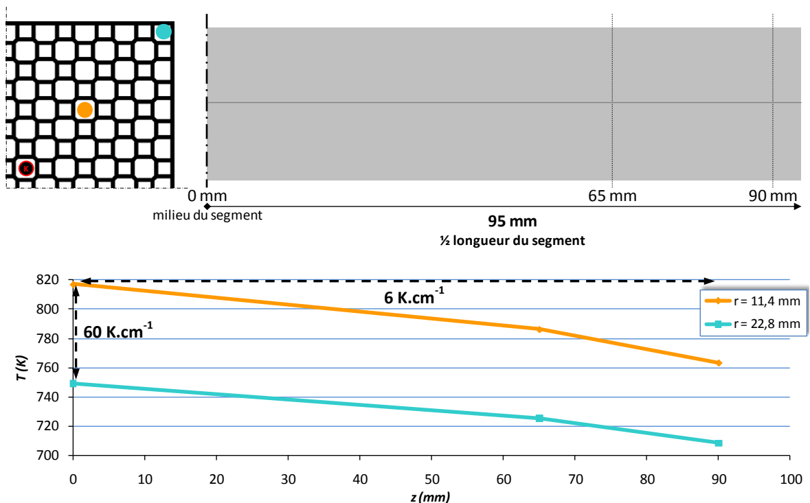
Figure 69 : Températures mesurées en configuration C pour deux positions radiales et trois positions axiales dans le segment à une puissance de 0,87 \text{ W.mm}^{-1}
