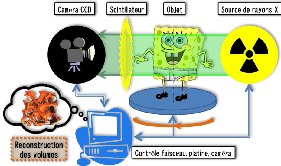
Figure 19 : Principe d'obtention des images 3D en microtomographie par rayons X
