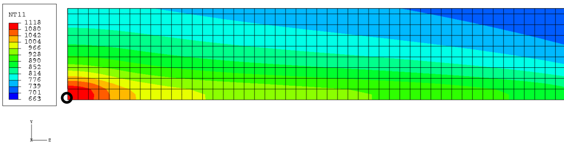
Figure 116 : Carte des températures à rupture (K) simulée en configuration CC (vue intérieure, le cercle noir correspond au barycentre du segment)
