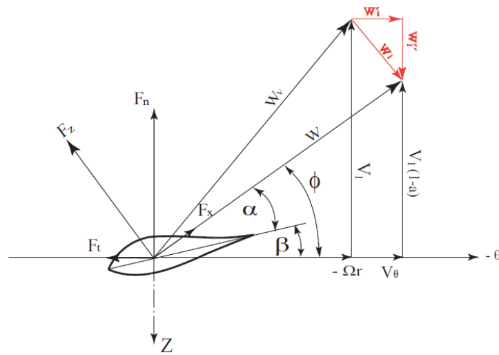
Fig. 2.6 Forces agissant sur un élément de pale
