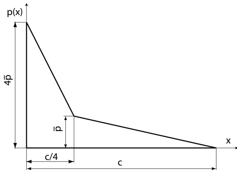
Fig. 6.1 Distribution de pression simplifiée
