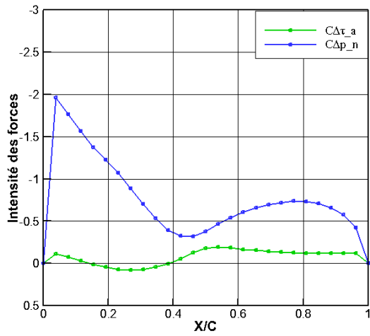
Angle d'incidence 20°
