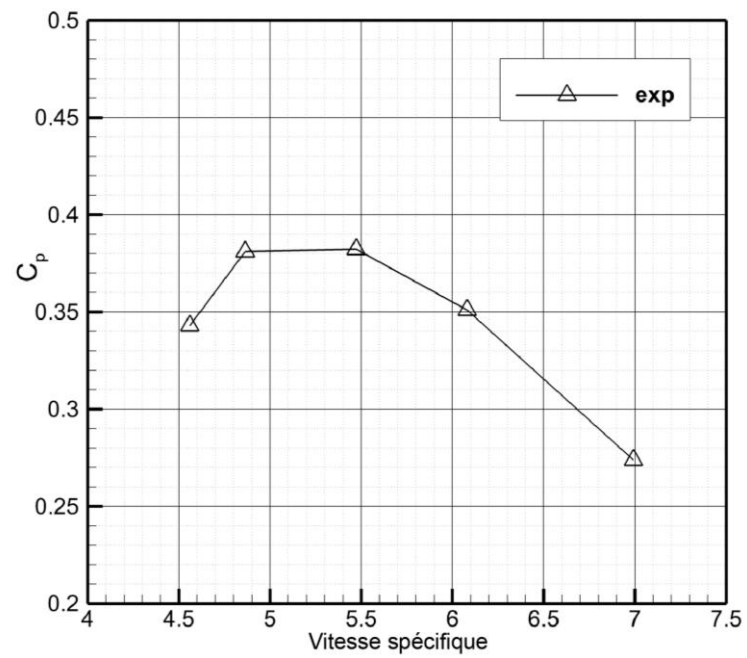
Fig. 5.7 Coefficient de puissance en fonction de la vitesse spécifique
