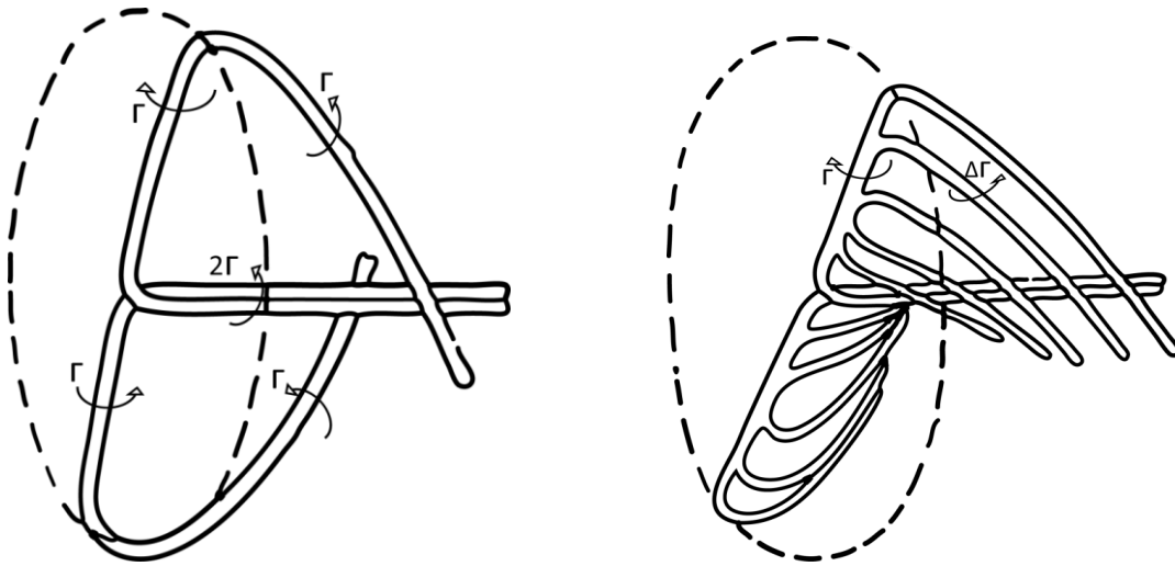
Fig.2.7 Système tourbillonnaire du rotor
