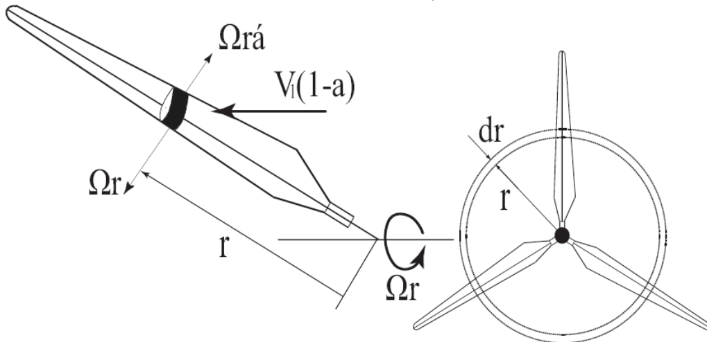
Fig. 2.3 Coupe élémentaire de pale et l'anneau balayé
