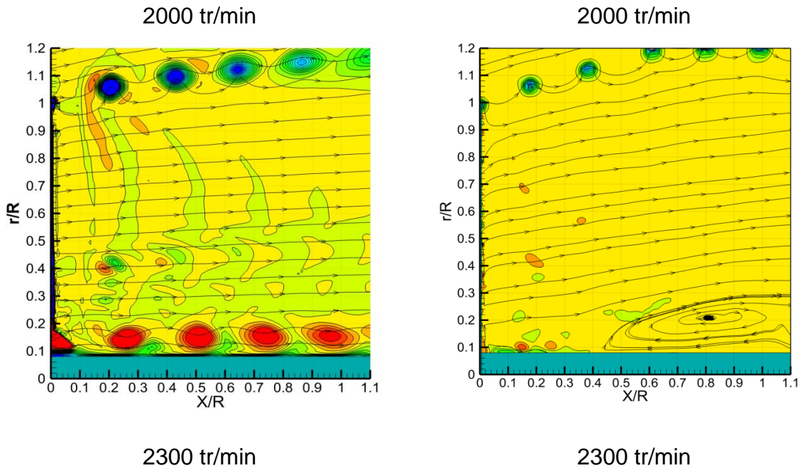
Fig.6.9 Vorticité à plusieurs vitesses de la rotation issues du calcul (à gauche) et d'essais expérimentaux (à droite)
