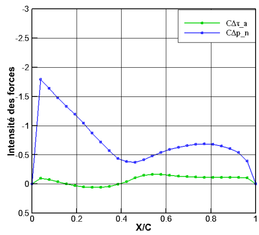
Angle d'incidence 24°
