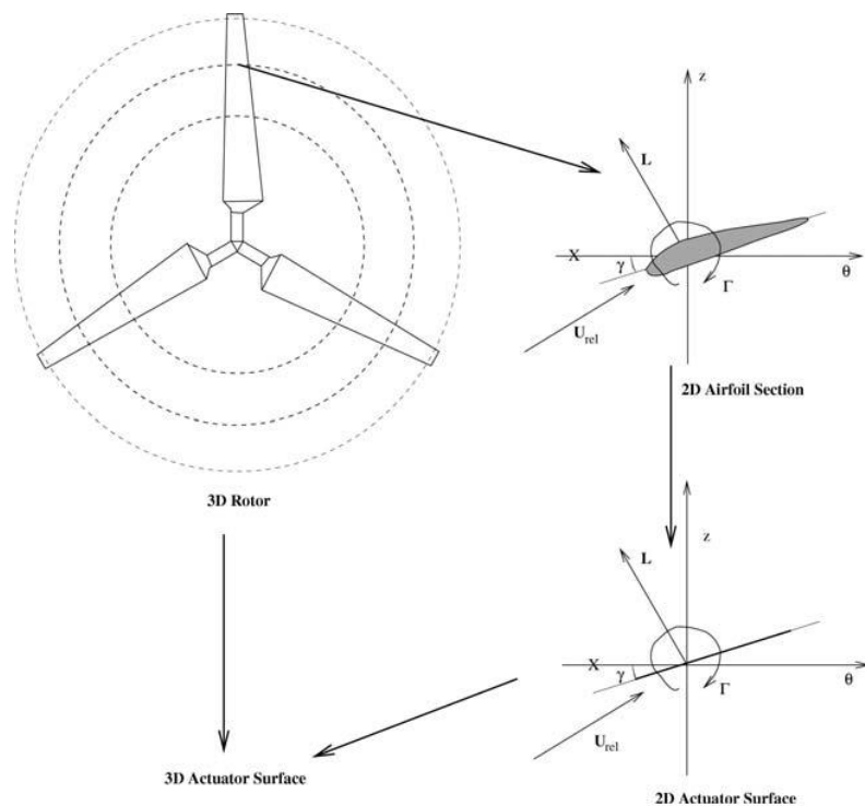
Fig. 3.9 Représentation schématique de la modélisation hybride de la surface active [80]
