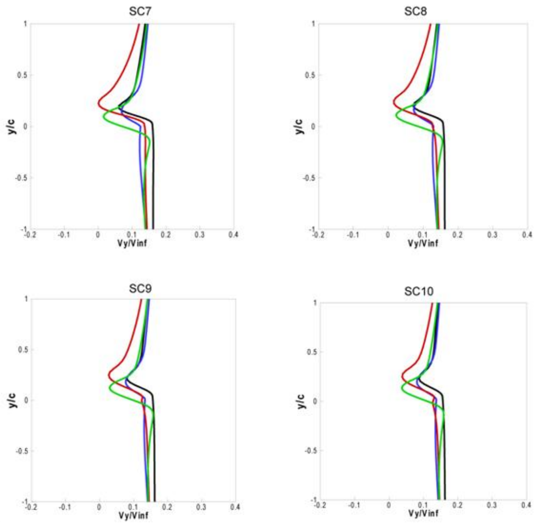
Fig. B.1 (b) Comparaison des calculs du sillage - vitesse normale à la corde- profil S809 - \alpha = 10^\circ
