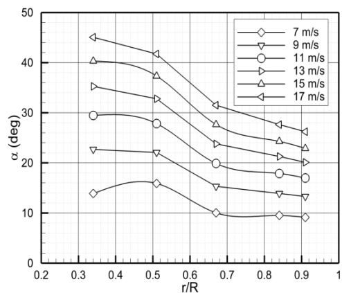
Fig. 3.16 La répartition de l'angle d'incidence le long de la pale
