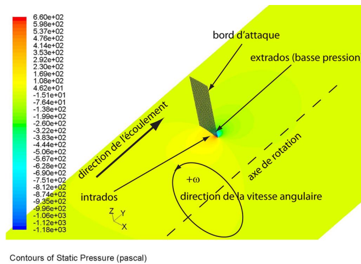
Fig.6.4 Contours de pression statique
