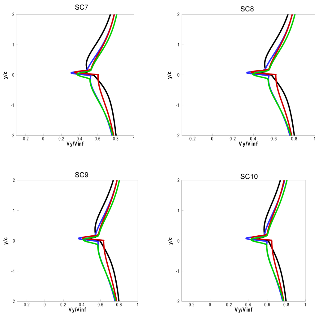
Fig. 4.13 (b) Comparaison des calculs du sillage - vitesse normale à la corde - profil S809 - \alpha = 5^\circ
