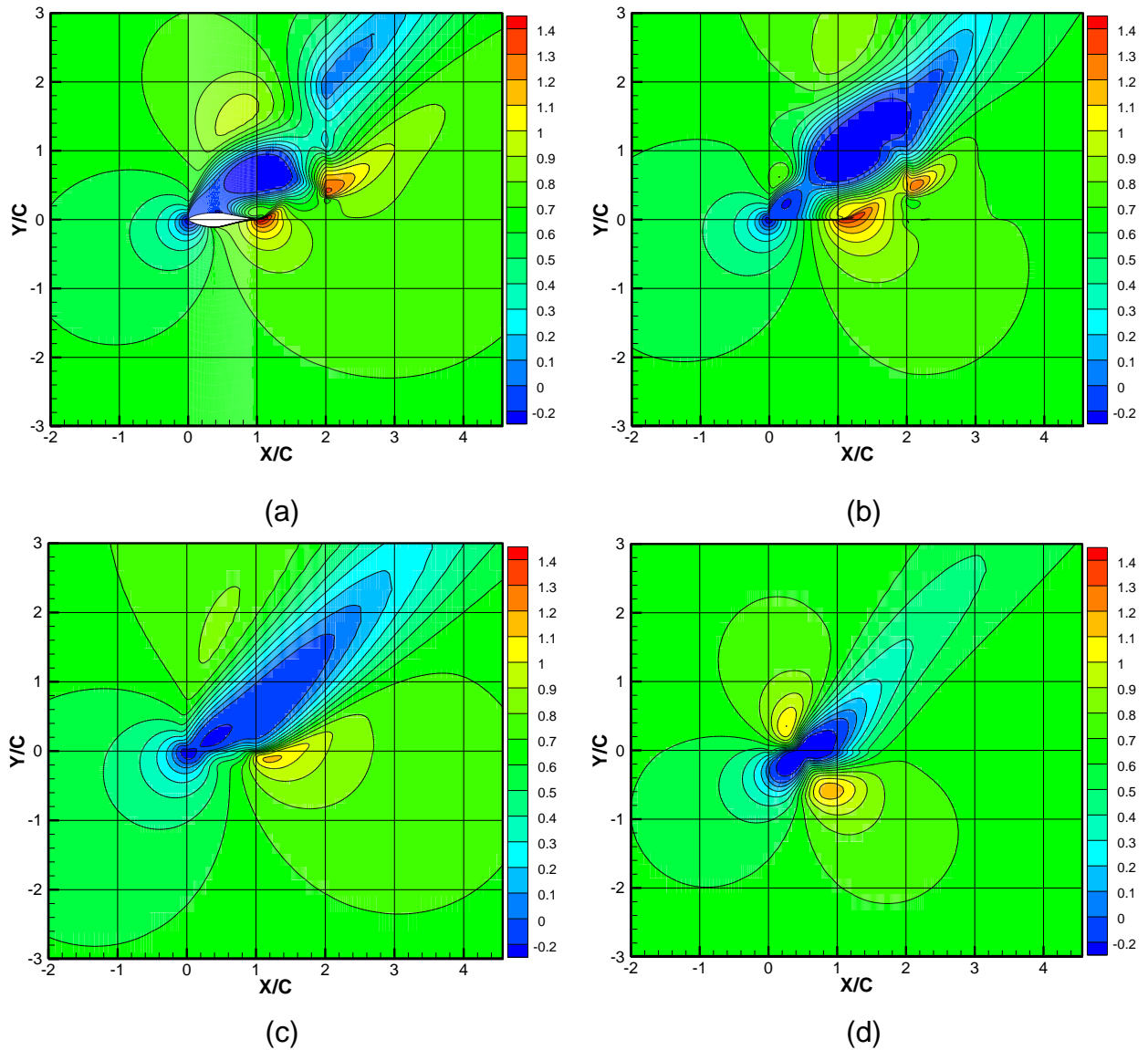
Fig. A.1 Champ de vitesse \alpha=50^\circ : (a) profil S809 ; (b) nouveau modèle proposé ; (c) cas de la surface active ; (d) cas de la ligne active
