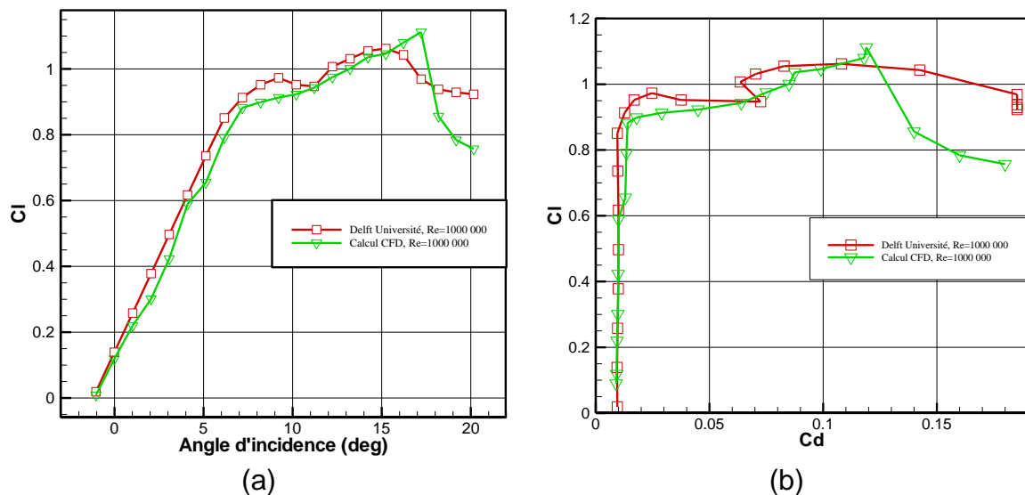
Fig. 4.3 Simulations numériques et résultats d'essais de l'Université de Delft : (a) portance en fonction de l'angle d'incidence; (b) portance en fonction de la traînée.
