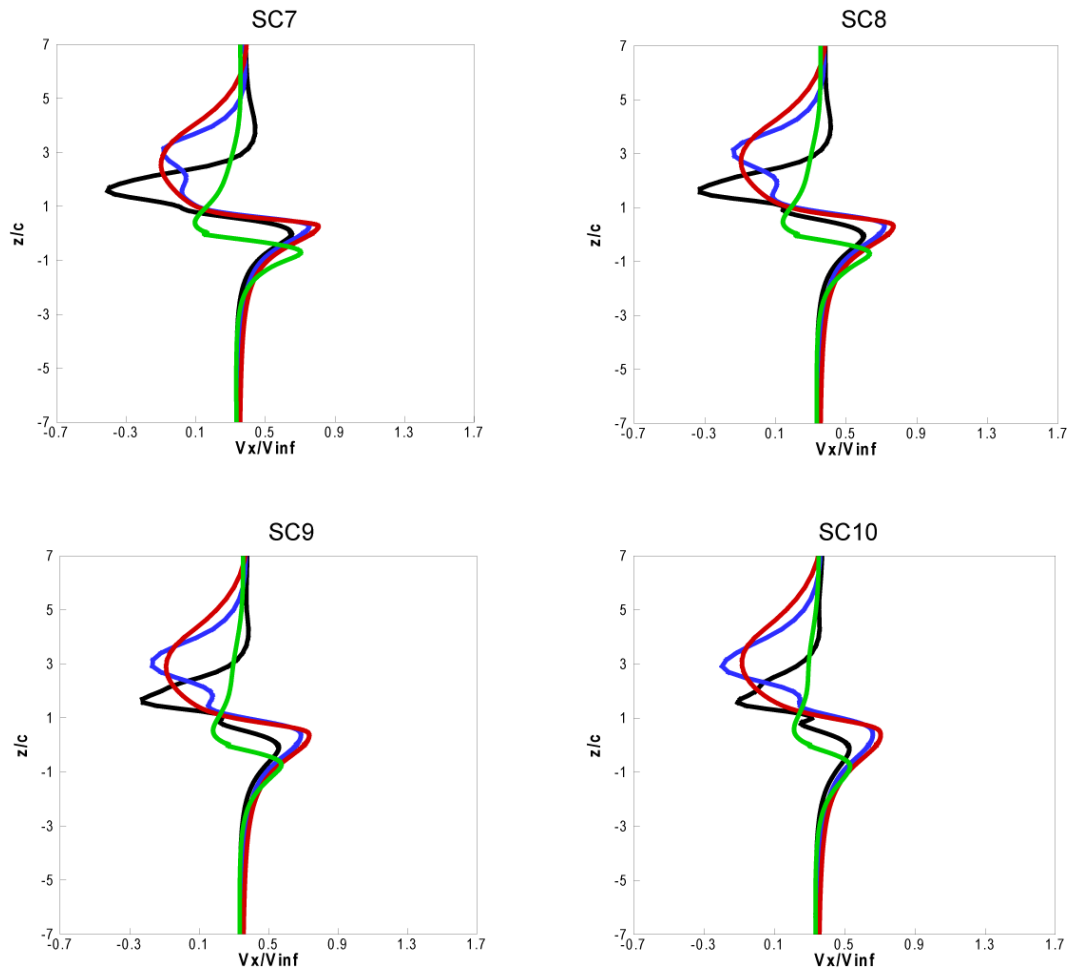
Fig. B.5 (a) Comparaison des calculs du sillag - vitesse le long de la corde-profil S809 - \alpha=70^\circ
