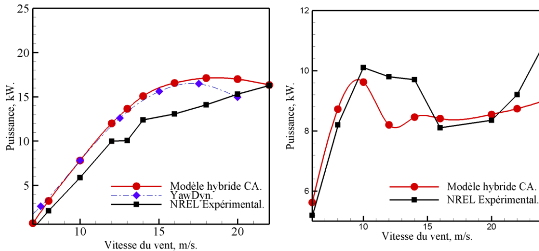
Fig. 3.6 Comparaison du calcul de la puissance par le modèle de cylindre actif avec les essais d'éoliennes NREL phase II (gauche) et phase VI (droite) [41]
