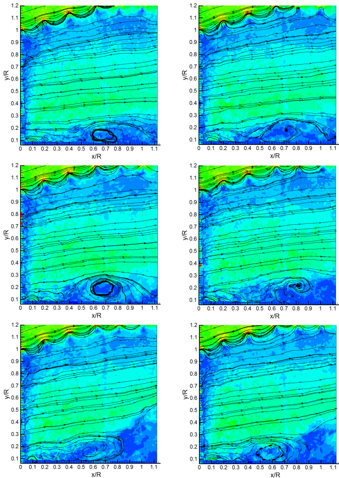
Fig.5.9 Champs d'écoulement instantané à différents instants.
