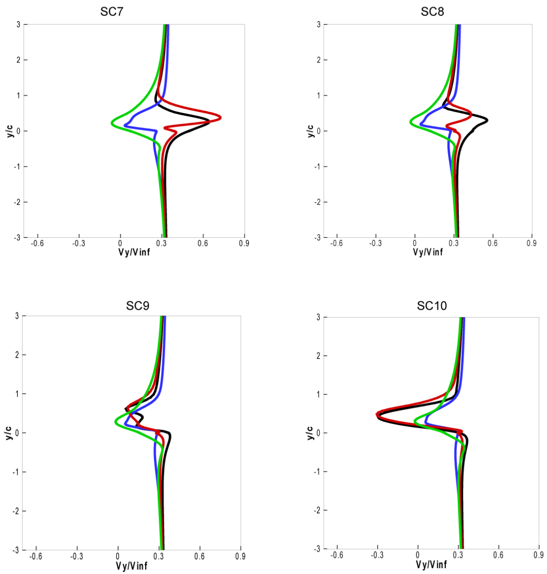
Fig. 4.14 (b) Comparaison des calculs du sillage - vitesse normale à la corde- profil S809 - \alpha = 20^\circ
