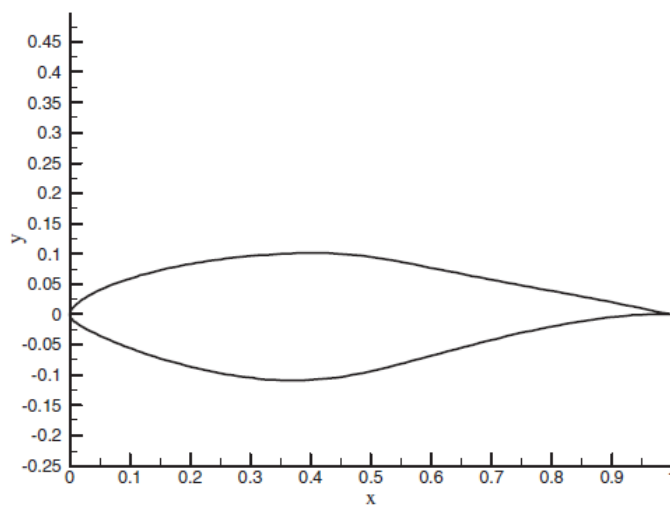
Fig. 4.1: Profil NREL S809
