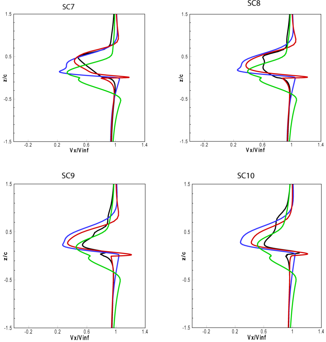
Fig. 4.14 (a) Comparaison des calculs du sillage - vitesse le long de la corde-profil S809 - \alpha=20^\circ
