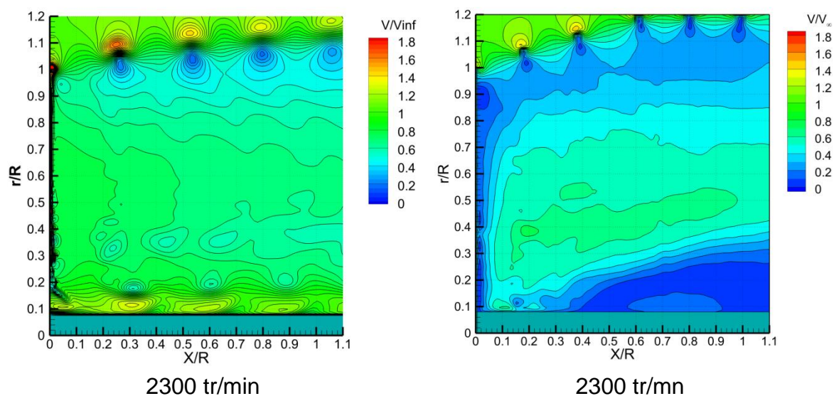
Fig.6.8 Tourbillons marginaux aux vitesses de la rotation, issus du calcul (à gauche) et d'essais expérimentaux (à droite)
