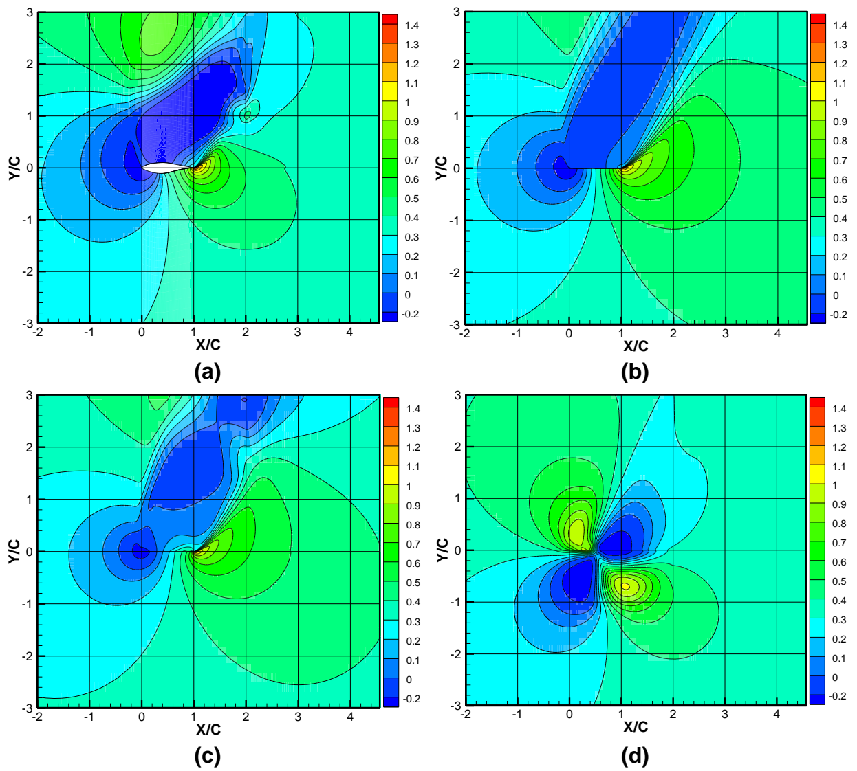
Fig. A.2 Champ de vitesse \alpha=70^\circ : (a) profil S809 ; (b) nouveau modèle proposé ; (c) cas de la surface active ; (d) cas de la ligne active
