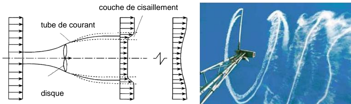
Fig.1.3 Représentation schématique du déficit de vitesse (à gauche) et visualisation du sillage éolien (à droite) [92]
