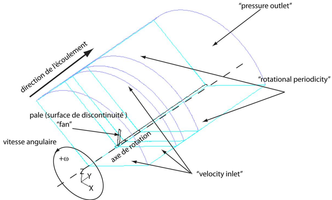
Fig. 6.2 Domaine de calcul et conditions aux limites
