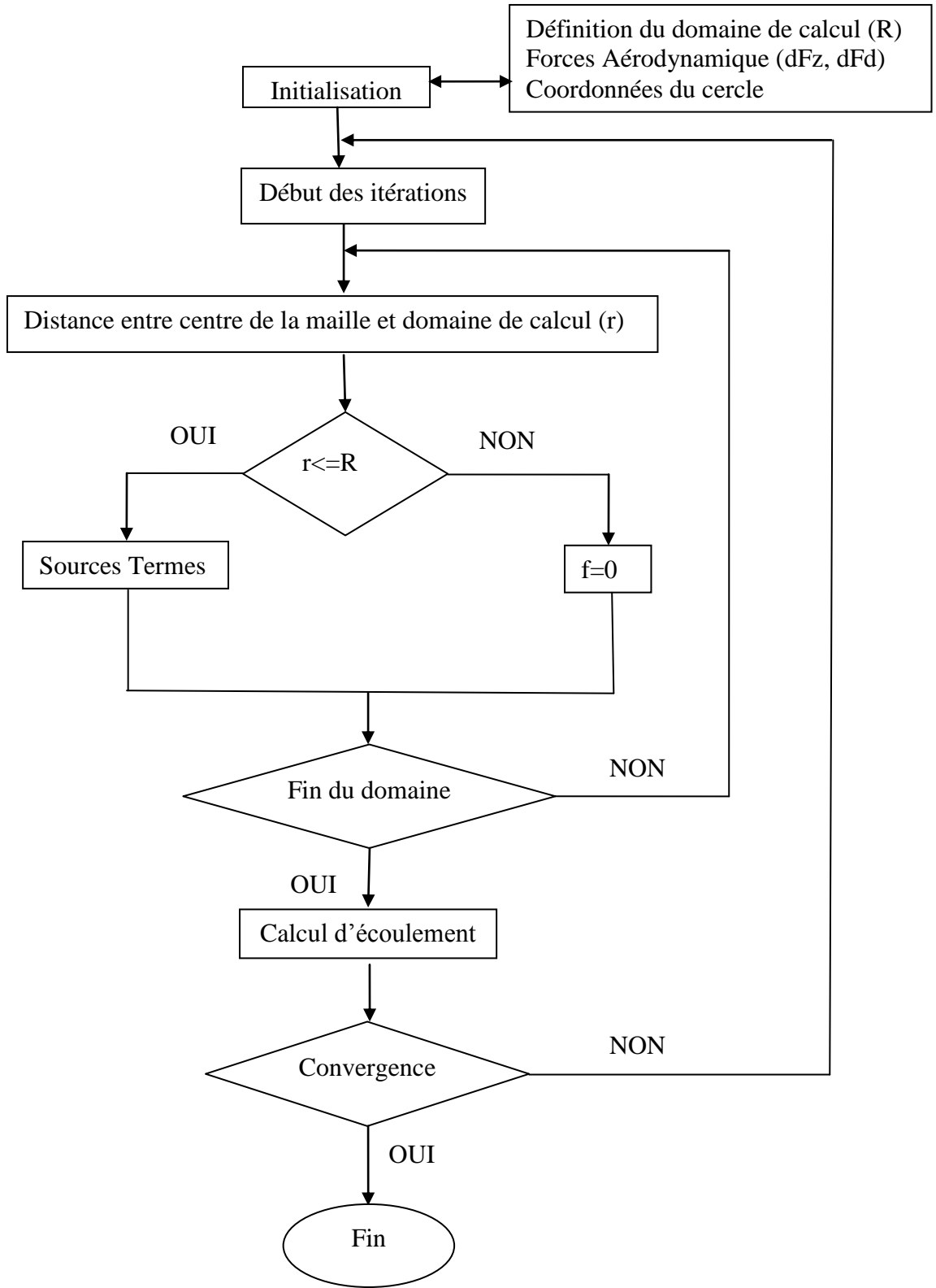
Fig. 4.5 Organigramme du modèle hybride de ligne actif
