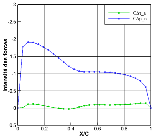
Angle d'incidence 40°
