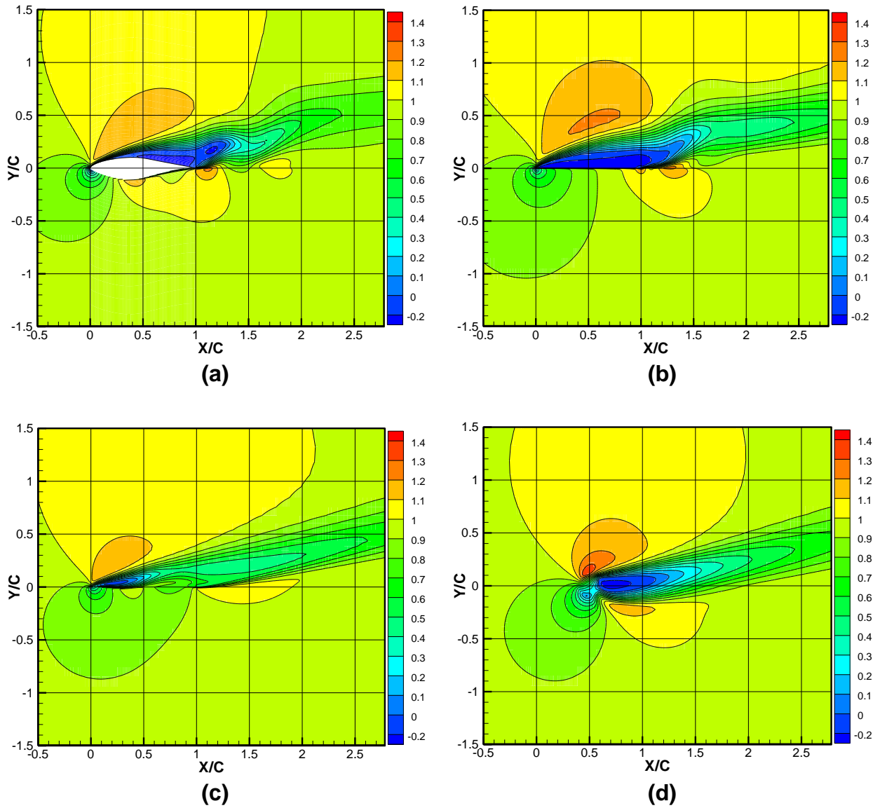
Fig. 4.9 Champ de vitesse \alpha=15^\circ : (a) profil S809 ; (b) nouveau modèle proposé ; (c) cas de la surface active ; (d) cas de la ligne active
