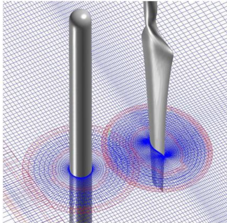
Fig. 2.9 Le maillage autour de la tour, de la pale et le champ lointain [91]
