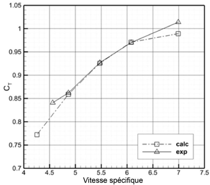
Fig. 6.12 Coefficient de poussée en fonction de vitesse spécifique
