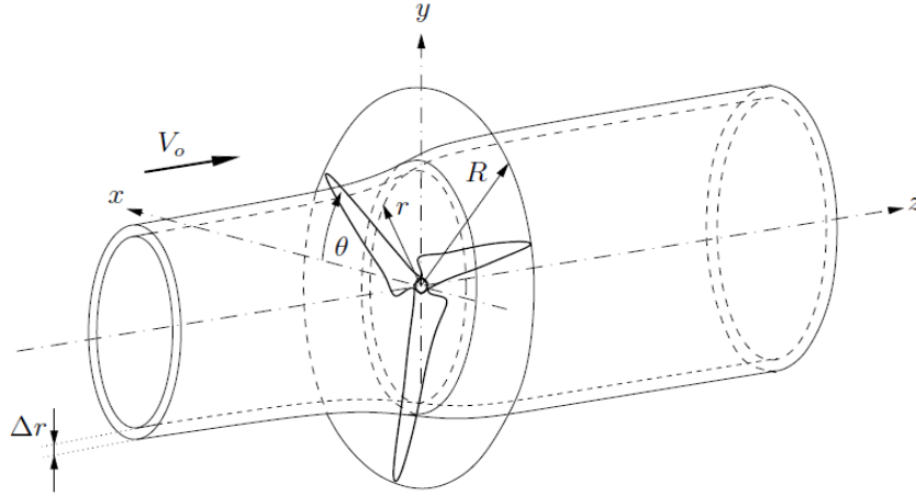
Fig. 3.1 Concept du disque actif
