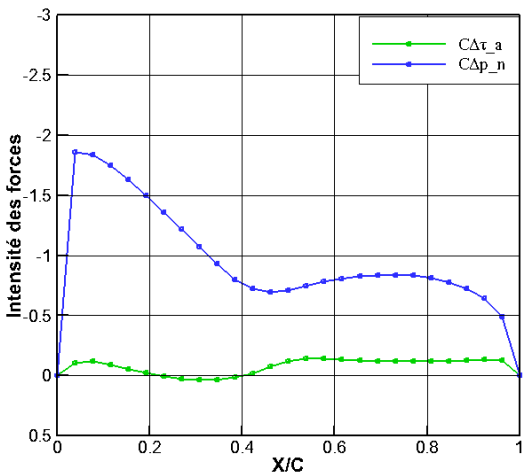
Angle d'incidence 30°
