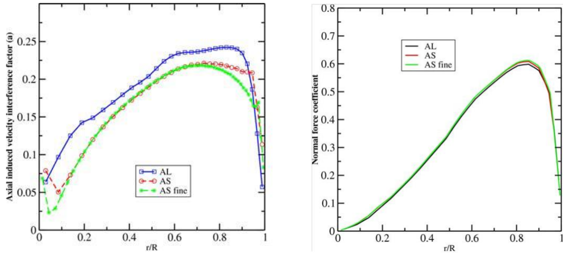
Fig.3.10 (a) la vitesse axiale induite (b) la force normale le long de pale [80]
