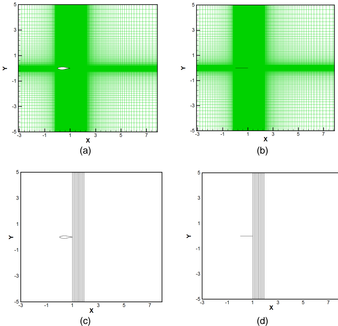
Fig. 4.2 Maillage et lignes de contrôle (a; c) profil S809 (b, d) coupe normale à la surface active
