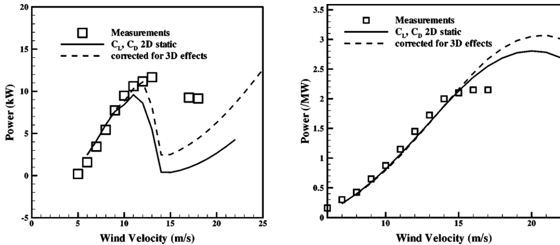
Fig. 3.3 Comparaison de puissance de modèle hybride du disque actif et les données expérimentales, NREL phase IV (à gauche) et Tjaereborg turbine (à droite) [78]
