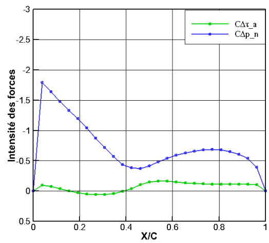
Angle d'incidence 24°
