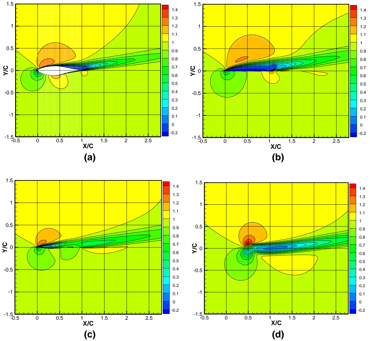
Fig. 4.8 Champ de vitesse \alpha=10^\circ : (a) profil S809 ; (b) nouveau modèle proposé ; (c) cas de la surface active ; (d) cas de la ligne active
