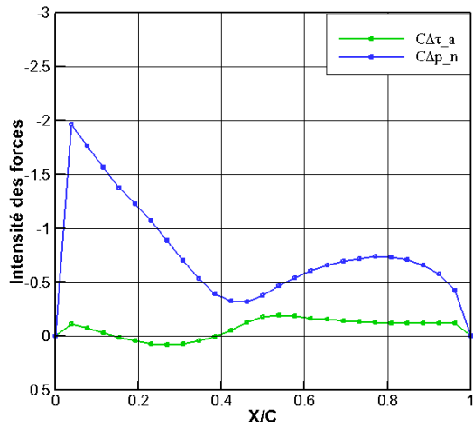
Angle d'incidence 20°
