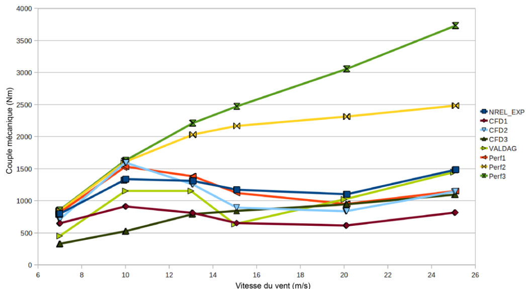
Fig. 1.4 Comparaison des méthodes de simulation avec les essais de l'éolienne NREL-Phase VI [6]
