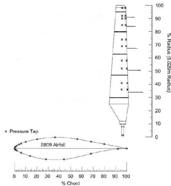
Fig.3.13 Pale instrumentée avec des capteurs de pression et les tubes de Pitot à cinq trous [76]
