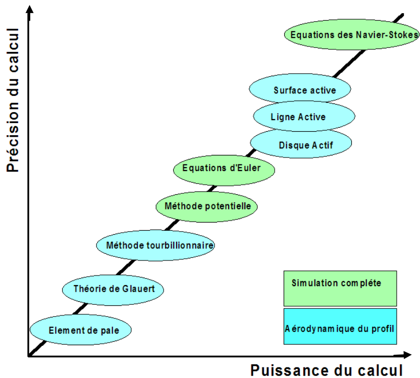
Fig. 2.10 Comparaison des différentes méthodes de modélisation des éoliennes par rapport à la puissance et la précision du calcul
