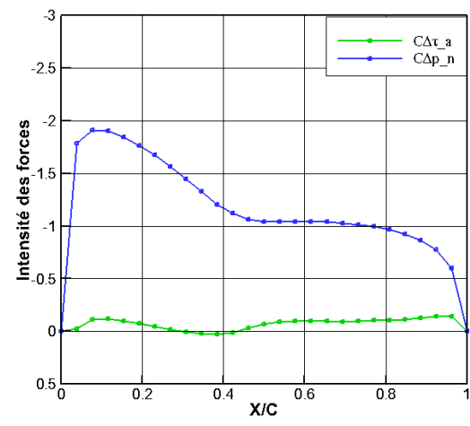
Angle d'incidence 39°
