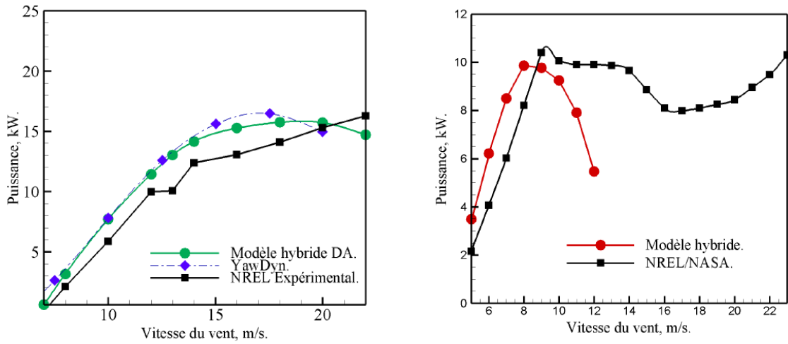
Fig. 3.2 Comparaison des puissances entre le modèle hybride de Disque actif et les données expérimentales, NREL phase II (à gauche) et NREL phase VI (à droite) [41]
