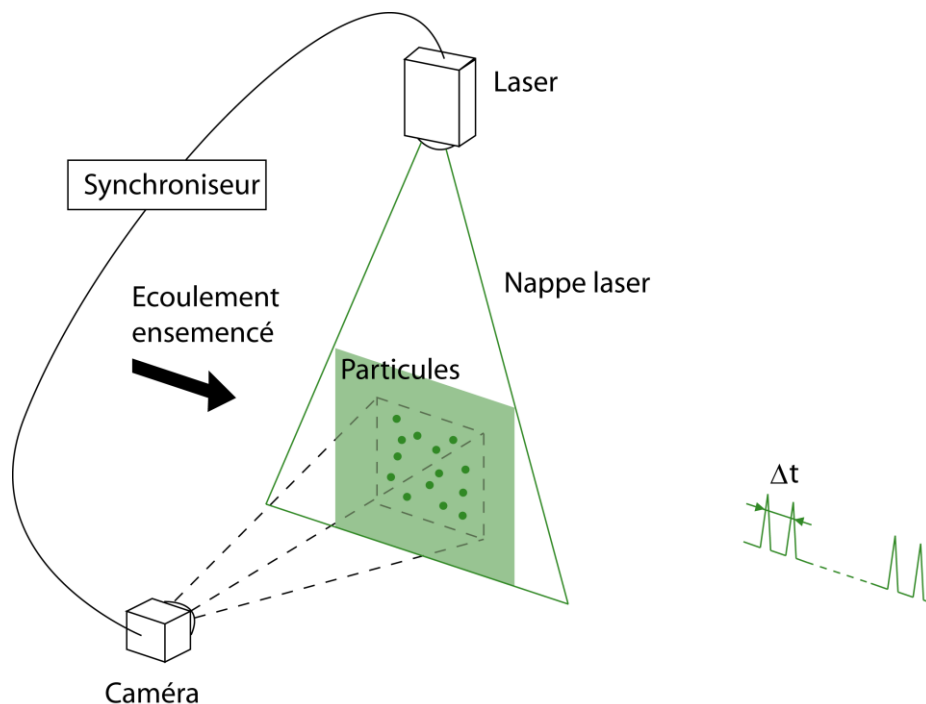
Fig. 5.1 Schéma d'un montage PIV
