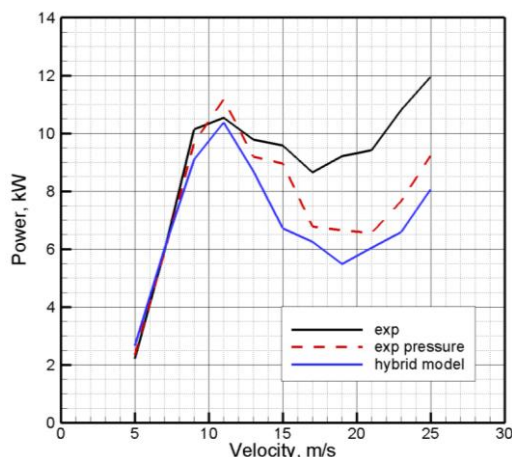
Fig.3.8 Puissance mesurée de l'éolienne NREL Phase VI et simulée à l'aide de surface active [83]
