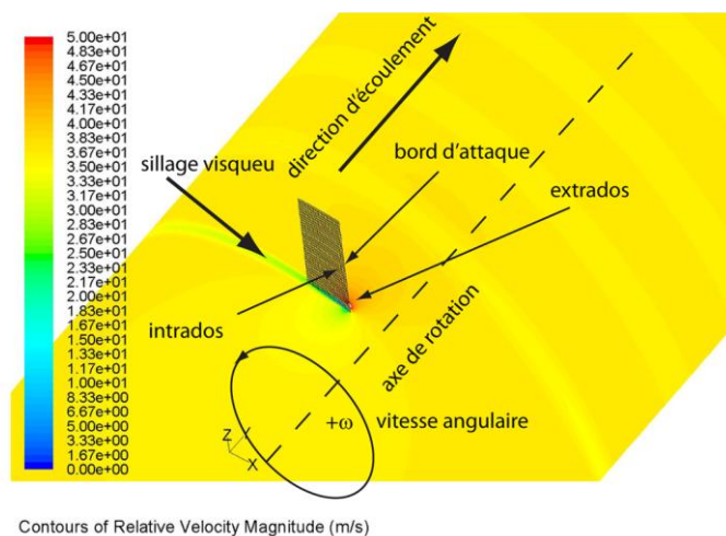
Fig.6.5 Calcul du modèle hybride et sillage visqueux de la pale
