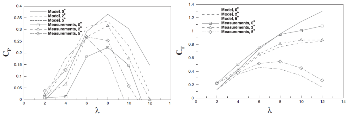
Fig.3.11 coefficient de (a) puissance (b) poussée, en fonction de \lambda [81]
