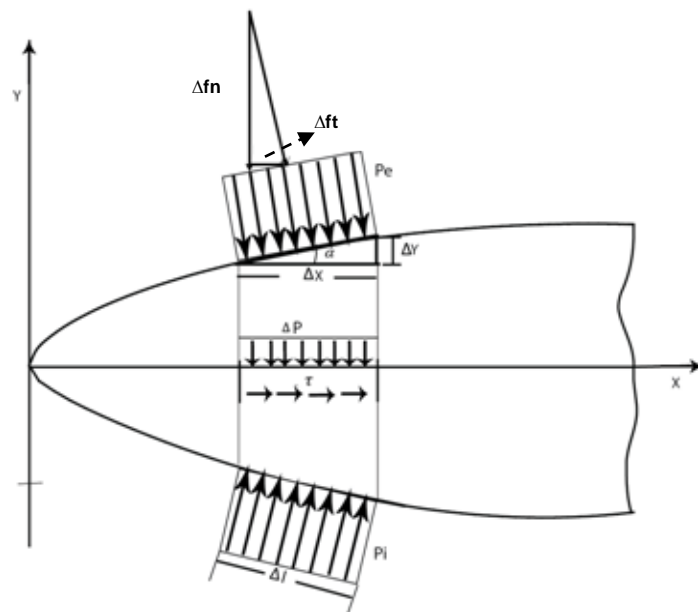
Fig. 4.7. Répartition des forces normales et tangentielles sur le profil
