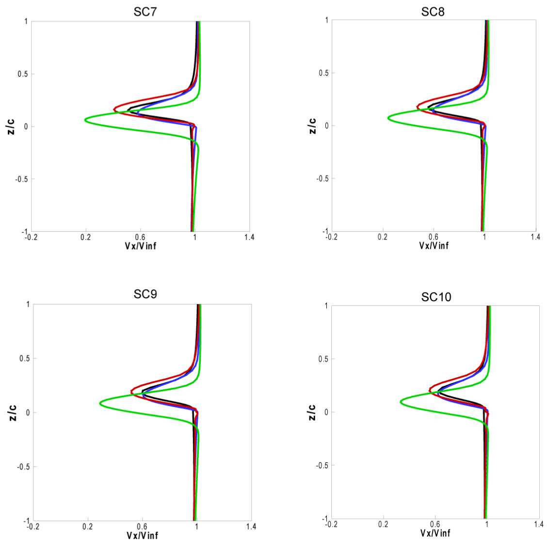
Fig. B.1 (a) Comparaison des calculs du sillage- vitesse le long de la corde-profil S809 - \alpha=10^\circ
