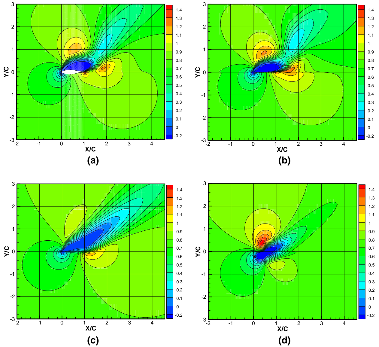
Fig. 4.12 Champ de vitesse \alpha-40 : (a) profil S809 ; (b) nouveau modèle proposé; (c) cas de la surface active ;(d) cas de la ligne active
