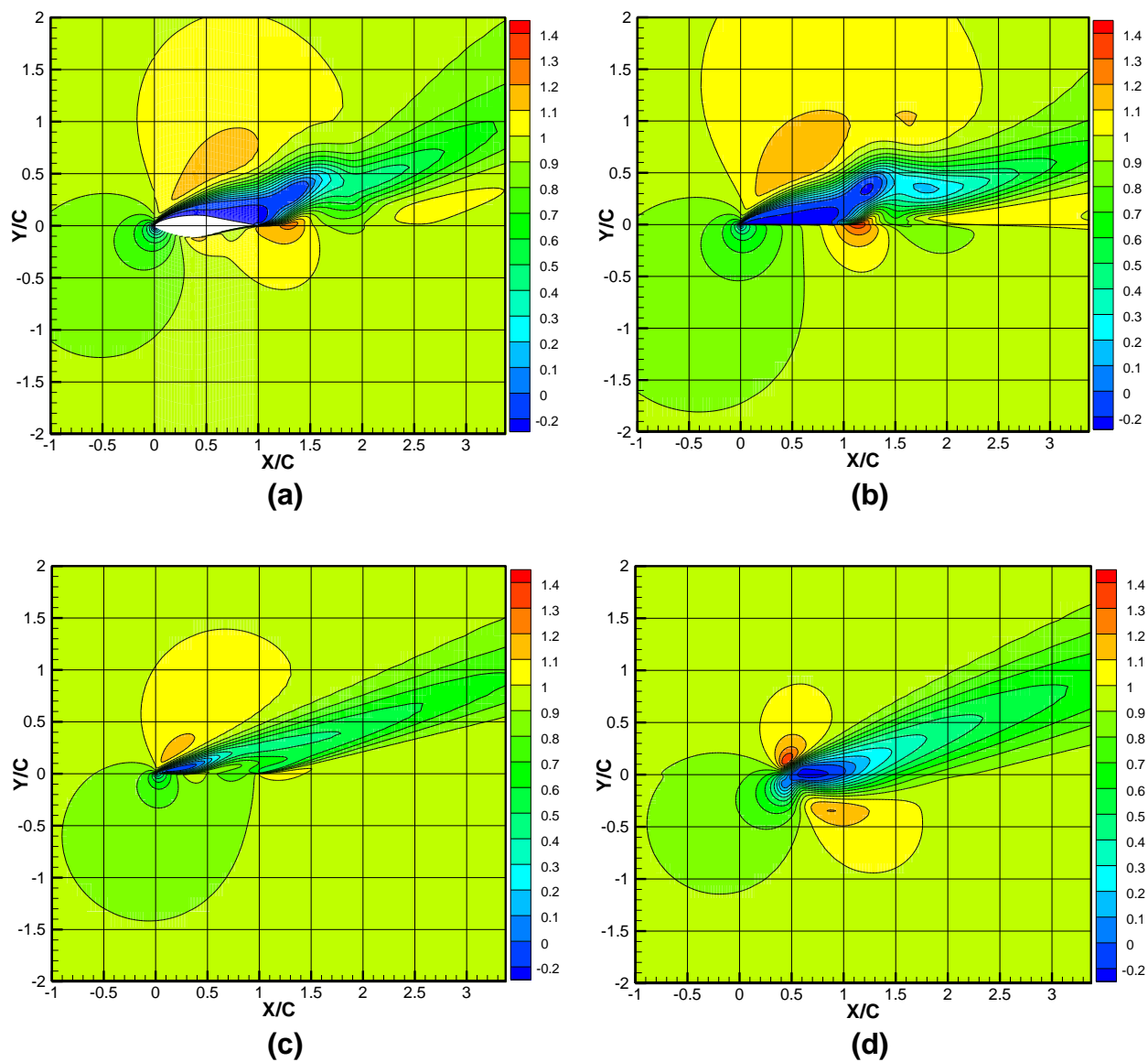
Fig. 4.10 Champ de vitesse \alpha=20^\circ : (a) profil S809 ; (b) nouveau modèle proposé ; (c) cas de la surface active ; (d) cas de la ligne active
