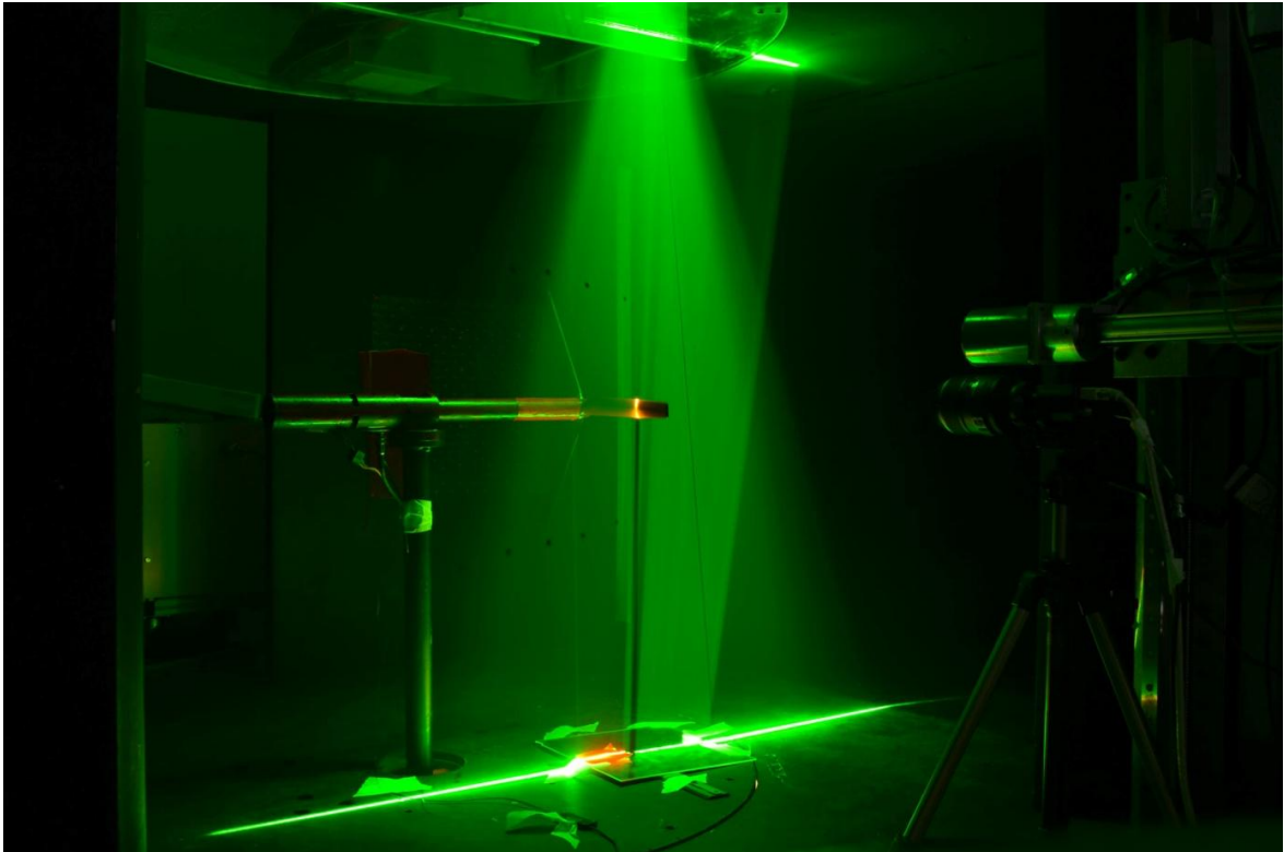
Fig.5.4 Expérimentation PIV à la soufflerie d'Arts et Métiers ParisTech
