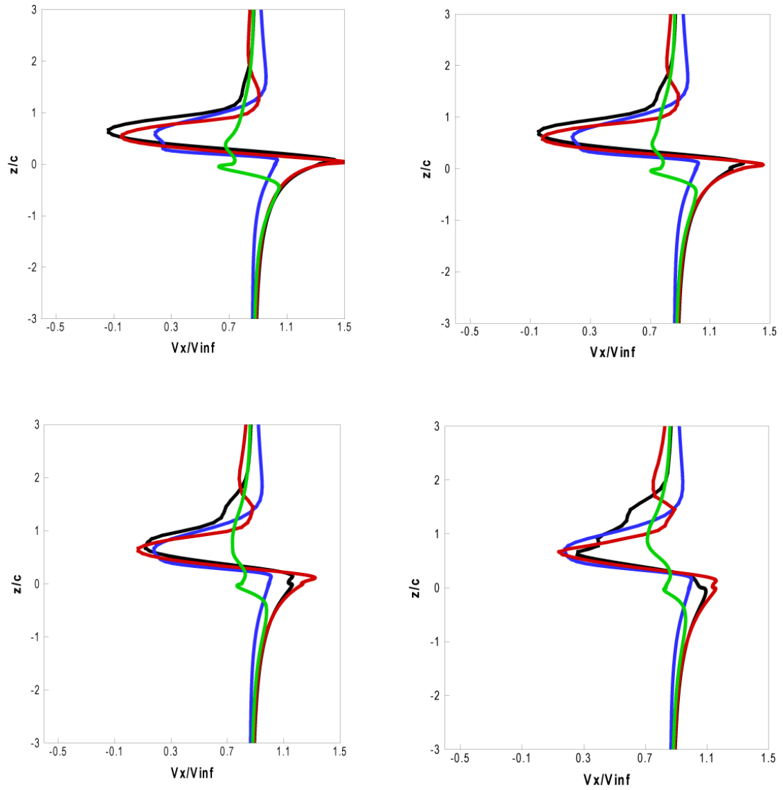
Fig. 4.15 (a) Comparaison des calculs du sillage - vitesse le long de la corde-profil S809 - \alpha=30^\circ
