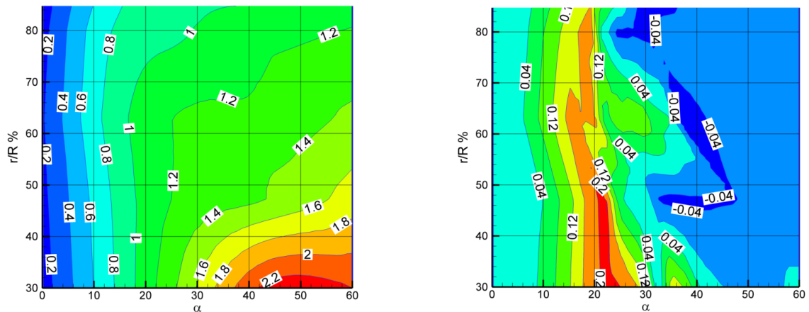
Fig.3.14 Coefficients de forces en fonction de l'angle d'incidence : forces normales (à gauche); forces tangentielles (à droite)
