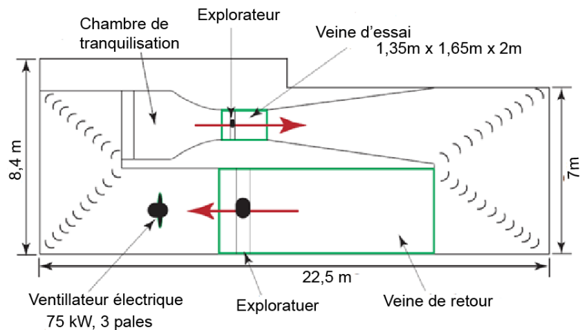
Fig.5.2 Soufflerie du Laboratoire de Mécanique des Fluides d'Arts et Métiers ParisTech
