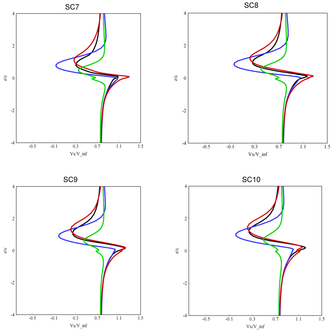
Fig. B.3 (a) Comparaison des calculs du sillage - vitesse le long de la corde-profil S809 - \alpha = 40^\circ
