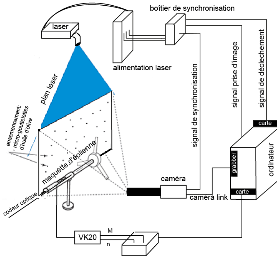
Fig. 5.5 Banc de mesure PIV
