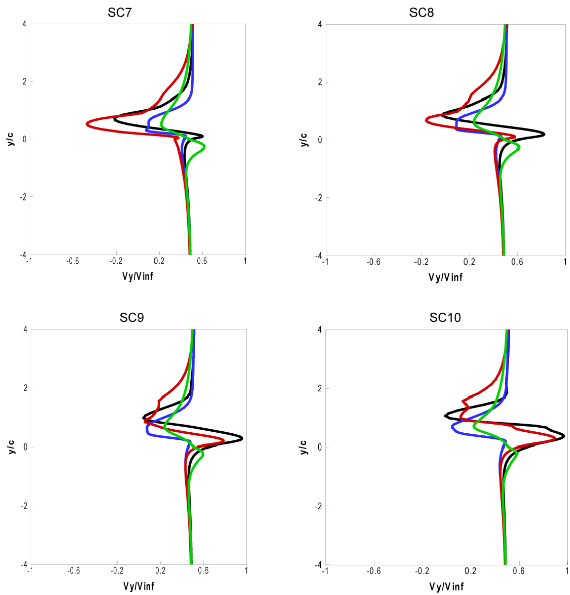
Fig. 4.15 (b) Comparaison des calculs du sillage - vitesse normale à la corde- profil S809 - \alpha=30^\circ
