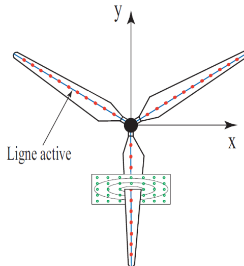
Fig. : 3.4 Modèle hybride de la ligne active
