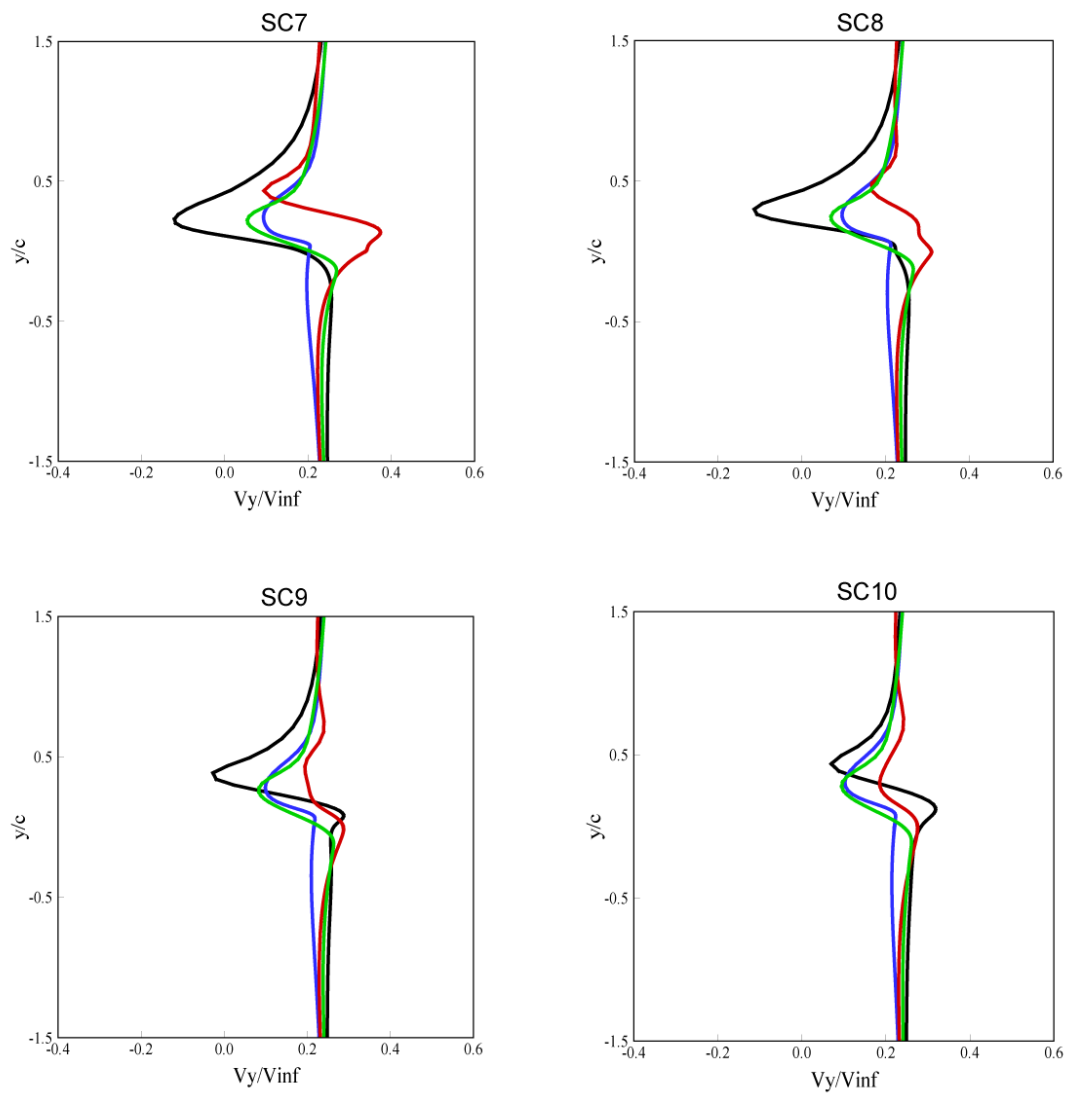
Fig.B.2 (b) Comparaison des calculs du sillage - vitesse normale à la corde- profil S809 - \alpha=15^\circ
