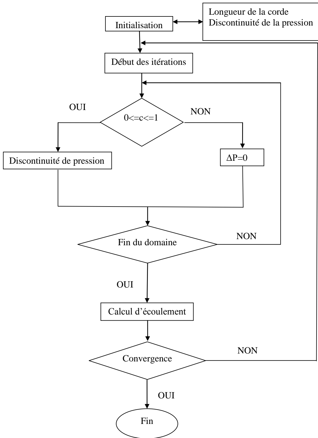
Fig. 4.6 Organigramme du modèle hybride de surface active avec discontinuité de pression
