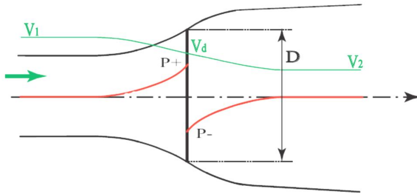
Fig. 2.4 disque perméable et tube de courant
