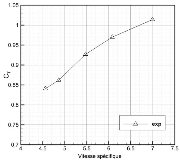
Fig. 5.8 Coefficient de poussée en fonction de la vitesse spécifique
