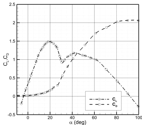
Fig. 6.7 Caractéristiques aérodynamiques du profil NACA 4418 [93]
