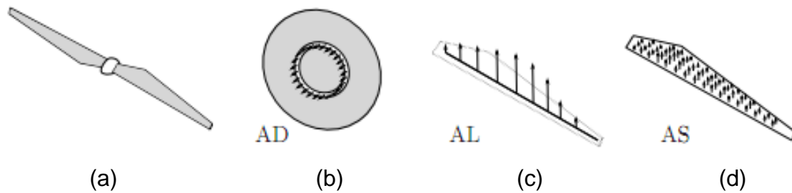
Fig. 2.8 Représentation (a) géométrie complète (b) disque actif (c) ligne active (d) surface active [77]
