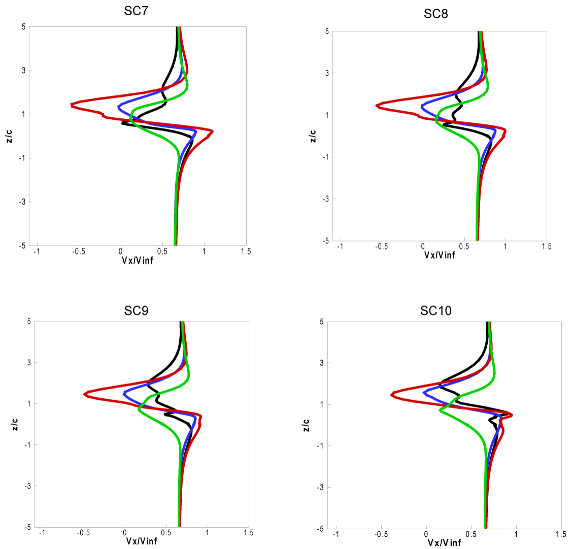
Fig. B.4 (a) Comparaison des calculs du sillage - vitesse le long de la corde-profil S809 - \alpha = 50^\circ
