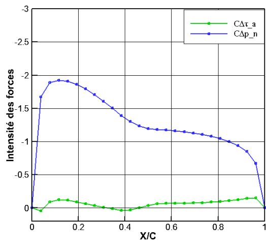
Angle d'incidence 45°
