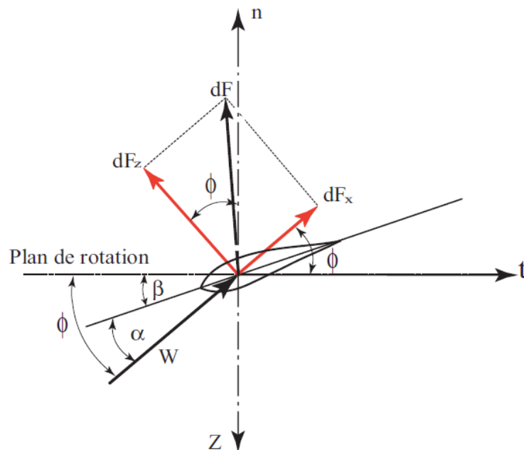
Fig. 2.2 Forces agissant sur un élément de pale
