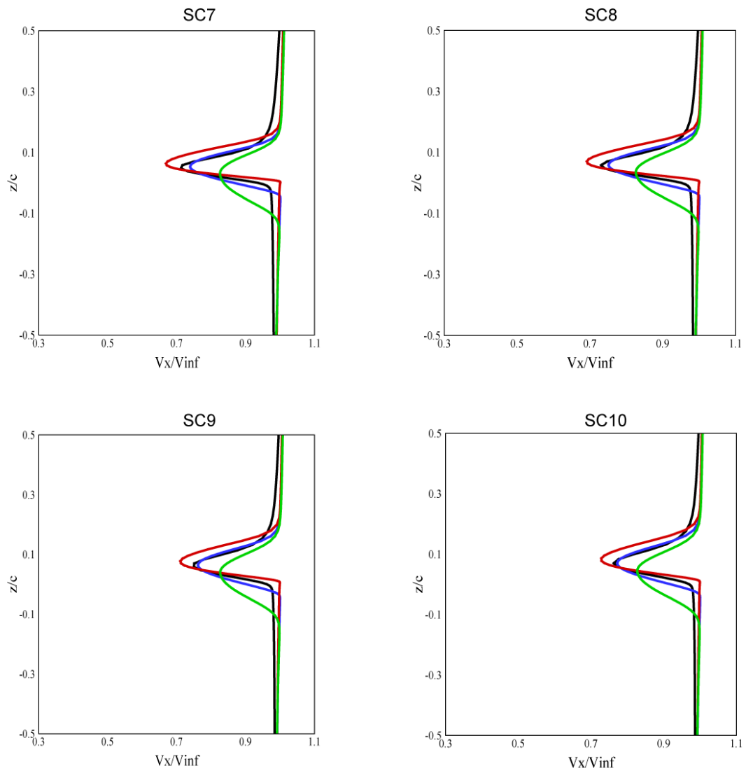
Fig. 4.13 (a) Comparaison des calculs du sillage - vitesse le long de la corde-profil S809 - \alpha=5^\circ
