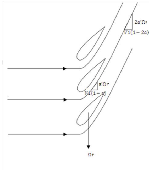
Fig. 2.5 Vitesse tangentielle à travers l'éolienne
