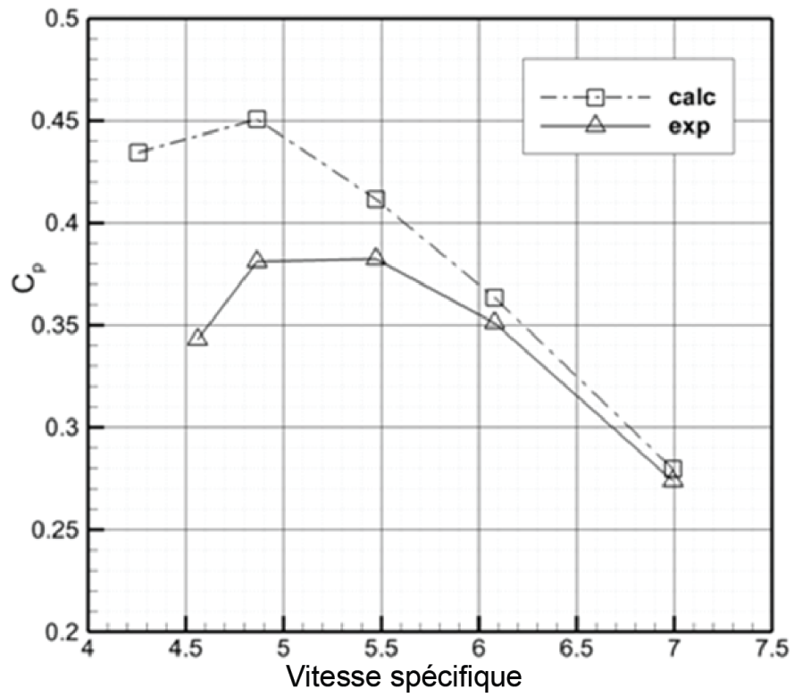
Fig. 6.11 Coefficient de puissance en fonction de vitesse spécifique
