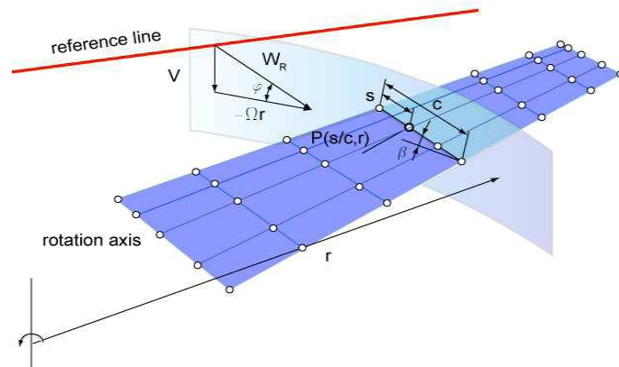
Fig. 3.7 Géométrie de la surface active [56]
