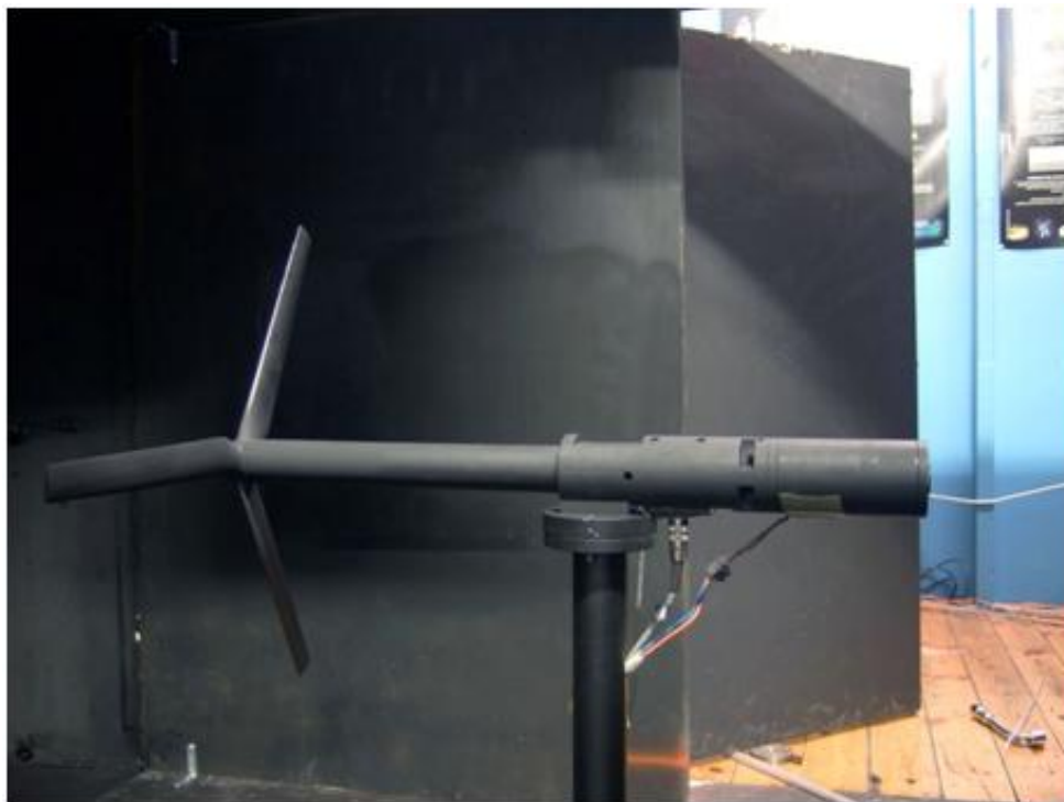
Fig. 5.3 Eolienne à axe horizontal testée à la soufflerie
