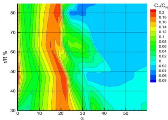
Fig. 3.15 Rapport des coefficients de forces C_n/C_t
