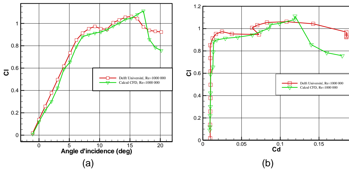
Fig. 4.3 Simulations numériques et résultats d'essais de l'Université de Delft : (a) portance en fonction de l'angle d'incidence; (b) portance en fonction de la traînée.
