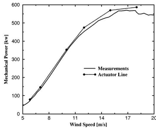
Fig. 3.5 Comparaison de la puissance mécanique entre le modèle de ligne active et éolienne Nordtank 500/41 [57]
