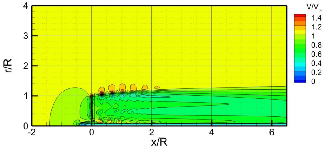
Fig. 6.6 Champ d'écoulement issu du calcul
