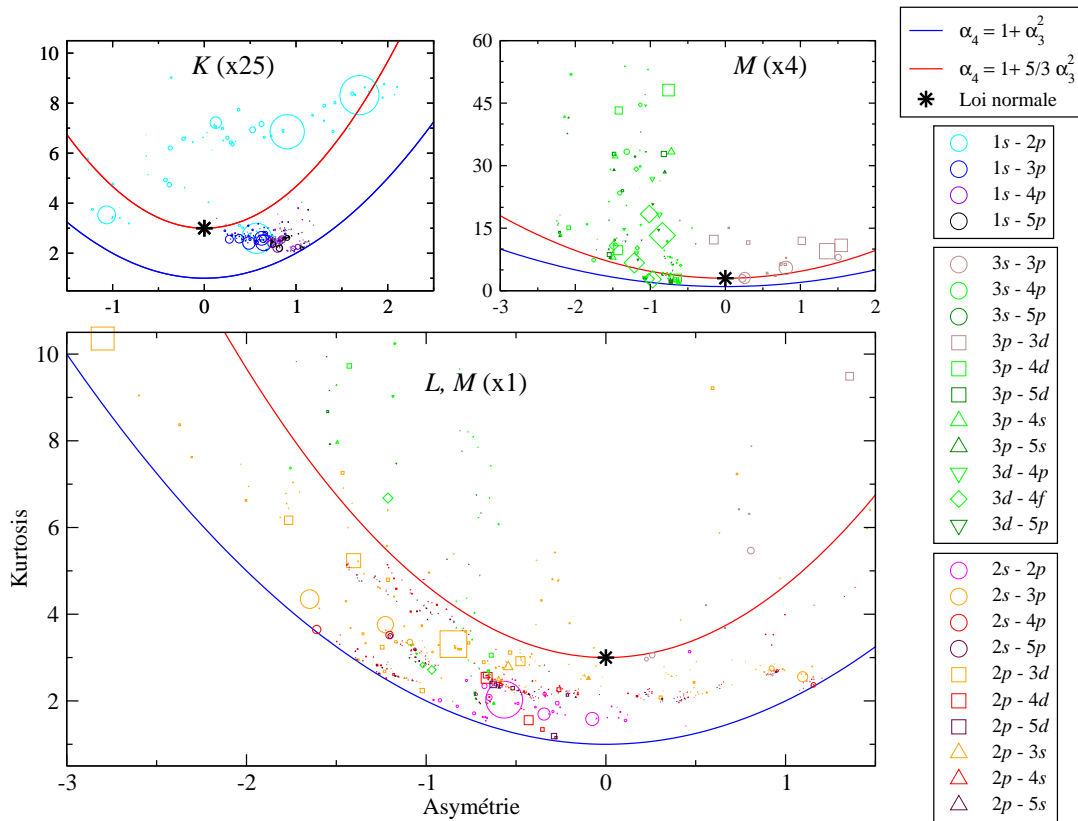
FIGURE 8.3 – Cartographie de l’asymétrie (abscisses) et du kurtosis (ordonnées) des faisceaux de transition de l’aluminium à 40 eV et 10 mg/cm 3 . L’intensité des faisceaux est proportionnelle à l’aire contenue dans chaque cercle, triangle et carré; la couleur dénote les couches initiale et finale tandis que la forme dénote les \ell initial et final. Les intensités ont été multipliées pour les couches K et M. La parabole bleue minore en \alpha_4 le domaine dans lequel asymétrie et kurtosis peuvent prendre leurs valeurs pour toute distribution positive; la parabole rouge minore en \alpha_4 le domaine dans lequel la NIG (voir Sec. C.2 dans les annexes.) est calculable.
