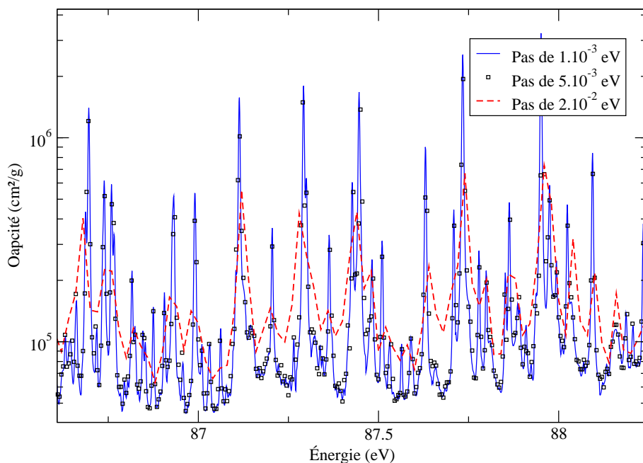
FIGURE 5.5 – Détail de l’opacité autour de 87 eV montrant l’effet de la résolution de la grille sur la forme du spectre.
