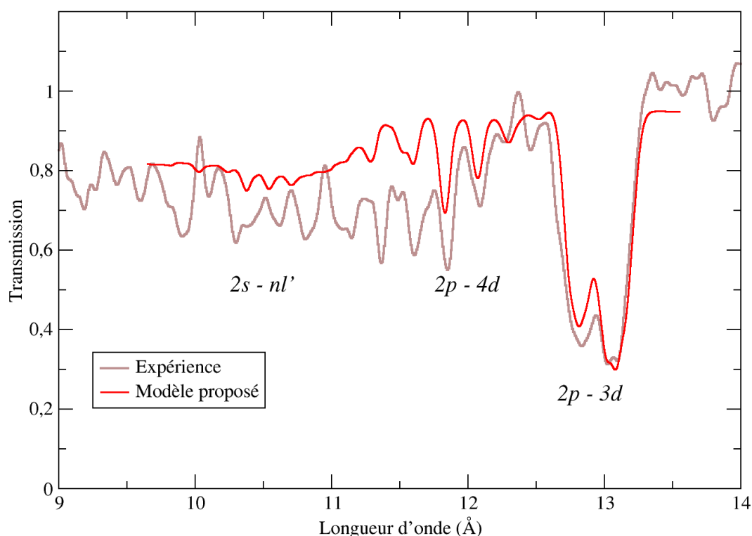
FIGURE 3.2 – Comparaison entre le spectre produit à une température de 16 eV et une densité de 5 \text{ mg/cm}^3 par notre approche et un spectre expérimental en transmission à la masse surfacique de 40 \text{ } \mu\text{g/cm}^2 [54, 55].
