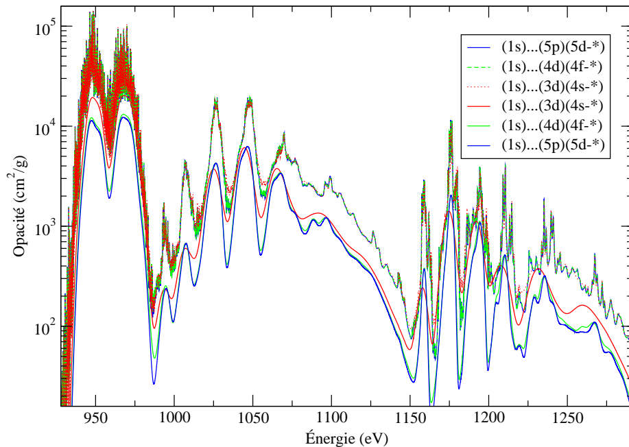
FIGURE 5.6 – Comparaisons des contributions détaillée et statistique en fonction de la supracouche-chapeau.
