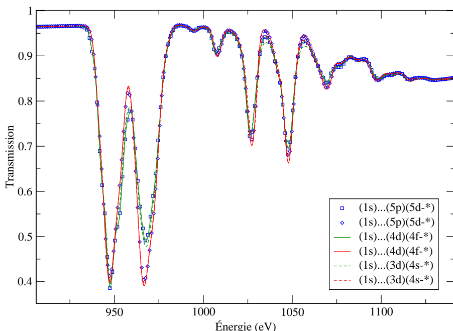
FIGURE 5.7 – Comparaison de transmissions à travers un milieu optiquement mince en fonction de la supracouche-chapeau. Les courbes plus ou moins discontinues au-dessus indiquent l'opacité lié-lié totale, les courbes continues dessous indiquent la contribution statistique au lié-lié.
