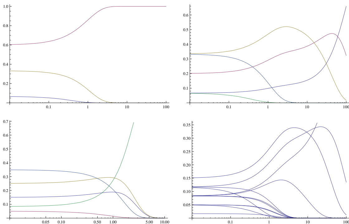
FIGURE 8.14 – Probabilités des termes spectroscopiques (gauche) et des niveaux (droite) en fonction de l'inverse de la température \beta pour la configuration P II 3s^23p^2 (haut) et 3s^23p3d (bas).
