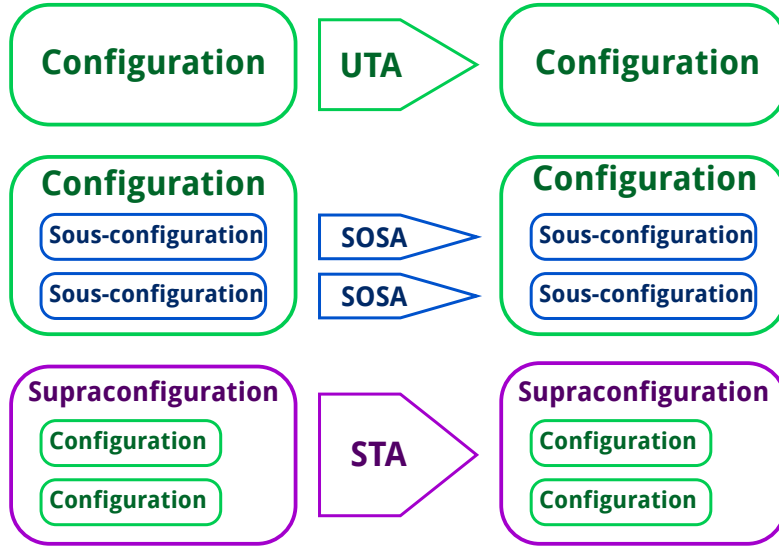
FIGURE 5.1 – Schéma des différents types de faisceaux de transition lié-lié rencontrés lors d'un calcul SCO.
