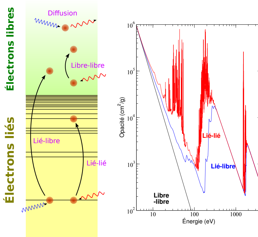
FIGURE 1.2 – Schéma des différents processus d'absorption (gauche) et opacité de l'aluminium à la température de 40 eV et 10 \text{ mg/cm}^3 montrant les trois contributions : libre-libre continue mais faible, lié-libre avec ses seuils et lié-lié caractérisée par de nombreuses raies (droite).
