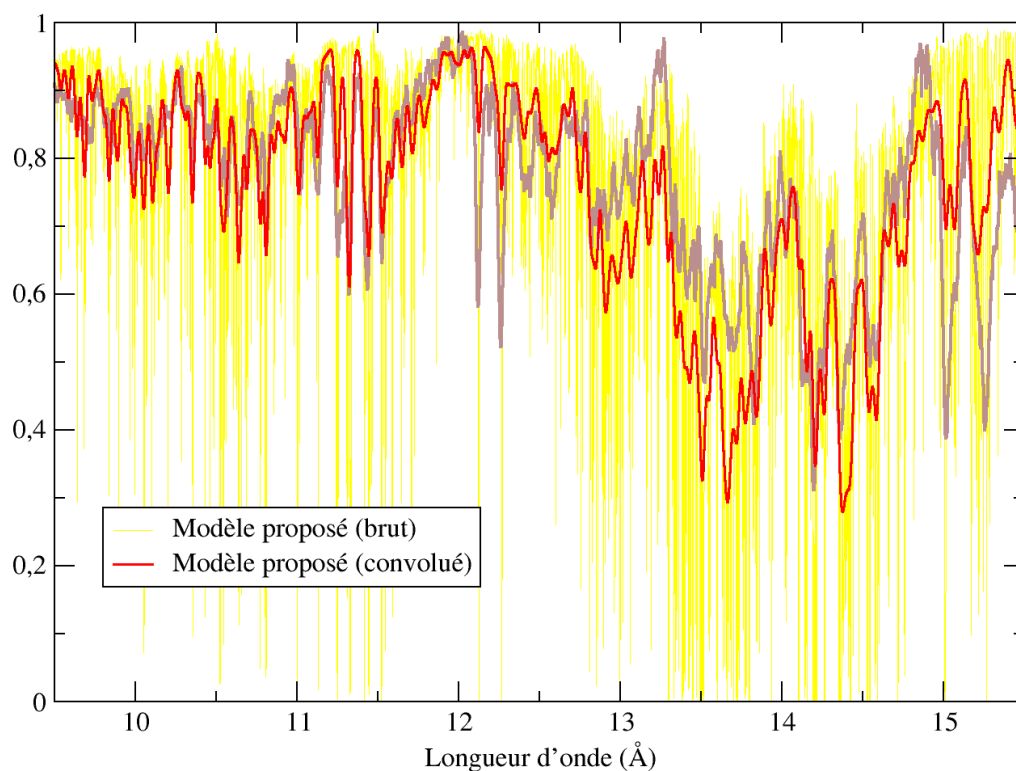
FIGURE 3.3 – Spectres en transmission du fer à 155 eV, avec une profondeur optique de 32,8 \mu\text{g}/\text{cm}^2 .
