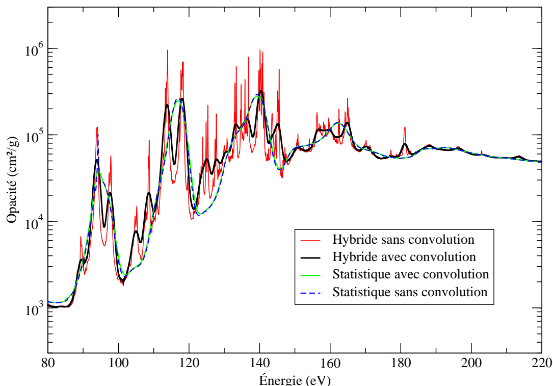
FIGURE 5.8 – Comparaison de l’opacité en couche L de l’aluminium à 20 eV et 10 \text{ mg/cm}^3 avec ou sans convolution des faisceaux et des raies par un élargissement expérimental de paramètre 0,7 eV.
