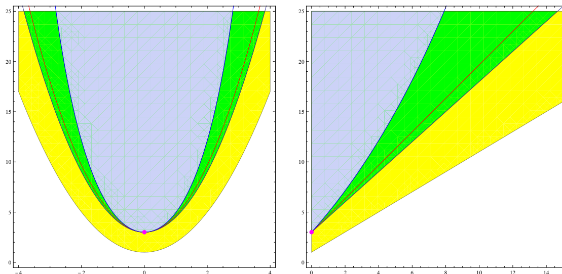
FIGURE C.6 – Domaines en (\alpha_3, \alpha_4) (à gauche) et (\beta_3, \alpha_4) (à droite) dans lesquels les différentes distributions de Pearson sont applicables. La Pearson IV s'applique dans la région bleue, la Pearson VI dans la région verte et la Pearson I dans la région jaune. La courbe rouge dénote la limite inférieure en \alpha_4 d'application de la NIG et le point rose la loi normale, symétrique et de kurtosis égal à 3.
