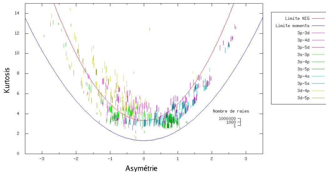
FIGURE 8.5 – Cartographie du nombre de raies des faisceaux du cobalt en fonction de l'asymétrie et du kurtosis des faisceaux.
