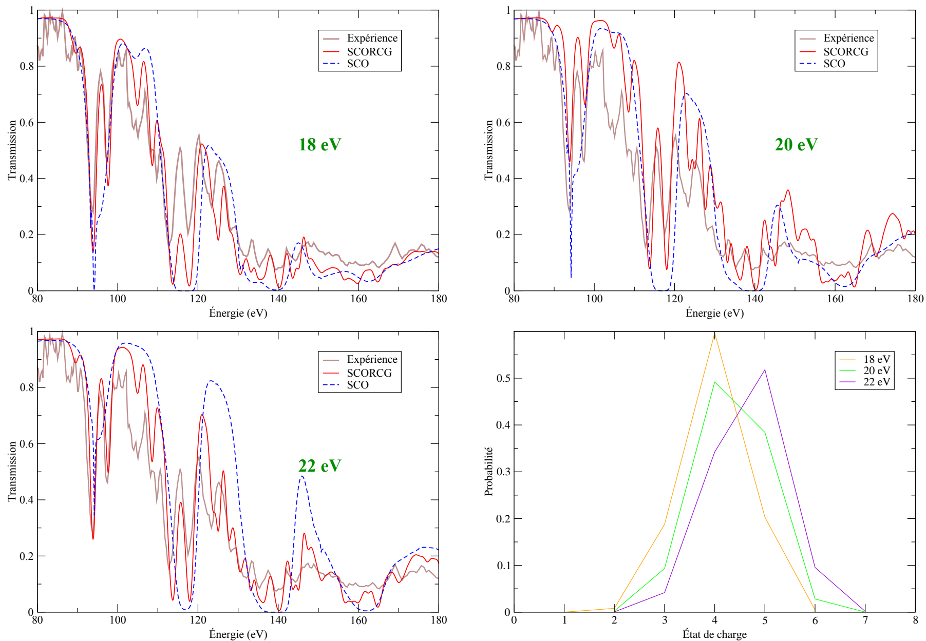
FIGURE 9.13 – Comparaison du spectre expérimental avec des spectres théoriques. Le diagramme en bas à droite représente la distribution ionique.
