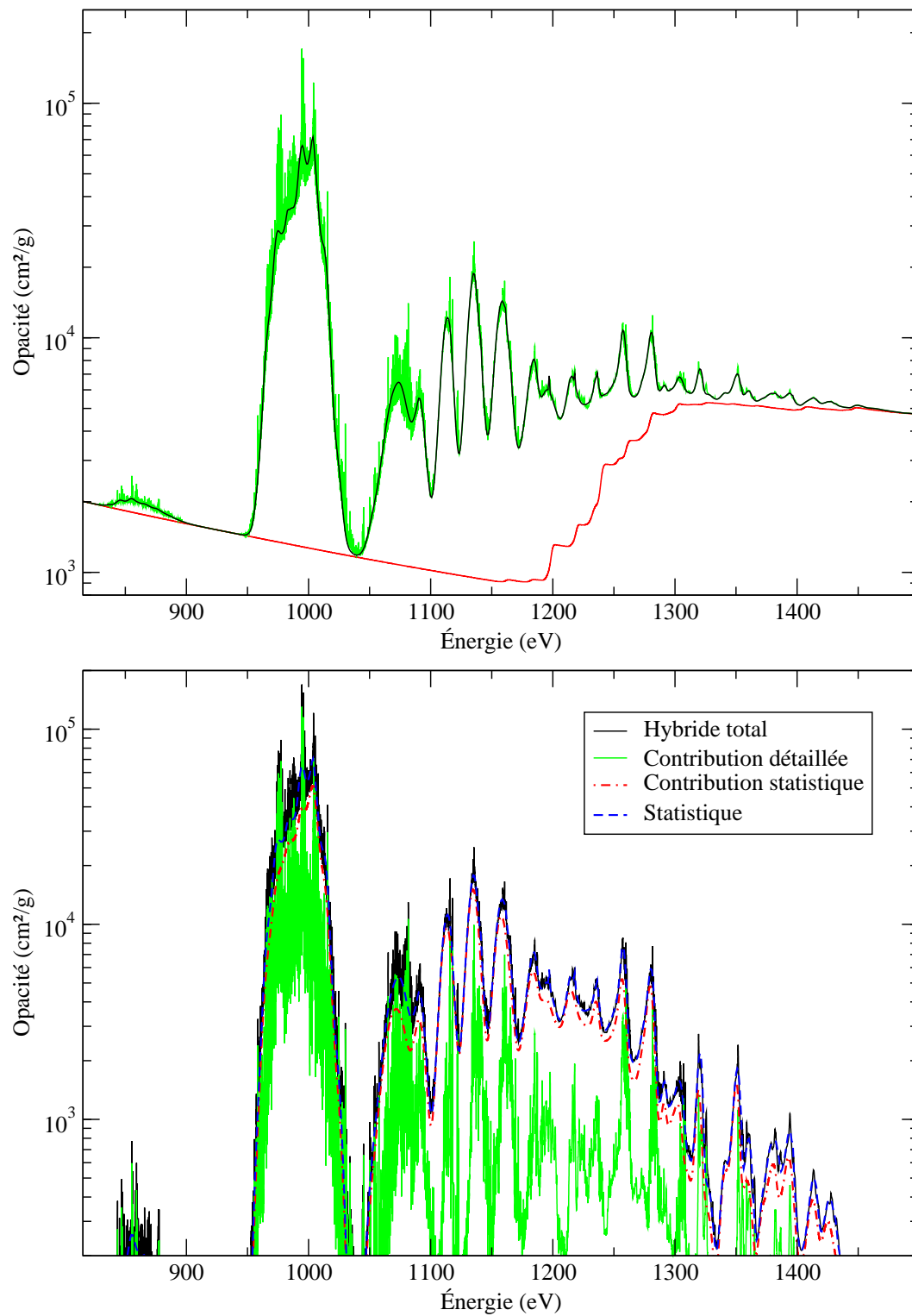
FIGURE 6.5 – Opacité et contributions du cuivre à 35 eV et 4 mg/cm³.
