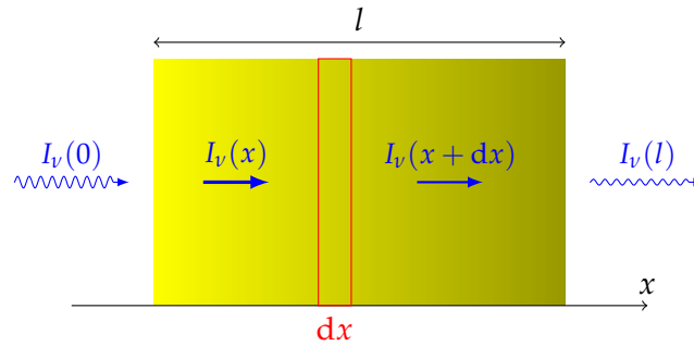
FIGURE 1.3 – Schéma de la propagation dans un milieu absorbant.
