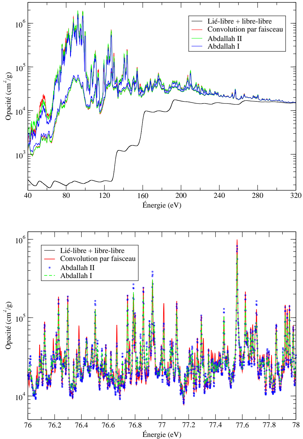
FIGURE 7.1 – Enveloppe (haut) et détail (bas) d'un spectre de cuivre à 10^{-3} \text{ g/cm}^3 et 20 eV calculé selon les trois méthodes de gestion des raies.
