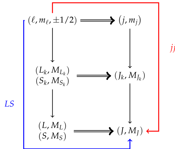
FIGURE 2.3 – Schéma de couplage des moments cinétiques envisageables entre les moments cinétiques de chaque électron (en haut) et les moments cinétiques de la configuration (en bas). La flèche bleue illustre la démarche du couplage LS , la flèche rouge illustre la démarche du couplage jj .
