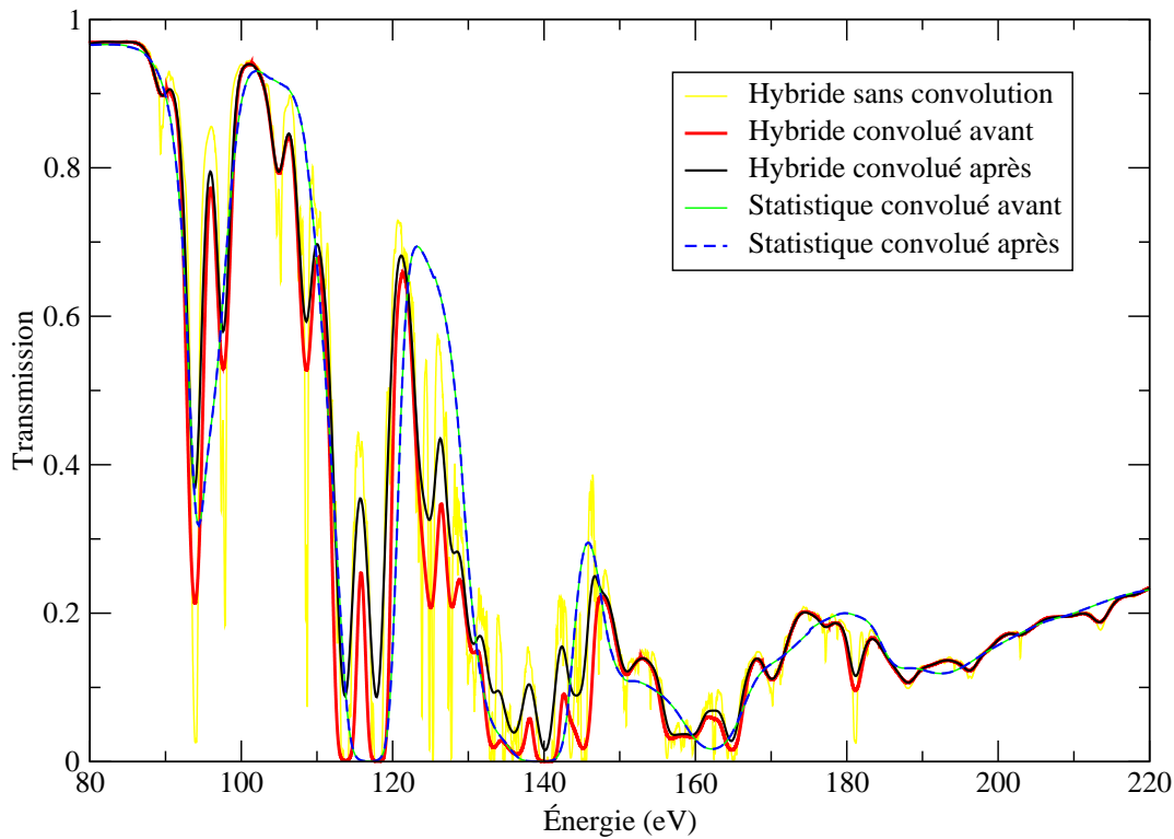
FIGURE 5.9 – Comparaison des spectres en transmission détaillés et statistiques obtenus par les deux méthodes de prise en compte de l'élargissement expérimental.
