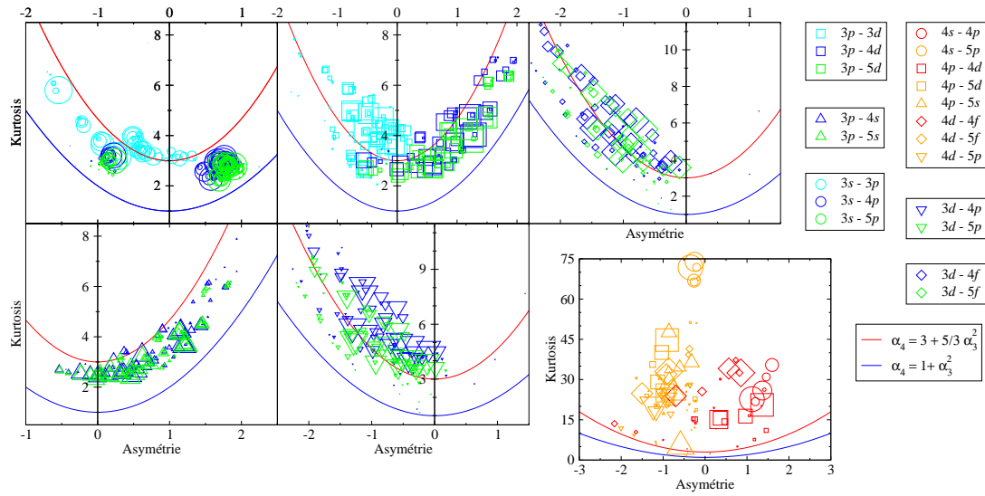
FIGURE 8.6 – Cartographie du nombre de raies (proportionnel à l’aire) des faisceaux du cobalt en fonction de l’asymétrie et du kurtosis des faisceaux.
