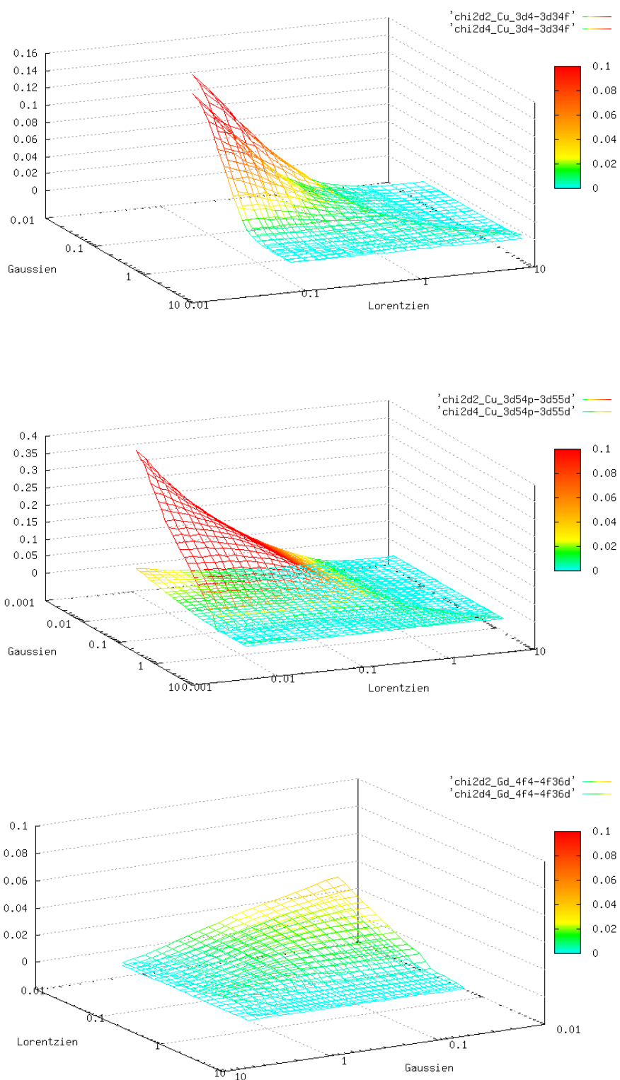
FIGURE 8.10 – Graphes de surface des indicateurs de forme à l'ordre 2 (légende chi2d2) et à l'ordre 4 (légende chi2d4), pour les faisceaux \text{Cu}^{7+}3d^4 - 3d^34f (en haut), \text{Cu}^{7+}3d^54p - 3d^55d (au milieu) et \text{Gd}^{6+}4f^44f^36d (en bas).
