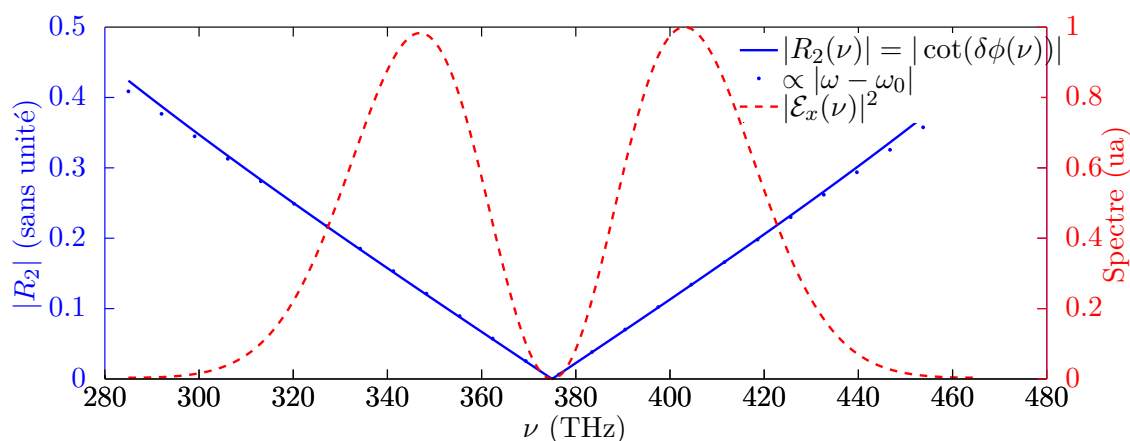
Figure 3.12: Module de la fonction de transfert complexe ( R_2 = \frac{\mathcal{E}_x}{\mathcal{E}_y} ) d'un BSB en Quartz ( \delta L_{\text{Quartz}} = 44.9 \mu\text{m} ) et le spectre du mode de mesure \mathcal{E}_x en fonction de la fréquence optique ( \rho = 99.9963 et Energie=0.008).
