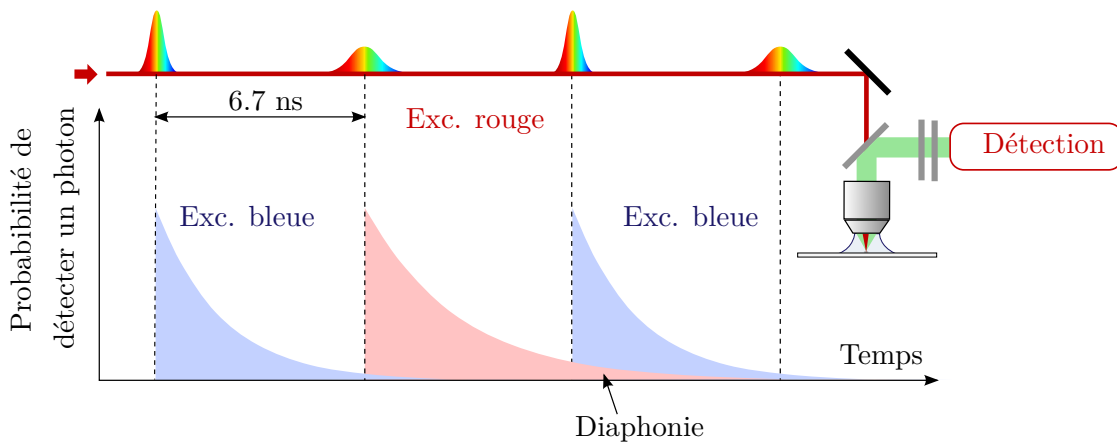
Figure 2.24: Représentation schématique de la synchronisation de la détection des signaux de fluorescence avec le train d'impulsions incident.
