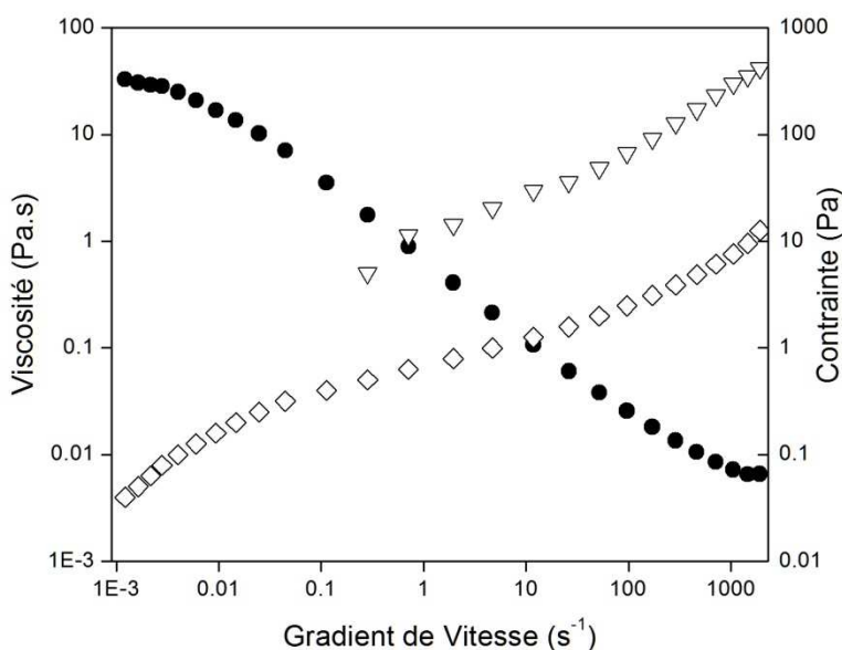
Figure 14: Propriétés rhéologiques d'une formulation utilisée en polymer flooding . La viscosité (●), la contrainte normale (▽) et la contrainte tangentielle (◇) en fonction du gradient de vitesse pour une solution aqueuse avec 2000 ppm de FLOPAM (Polyacrylamide hydrolysé SNF Floerger®)
