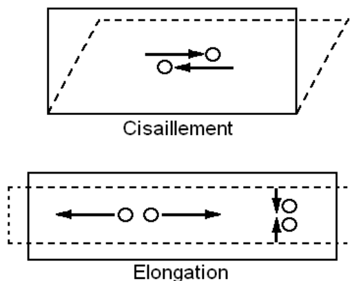
Figure 23 : Écoulement de cisaillement (deux particules adjacentes se croisent) et écoulement d'élongation (deux particules adjacentes s'éloignent ou se rapprochent)
