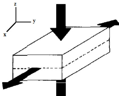
Figure 30 : Schéma d'une Élongation planaire dans la direction x
