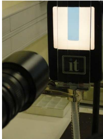
Figure 73 : Caméra, cellule et source de lumière
