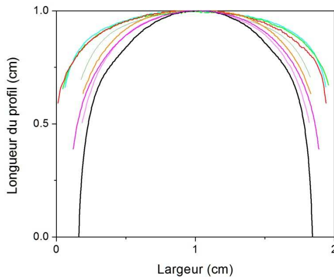
Figure 124 : Comparaison des profils de l'interface a v_{fi}=5 cm/s entre Canadou (noir), PEG-PEO8-800 (rouge), PAM-6000 (vert), PAM-4000 (cyan), PEG-PEO4-3000 (gris), PEG-PEO4-2000 (orange) PEG-PEO4-1000 (magenta) et PEG-PEO4-500 (rose). Longueur du profil en fonction de la largeur de la géométrie. A noter les différences pour la gamme des concentrations du PEG-PEO4.
