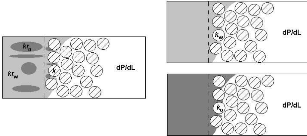
Figure 8 : La perméabilité relative d'un fluide dans un écoulement multiphasique (à gauche, gris obscur pour l'huile et gris claire par l'eau), peut être exprimée en fonction des perméabilités partielles des fluides en écoulement simple (à droite).
