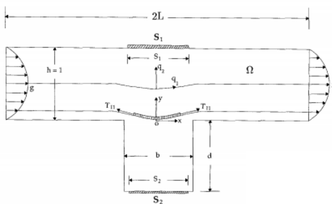
Figure 16 : Représentation schématique d'un écoulement a trou. La surpression due a N_1 est aussi affecte par les dimensionnes du trou. D'après [28].
