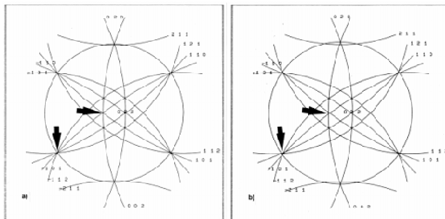
Figure I-41 : Simulation des lignes de Kossel d'un FeAl a) maille cubique b) maille quadratique avec \Delta c = 0,004 \text{ nm} [55]
