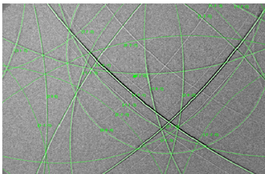
Figure IV-15 : Superposition du cliché simulé et du cliché expérimental d'une analyse relative
