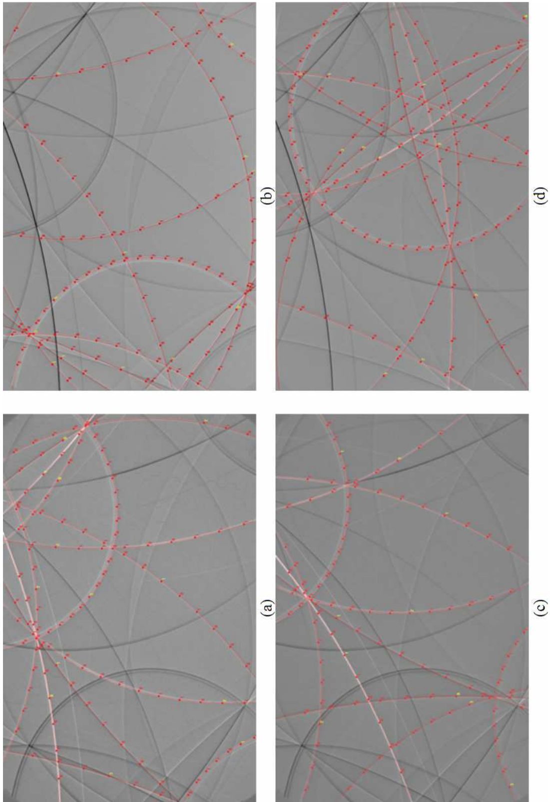
Figure V-16 : Clichés Kossel et coniques utilisées pour l'analyse relative, avec indication des écarts après la corrélation automatique pour les grains 1 (a), 2 (b), 3 (c) et 4 (d)
