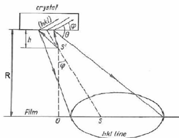
Figure I-27 : Géométrie de la diffraction pseudo-Kossel en réflexion [63]
