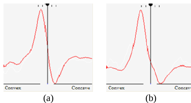
Figure III-8 : Comparaison du profil d'intensité d'une ligne dite claire/sombre pour deux distances caméra - échantillon : 32,5 mm (a) et 51,6 mm (b)
