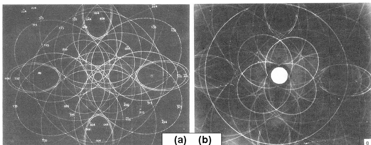
Figure I-31 : (a) Simulation par ordinateur d'un cliché de réflexion pseudo-Kossel (rayonnement \text{CuK}_\alpha ) pour un cristal de silicium orienté \langle 111 \rangle , (b) cliché expérimental correspondant [63]
