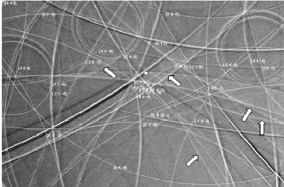
Figure V-11 : Cliché Kossel obtenu pour le grain 6 au point de chargement n°3 dans une zone plus riche en martensite et superposition de la simulation relative au cliché obtenu au centre du grain
