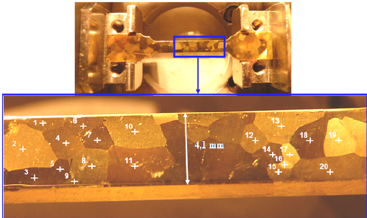
Figure V-2 : Epreuve de traction utilisée pour l'analyse de contraintes in situ avec repérage des 20 grains étudiés par microdiffraction Kossel
