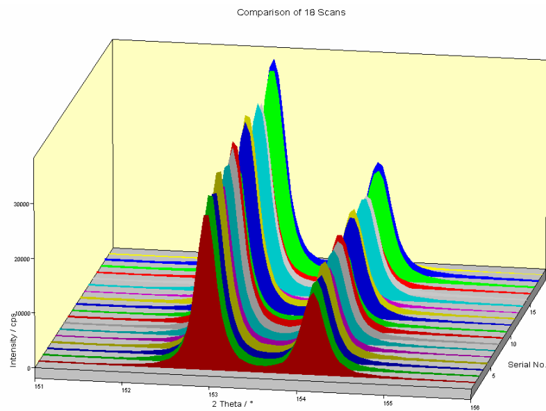
Figure IV-7 : Superposition des 18 acquisitions pour la détermination des angles de Bragg 2 \theta associés aux 18 plans interréticulaires choisis pour le calcul de l'état de contraintes du monocristal de germanium par analyse DRX
