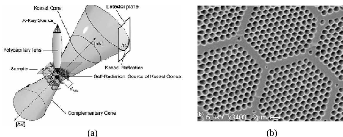
Figure I-21 : (a) Principe de la technique avec mise en place d'une lentille pour focaliser le faisceau (b) Vue de la section d'une lentille polycapillaire au MEB
