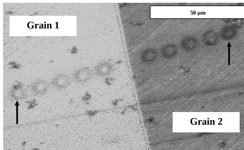
Figure V-13 : Image MEB de la microstructure du FeSi. Les 5 points de mesure par grain (espacés de 10 \mu\text{m} ) sont visibles grâce à la contamination due à la focalisation du faisceau électronique. Les flèches indiquent les points utilisés pour l'analyse intergranulaire
