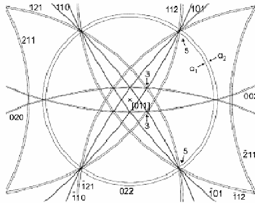
Figure I-40 : Simulation d'une variation de paramètre de maille \Delta a = a_2 - a_1 = 0,001 \text{ nm} sur le cliché Kossel d'un monocristal de fer [67]
