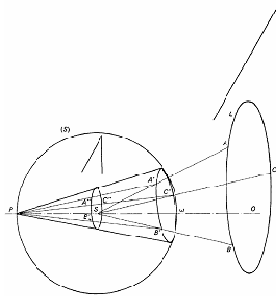
Figure I-33 : Méthode de Peters et Ogilvie - projections stéréographique et gnomonique [36]
