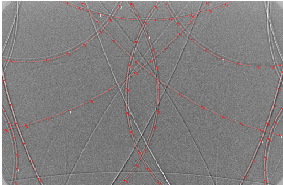
Figure IV-8 : Cliché expérimental obtenu pour le monocristal de cuivre avec superposition des 11 lignes positionnées par l'opérateur
