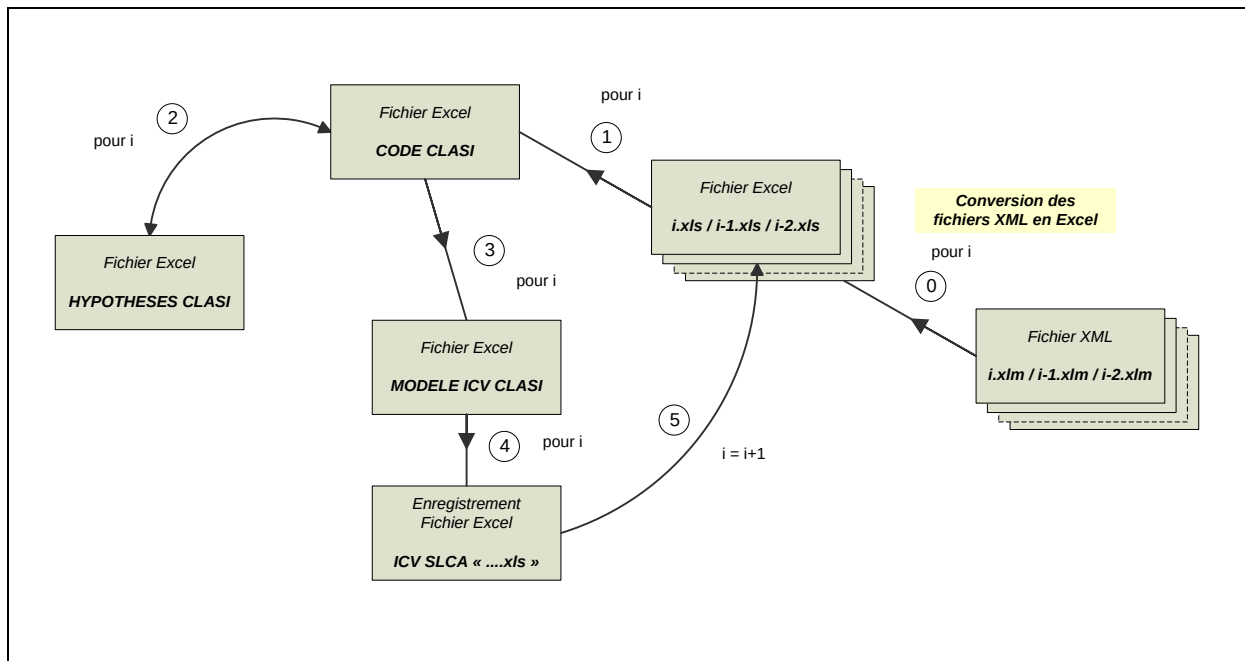
Annexe 1. Principe de la procédure informatique CLASI
