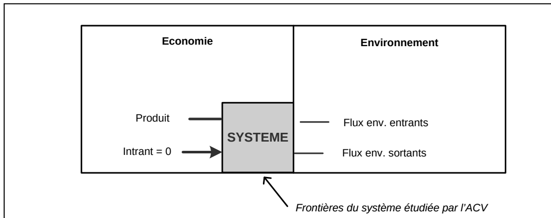
Figure 6. Principe de modélisation systémique appliquée à l'ACV adapté de Jolliet et al (2005)
