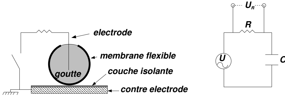
FIGURE 2.9 – Schéma du dispositif expérimental.
