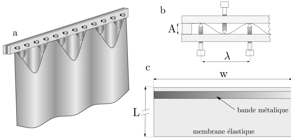
FIGURE 4.13 – Dispositif expérimental pour la mise en place des rideaux suspendus, a) vue isométrique, b) détail de l'imposition du profil sinusoïdal avec l'arrangement de vis, c) position de la bande métallique utilisée pour protéger le bord de la membrane.
