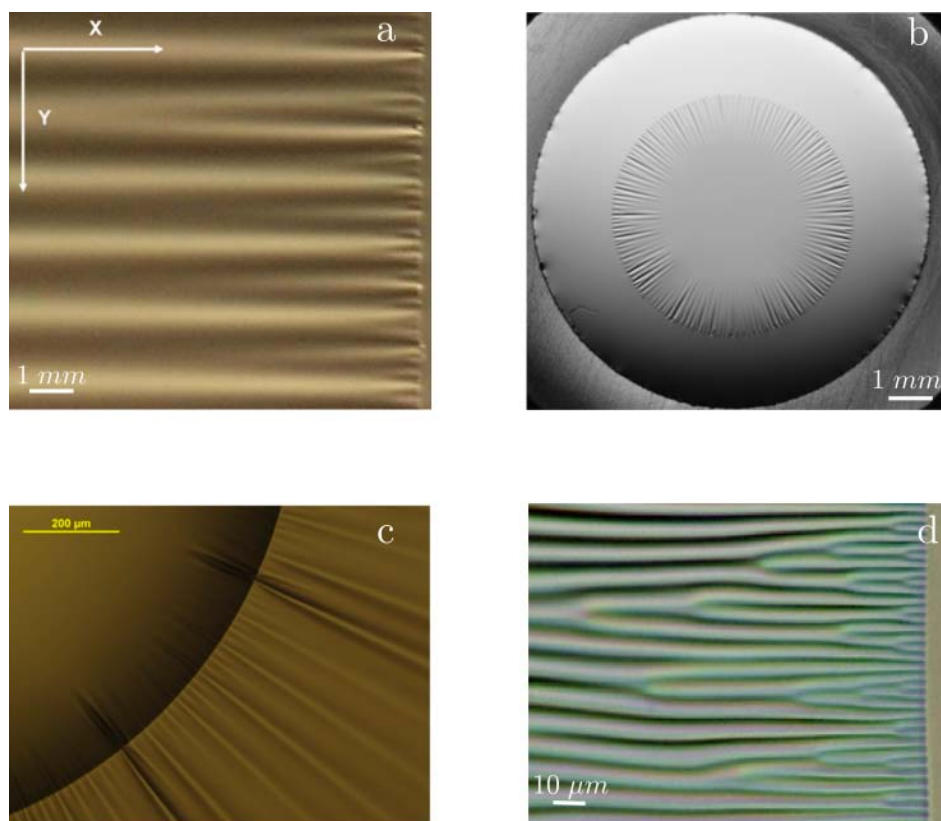
FIGURE 4.1 – Exemples de cascade de plis (a) membrane de polystyrène ultra mince (50 nm) comprimée à la surface de l'eau (tiré de [30]) (b) Un disque d'une telle membrane, posé sur une goutte d'eau (photo Hunter / N.Menon ) (c) Une goutte d'eau déposée sur un tel film flottant le plisse, mais près de la ligne de contact, une cascade peut être observée. (d) Couche de titane déposée sur une couche de polystyrène dans laquelle diffuse un solvant (cliché H.Vandeparre)
