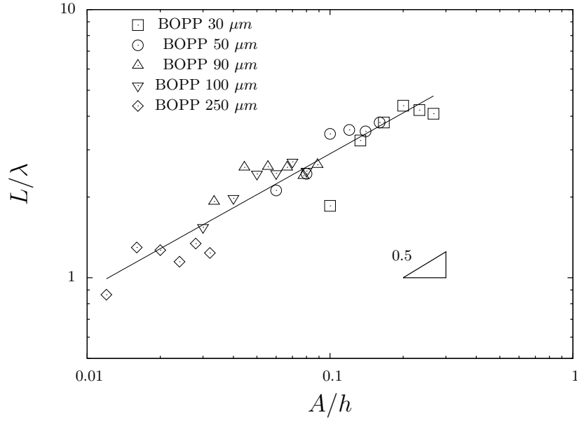
FIGURE 4.6 – Longueur de la transition de la longueur d’onde en fonction de l’amplitude du confinement et de l’épaisseur de la feuille.
