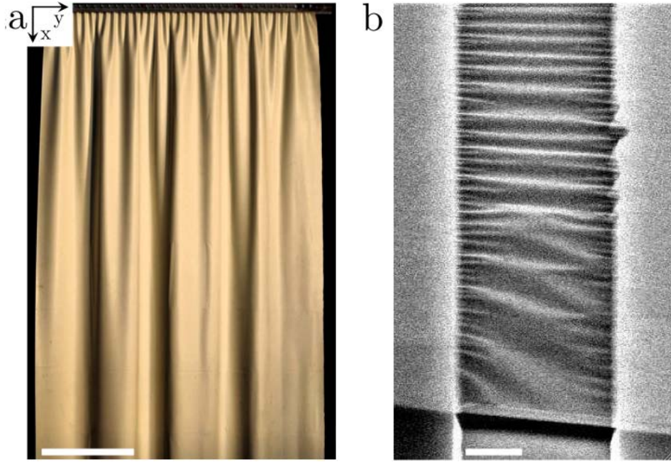
FIGURE 4.2 – Cascade de plis le long d'un rideau : les plis imposés nombreux aux bords se raréfient progressivement. (a) Rideau macroscopique en latex (barre d'échelle : 25 cm) ; (b) Bicouche de graphène tendue au-dessus d'une rainure (barre d'échelle : 1 \mu\text{m} ).
