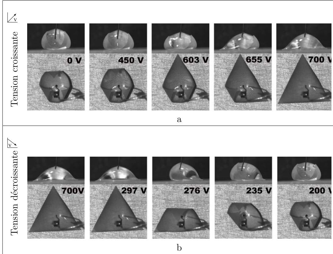
FIGURE 2.13 – Vues latérale et vue de haut de l'expériences, a) lorsque l'on augmente la tension, b) lorsque l'on décroît la tension pour revenir à une tension nulle. L = 7 \text{ mm} , h = 80 \text{ }\mu\text{m} , d = 60 \text{ }\mu\text{m} et L_{EC} = 0.47 \text{ mm} .
