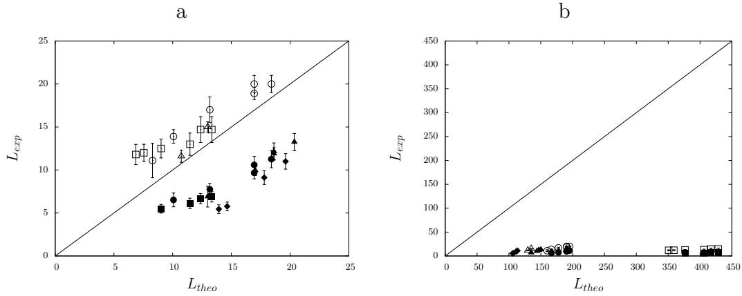
FIGURE 3.27 – Confrontation des données expérimentales contre les théories a) près du seuil, b) loin du seuil. Les données correspondent à la mesure de la longueur L_1 à partir du point d'inflexion des profils (symboles pleins) et L_2 à partir de l'amplitude de déformation nulle (symboles ouverts). Pour toutes les séries L_{ec}/L_c est constante et d'ordre 0.065
