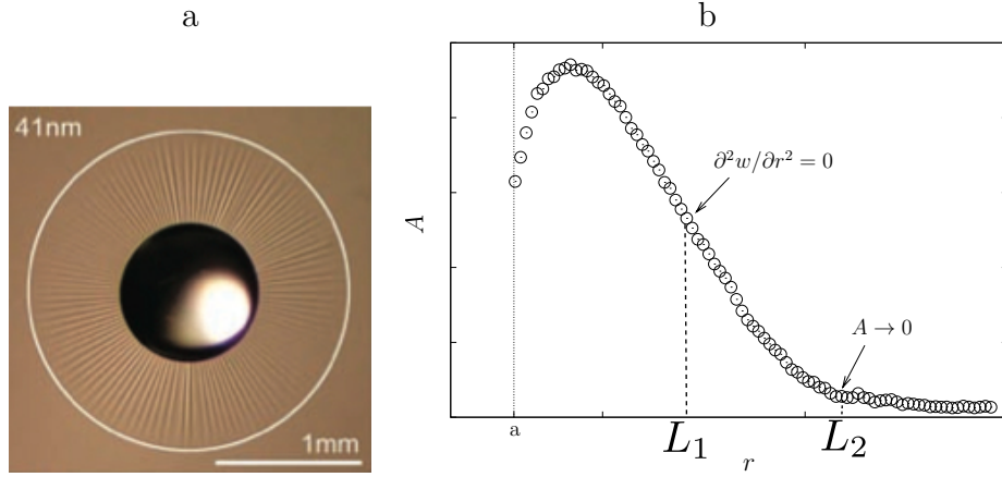
FIGURE 3.25 – a) Image de la formation des plis sur une membrane mince. Le cercle pointillé indique la longueur des plis formés [28]. b) Profil typique obtenu dans nos expériences à partir des champs de hauteur mesurés. Des profils semblables ont été aussi trouvés par [56].
