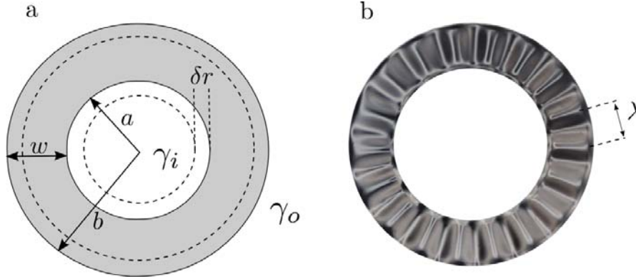
FIGURE 3.3 – a) Schéma d'une couronne qui se contracte d'une distance \delta r à cause d'une différence de tension. b) Définition de la longueur d'onde sur une couronne flambée.
