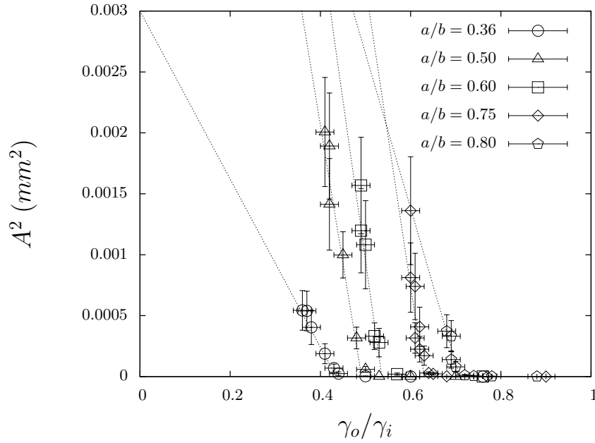
FIGURE 3.21 – Valeurs expérimentales de l’amplitude de déformation en fonction du rapport des tensions appliquées. Les résultats correspondent à des couronnes de différents rapports d’aspect a/b . Les lignes en pointillés correspondent à l’ajustement de chaque une des séries de données à une expression de la forme A^2 = \alpha \gamma_o / \gamma_i + \beta .
