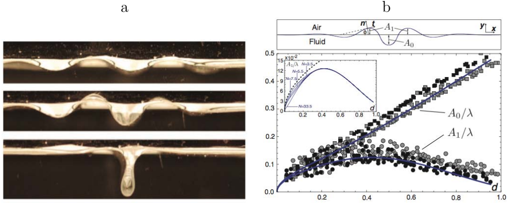
FIGURE 3.32 – a) Profil d’une membrane flottant dans l’eau soumise à une compression latérale. La compression augmente entre chacune des images, du haut vers le bas. Clichés pris de [62]. b) Données expérimentales de l’amplitude en fonction de la compression imposée obtenues par Pocivavsek [62].
