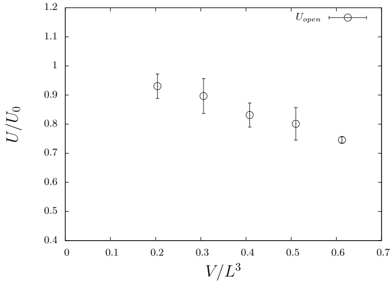
FIGURE 2.18 – Variation de la tension d'ouverture en fonction du volume de la goutte. L/L_{ec} = 12 = cte , avec L = 7 \text{ mm} et h = 100 \text{ }\mu\text{m} . L'épaisseur de la couche isolante reste aussi constante d = 50 \text{ }\mu\text{m} et donc U_0 \sim 800 \text{ V}
