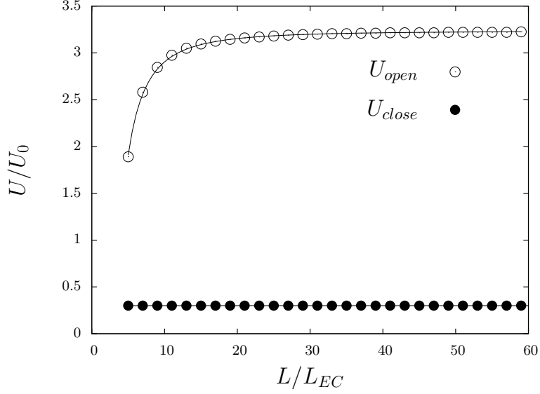
FIGURE 2.21 – Résultats de la simulation numérique pour les variations des tensions d'ouverture et de fermeture en fonction de L/L_{EC} .
