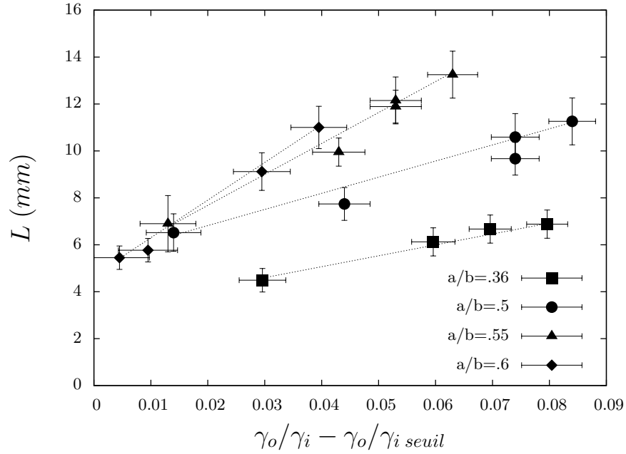
FIGURE 3.28 – Résultats expérimentaux de la longueur des plis en fonction de la tension appliquée. Les données correspondent à la mesure de la longueur à partir du point d’inflexion des profils. Pour toutes les séries L_{ec}/L_c est constante et d’ordre 0.065.
