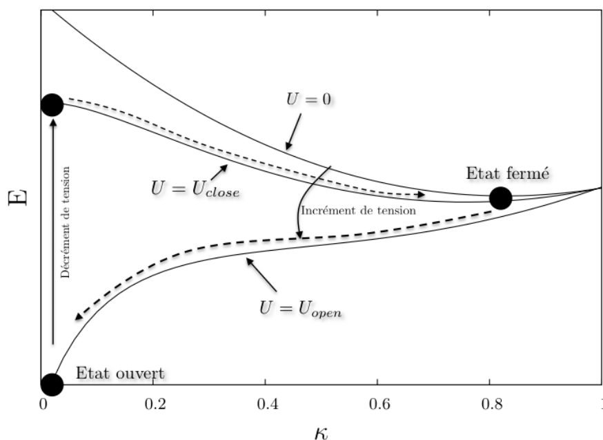
FIGURE 2.20 – Variation de l'énergie total du système en fonction de la courbure de la tige. Les lignes pointillées montrent les transitions entre l'état ouvert et fermé.
