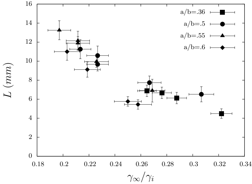
FIGURE 3.29 – Résultats expérimentaux de la longueur des plis en fonction de \gamma_\infty . Les données correspondent à la mesure de la longueur à partir du point d’inflexion des profils. Pour toutes les séries L_{ec}/L_c est constante et \sim 0.065 .
