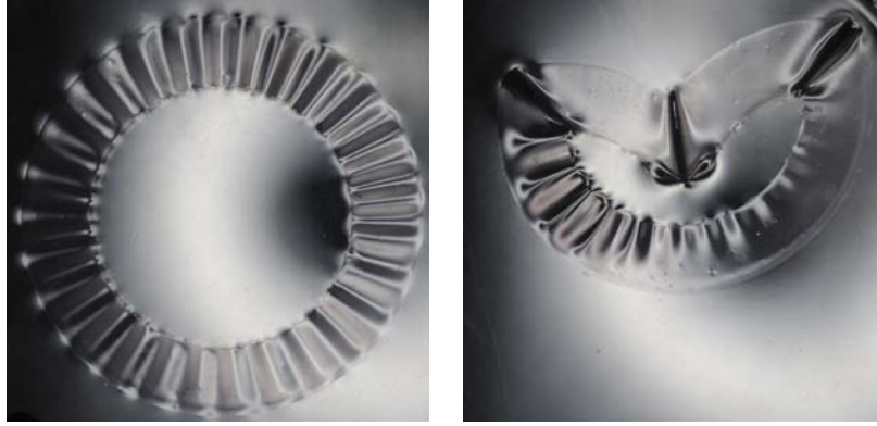
FIGURE 3.31 – Images d'un anneaux avant et après effondrement.
