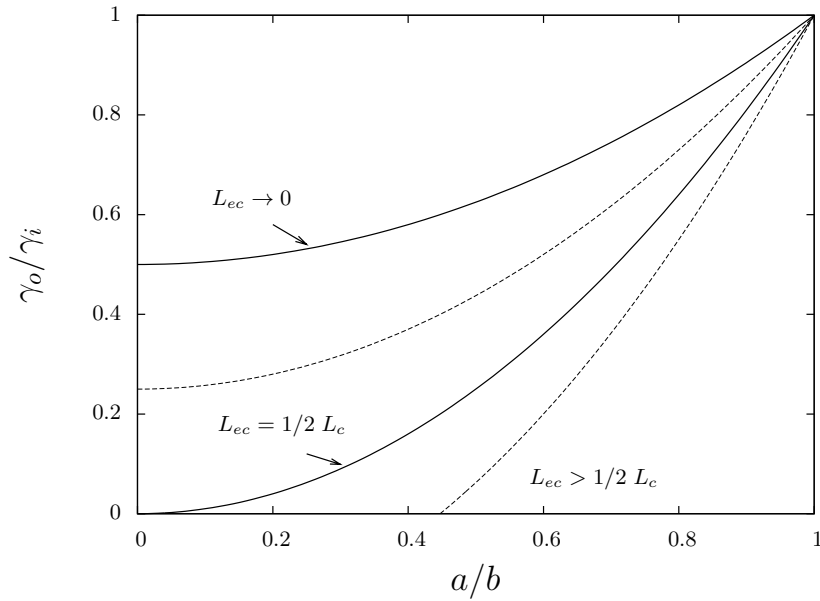
FIGURE 3.18 – Seuil de flambage \gamma_o/\gamma_{i \text{ seuil}} en fonction du rapport d'aspect a/b pour différentes valeurs de L_{ec} .
