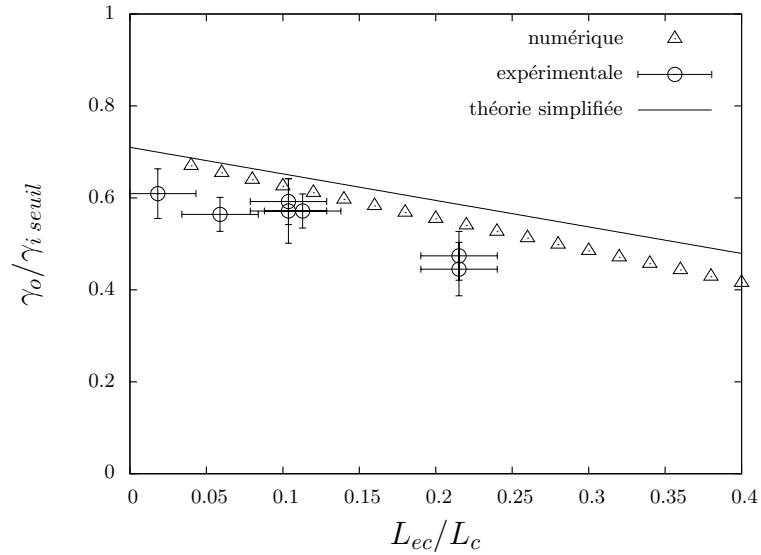
FIGURE 3.24 – Valeurs expérimentales (cercles) et numériques (triangles) pour le seuil de flambage en fonction de la longueur élasto-capillaire. Les lignes continues correspondent à l’estimation du seuil de flambage théorique donnée par l’équation 3.47 .
