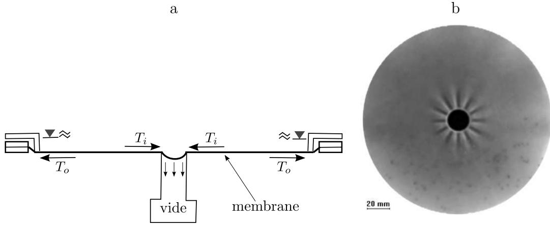
FIGURE 3.2 – a) Schéma du dispositif expérimental utilisé par Géminard et al. [56]. b) Vue de dessus des rides formées sur la membrane flexible (cliché pris de [56]).
