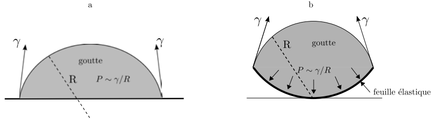
FIGURE 2.2 – Schéma d’une goutte d’eau déposée sur a) un substrat solide, b) un substrat flexible.
