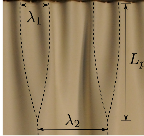
FIGURE 4.4 – Cascade élémentaire sur un rideau suspendu.
