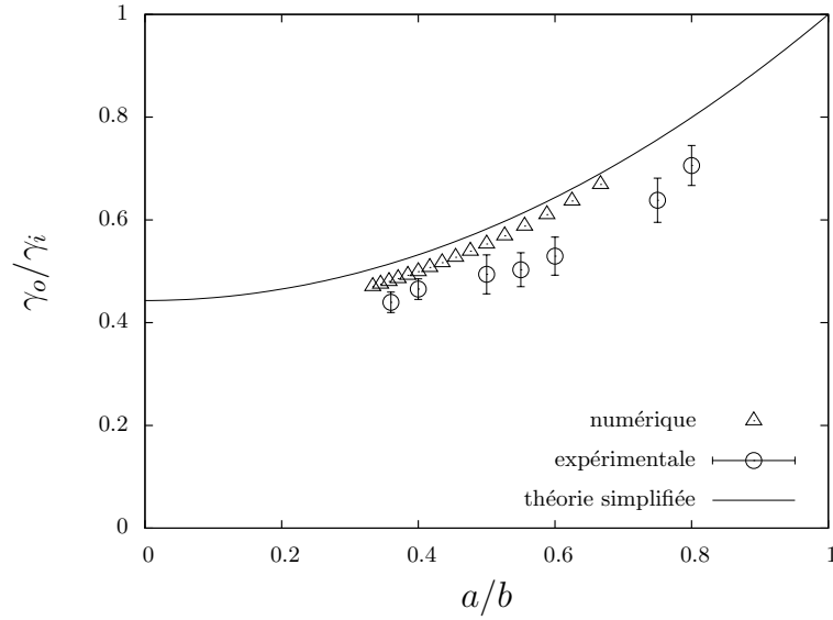
FIGURE 3.23 – Valeurs expérimentales (cercles) et numériques (triangles) pour le seuil de flambage en fonction du rapport d’aspect a/b . La ligne continue correspond à l’estimation du seuil de flambage théorique donnée par l’équation 3.47.
