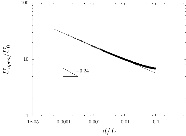
FIGURE 2.26 – Dépendance de la tension d’ouverture pour des petites valeurs de d .
