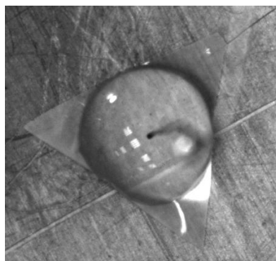
FIGURE 2.11 – Exemple d'une feuille qui reste collée sur le substrat empêchant l'enrobage de la goutte.
