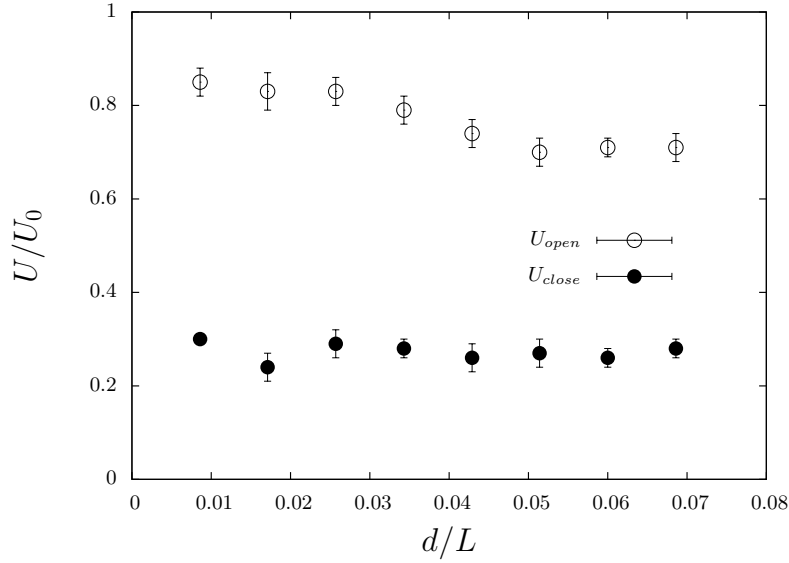
FIGURE 2.16 – Tensions d’ouverture et fermeture en fonction de l’épaisseur de la couche isolante. L/L_{EC} = 12 = cte , avec L = 7 \text{ mm} et h = 100 \text{ }\mu\text{m} , U_0 \sim 800 \text{ V}
