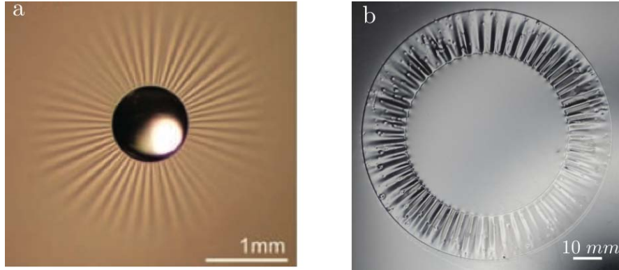
FIGURE 1.5 – (a) Rides générées par le dépôt d'une goutte sur une membrane flexible flottant dans l'eau [28]. (b) Rides formées sur un couronne flexible dues à une différence de tension de surface entre ses bords intérieur et extérieur
