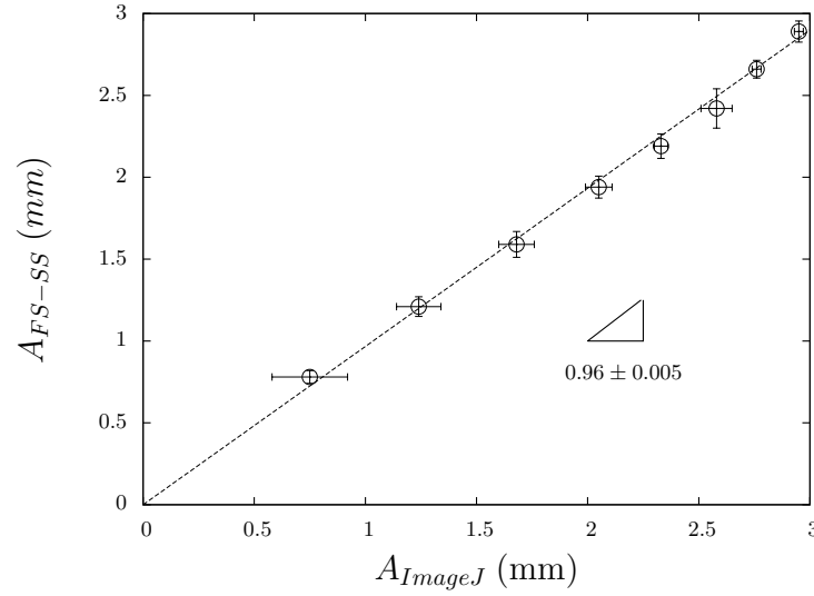
FIGURE 3.12 – Comparaison de l’amplitude de déformation mesurée en utilisant la technique FS-SS et ImageJ.
