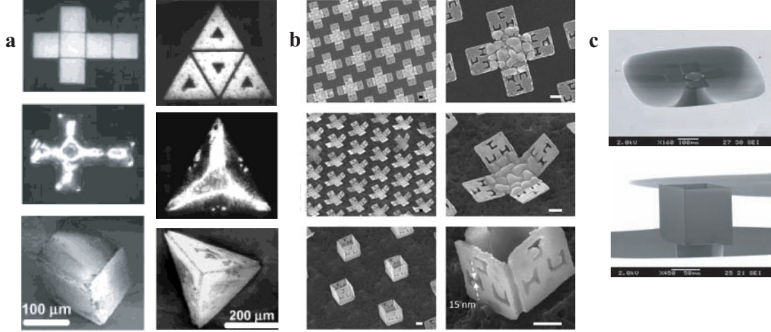
FIGURE 2.1 – (a) Repliement de panneaux pré-marqués autour d’une goutte de soudure (images extraites de [33]), (b) boîtes cubiques obtenues après fusion de la soudure déposée sur les charnières du patron initial (images extraites de [38]), (c) boîte obtenue après dépôt puis évaporation d’une goutte d’eau sur le patron en silicium (clichés J. van Honschoten).
