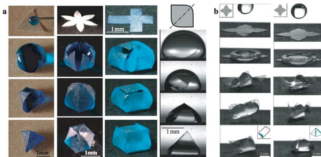
FIGURE 2.4 – (a) Origami capillaire : différentes formes tridimensionnelles peuvent être obtenues en fonction de la découpe initiale de la feuille. (b) Origami dynamique : une même feuille conduit à différents états finaux en fonction de la vitesse d’impact de la goutte (clichés Arnaud Antkowiak).
