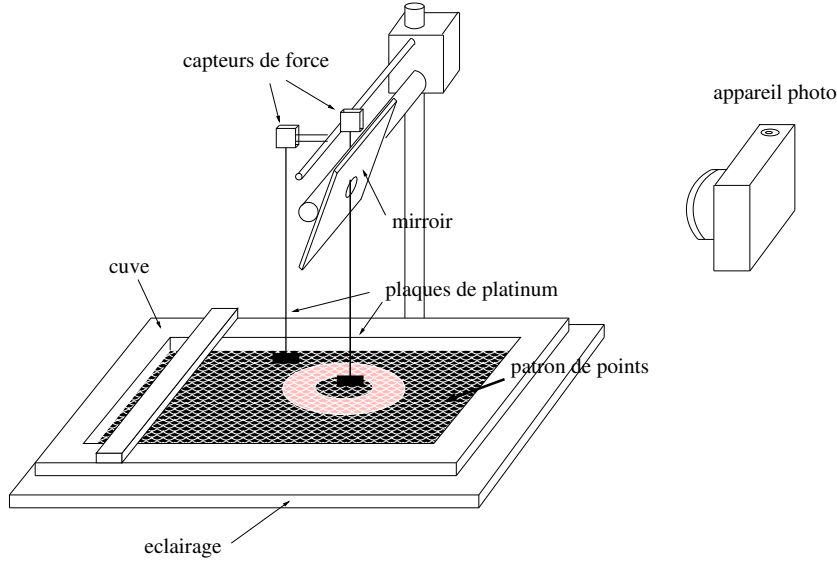
FIGURE 3.6 – Configuration du dispositif expérimental.
