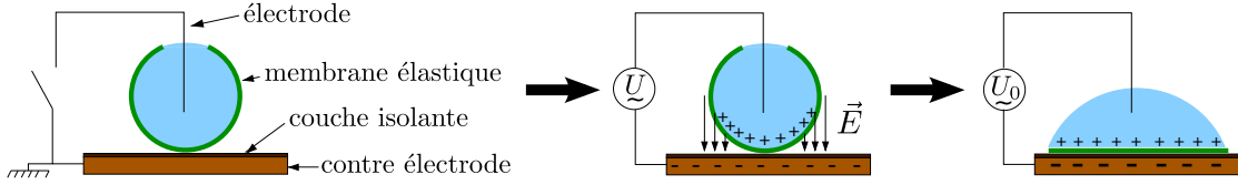
FIGURE 2.7 – Schéma de l'actuation d'un origami capillaire par un champ électrique.
