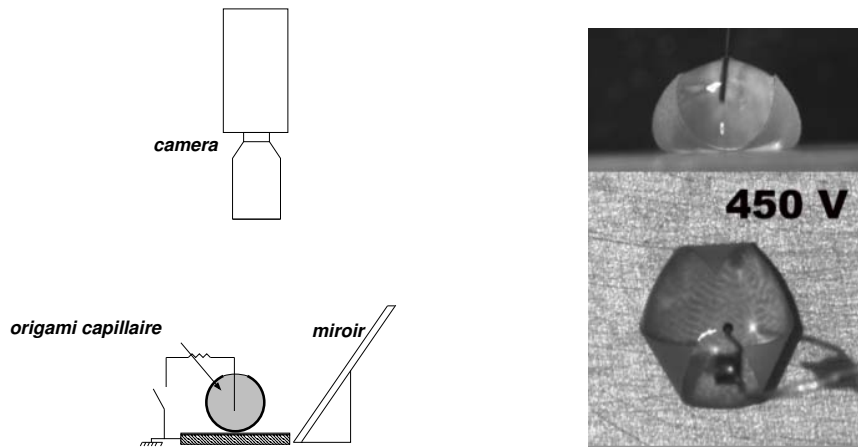
FIGURE 2.10 – À gauche : schéma de la disposition des éléments pour la prise des images. À droite : exemple d'image enregistrée avec la valeur de la tension appliquée correspondante.
