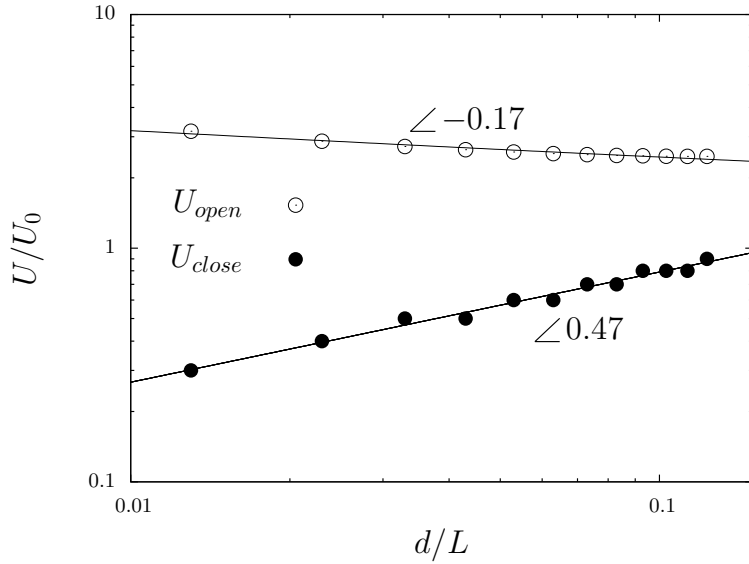
FIGURE 2.22 – Résultats de la simulation numérique pour les variations des tensions d'ouverture et de fermeture en fonction de l'épaisseur de la couche isolante.
