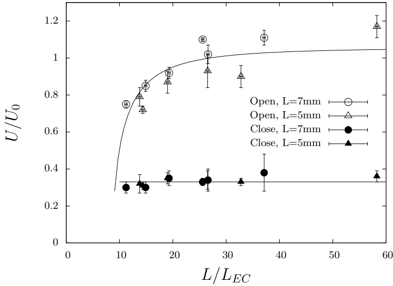
FIGURE 2.15 – Tensions d’ouverture et fermeture renormalisés par U_0 en fonction du rapport entre la longueur de la feuille et la longueur élastocapillaire. Les variations de la longueur élasto-capillaire ont été atteints en variant l’épaisseur de la feuille entre 50 et 100 \mu m ainsi qu’en variant le module d’élasticité du PDMS. L’épaisseur de la couche isolante demeure constant d = 50 \mu m . Pour les paramètres utilisés nous avons une tension caractéristique U_0 \sim 800 V . Les symboles ouverts représentent les tensions d’ouverture et les symboles solides les tensions de fermeture.
