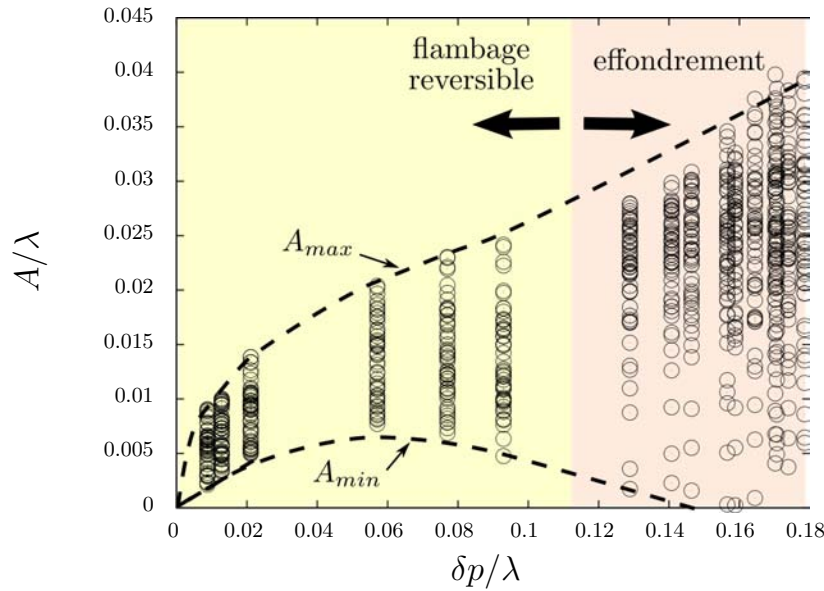
FIGURE 3.33 – Résultats expérimentaux sur l'amplitude des plis en fonction de la compression appliquée pour une couronne de 90\mu m d'épaisseur et de rapport d'aspect a/b = 0.65 .
