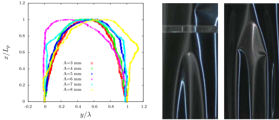
FIGURE 4.8 – (a) Profil du défaut de pliage pour des amplitudes des confinement croissantes. La symétrie parabolique est brisée pour les plus grandes amplitudes. (b) Focalisation de la déformation à grande amplitude : la feuille est froissée.
