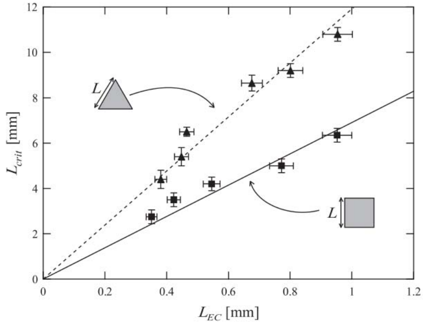
FIGURE 2.3 – Longueurs critiques de fermeture pour des feuilles carrées et triangulaires en fonction de la longueur élasto-capillaire. (Image extraite de [26]).
