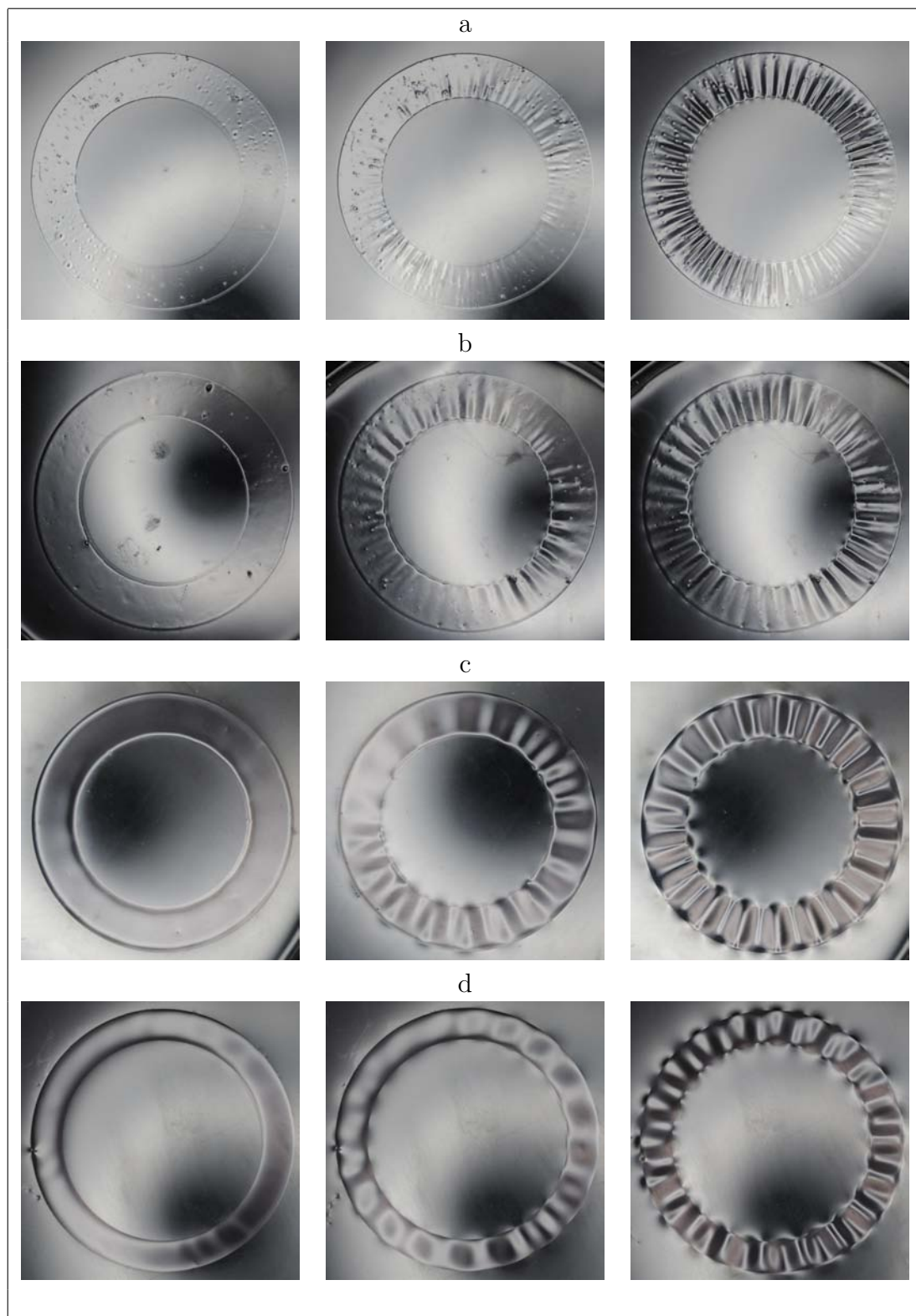
FIGURE 3.20 – Images des couronnes d'épaisseurs différentes durant leur déformation hors du plan. a) h = 16\mu m et a/b = 0.65 , b) h = 50\mu m et a/b = 0.65 , c) h = 81\mu m et a/b = 0.65 , d) h = 110\mu m et a/b = 0.70 . La valeur du rayon interne est a = 50mm dans tout les cas.
