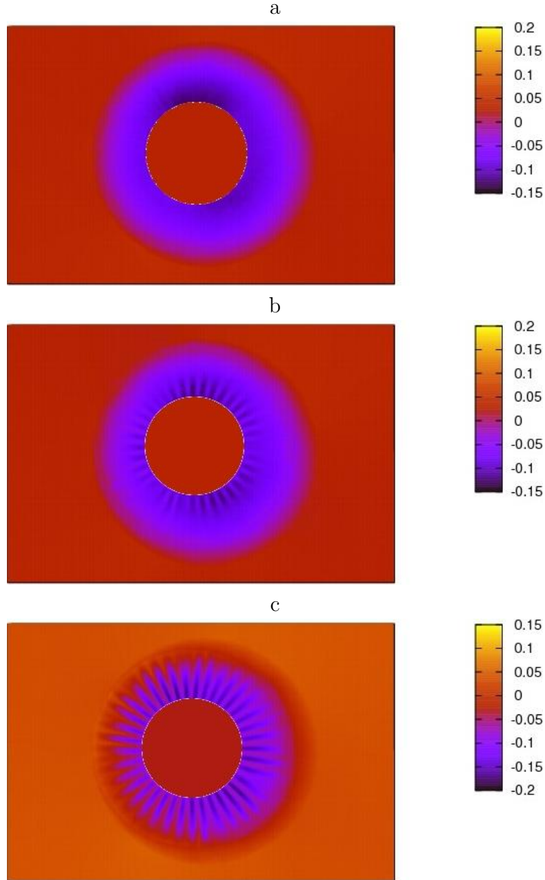
FIGURE 3.9 – Images des champs de hauteur obtenues à partir de PIVMat pour un anneau h = 30\mu m et a/b = 0.5 . Chaque image correspond à une valeur de \gamma_o/\gamma_i différent, a) \gamma_o/\gamma_i = 0.9 en dessous du seuil, b) 0.42 et c) 0.37. L'échelle est en mm .
