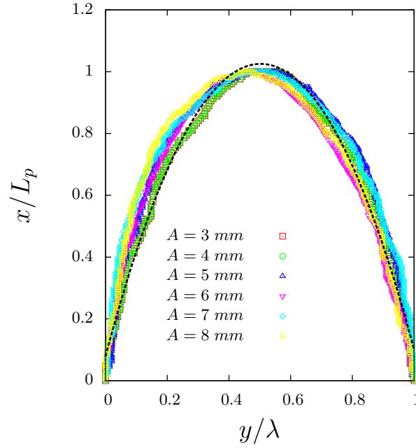
FIGURE 4.7 – Profil du défaut de pliage lors de la réunion de deux plis. L’adimensionnement par L_p et par \lambda permet d’obtenir une forme maîtresse (approximativement parabolique). La ligne pointillée correspond au fit parabolique de la forme a(0.5-x)^2+1 , avec a = -3.7 .
