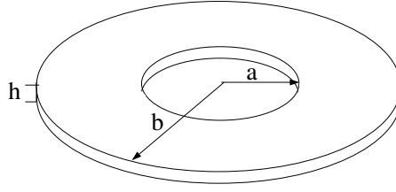
FIGURE 3.4 – Géométrie des couronnes.
