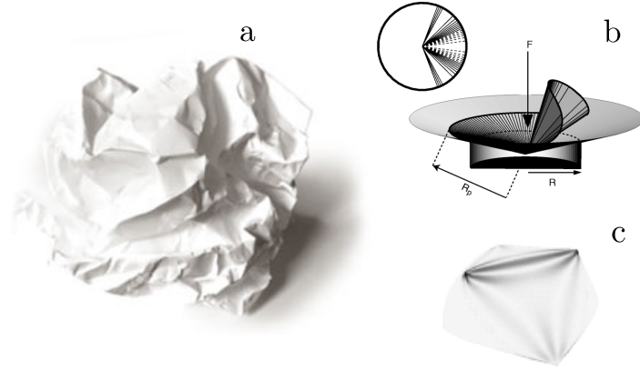
FIGURE 4.9 – Feuille comprimée à la main : les zones étirées sont focalisées en des points singuliers, ce qui permet de préserver une surface développable malgré le grand changement topographique imposé (a). Dans sa structure on peut trouver différents types de singularités, des cônes (b, clichés extraits de [72]) et ridges (c, clichés extraits de [73]).
