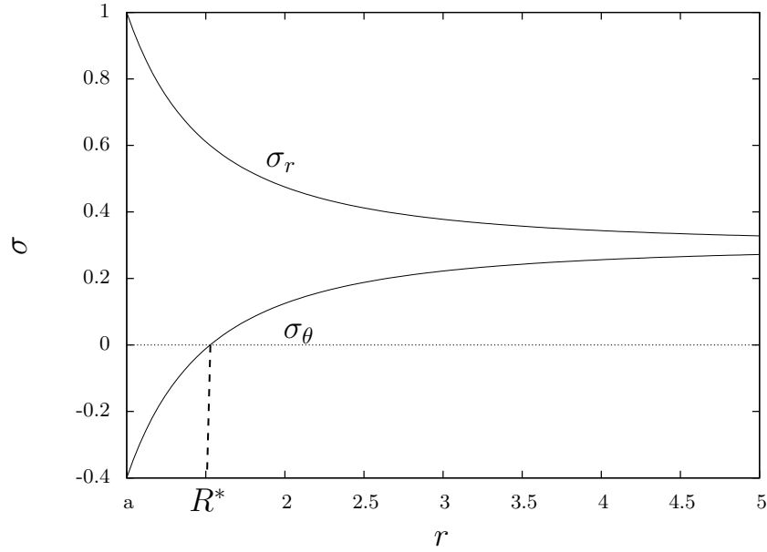
FIGURE 3.14 – Contraintes radiale et orthoradiale en fonction de la distance au rayon intérieur a de la couronne. Si la condition 3.25 est vérifiée, la contrainte orthoradiale est négative en dessous d'un certain seuil R^* .
