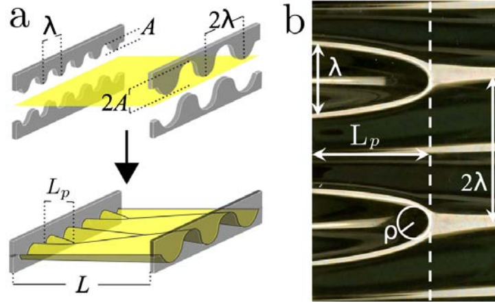
FIGURE 4.5 – (a) Expérience modèle permettant d’isoler le doublement de longueur d’onde des plis. En amont une longueur d’onde et une amplitude A sont imposées, alors qu’en aval les mords ont une longueur d’onde 2 et une amplitude 2A (qui permet de préserver la largeur de la feuille). (b) Plis vus du dessus, le doublement de longueur d’onde s’effectue à une distance L_p du premier mord (de longueur d’onde \lambda ).
