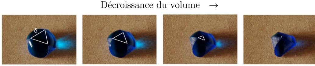
FIGURE 2.17 – Variation de la distance entre les coins de la feuille en fonction du volume de la goutte. Photos Charlotte Py.
