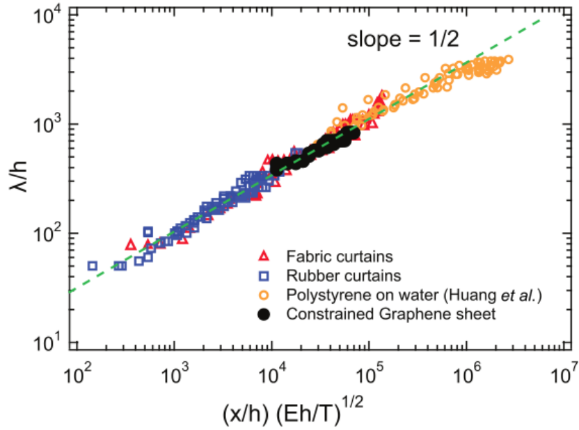
FIGURE 4.16 – Longueur d’onde en fonction de la distance au bord pour le régime sous tension. Les données incluent les résultats obtenus pour les rideaux en latex, pour le rideau long de Vandeparre [79], pour les membranes flottantes ultra-minces [30] et pour les membranes de graphène [80].
