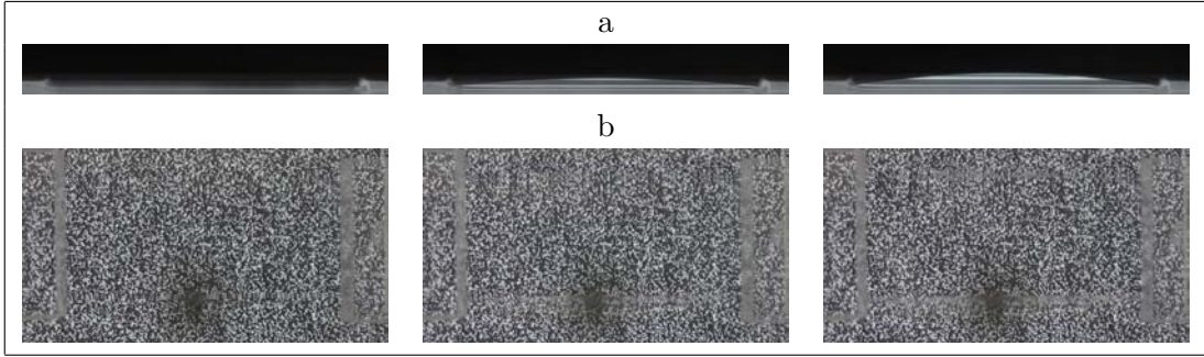
FIGURE 3.11 – Images de l'expérience de calibration, a) vue latérale et b) vue de dessus.
