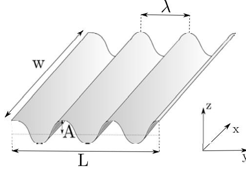
FIGURE 4.3 – Membrane de profil sinusoïdal d’amplitude A et de longueur d’onde \lambda .
