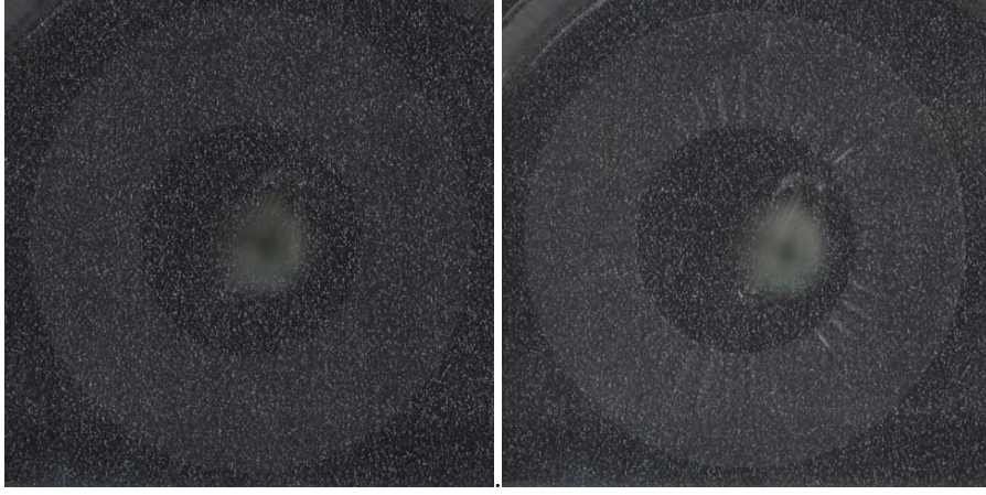
FIGURE 3.7 – Images de l’anneau avant et après déformation.
