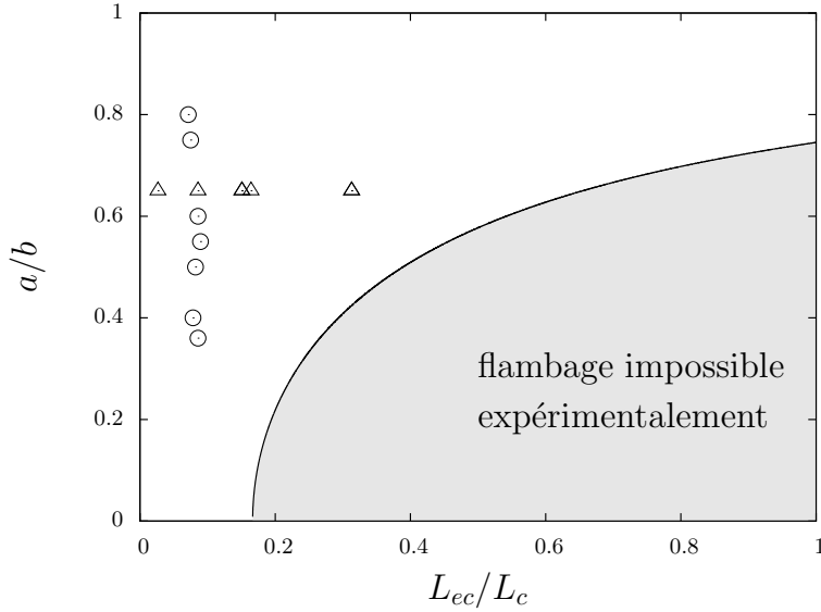
FIGURE 3.22 – Régions de susceptibilité de flambage dans une espace L_{ec}/L_c vs a/b . La ligne solide a été calculé à partir de l'équation 3.47 avec \sigma_o/\sigma_i = 1/3 . Les cercles et les triangles indiquent les caractéristiques des anneaux utilisés dans nos expériences.
