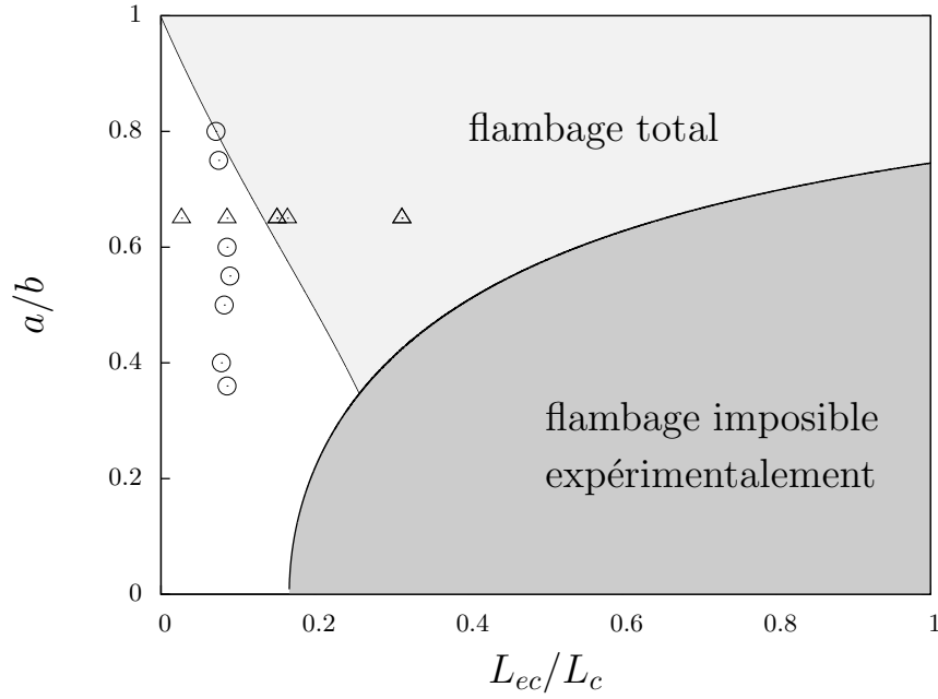
FIGURE 3.26 – Regions de susceptibilité de flambage dans une espace L_{ec}/L_c vs a/b . La ligne solide a été calculée à partir de l'équation 3.47 avec \sigma_o/\sigma_i = 1/3 . Les cercles et triangles indiquent les caractéristiques des anneaux utilisés dans nos expériences.
