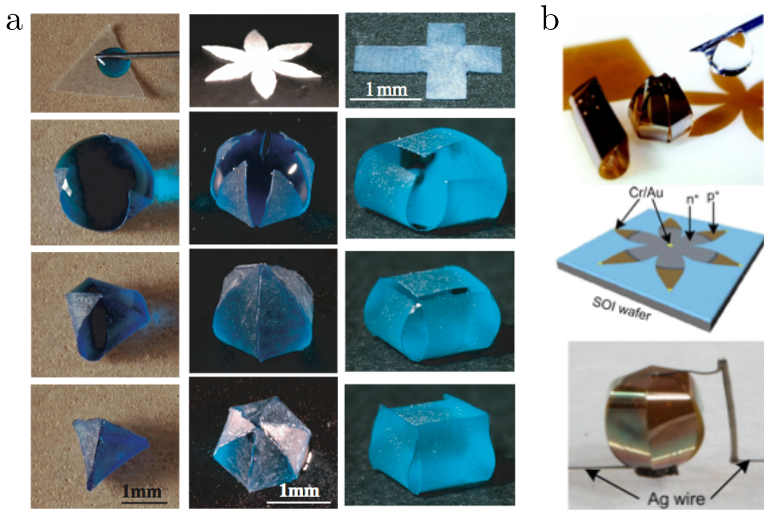
FIGURE 1.4 – (a) Origami capillaire : différentes formes tridimensionnelles peuvent être obtenues en fonction de la découpe initiale de la feuille. (b) Utilisation de la technique d'origami pour réaliser des capteurs solaires tridimensionnels (clichés X. Guo [27]) .
