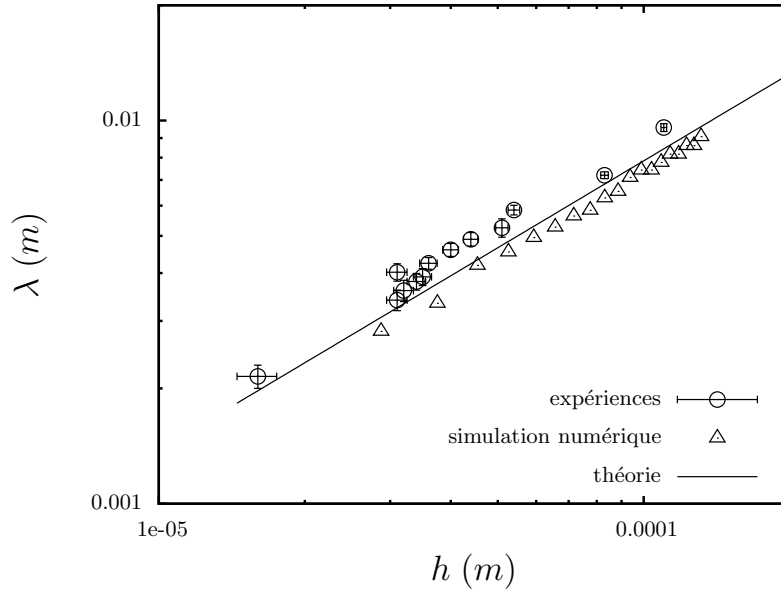
FIGURE 3.19 – Valeurs expérimentales (cercles) et numériques (triangles) pour la longueur d’onde en fonction de l’épaisseur de l’anneau. La ligne continue correspond à l’expression théorique \lambda \sim 2\pi(E/(12(1-\nu^2)\rho g))^{1/4}h^{3/4} .
