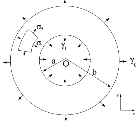
FIGURE 3.13 – Élément infinitésimal pour le calcul des contraintes.
