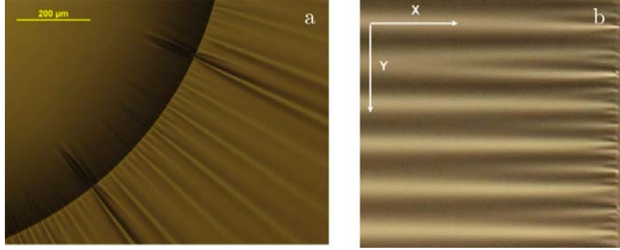
FIGURE 1.6 – Variation de la longueur d’onde près de la ligne de contact, a) rides générés par la déposition d’une goutte sur une membrane flexible flottant dans l’eau (cliché N.Menon), b) plissement d’une membrane flottante à la suite d’une compression mécanique latérale [30].
