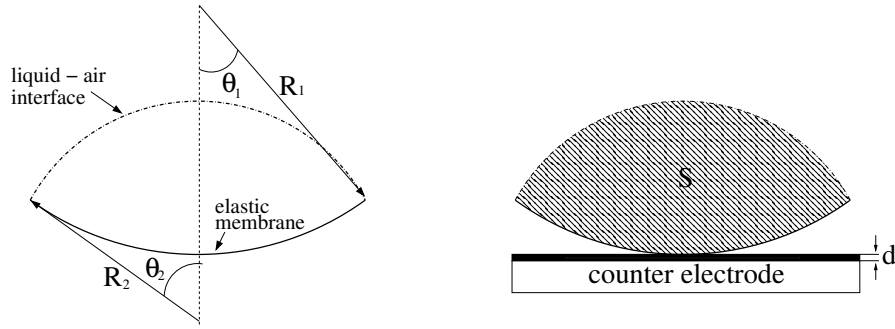
FIGURE 2.19 – Schéma du modèle 2-D.
