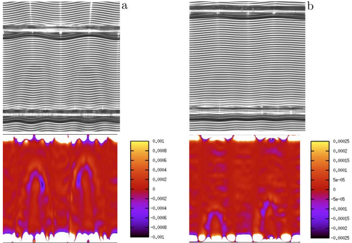
FIGURE 4.11 – Mesures de la courbure de gauss à partir du profil de hauteur d'une feuille déformée. L'épaisseur de la feuille est h = 50 \mu m . a) profil imposé au bord A = 5 mm , \lambda = 24 mm , b) A = 3 mm , \lambda = 24 mm . Nous avons utilisé une technique de profilométrie développé par Maurel et al. [76] pour réaliser les mesures du profil.
