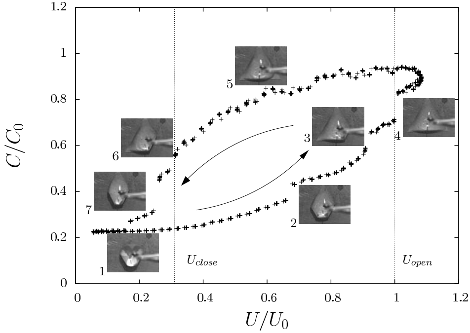
FIGURE 2.14 – Capacité du système le long de 5 cycles d'ouverture et de fermeture successifs. C_0 correspond à la capacité d'un condensateur de plaques parallèles de surface triangulaire de côté L = 7\text{mm} .
