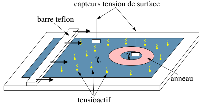
FIGURE 3.5 – Dispositif expérimental.
