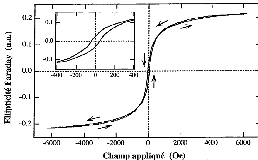
Figure V.16. : On note l'apparition d'un hystérésis lors des mesures d'ellipticité Faraday d'échantillons préparés sous champ statique (ici, l'exemple d'un gel synthétisé sous champ perpendiculaire à sa surface). Cet hystérésis confirme l'existence de particules de ferrofluide dont l'orientation est gelée.
