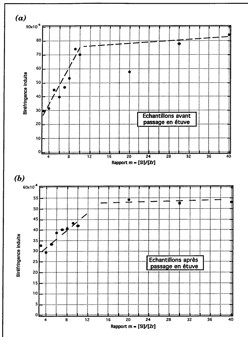
Figure II.9 : Biréfringences induites à saturation dans des gels mixtes Zr-Si dopés par des molécules de rhodamine 640, pour divers taux de zirconium : (a) avant passage en étuve sèche, (b) après passage en étuve. Les lignes pointillées sont des guides pour les yeux.
