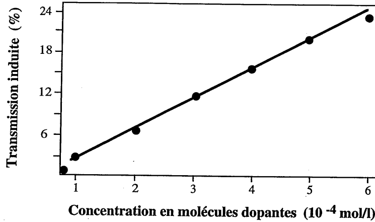
Figure I.11. : Évolution de la biréfringence induite à saturation, en fonction du nombre de molécules optiquement actives dopant le gel.
