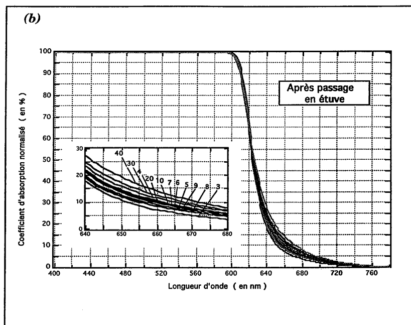
Figure II.8. : Spectres d'absorption des gels mixtes de silice et de zircone à taux de zirconium variable, selon le rapport molaire m = [Si]/[Zr] : (a) avant séchage en étuve, (b) après séchage en étuve.
