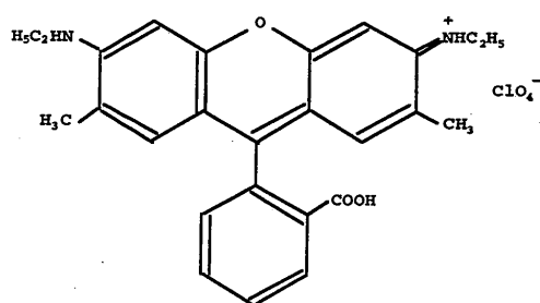
Rhodamine 19 Rhodamine 575
