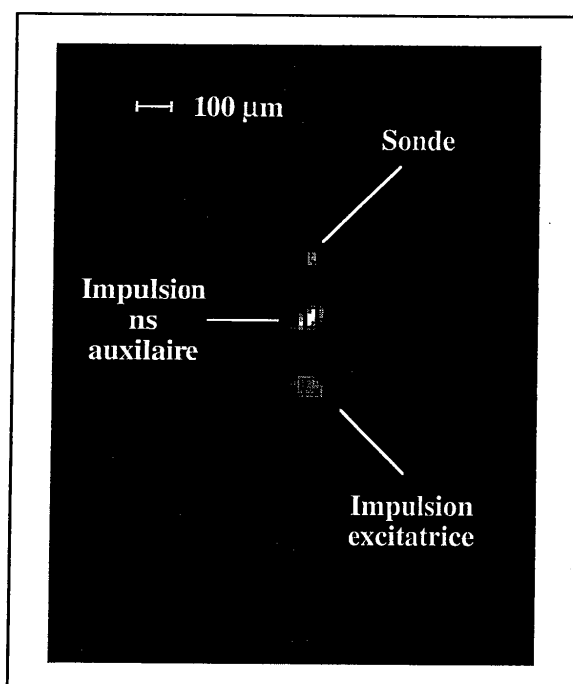
Figure II.19. : Tailles relatives des faisceaux lumineux sur la face avant de l'échantillon. L'image a été enregistrée à l'aide d'une caméra CCD. En configuration expérimentale, les spots sont spatialement confondus.
