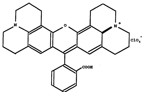
Rhodamine 640 Rhodamine 101
