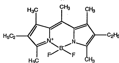
Pyrrométhène 567
