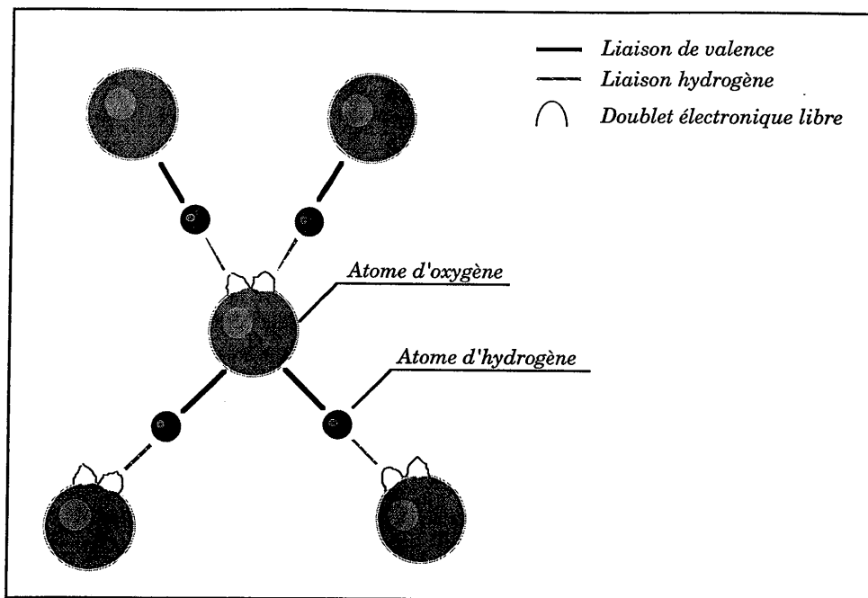
Figure I.18. : Principe de l'établissement de liaisons hydrogène, dans le cas simple et classique de la molécule d'eau.
