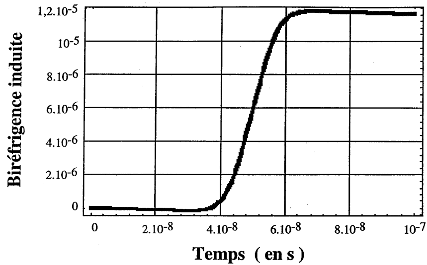
Figure III.2. : Simulation numérique de la réponse orientationnelle impulsionnelle de dopants soumis à une impulsion dont la composante nanoseconde apporte une énergie de 15 \mu\text{J} pendant 10 ns.
