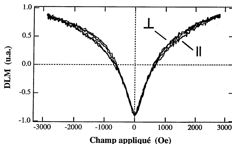
Figure V.14 : Comparaison des dichroïsmes linéaires magnétiques à 543,5 nm de deux échantillons préparés sous champ magnétique statique, respectivement parallèle (||) et perpendiculaire (⊥) à la surface du gel. Le champ appliqué lors de la mesure est, lui, parallèle à la surface des échantillons.
