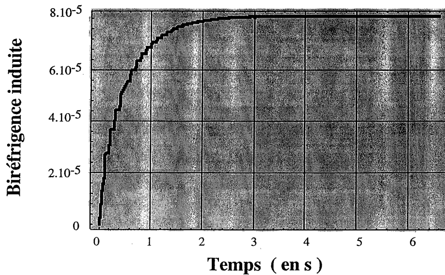
Figure III.3. : Évolution simulée de la biréfringence induite au sein d'une assemblée de molécules en rotation en fonction du nombre d'impulsions incidentes.
