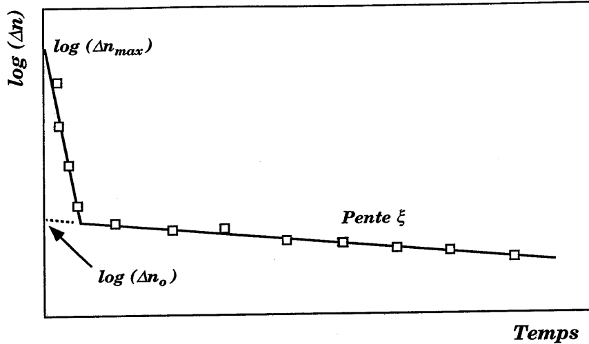
Figure II.2 : Représentation schématique semi-logarithmique d'une cinétique de relaxation classique de l'anisotropie moléculaire photo-induite. Introduction des paramètres caractéristiques repris tout au long de l'étude.
