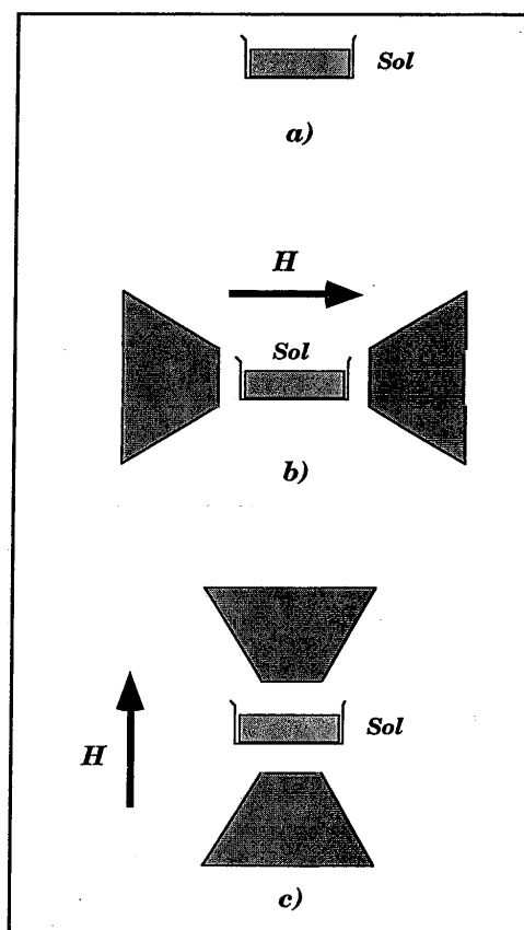
Figure V.12. : Les trois types d'échantillons synthétisés (a) sans champ statique appliqué, (b) sous champ parallèle à la surface de l'échantillon, (c) sous champ perpendiculaire à la surface de l'échantillon
