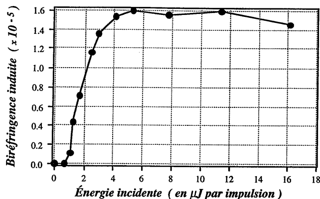
Figure V.5. : Réponse d'un gel dopé par un ferrofluide de maghémite à l'application d'un trains d'impulsions lumineuses ultra-brèves. On notera l'analogie avec le comportement de dopants organiques.
