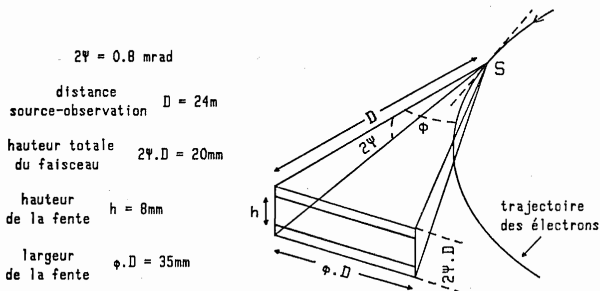
Figure 2.2(1) : Schéma du faisceau synchrotron utilisé au LURE - DCI .
