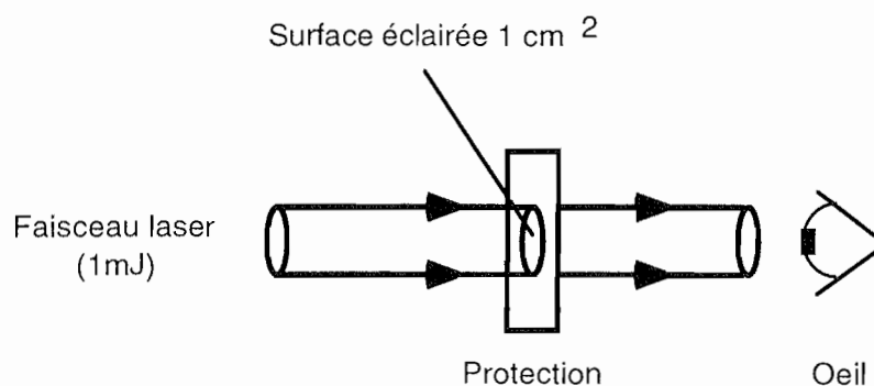
Figure 3. Limiteur optique sans plan focal intermédiaire.
