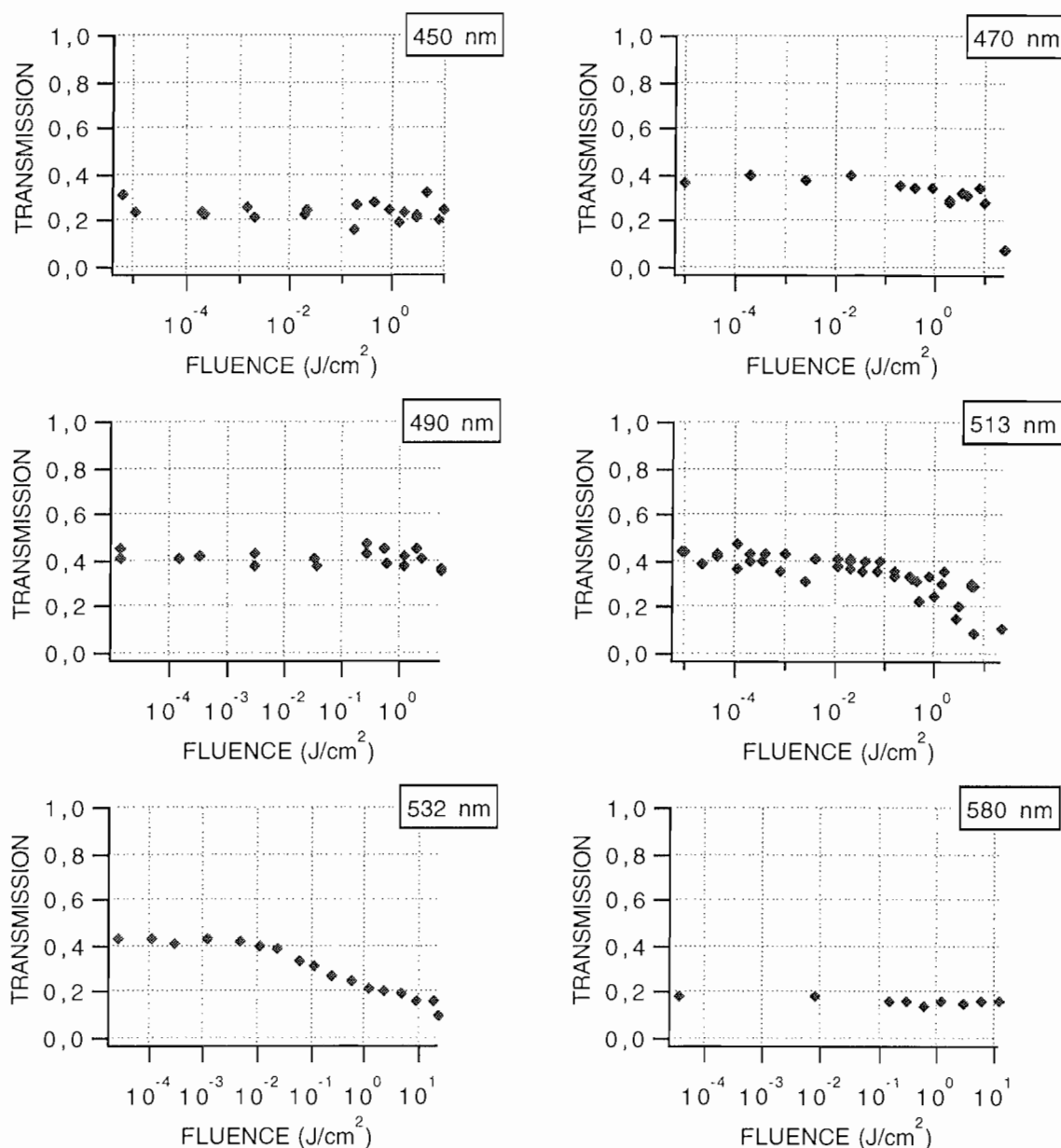
Figure 76. Résultats expérimentaux obtenus avec la matrice VTEOS dopée avec des molécules de HITCI aux différentes longueurs d'onde d'étude.
