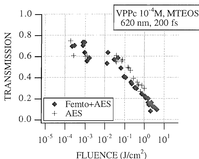
Figure 100. Mesure de la transmission d'une matrice MTEOS dopée avec des molécules de la famille des vanadyl-phtalocyanines en fonction de la fluence incidente pour des impulsions de durée 100 fs environ à la longueur d'onde 620 nm, et pour des impulsions dues uniquement à de l'amplification par émission spontanée (AES).
