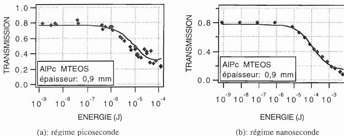
Figure 31. Extrapolations avec un modèle à quatre niveaux des résultats expérimentaux obtenus avec une matrice MTEOS* dopée avec des chloro-alumino-phtalocyanines (CIAIPc).
