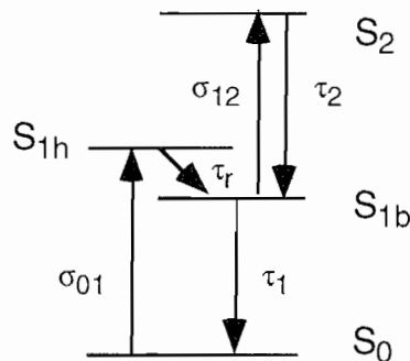
Figure 93. Modèle simple à quatre niveaux d'énergie pour expliquer le processus de transmission saturable.
