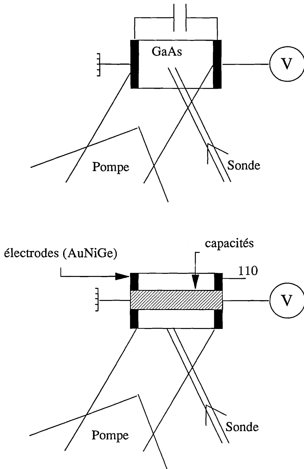
Fig V.2: Application d'un champ statique sur GaAs semi-isolant.
