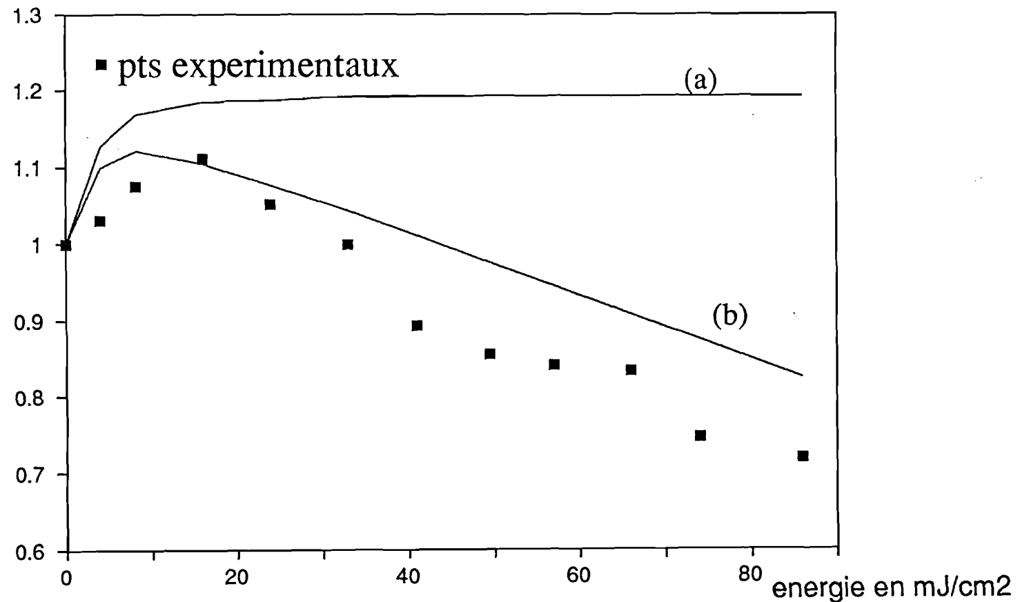
Fig IV.4: Variation de transmission de GaAs semi-isolant en fonction de l'énergie incidente. Les courbes théoriques (a-b) représentent la variation de transmission en tenant compte uniquement de l'évolution de EL2+ (a), ou bien de l'évolution de EL2+, de l'absorption à 2 photons et l'absorption par les porteurs libres (b).
