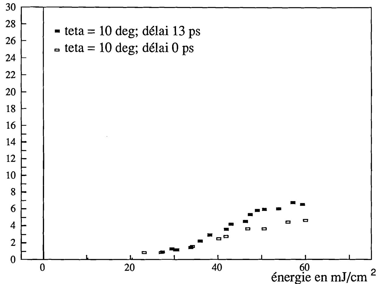
Fig V.11: Gain en fonction de l'énergie totale lorsque pompe et sonde sont en coincidence (□) et lorsque la pompe est en retard de 13 ps par rapport à la sonde (■).
