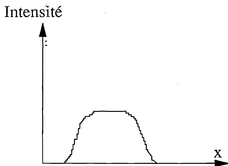
Fig IV.3: repartition de l'intensité dans la tache laser.
