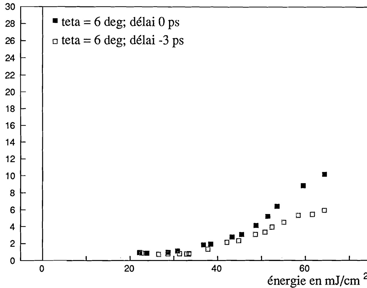
Fig V.10: Gain en fonction de l'énergie totale lorsque pompe et sonde sont en coincidence (■) et lorsque la pompe est en avance de 3 ps par rapport à la sonde (□).
