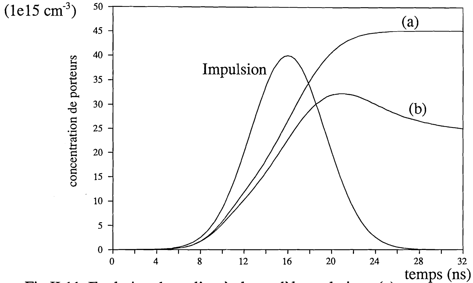
Fig II.11 Evolution de n_0 d'après le modèle analytique (a) et d'après les simulations (b) pour une énergie totale de 30 \text{ mJ/cm}^2
