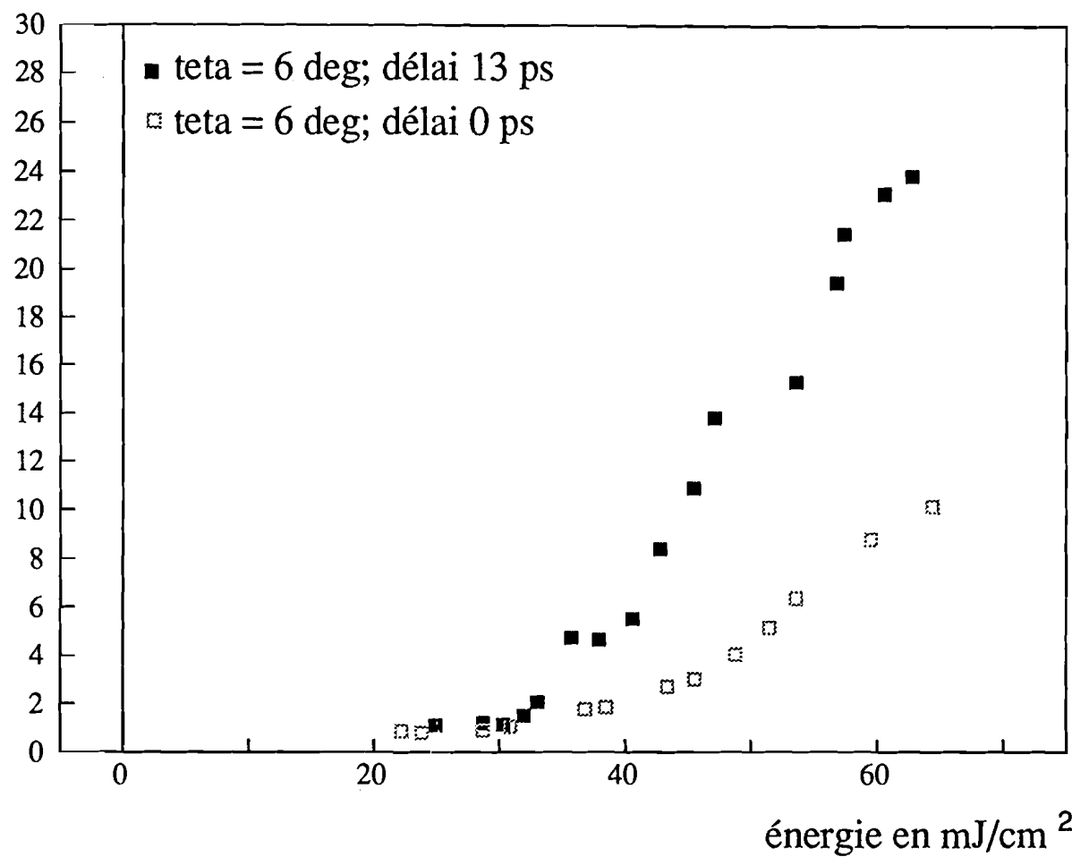
Fig V.8: Gain en fonction de l'énergie totale lorsque pompe et sonde sont en coincidence (□) et lorsque la pompe est en retard de 13 ps par rapport à la sonde (■).
