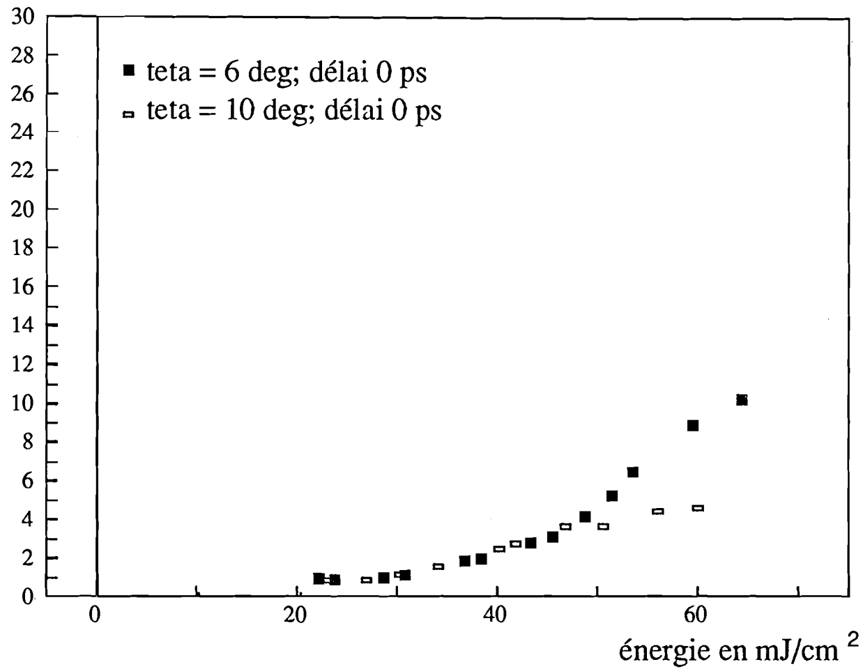
Fig V.7: Gain en fonction de l'énergie totale pour deux angles d'incidences entre les impulsions.
