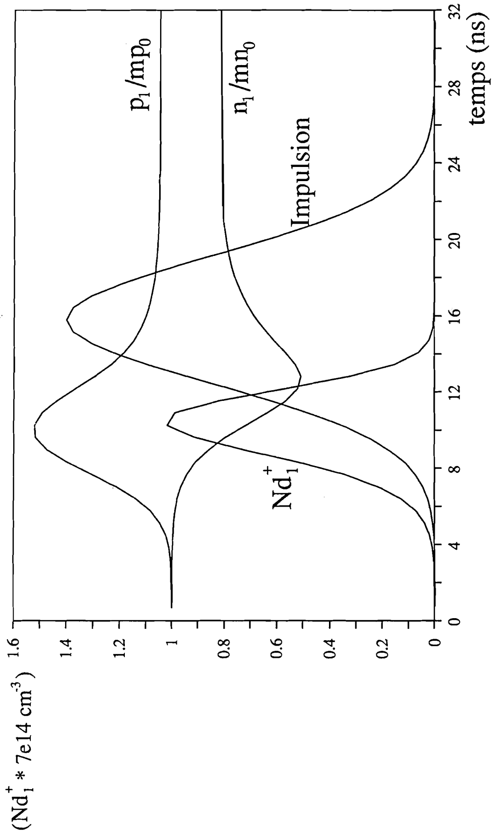
Fig II.5 Evolution d'après le modèle analytique de n_1/mn_0 , p_1/mp_0 et \text{Nd}_1^+ pour une énergie totale de 30 \text{ mJ/cm}^2
