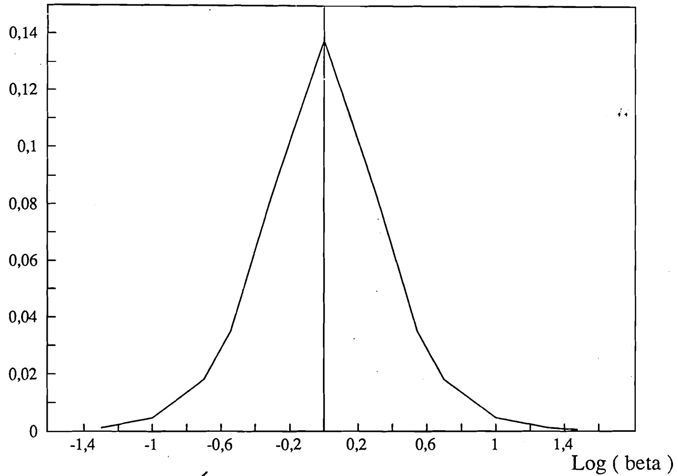
Fig III.6 Reflectivité du mélange à quatre ondes en fonction du rapport \beta des intensités des deux pompes.
