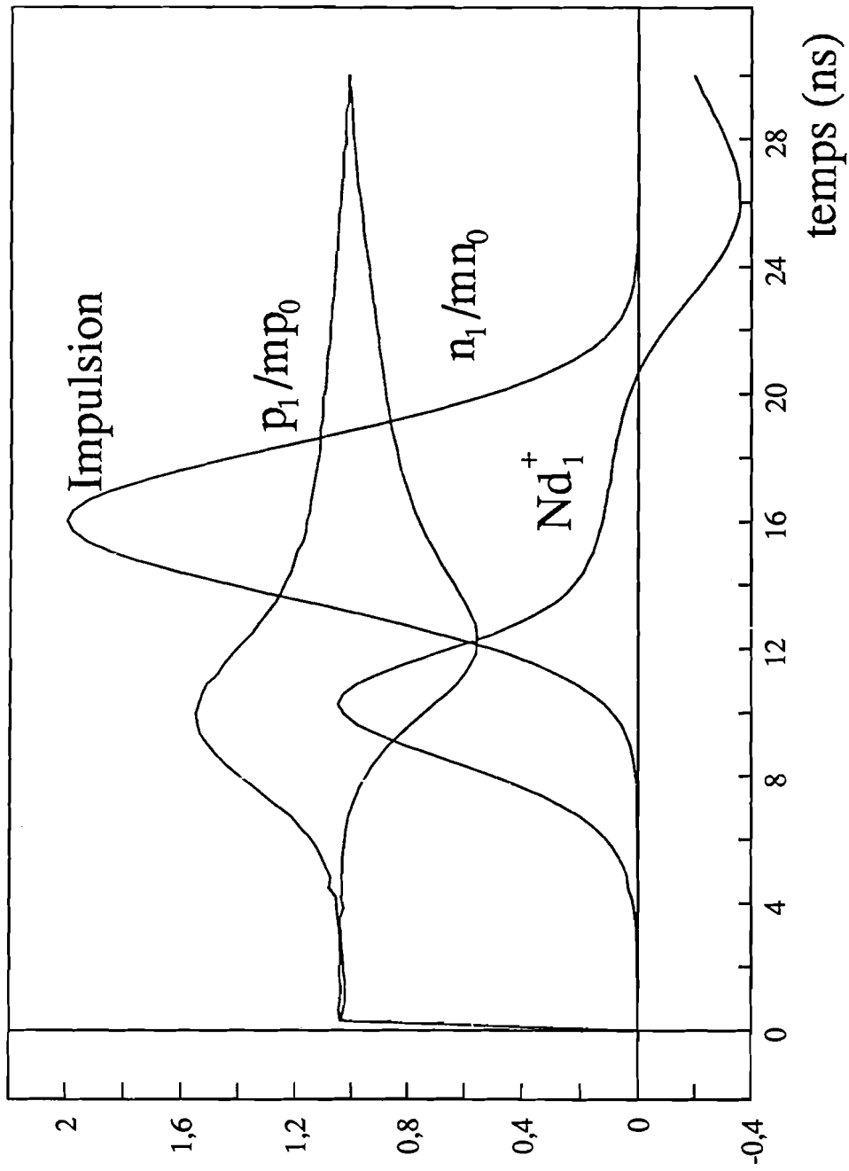
Fig II.14 Evolution d'après les simulations de p_1/mp_0 et n_1/mn_0 pour une énergie totale de 30 \text{ mJ/cm}^2
