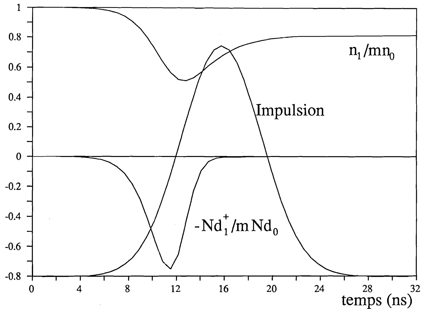
Fig II.7 Evolution d'après le modèle analytique de n_1/mn_0 et -Nd_1^+/mNd_0 pour une énergie totale de 30 \text{ mJ/cm}^2
