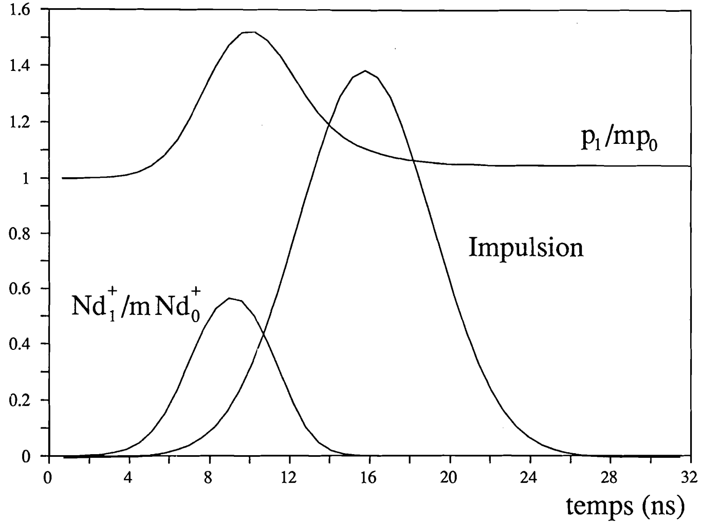
Fig II.6 Evolution d'après le modèle analytique de p_1/mp_0 et Nd_1^+/mNd_0^+ pour une énergie totale de 30 \text{ mJ/cm}^2
