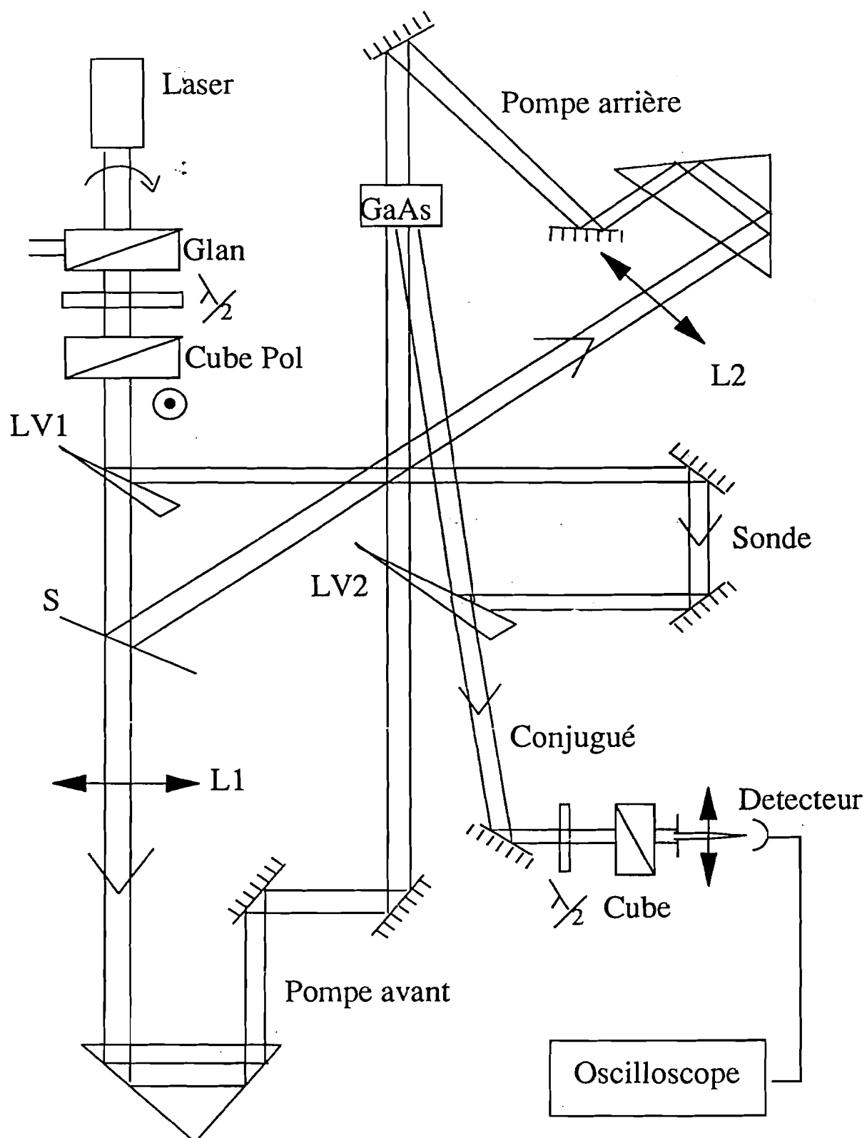
Fig IV.1: Montage expérimental de conjugaison de phase par l'arrière.
