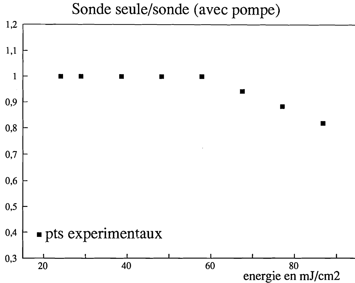
Fig IV.7: Variation de transmission de GaAs semi-isolant mince ( l = 500 micron ) en fonction de l'énergie incidente.
