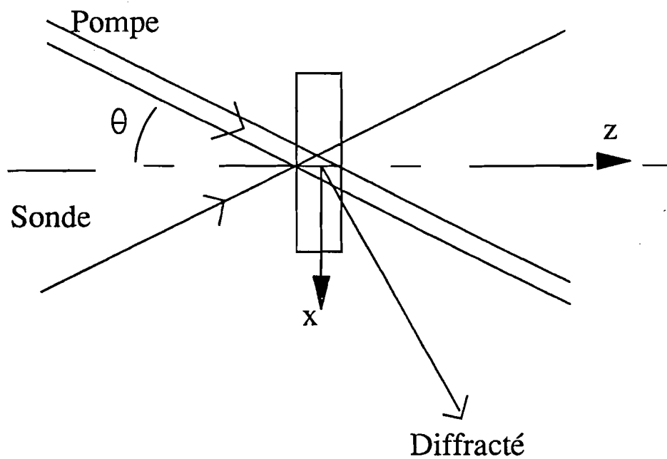
Fig III.1: montage de conjugaison de phase par l'avant.
