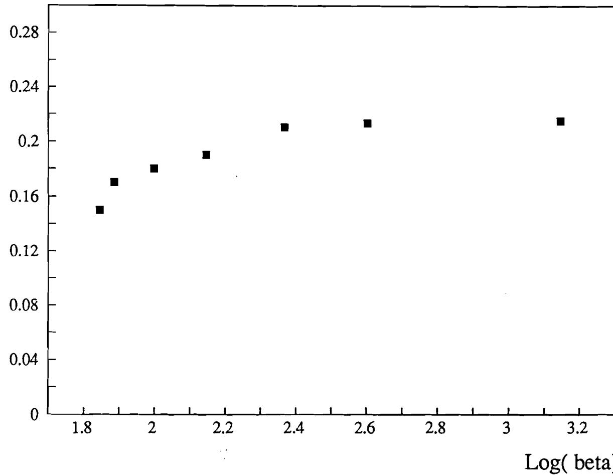
Fig IV.12: Variation de la réflectivité dans GaAs semi isolant épais en fonction du rapport \beta entre la pompe et la sonde pour une energie de 80 mJ/cm 2 .
