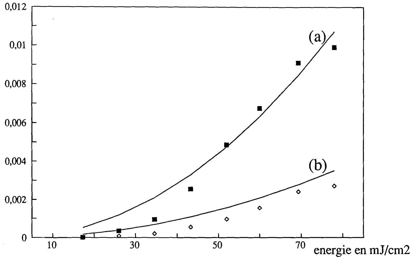
Fig IV.13: Réflectivité en conjugaison de phase par l'arrière dans GaAs dopé n en fonction de l'énergie incidente lorsque les polarisations des pompes sont parallèles (■) ou croisées (◇). Les courbes théoriques (a) et (b) sont déduites des équations III.10 et III.11.
