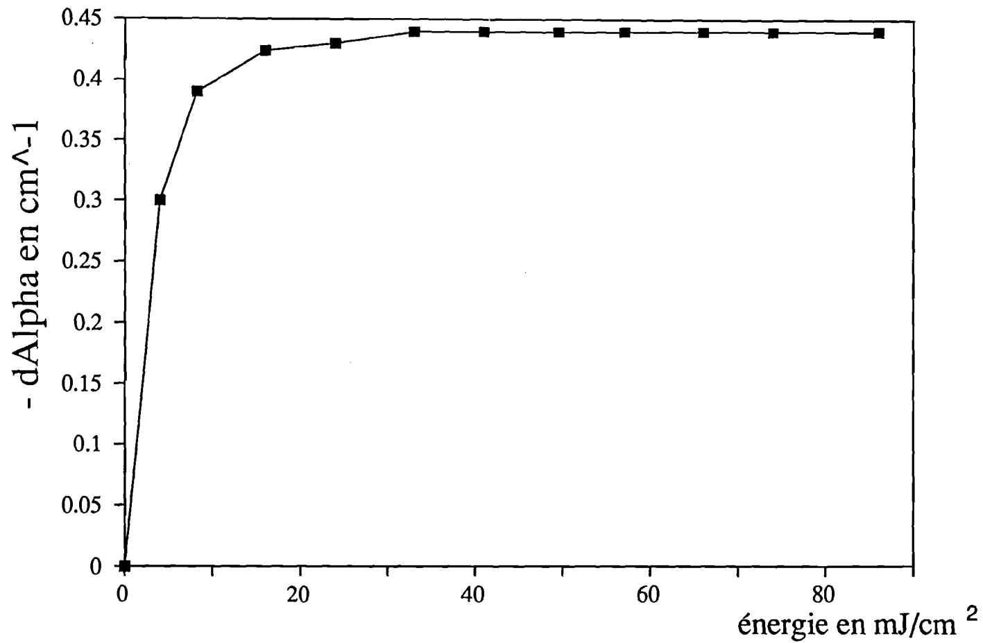
Fig II.17: Variation de l'absorption ( d\alpha ) due aux centres EL2 en fonction de l'énergie incidente.
