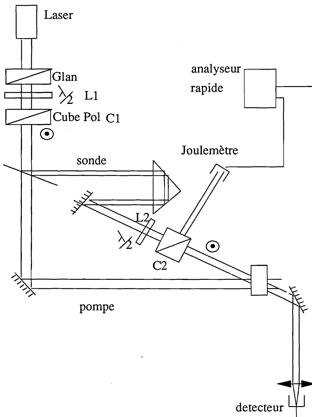
Fig V.5: Montage expérimental de couplage d'onde en picoseconde.
