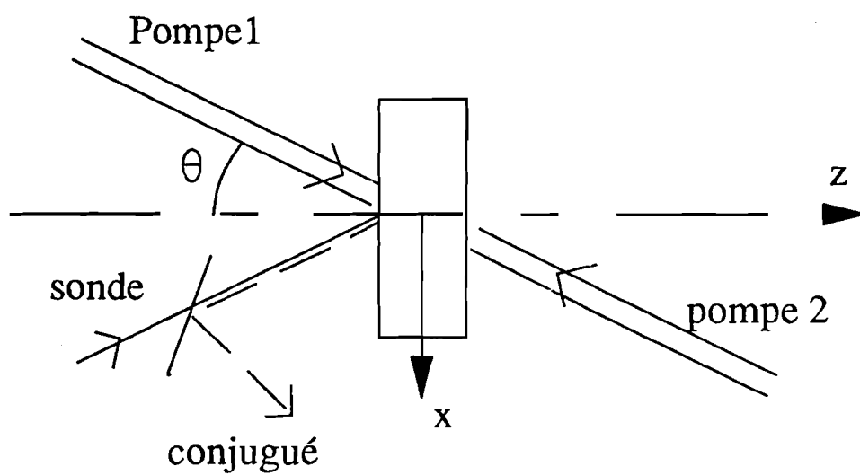
Fig III.2: montage de conjugaison de phase par l'arrière.
