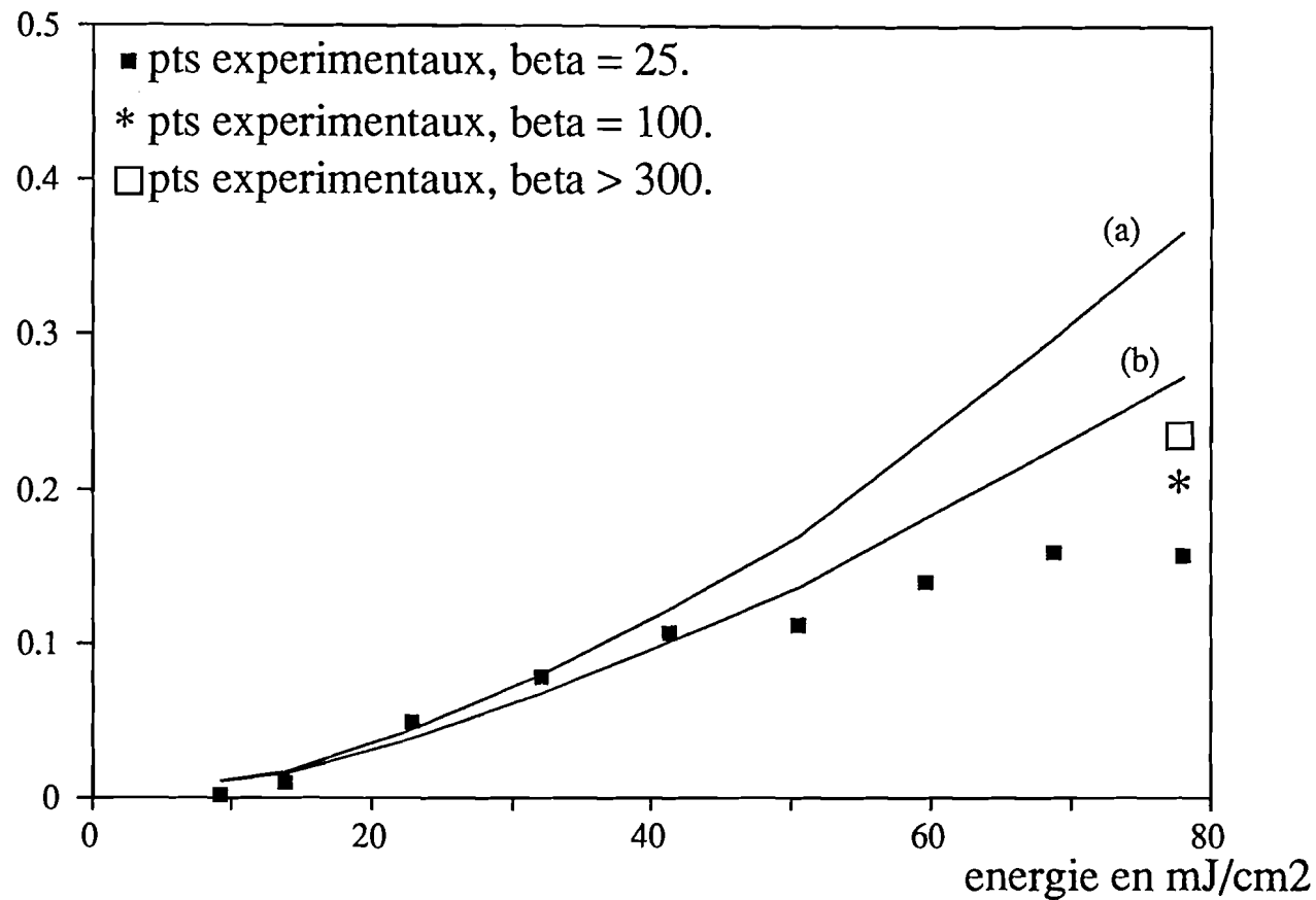
Fig IV.15: Réflectivité en fonction de l'énergie incidente dans GaAs semi-isolant épais. Les courbes théoriques (a) et (b) sont déduites de l'équation III-9. La variation d'indice est calculée soit par le modèle de Drude-Lorentz (a) soit en tenant compte de ce modèle et du mouvement anharmonique des porteurs photocréés (b).
