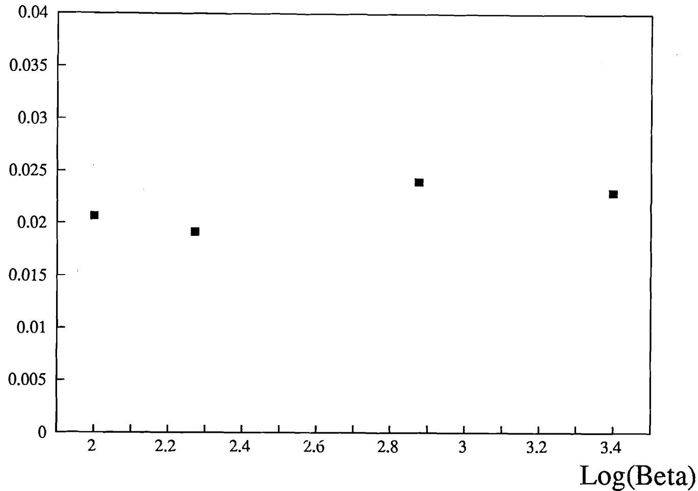
Fig IV.8: Variation de la réflectivité en conjugaison de phase par l'avant dans GaAs semi-isolant en fonction du rapport beta entre la pompe et la sonde pour une énergie incidente de 86 mJ/cm 2 .
