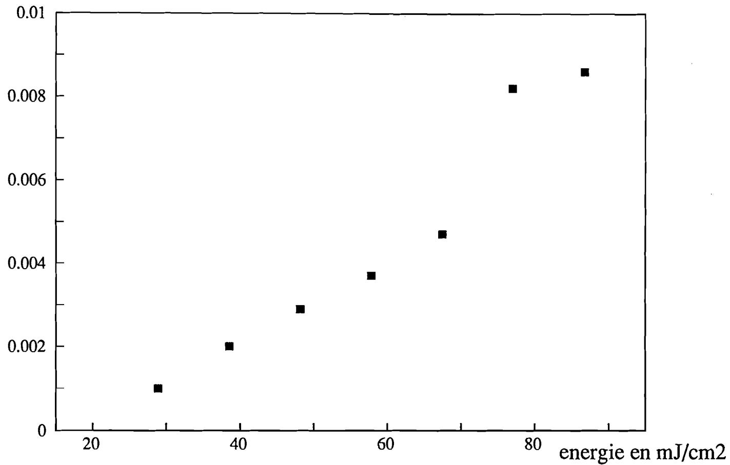
Fig IV.14: Réflectivité en conjugaison de phase par l'avant dans GaAs dopé n en fonction de l'énergie incidente.
