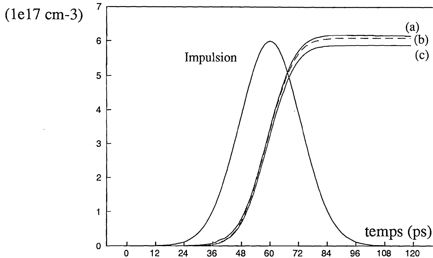
Fig V.4: Evolution de n_0 et p_0 d'après les simulations numériques pour une énergie totale de 20 \text{ mJ/cm}^2 . Les densités d'électrons (a) et de trous (b) sont calculées en tenant compte des centres EL2, tandis qu'intervient seulement l'absorption à deux photons dans la courbe (c) (électrons ou trous).
