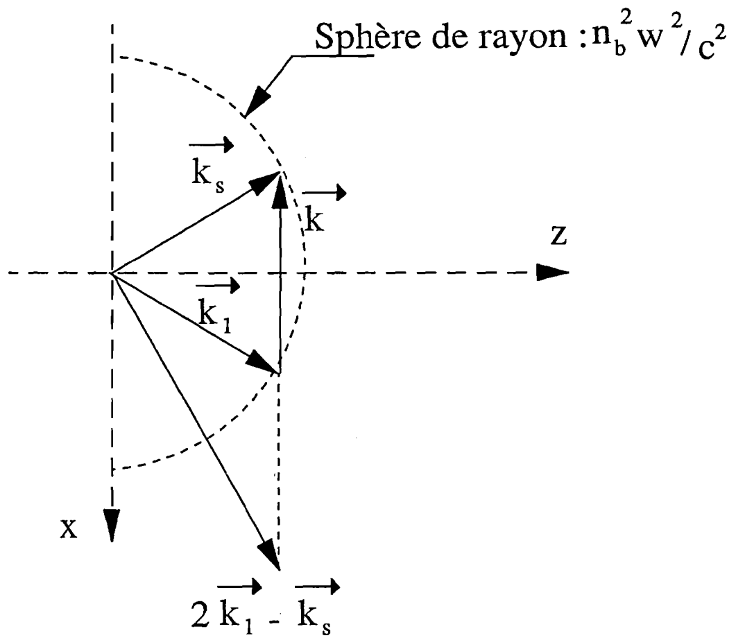
Fig III.3: Désaccord à Bragg du faisceau diffracté
