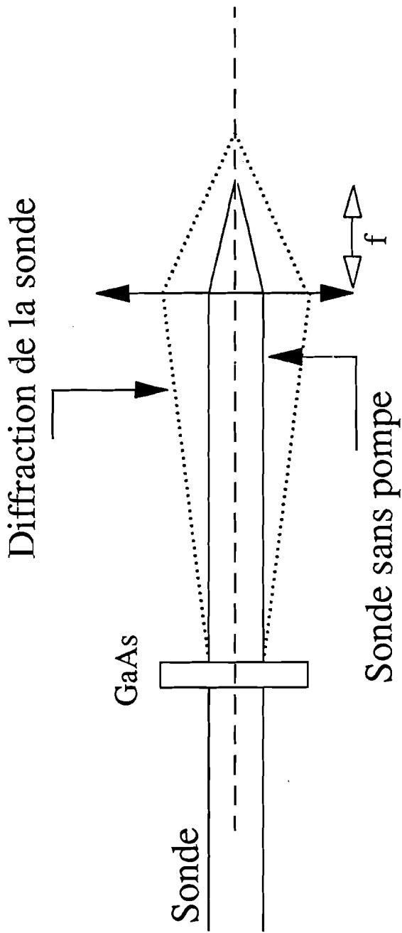
Fig V.6: diffraction de la sonde en présence de pompe.
