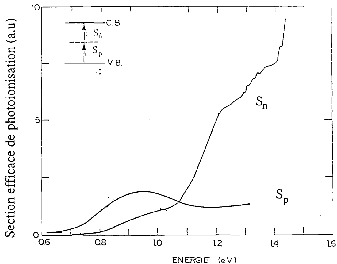
Fig II.2: spectre des sections efficaces de photoionisation du niveau EL2.
