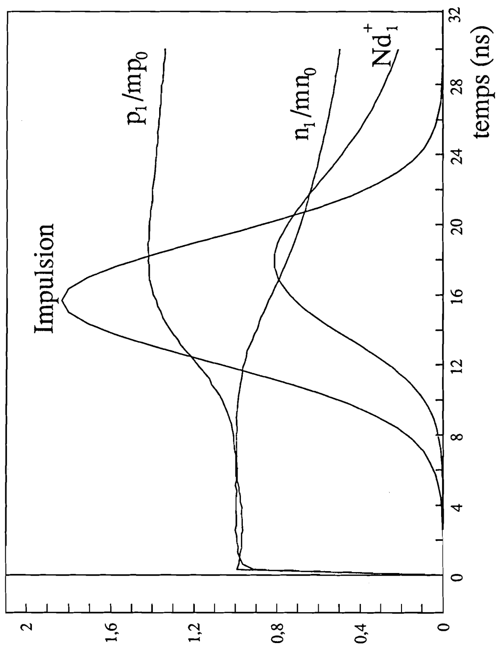
Fig II.13 Evolution d'après les simulations de p_1/mp_0 et n_1/mn_0 pour une énergie totale de 1 \text{ mJ/cm}^2
