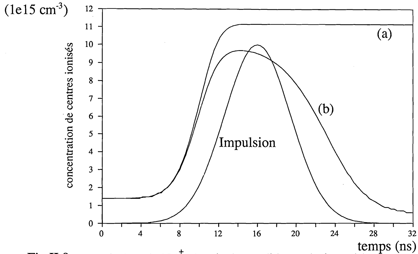
Fig II.9 Evolution de \text{Nd}_0^+ d'après le modèle analytique (a) et d'après les simulations (b) pour une énergie totale de 30 \text{ mJ/cm}^2
