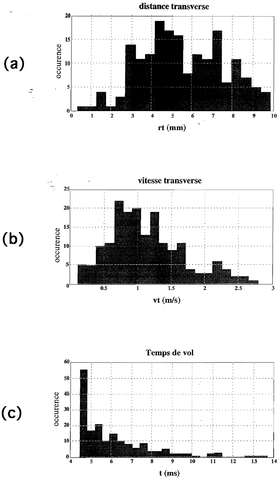
Figure A.IV-5 : distribution des atomes ralentis.
