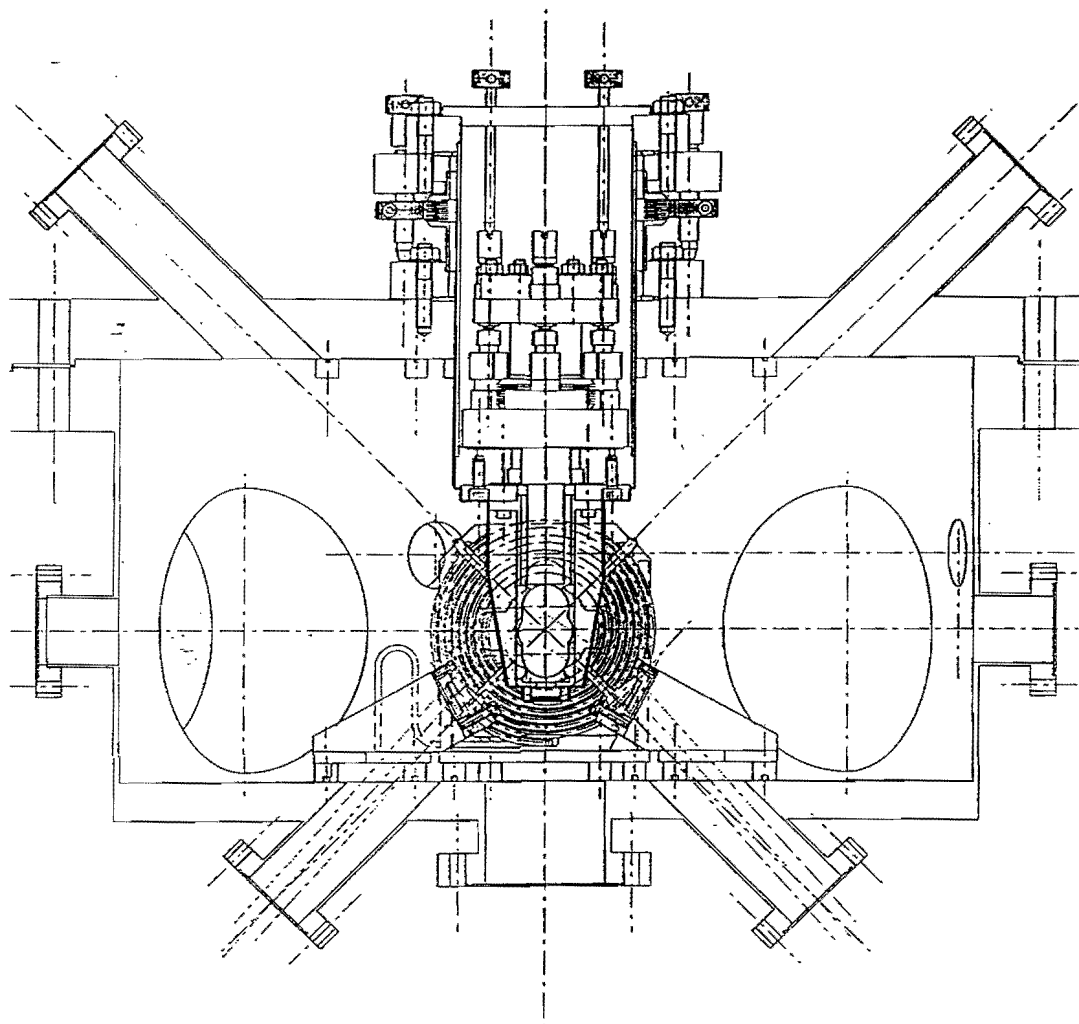
Figure A.I-1 : Coupe verticale de l'enceinte ultravide incluant la cavité. L'axe horizontal correspond à la direction du jet atomique. Les deux directions orthogonales entre elles, faisant 45^\circ avec cet axe, débouchent sur des hublots qui laissent passer les faisceaux du piège copropageants et contrepropageants. Dans la région centrale, on distingue les enroulements des bobines de champ magnétique. L'ensemble mécanique qui part de cette zone centrale et qui surmonte l'enceinte constitue la cavité interférométrique, conçue par P. Fournet, dessinateur à l'institut d'optique. L'axe joignant les centres optiques des deux miroirs est vertical. Entre les deux miroirs, tout à fait au centre de la figure, on remarque une ouverture qui permet le passage du troisième axe de faisceaux piégeants. Cet axe est horizontal et perpendiculaire au plan de la figure. A l'extérieur de l'enceinte, on distingue les vis de réglage qui agissent sur les deux sous-ensembles mécaniques qui sont solidaires chacun d'un miroir : la transmission des mouvements dans l'enceinte est possible grâce à deux soufflets étanches.
