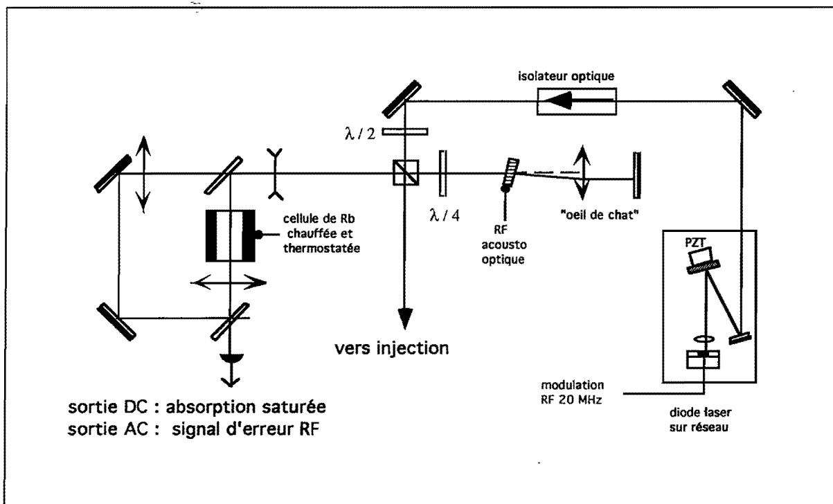
Figure B.III-3 : réalisation du laser "maître"
