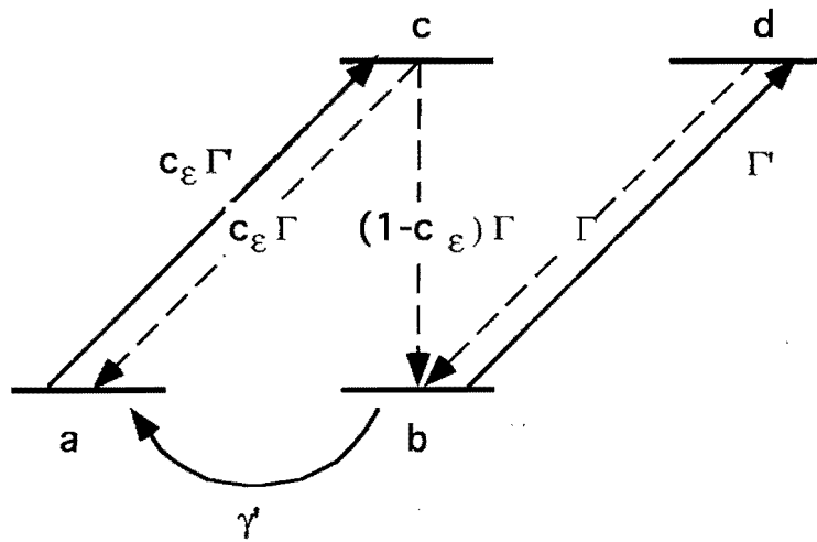
Figure A.III-3 : Mod \text{\e}le \text{\a} quatre niveaux pour inclure ph \text{\e}n\text{\u00f4}m\text{\e}n\text{\u00f4}logiquement les effets d \text{\u00f4}s au pompage optique
