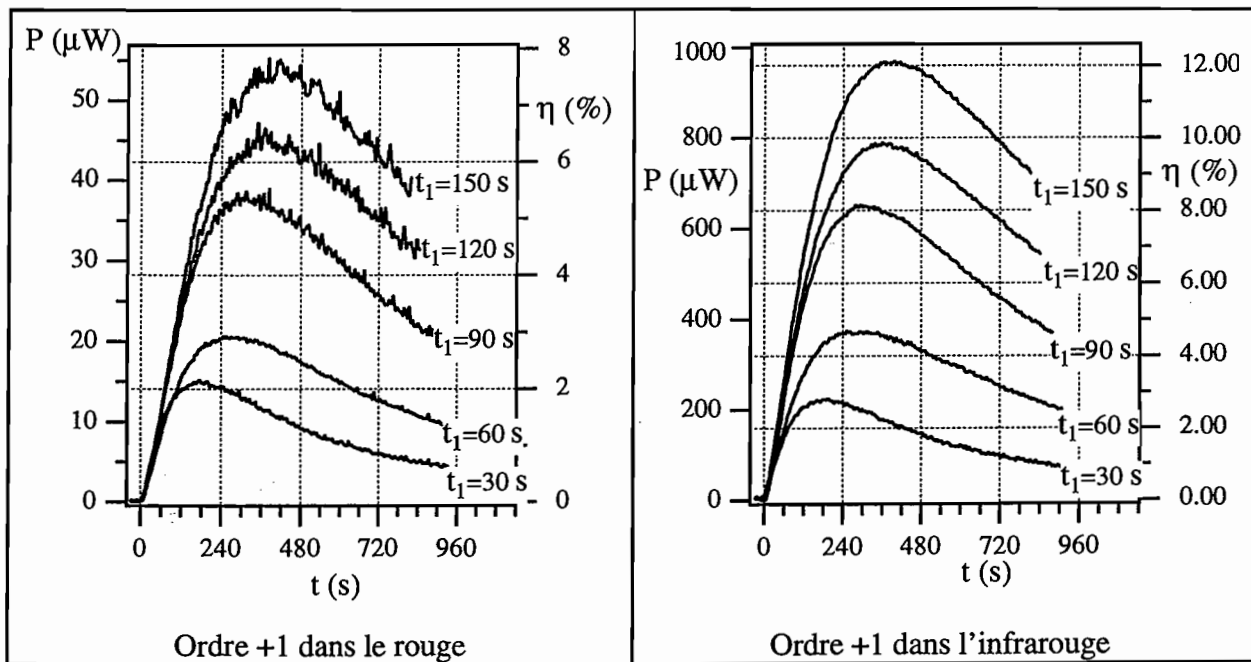
Figures 8 et 9: Rendements de diffraction d'un échantillon PMMA/Spiropyrane ( p=14,2 \mu\text{m} ); t=0 correspond au début de l'écriture dans le visible et à la fin du pompage U.V.. P(400\text{ nm})=215 \mu\text{W} sur \varnothing=4 mm, P(633\text{ nm})=705 \mu\text{W} sur \varnothing=4 mm et P(829\text{ nm})=8 mW sur \varnothing=2 mm.
