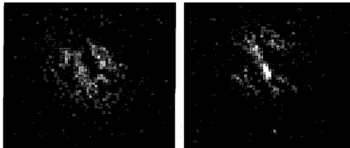
Figure (3.42): Contraste magnétique en fonction de l'angle de l'analyseur et images complémentaires obtenues en champ nul après application d'un champ de 20 Oe, pour des angles de l'analyseur valant respectivement 60^\circ (à gauche) et 120^\circ (à droite).
