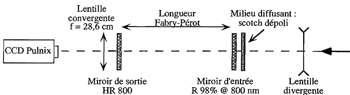
Figure III-(77) : Cavité Fabry-Pérot d'analyse du signal.
