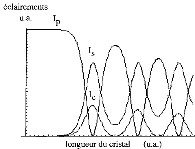
Figure I-(18) : Représentation de l'évolution des éclairements signal, complémentaire et pompe au cours de la propagation dans le cristal. Seule l'onde complémentaire présente de l'absorption. On voit que l'influence de l'absorption se fait sentir sur les deux autres ondes qui voient leur éclairement maximal diminuer au cours de la propagation.
