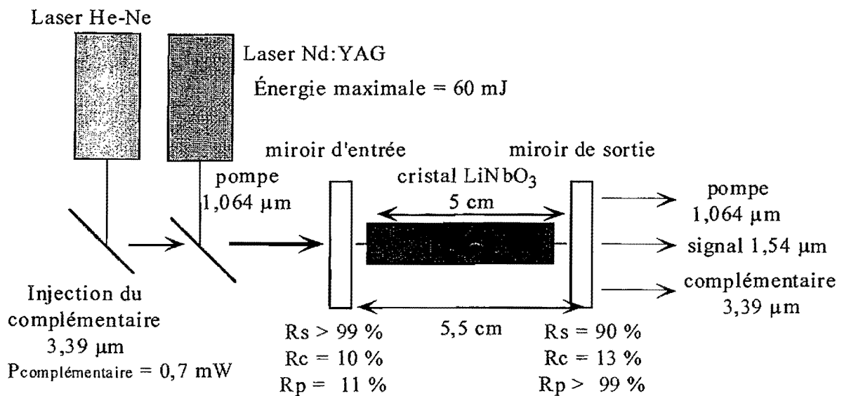
Figure III-(14) : Schéma général de l'OPO injecté. Le laser de pompe est un Nd:YAG à 1064 nm. Le laser d'injection est un He-Ne continu de puissance 0,7 mW émettant à 3,39 µm.
