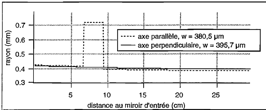
Figure III-(56) : Représentation de l'évolution des rayons du faisceau dans la cavité. Le saut de la valeur du rayon dans le miroir perpendiculaire est dû à l'angle de Brewster et à la coupe du cristal. Les rayons de cols, situés sur le miroir de sortie, sont respectivement égaux à w_{\text{parallèle}} = 380,5 \mu\text{m} et w_{\text{perpendiculaire}} = 395,7 \mu\text{m} .
