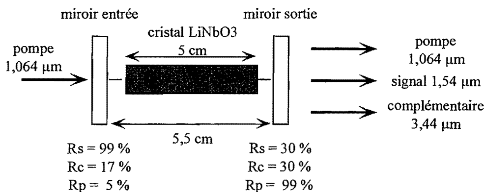
Figure III-(7) : Représentation de l'OPO non-injecté réalisé par Thomson. Le laser de pompe est un laser Nd:YAG nanoseconde émettant à 1064 \text{ nm} des impulsions de 20 \text{ ns} à mi-hauteur et de rayons de col 1,6 \text{ mm} . L'OPO est composé d'un cristal de \text{LiNbO}_3 taillé à l'accord de phase de type I permettant d'émettre à 1,54 \mu\text{m} et 3,44 \mu\text{m} , placé entre deux miroirs plans. Les coefficients de réflexion sont choisis afin de réaliser un OPO simplement résonant sur le signal.
