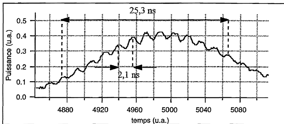
Figure III-(63) : Profil de l'impulsion lorsque le fonctionnement du laser est bimode. La période de battement est de T = 2,1 ns ( 12 T = 25,3 ns). Le chemin optique de la cavité est L_{Laser-opt} = c T/2 = 31,6 cm. Cela correspond, si l'on tient compte des indices des cristaux de saphir dopé au titane (1,76) et de titanate de baryum (2,1) et du prisme SF10 (1,71), à une longueur géométrique de L_{Laser} = 29,5 cm. On retrouve la valeur expérimentale mesurée précédemment.
