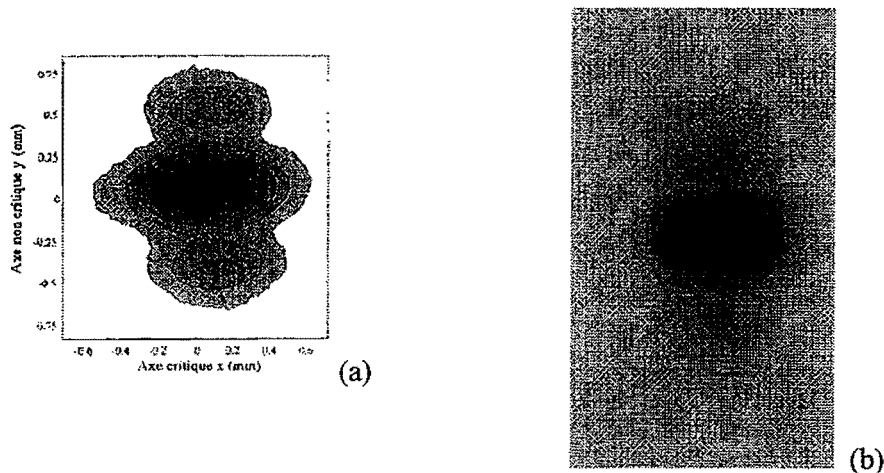
Figure III-6) : Répartition transverse de fluence du faisceau signal, 30 cm derrière le miroir de sortie de l'OPO pompé avec une énergie de 11,6 mJ par impulsion, soit 3,5 fois au-dessus de son seuil d'oscillation. (a) coupe transverse expérimentale, (b) coupe transverse théorique.
