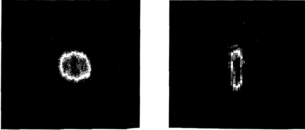
Figure IV.18: Image en absorption d'un piège de Ioffe-Pritchard : (a) adaptation pour le transfert du PMO vers le piège magnétique avec B'' = 150 Gauss/cm 2 , B_0 = 150 Gauss et B' = 260 Gauss/cm. (b) La compression adiabatique est effectuée en augmentant le gradient du quadrupôle à B' = 900 Gauss/cm et en gardant un champ dipolaire constant. Au cours de cette opération, la température augmente ce qui provoque un étalement du nuage dans la direction du dipôle.
