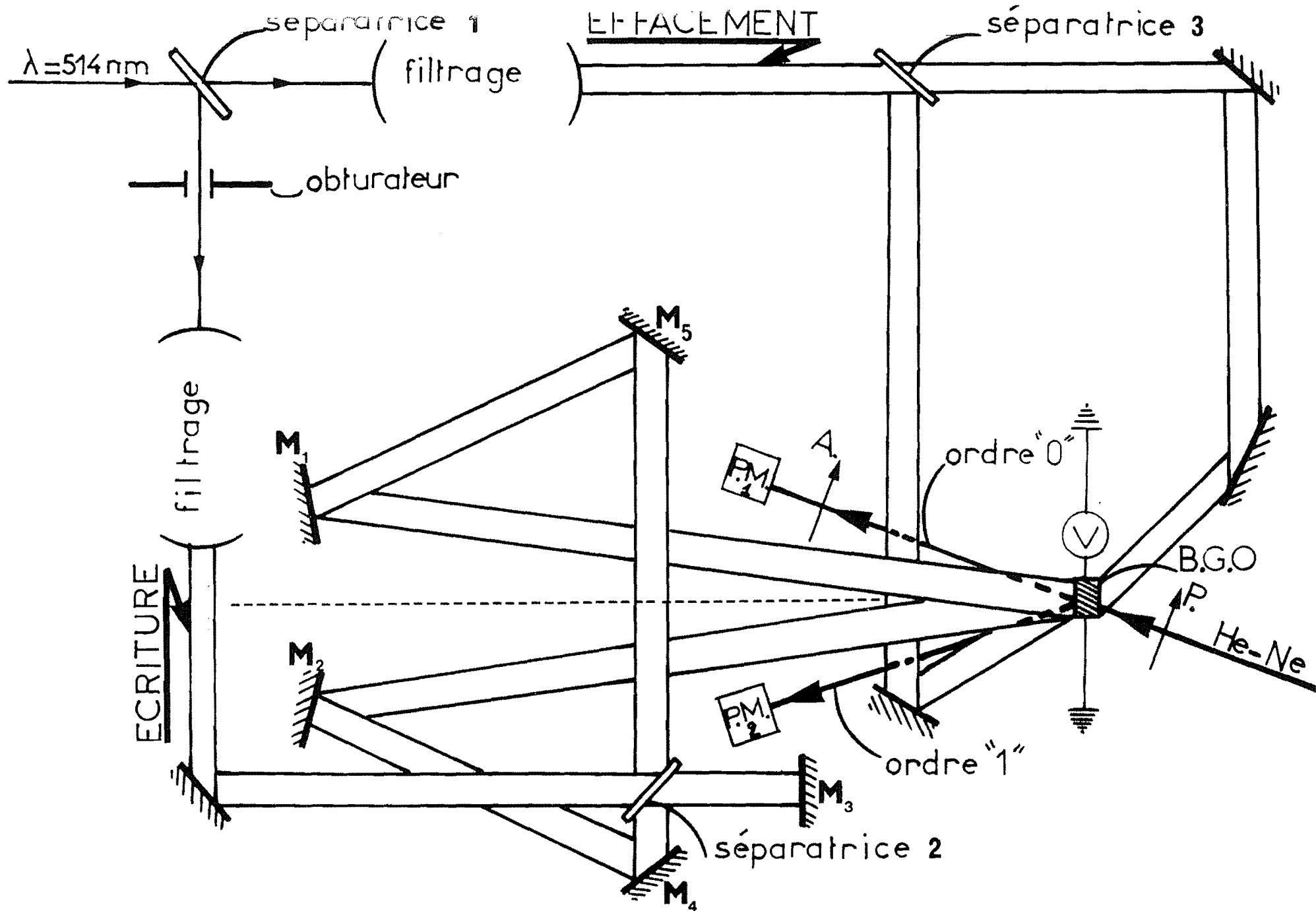
Figure III-14 : Montage expérimental de caractérisation des paramètres photoréfractifs. PM1 et PM2 sont deux photomultiplicateurs P et A sont respectivement un polariseur et un analyseur.
