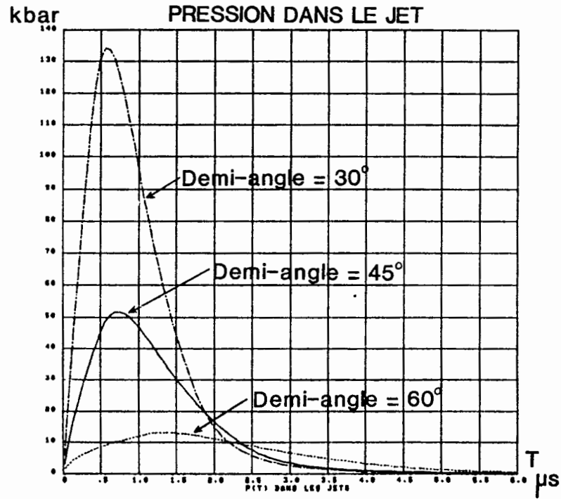
Figure 84 : Evolution de la pression dans les 3 jets au cours du temps.
