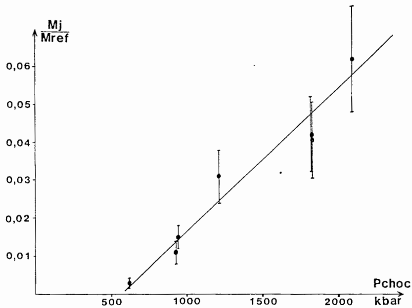
Figure 61 : Résultats obtenus sur tantale concernant l'influence de la pression de choc.
