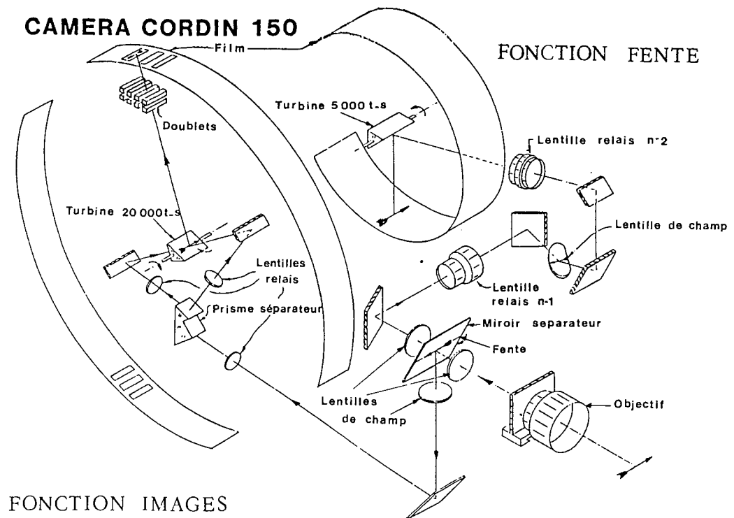
Figure 49 : Principe de fonctionnement des deux voies optiques d'une caméra ultra-rapide à activité totale.
