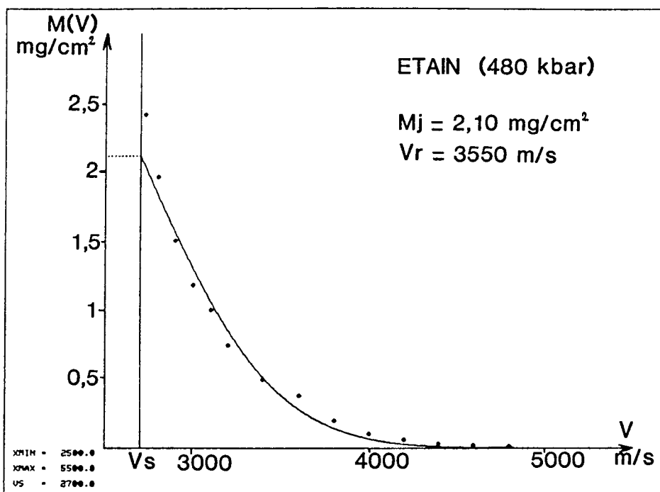
Figure 55 : Courbes M (V) expérimentale et extrapolée obtenues pour l'étain.
