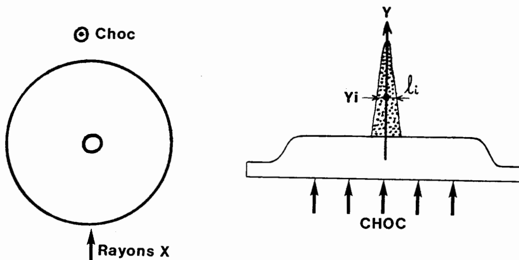
Figure 44 : Echantillon utilisé et résultat obtenu pour l'étude des trous coniques.
