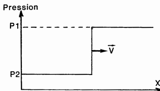
Figure 2 : Propagation d'une onde de détente.
