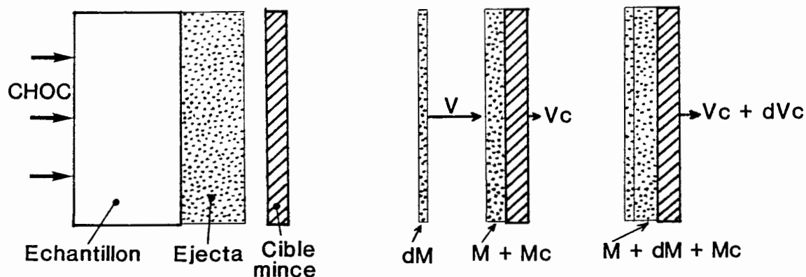
Figure 21 : Principe de la mesure de masse éjectée par I.D.L. cible mince.
