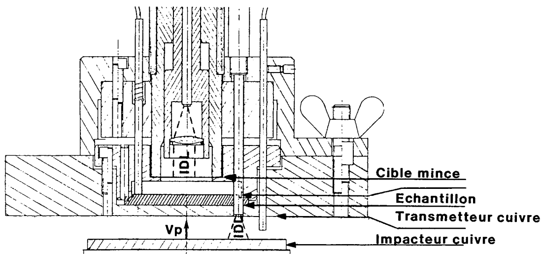
Figure 22 : Dispositif expérimental adapté aux lanceurs.
