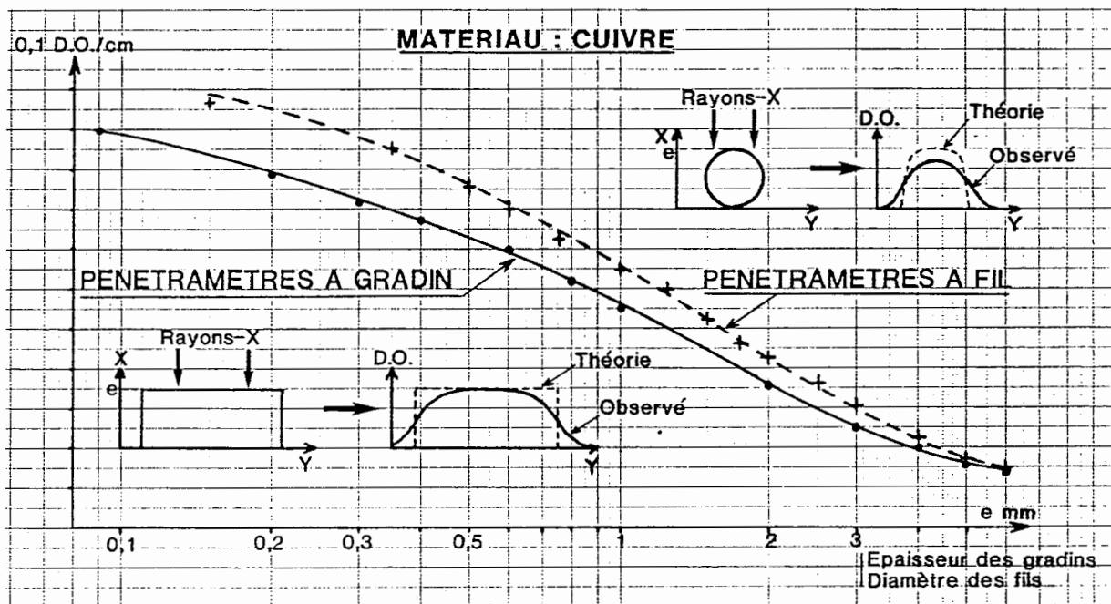
Figure 43 : Comparaison entre deux étalonnages du film obtenus avec des pénétramètres à fil et à gradin.
