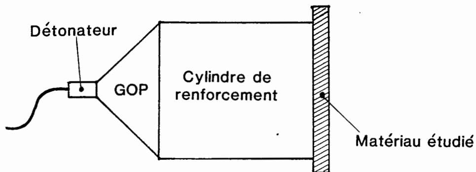
Figure 15 : Edifice expérimental avec un générateur de choc explosif.
