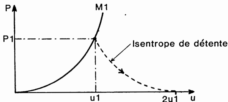
Figure 6 : Cas d'une onde de choc débouchant dans le vide.
