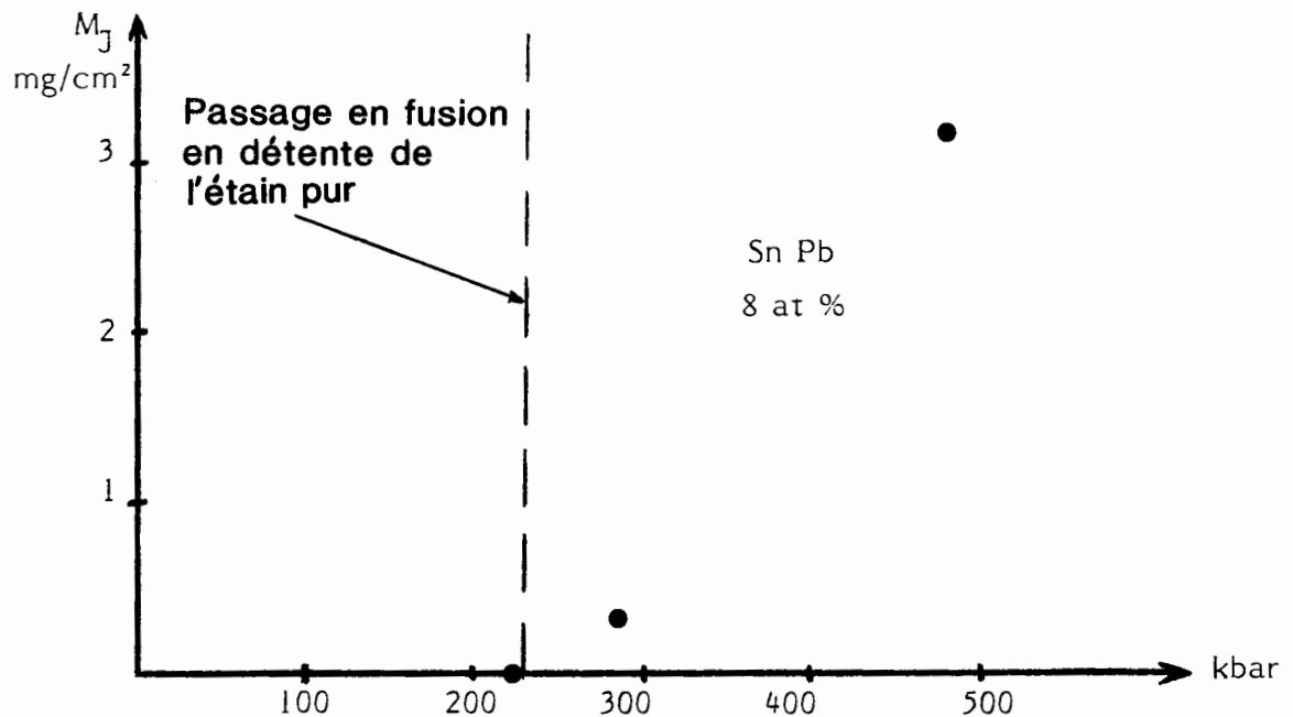
Figure 70 : Influence de la pression de choc sur la masse totale éjectée pour des alliages SnPb à 8 at % de Pb.
