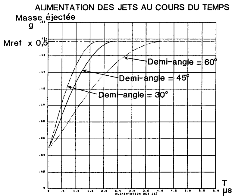
Figure 83 : Loi d'alimentation des jets en fonction du temps.
