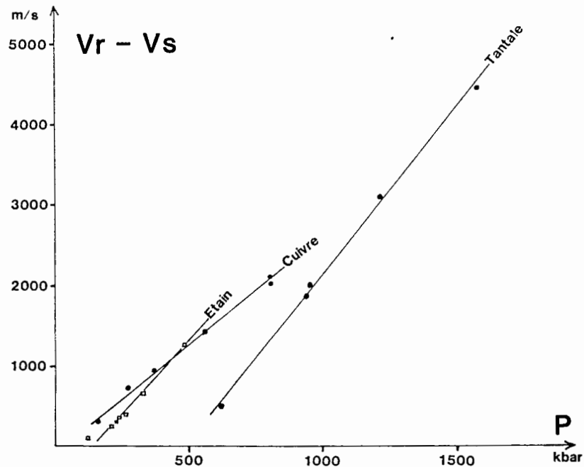
Figure 64 : Influence de la pression de choc sur la vitesse des particules éjectées.
