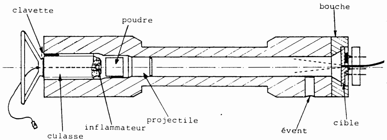
Figure 9 : Le lanceur à poudre de calibre 60mm.
