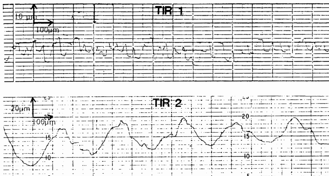
Figure 65 : Relevés de rugosité des deux échantillons de tantale.
