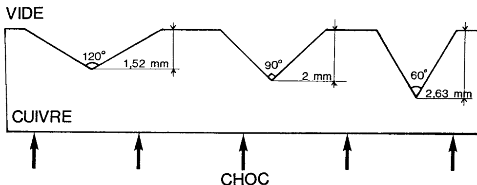
Figure 82 : Etude de trois jets localisés issus de rainures diédriques d'angle différent mais de volume constant.
