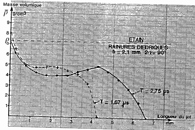
Figure 42 : Répartition de la masse volumique à deux instants différents.
