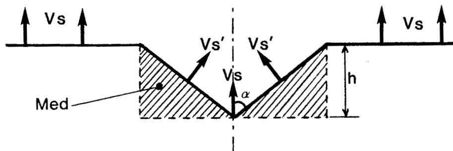
Figure 78 : Délimitation de la masse éjectée disponible.
