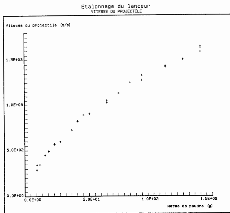
Figure 10 : Courbe d'étalonnage en vitesse du lanceur à poudre de calibre 60mm.
