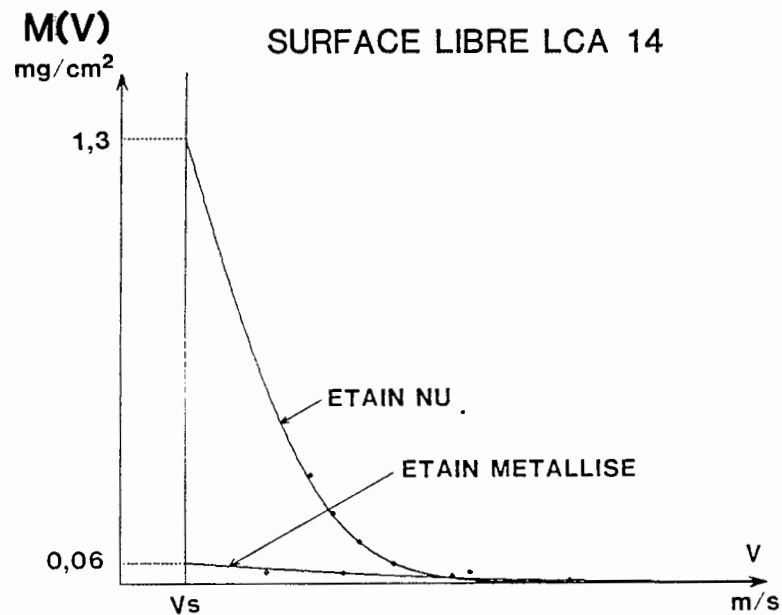
Figure 93 : Influence d'une métallisation de cuivre de 5 \mu\text{m} déposée sur la surface libre usinée LCA14 d'un échantillon d'étain.
