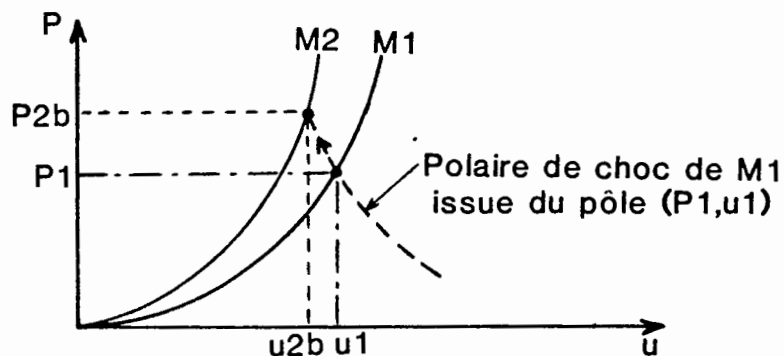
Figure 5 : Calcul de l'état de choc du matériau M_2 dont la polaire est située au-dessus de celle de M_1 .
