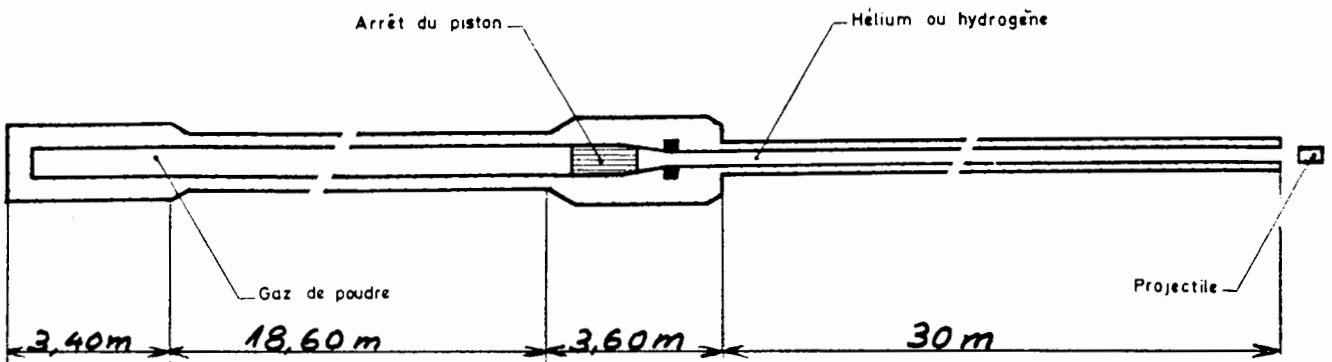
Figure 14 : Fonctionnement du C.A.G.L. : lancement du projectile.
