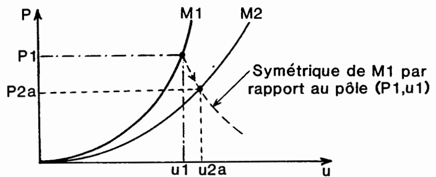
Figure 4 : Calcul de l'état de choc du matériau M_2 dont la polaire est située en-dessous de celle de M_1 .
