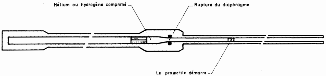
Figure 13 : Fonctionnement du C.A.G.L. : mise en vitesse du projectile.
