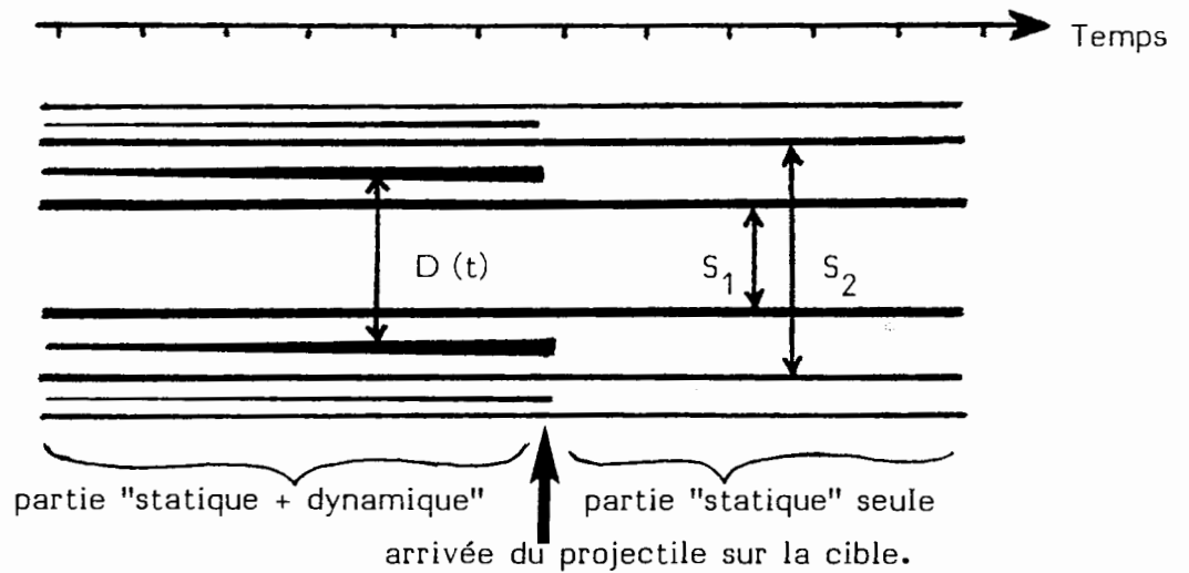
Figure 28 : Interférogramme obtenu lors d'une mesure de vitesse de projectile par I.D.L. monofibre.
