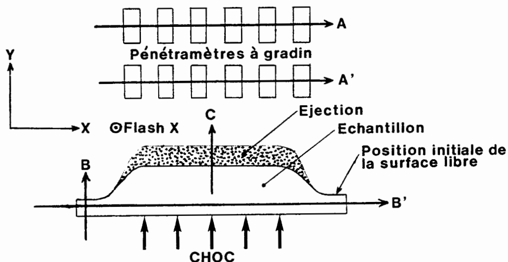
Figure 35 : Principe de dépouillement des images radiographiques d'éjection répartie au moyen du microdensitomètre Joyce & LoebI
