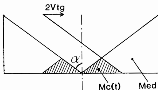
Figure 80 : Calcul de l'alimentation du jet dans le cas du trou conique.
