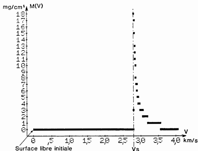
Figure 40 : Courbe M (V) de masse cumulée de matière éjectée en fonction de la vitesse des particules.
