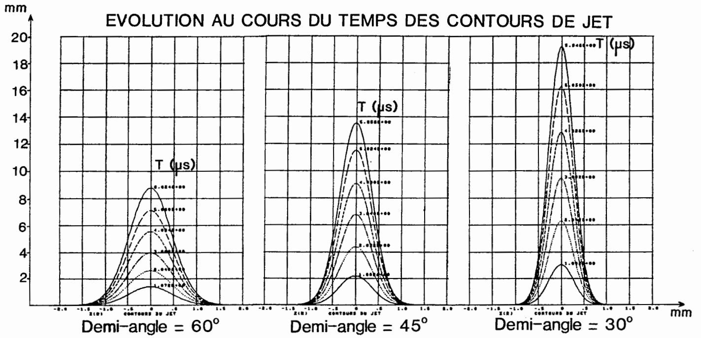
Figure 86 : Contours extérieurs des jets à différents instants.
