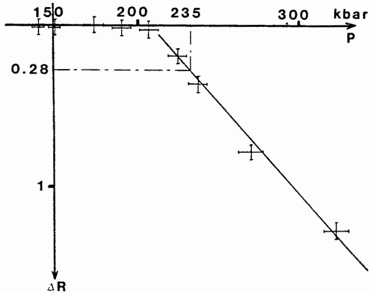
Figure 32 : Variation de la réflectivité de l'étain en fonction de la pression du choc incident.
