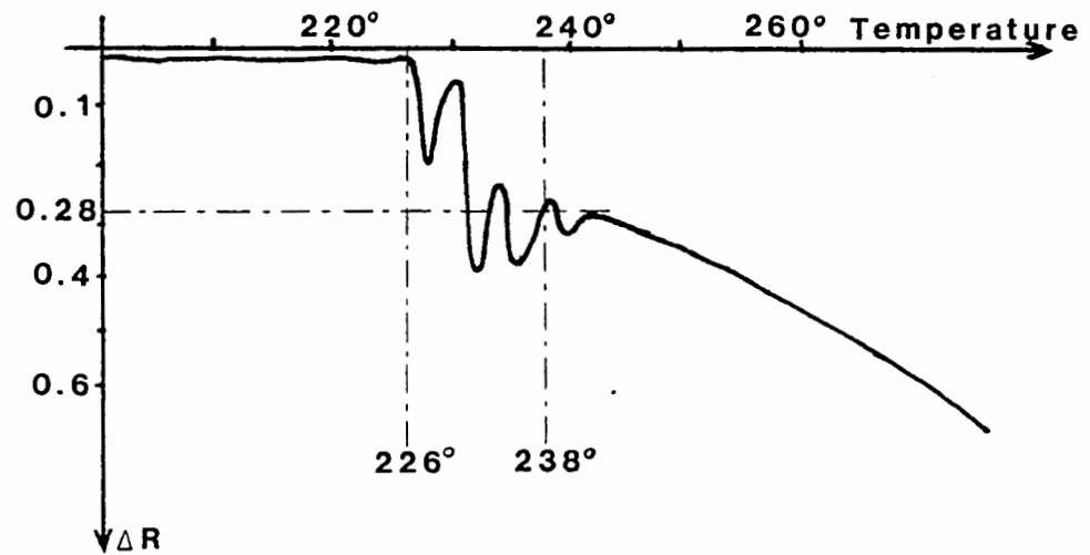
Figure 30 : Variation de réflectivité de l'étain en fonction de sa température.
