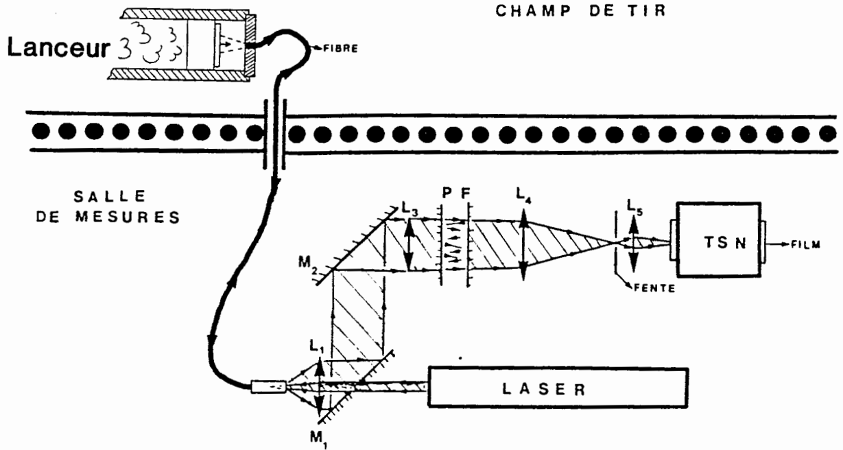
Figure 27 : Dispositif expérimental I.D.L. monofibre pour mesurer la vitesse d'impact du projectile.
