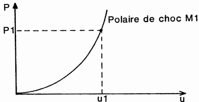
Figure 3 : Etat de choc du matériau M_1 .
