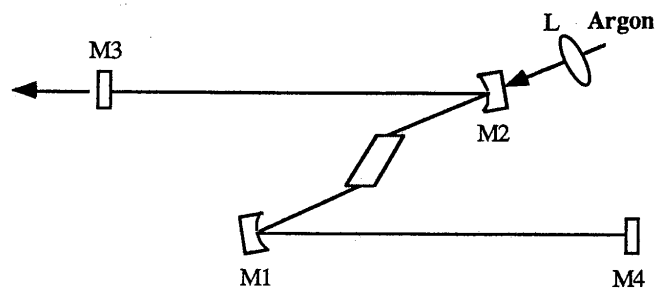
Figure 63 : Cavité à quatre miroirs, dite cavité en Z.
