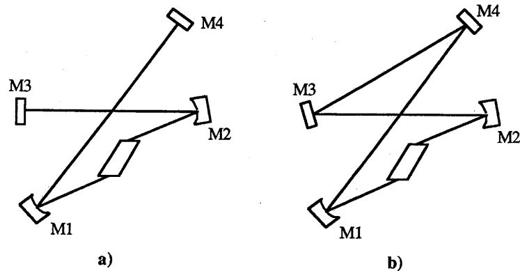
Figure 64: Cavit      quatre miroirs, dite cavit   en \gamma , en configuration lin  aire (a) ou en anneau (b).
