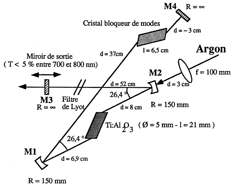
Figure 68 : Laser à saphir dopé au titane, à modes couplés par un acousto-optique (Le dessin n'est pas à l'échelle).
