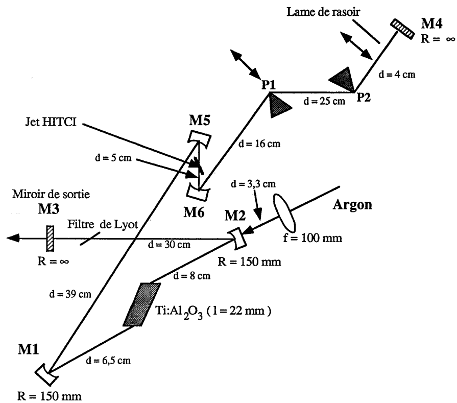
Figure 76 : Laser à saphir dopé au titane, à modes couplés passivement, avec contrôle de la dispersion intracavité (Le dessin n'est pas à l'échelle).
