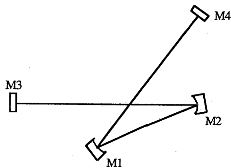
Figure 65 : Cavit      quatre miroirs, en \gamma vide.
