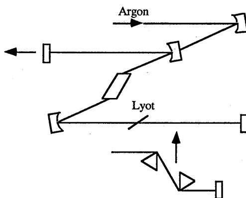
Figure 58 : Le couplage de modes magique.
