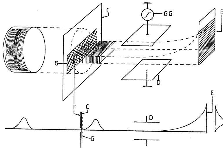
Figure 23 : Schéma de principe d'une caméra à balayage de fente : F = fente, C = photocathode, G = grille, D = plaques de déflection, GG = générateur de balayage, E = écran.
