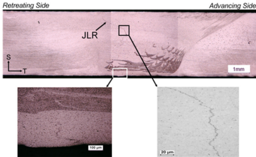
Figure 3.7 – Observations par microscopie optique d'une coupe transversale d'une soudure contenant un JLR (les traces noires sont des artefacts d'attaque systématique et n'ont aucun rôle mécanique)
