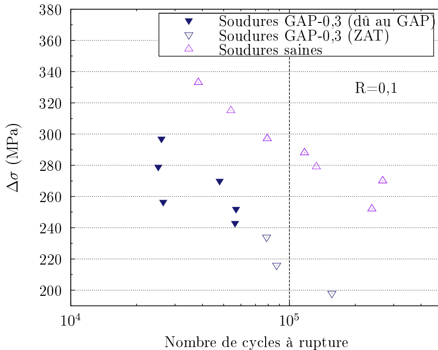
Figure 5.22 – Courbe de Wöhler des soudures GAP-0,3 donnant la localisation de l'amorçage, comparée à celle des soudures saines
