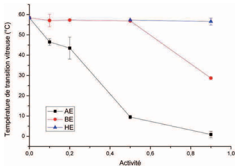
Figure 4.4. Température de transition vitreuse du P(D,L)LA Biomer L9000, mesurée par DSC, avant et après contact vapeur pendant 15 jours avec les trois esters éthyliques (AE,BE,HE) à différentes activités.
