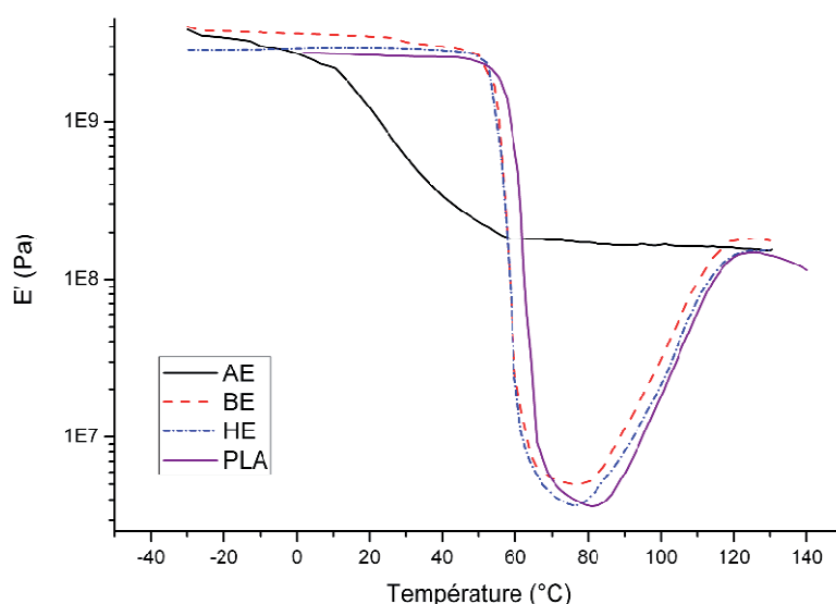
Figure 4.6. Evolution du module de conservation ( E' ), mesuré par DMA, avec la température, du P(D,L)LA Biomer L9000, avant contact (PLA) et après contact avec l'acétate d'éthyle (AE), le butyrate d'éthyle (BE) et l'hexanoate d'éthyle (HE) à une activité de 0,5 pendant 15 jours.
