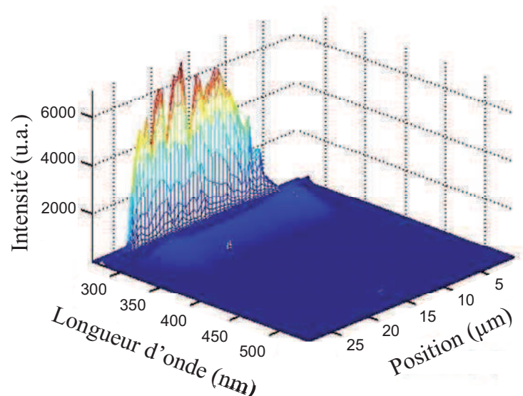
Figure 5.8. Profils spectraux de fluorescence du biphenyl en 2D sur les coupes transversales de PP (longueur d'onde \times position).
