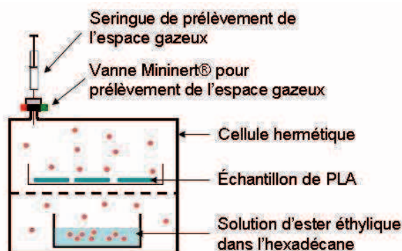
Figure 2.11. Schéma de la cellule de conditionnement des échantillons de polymère contenant une solution d'ester éthylique.
