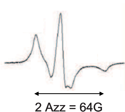
Figure 2.12. Spectre d'une sonde immobile.
