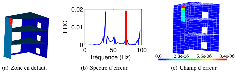
Figure E.12: Localisation d'un défaut de 20% de module d'Young sur 5 éléments du voile. La fréquence de localisation est mise en évidence en rouge.
