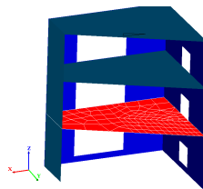
Figure E.2: Défaut étudié. La sollicitation sismique s'exerce dans les direction X et Y.
