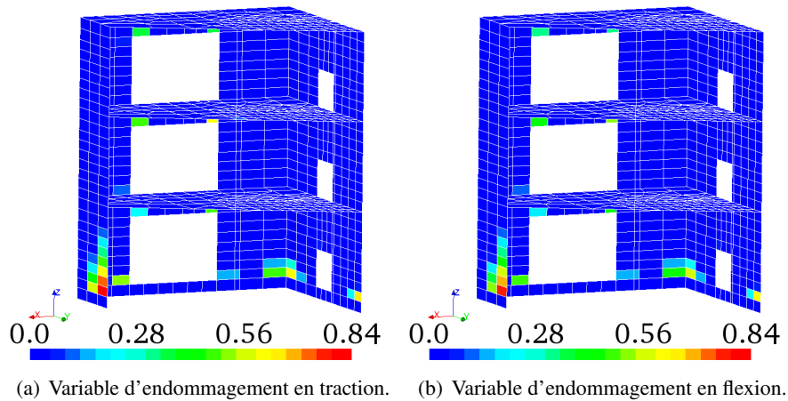
Figure E.33: Champs d'endommagement à la fin du calcul.
