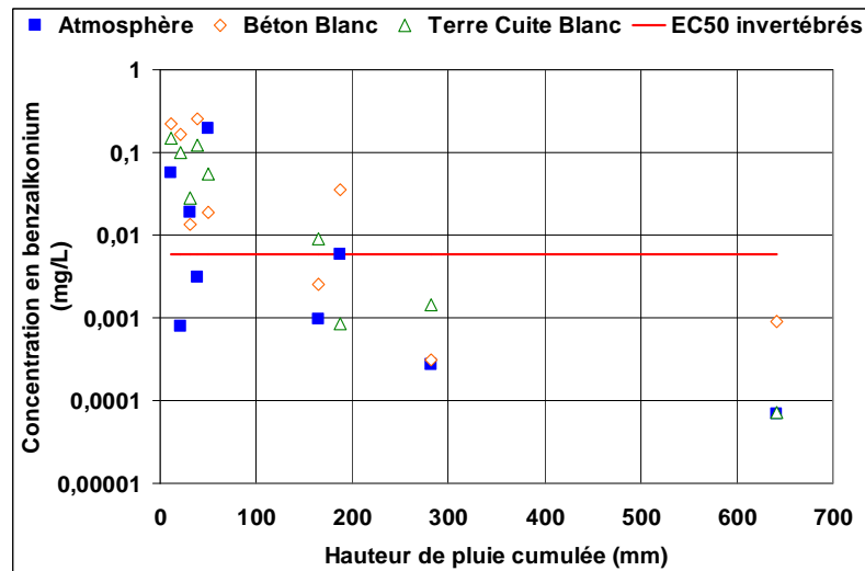
Figure 51 : Evolution de la concentration en benzalkonium dans les retombées atmosphériques et les bancs d'essais blancs
