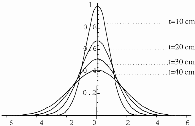
Figure IV-26: Réponses normalisées du système de détection caractérisé par les équations (18) en fonction de l'éloignement t .
