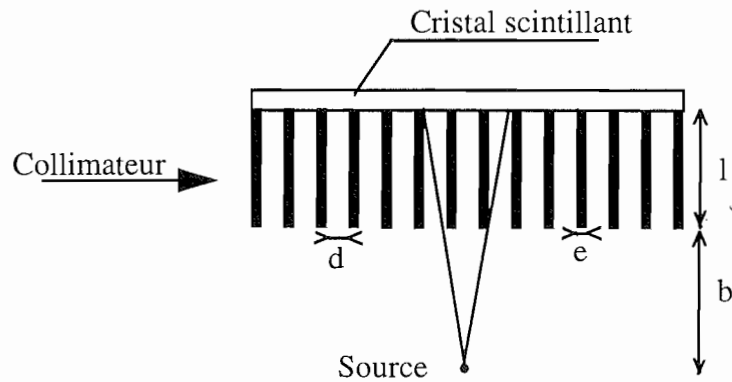
Figure II-8: Description des différents paramètres d'un collimateur.
