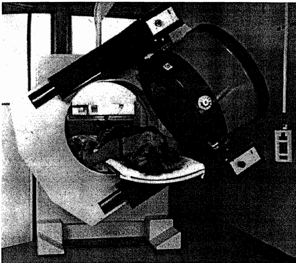
Figure I-10: Exemple de gamma-caméra, (dessus) la Gammatome et (dessous) la 3 têtes Picker.
