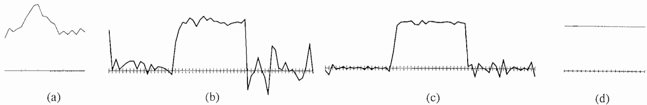
Figure V-10: Profils des activités de la figure V-9. (a) Reconstruction par rétroprojection filtrée, (b) Reconstruction avec le modèle initial du VG, (c) Reconstruction après convergence du processus., (d) Distribution simulée.
