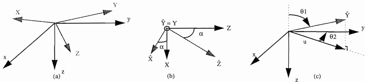
Figure IV-10: Définition des différents angles de rotation définissant le modèle d'objet global. (a) superposition du repère des ellipsoïdes (XYZ) avec le repère des images (xyz) , les figures (b) et (c) définissent les angles permettant le passage du repère (XYZ) au repère (xyz) .
