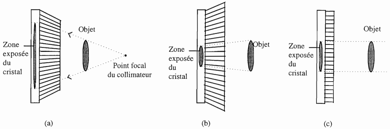
Figure II-7: Description des différents types de collimateurs: (a) collimateur convergent, (b) collimateur divergent et (c) collimateur parallèle.
