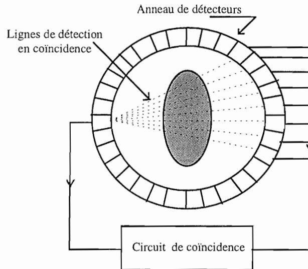
Figure I-7: Configuration de détection en Tomographie d'émission de positons.
