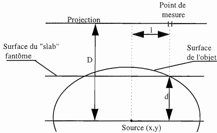
Figure II-17: Définition des variables de la fonction caractéristique du "slab" fantôme.
