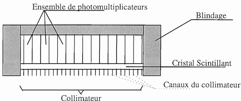
Figure I-11: Description des différents éléments d'une gamma-caméra.
