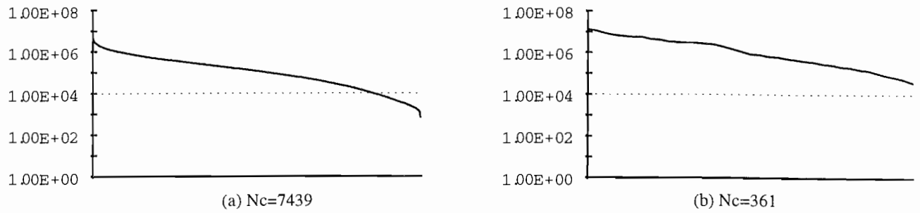
Figure V-2: Spectre des valeurs singulières en fonction du champ de la reconstruction (l'axe des y est représentée en échelle log). (a) Les pixels de reconstruction sont carrés et régulièrement répartis sur une grille 32 \times 32 , (b) les pixels de reconstruction sont adaptés aux formes des organes et localisés uniquement sur les régions émettrices.
