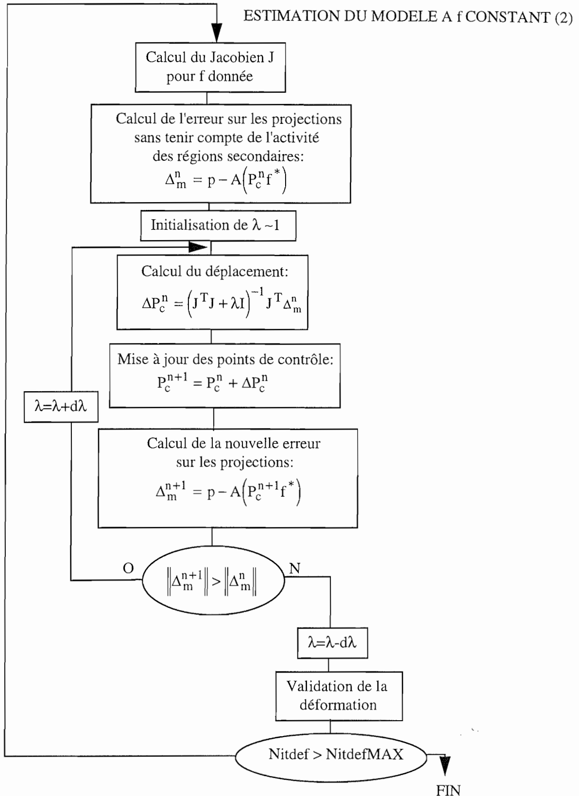
Figure IV-34: Détails de l'étape (2) de la reconstruction.
