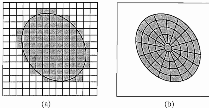
Figure III-1: Apport d'un modèle d'organe réaliste: (a) discrétisation rectangulaire (b) discrétisation s'appuyant sur la forme des organes.
