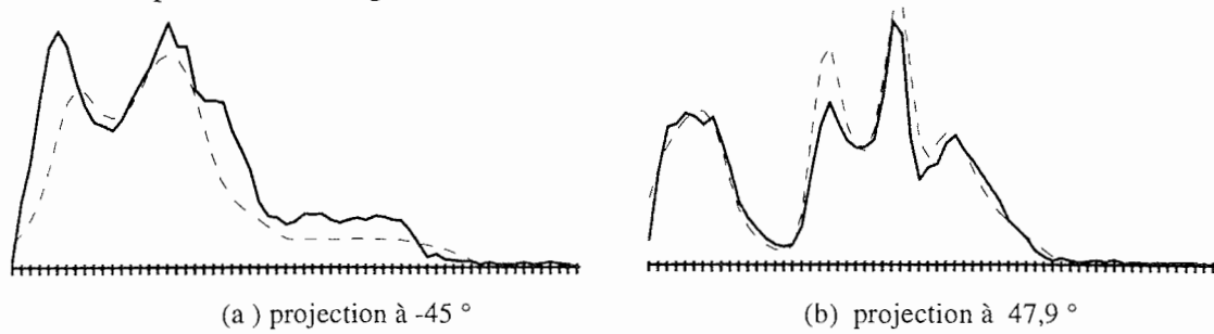
Figure V-18: Projections simulées (en pointillés) et mesurées (en trait plein).
