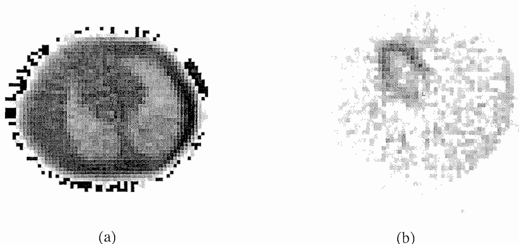
Figure V-24: Coupe en transmission corrigée en troncature (a) et coupe en émission (b).
