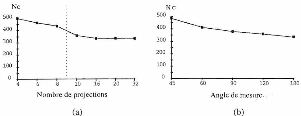
Figure V-3: Evolution du nombre de conditionnement en fonction du nombre de projections utilisé dans la reconstruction.
