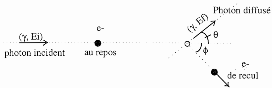
Figure II-3: Principe de l'interaction Compton.
