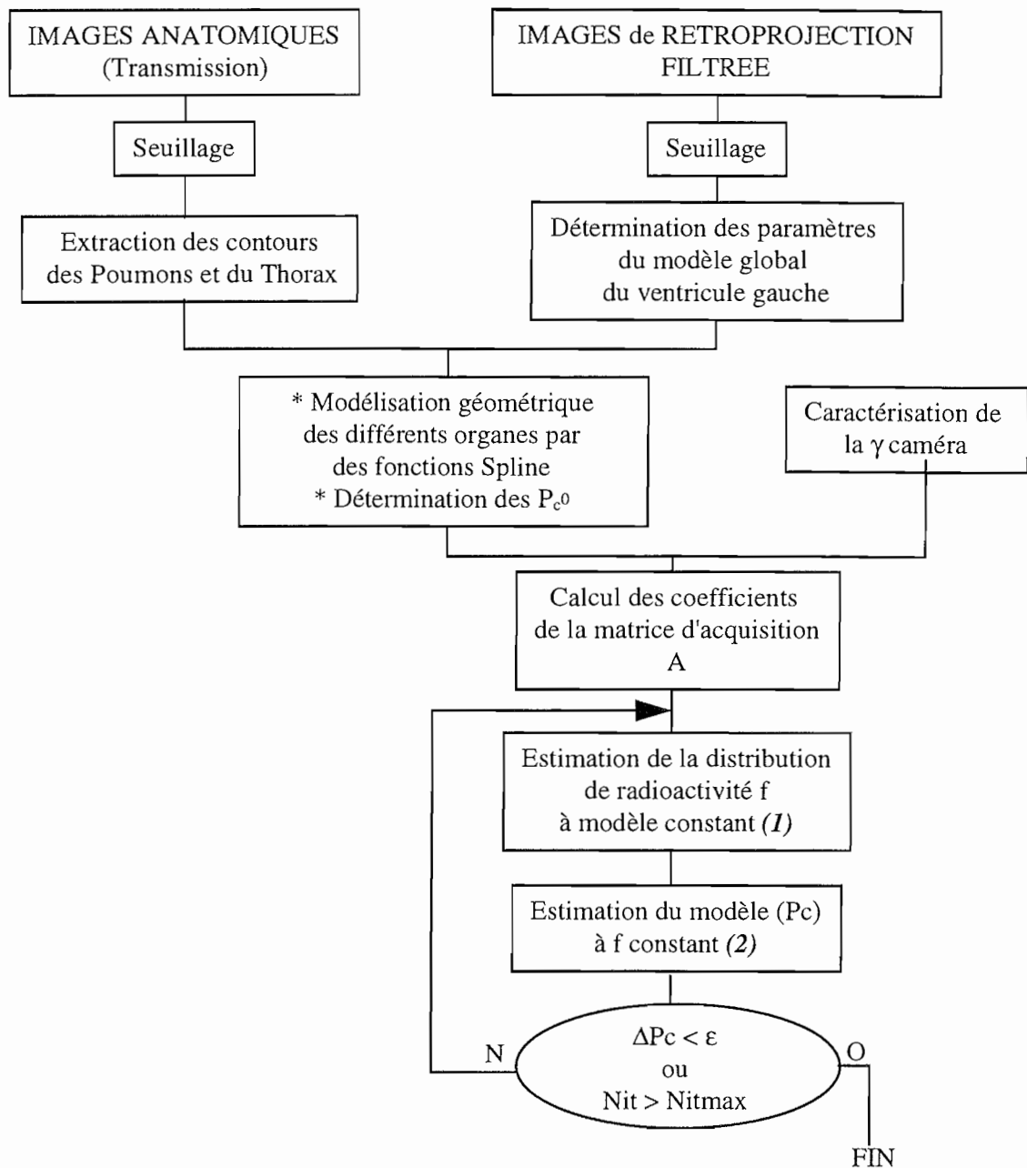
Figure IV-32: Organigramme de la méthode proposée.
