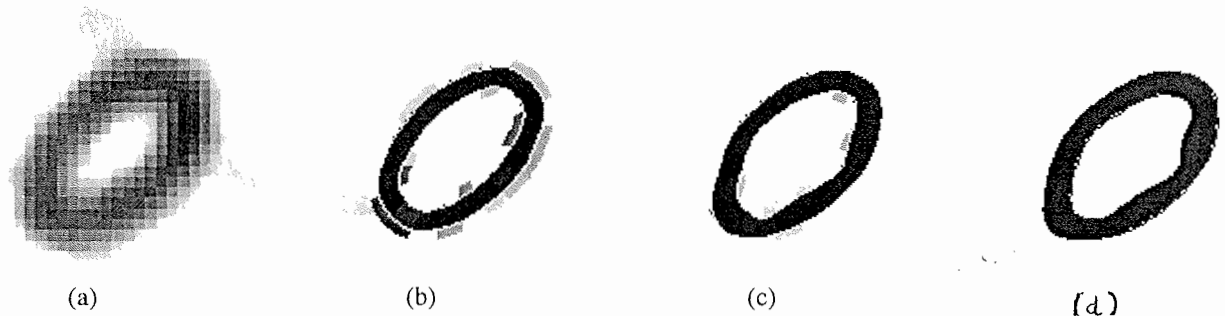
Figure V-9: Exemple de reconstruction par double estimation. (a) Reconstruction par rétroprojection filtrée, (b) Reconstruction avec le modèle initial du VG, (c) Reconstruction après convergence du processus., (d) Distribution simulée.
