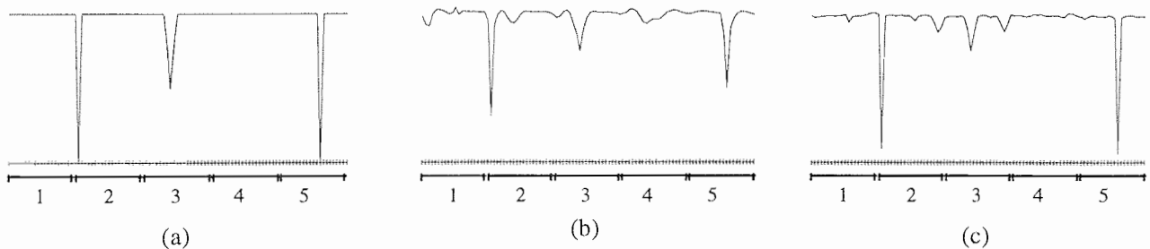
Figure VI-6: Visualisation des distributions de radioactivité dans chacun des cas de la figure VI-5. Les régions numérotées de 1 à 5 correspondent aux couronnes de la discrétisation du VG.
