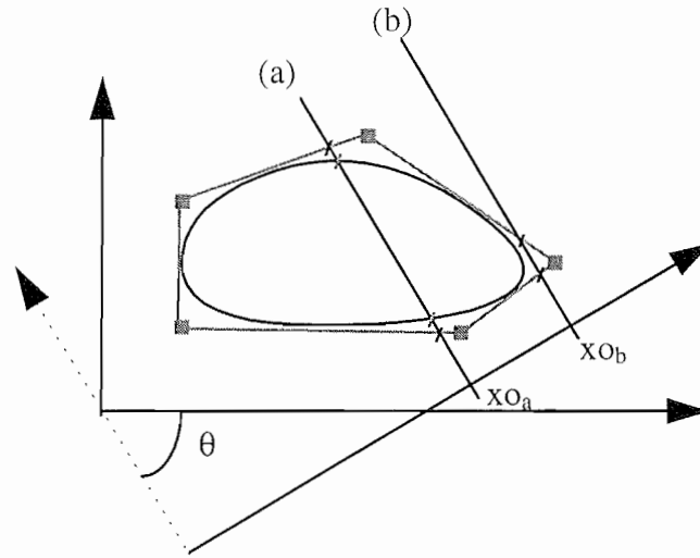
Figure AI-1: Intersection d'un rayon de projection avec une courbe Spline.
