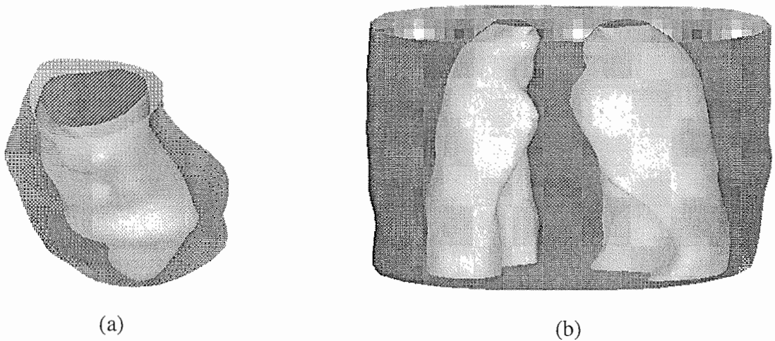
Figure VI-2: Représentation, (a) du modèle 3D du VG dans le repère des images IRM, (b) du modèle 3D des poumons/thorax dans le repère des poumons et du thorax.
