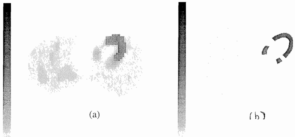
Figure V-6: Exemple de reconstruction avec une discrétisation classique (a) et une discrétisation adaptée à la forme des organes (b).
