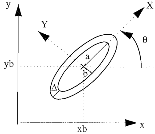
Figure IV-9: Définition du modèle global à deux dimensions.
