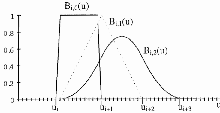
Figure IV-3: Exemple de fonction de base.
