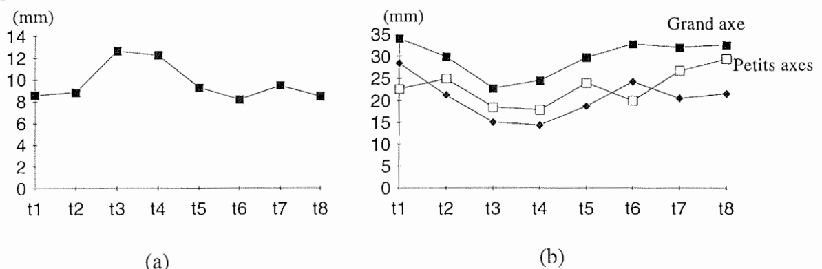
Figure VI-9: Evolution de l'épaisseur de la paroi ventriculaire (a) et des longueurs grand et petit axe (b) en fonction du cycle cardiaque.
