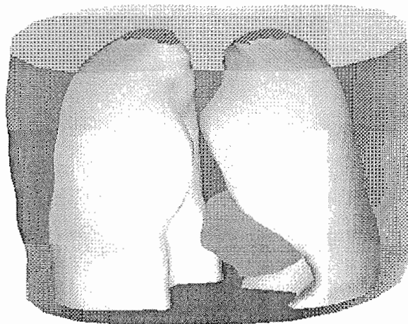
Figure VI-3: Représentation du modèle synthétique après recalage.
