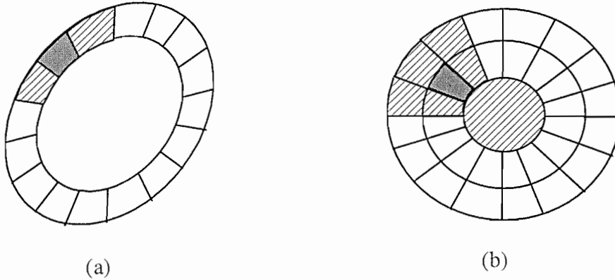
Figure IV-31: Description des différents voisinages utilisés pour le VG en 2D (a) et 3D (b). Les mailles hachurées correspondent aux mailles du voisinage de la maille grisée. En 3D on adopte une représentation en forme d'oeil de boeuf, la maille centrale correspondant à la maille située en pointe du ventricule gauche
