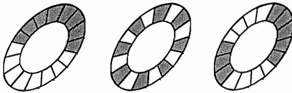
Figure IV-12: Représentation de différentes configurations correspondant à un même taux de remplissage (50%).
