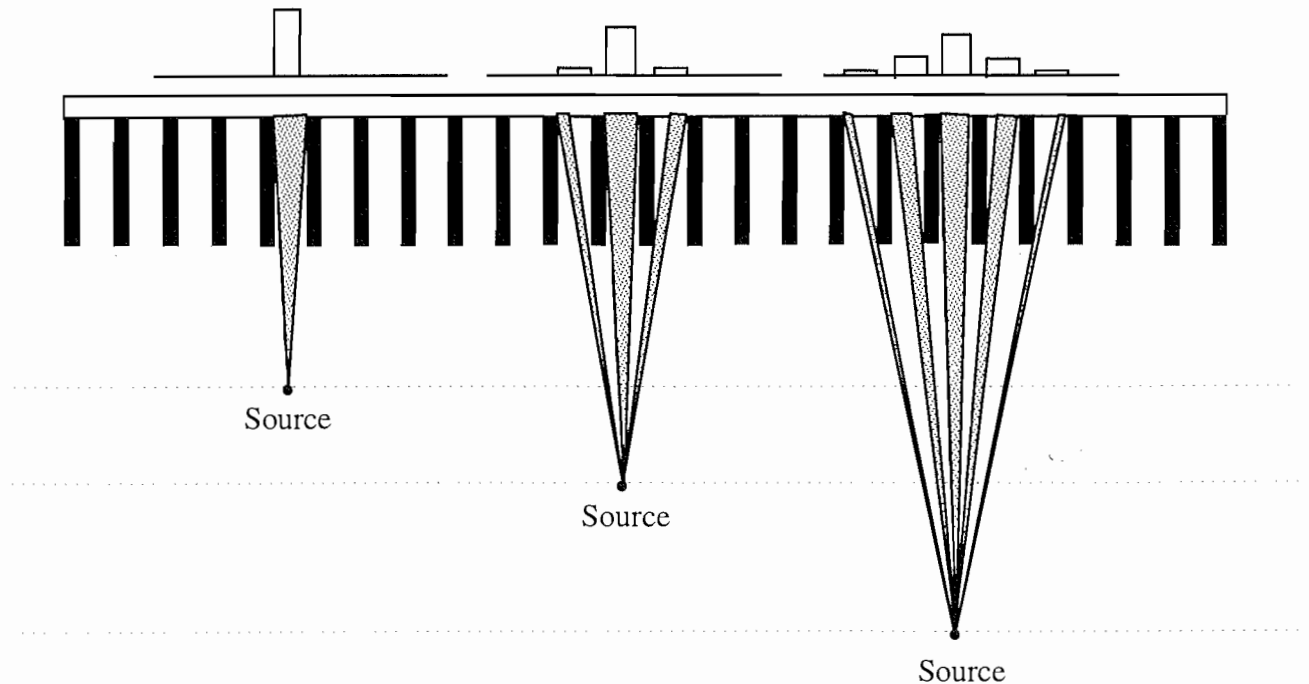
Figure II-9: Non invariance par translation de la détection.
