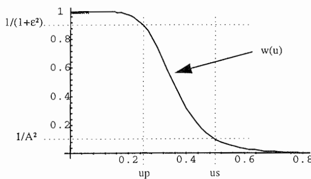
Figure II-13: Paramètres de la fonction filtre Butterworth.
