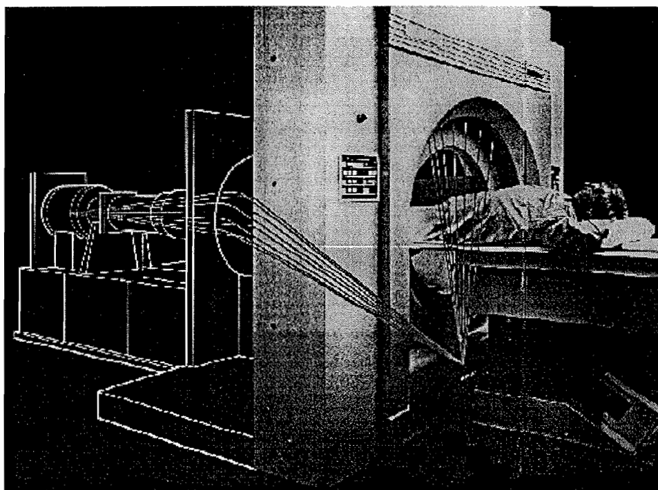
Figure I-2: Photographie de l'UFCT commercialisé par la société Imatron.
