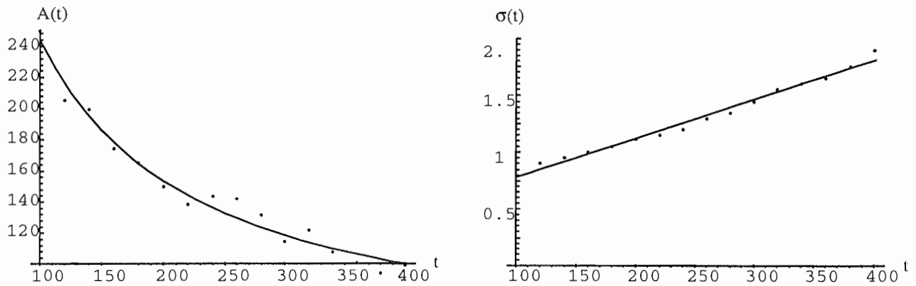
Figure IV-25: Evolution de l'amplitude et de la largeur à mi hauteur en fonction de l'éloignement.
