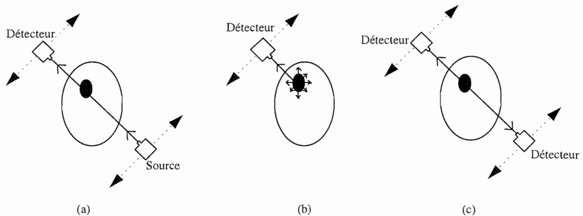
Figure I-5: (a) Principe de la tomographie par transmission, (b) Tomographie d'émission monophotonique, (c) Tomographie d'émission de positons.
