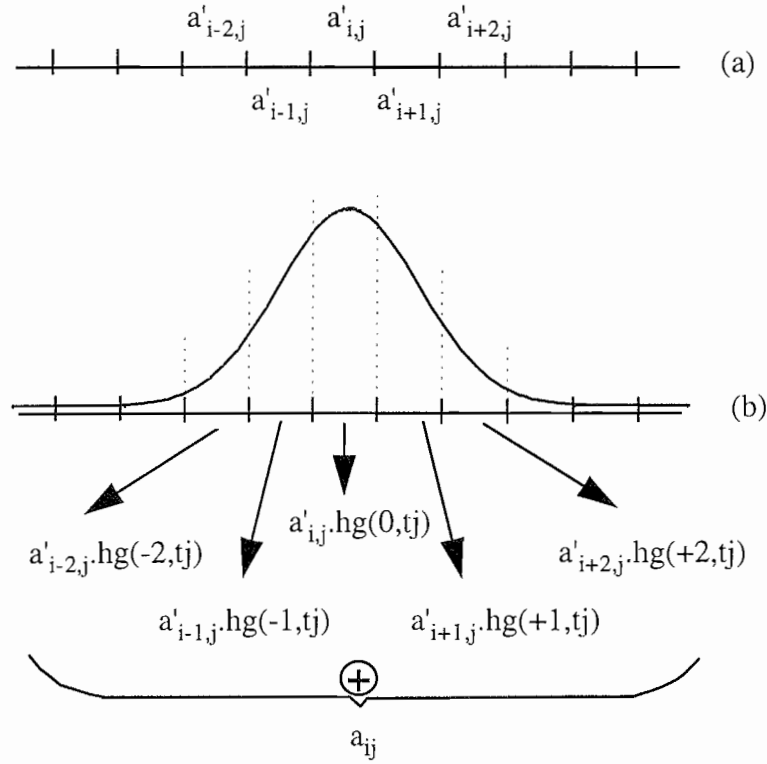
Figure IV-29: Prise en compte de la réponse du système de détection: (a) sans réponse des détecteurs, (b) avec réponse des détecteurs.
