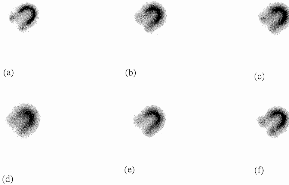
Figure II-14: Exemples de reconstruction avec ces différents types de filtres. Pour chacun des filtres (b) (c) et (d), la fréquence de coupure est fixée à 0.4 (fréquence réduite). (a) RAMP, (b) HAN, (c) HAM, (d) PARZN, (e) BUTER ( n=4 , uc=0.20 ) et (f) BUTER ( n=4 , uc=0.24 ).
