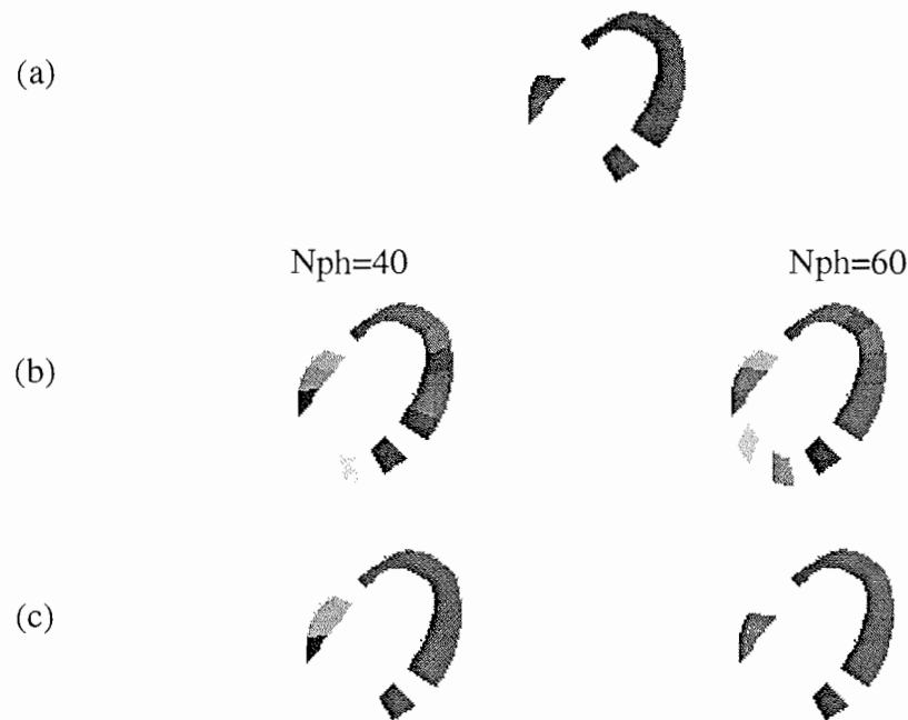
Figure V-5: Exemple de reconstruction obtenue pour différents niveaux de bruit avec 16 projections: (a) distribution simulée, (b) distribution reconstruite sans régularisation et (c) distribution reconstruite avec régularisation.
