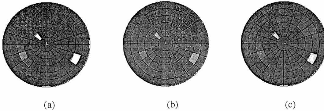
Figure VI-5: Exemples de reconstructions tridimensionnelles de la distribution simulée représentée en (a) avec 16 (b) et 32 (c) projections ( N_{ph}=60 ).
