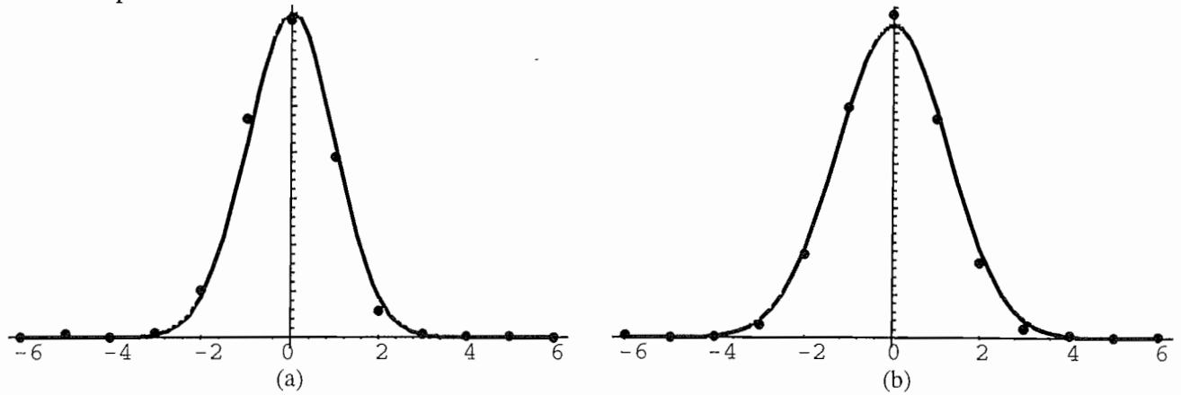
Figure IV-24: Exemple de modélisations pour des éloignements de 16 mm (a) et 24 mm (b). Le détecteur 0 correspond à la cellule située en face du tube. Les mesures sont représentées par les points et le modèle ajusté aux mesures en trait plein.
