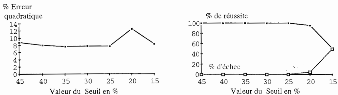
Figure IV-15: Evolution de l'erreur quadratique en fonction du seuillage sur la rétroprojection filtrée.
