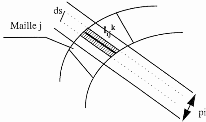
Figure IV-27: Calcul des aires d'intersection.
