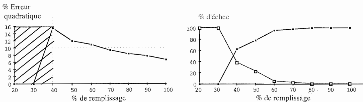
Figure IV-13: Evolution de l'estimation des paramètres en fonction du taux de remplissage. (a) Evolution de l'erreur quadratique (b) Evolution du % d'échec et du % de réussite.
