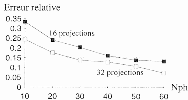
Figure V-4: Evolution de l'erreur relative en fonction du bruit contenu dans les projections.
