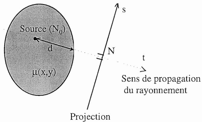
Figure II-5: Atténuation du rayonnement.
