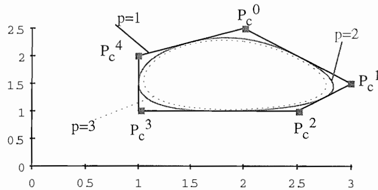
Figure IV-5: Evolution d'une courbe Spline cyclique en fonction de son ordre.
