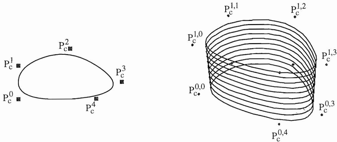
Figure IV-2: Exemple de courbe (gauche) et surface (droite) Splines. Les points de contrôles des fonctions Splines sont représentés par des points. Dans le cas d'une surface Spline (b), N=2 et M=5 .
