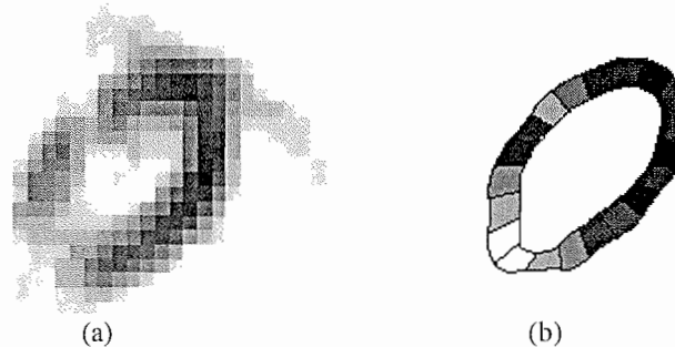
Figure V-19: Reconstructions obtenues à partir d'enregistrement sur fantôme: (a) Rétroprojection filtrée, (b) reconstruction par fusion de données.
