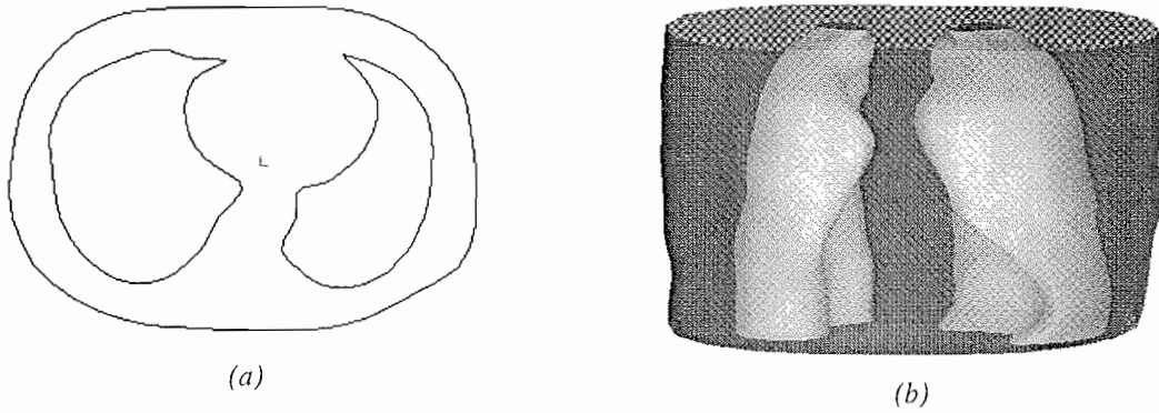
Figure IV-6: Représentation 2D (a) et 3D (b) du modèle géométrique du thorax et des poumons (obtenu à partir d'image scanner X).
