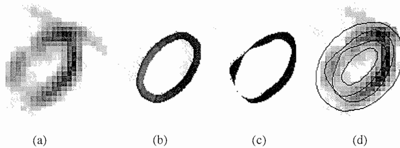
Figure V-23: Exemple de reconstruction par double estimation dans le cas de données réelles. (a) image de rétroprojection filtrée, (b) reconstruction avec le modèle initial du VG, (c) reconstruction après convergence du processus de déformation et (d) superposition du contour final avec l'image de rétroprojection filtrée.
