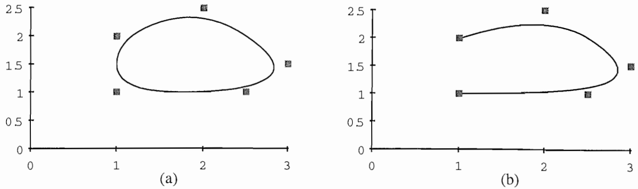
Figure IV-4: Exemple de courbe cyclique (a) et de courbe non cyclique (b).
