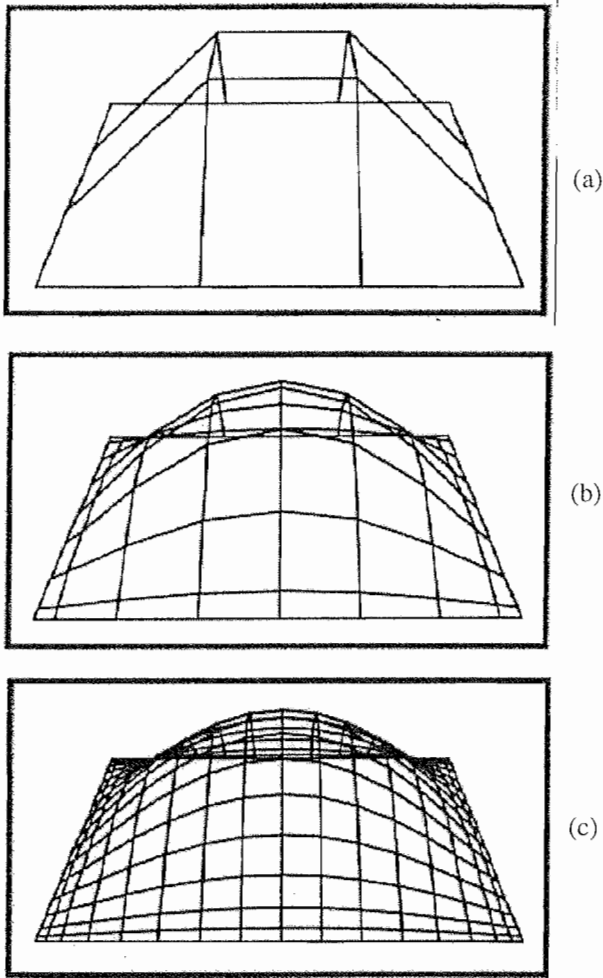
Figure AI-3: Exemple de raffinement d'une surface Spline. (a), points de contrôle initiaux, (b) points de contrôle avec un facteur de raffinement de 2, (c) points de contrôle avec un facteur de raffinement de 4.
