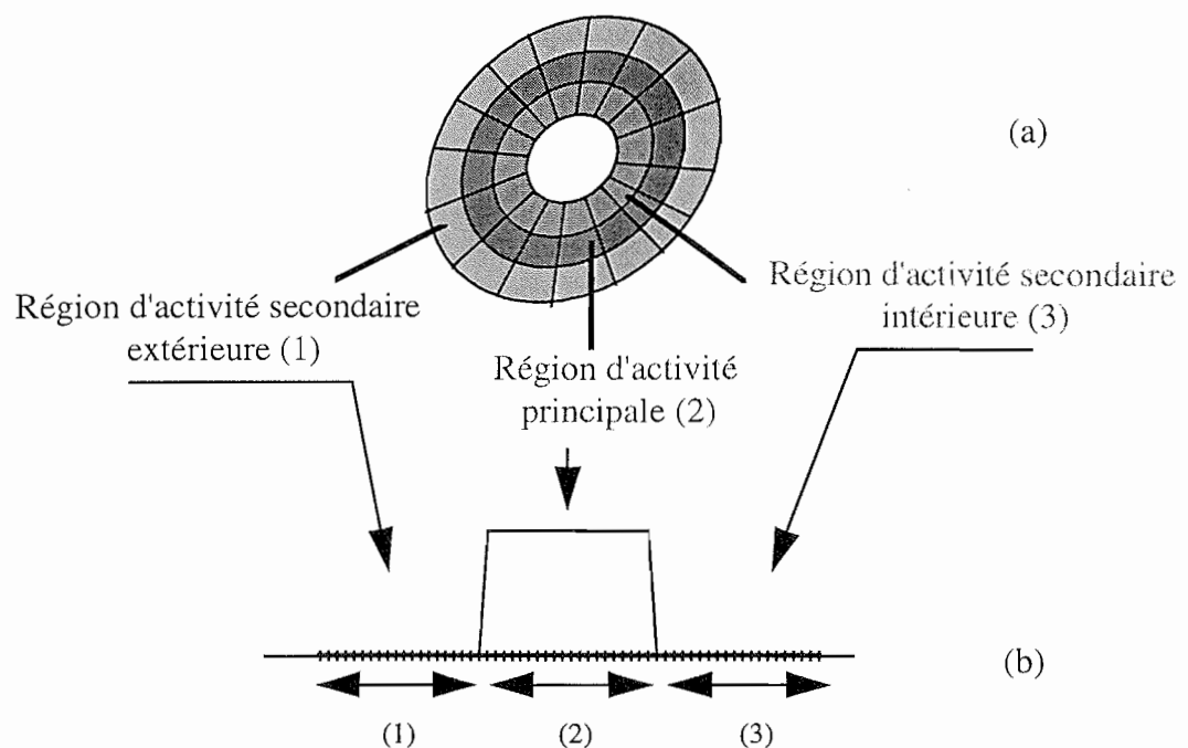
Figure V-12: Correspondance entre les profils des activités et la distribution reconstruite.
