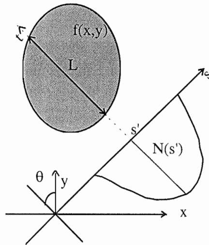
Figure II-2: Définition des différents systèmes d'axe.
