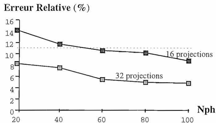
Figure VI-4: Evolution de l'erreur relative commise en fonction du bruit.
