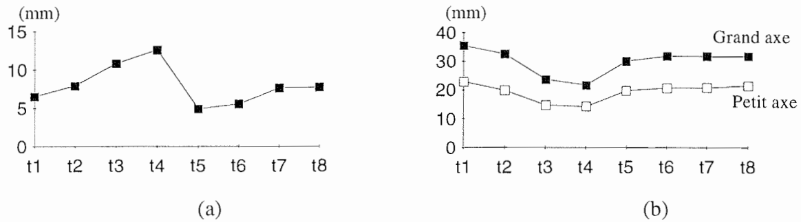
Figure V-26: Evolution de l'épaisseur de la paroi ventriculaire (a) et des longueurs grand et petit axe (b) en fonction de l'instant du cycle cardiaque.
