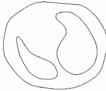
Figure V-28: Modélisation des poumons et du thorax.
