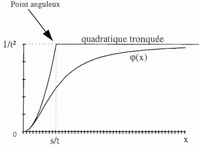
Figure IV-30: Représentation de la fonction de régularisation \varphi .
