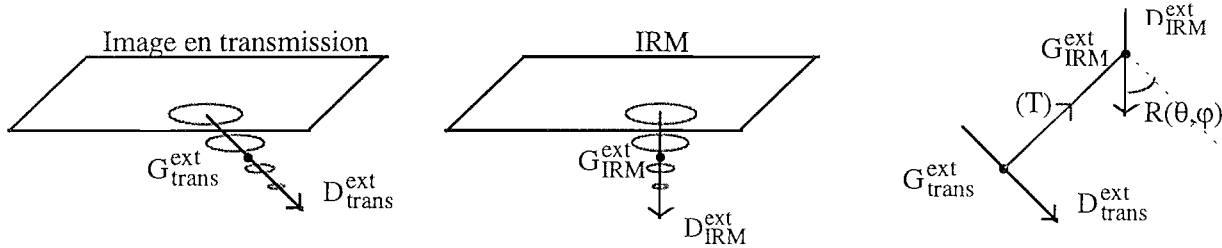
Figure IV-7: Principe du recalage. (a) calcul de la position ainsi que de l'orientation de la paroi externe dans le repère des images en transmission, (b) même chose dans le repère des images en IRM, (c) mise en coïncidence des deux repères, T: translation, R: rotation.
