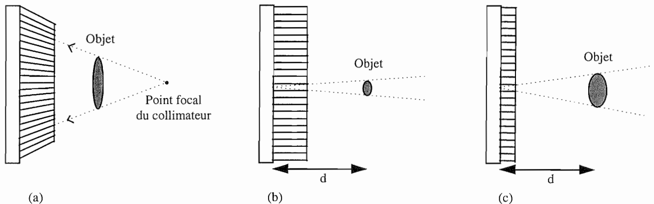
Figure I-12: Exemple de collimateurs, (a) convergent, (b) haute résolution et (c) basse énergie.
