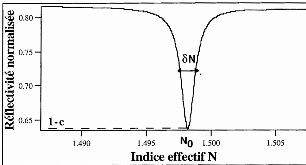
Figure A-1 : Module au carré de l'amplitude réfléchie TE du MR en fonction de l'indice effectif. La couche guidante est en \text{TiO}_2 d'indice 2,15 - j2,2 \cdot 10^{-4} et d'épaisseur 42 nm, le milieu espaceur est en \text{SiO}_2 d'indice 1,46 et d'épaisseur 700 nm.
