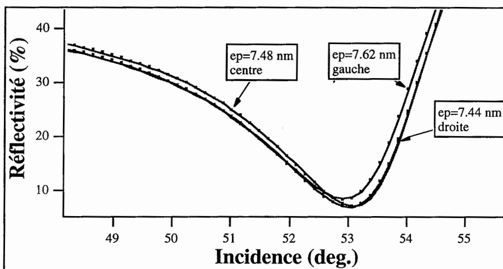
Figure III-24 : Contrôle de l'homogénéité de la surface d'un plot de polypyrrole d'une épaisseur annoncée de 7,5 nm sur une ligne de 9 mm de long. Les points expérimentaux sont en pointillés, les meilleurs ajustements de ces courbes sont en trait plein.
