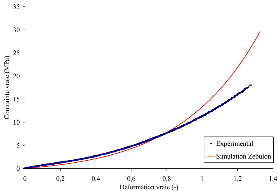
Figure 3.9 Optimisation des paramètres viscoélastiques sur un des essais d'écroutissage à 5.10^{-3} s^{-1} de déformation vraie
