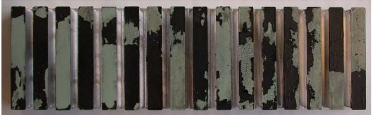
Figure 2.56 Faciès de rupture des essais à 300 \mu\text{m} –en sombre, la colle FMV, en clair, le substrat en aluminium peint
