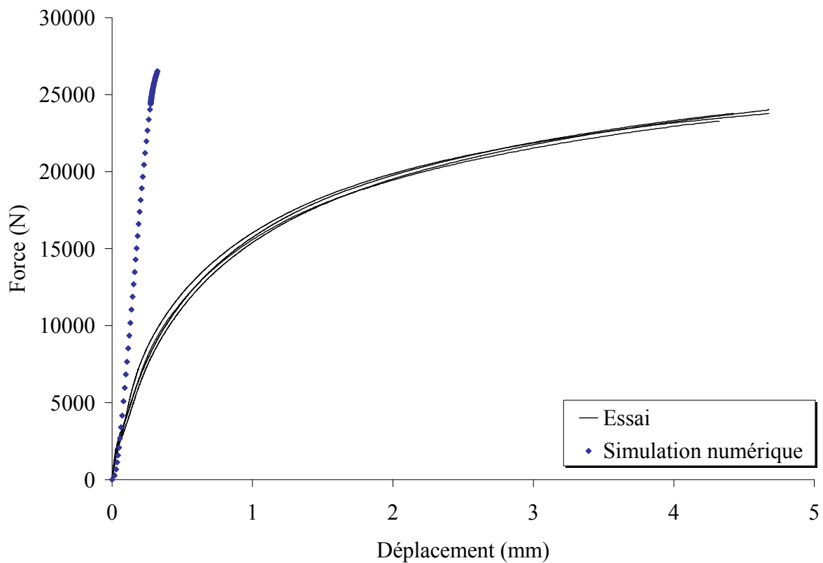
Figure 5.19 Comparaison essai-simulation sur éprouvettes boulonnées : courbe force-déflexion des fixations à 71 N/s
