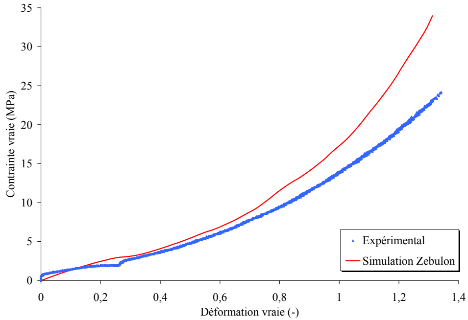
Figure 3.7 Optimisation des paramètres viscoélastiques sur un des essais d'écroutissage à 1.10^{-1} \text{ s}^{-1} de déformation vraie
