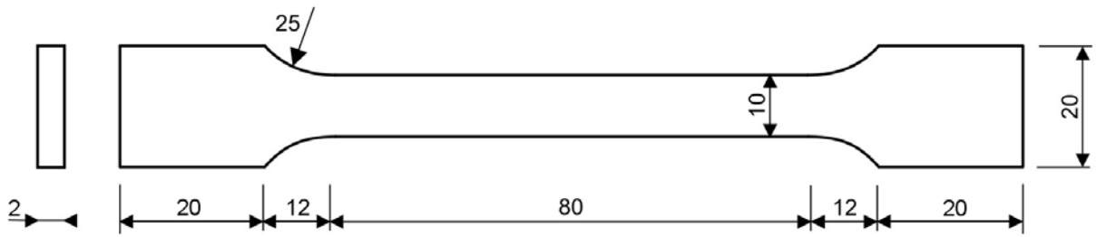
Figure 9.7 Géométrie des éprouvettes de colle XPU d'après la norme [AFNOR NF EN ISO 527, 1996].
