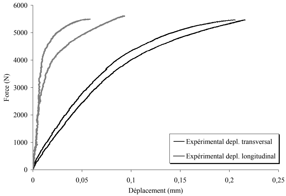
Figure 9.16 Essais Arcan-Mines à 60^\circ à 7 \text{ N.s}^{-1} , 2 spécimens - colle XPU
