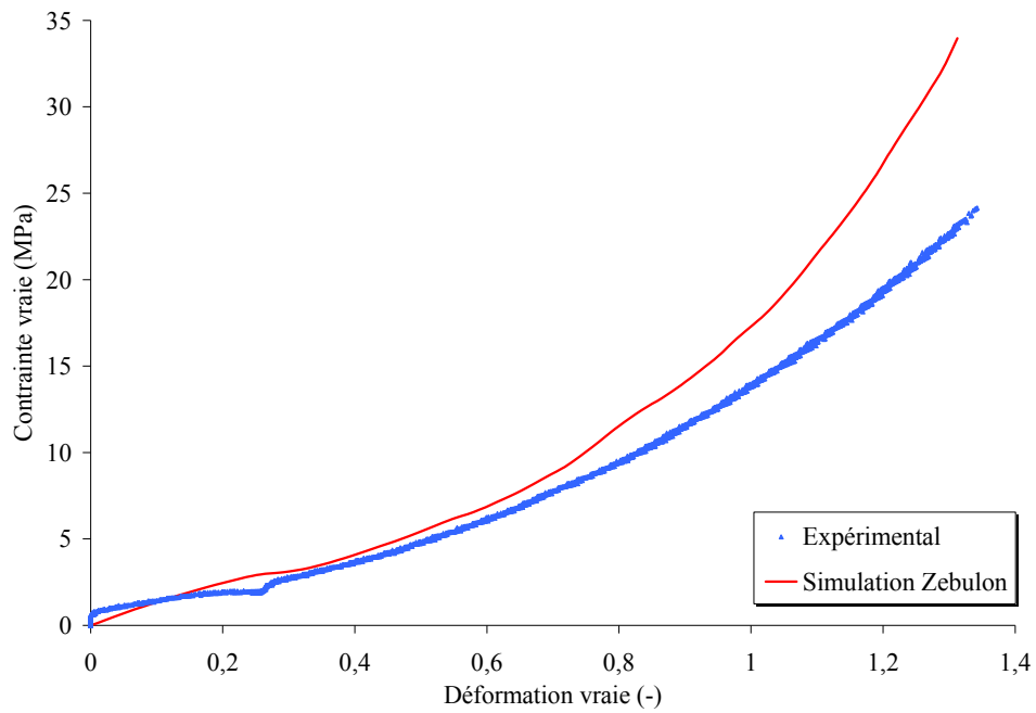
Figure 3.7 Optimisation des paramètres viscoélastiques sur un des essais d'écroutissage à 1.10^{-1} s^{-1} de déformation vraie
