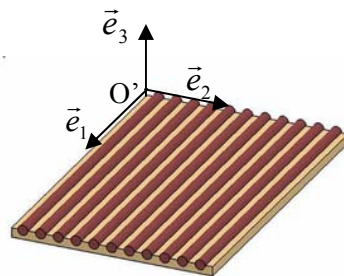
Figure 2.8 Axes d'orthotropie du pli unidirectionnel de base
