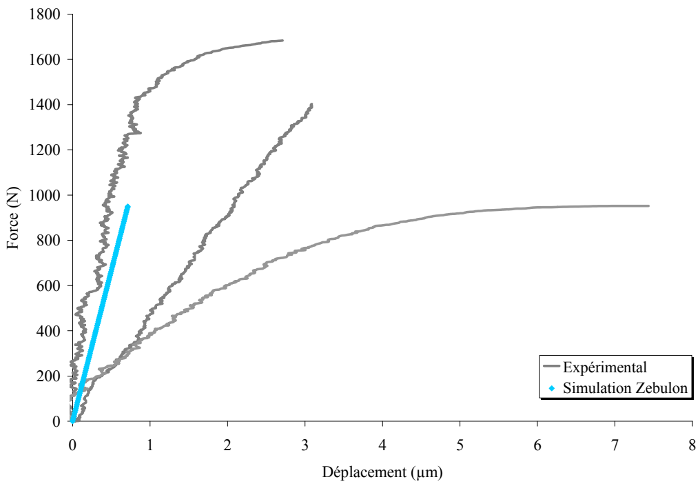
Figure 3.21 Simulation des essais Arcan-Mines à 0° à épaisseur nominale de 100 μm - colle FMV
