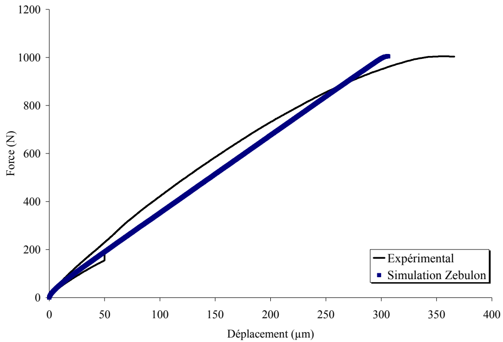
Figure 3.22 Simulation des essais Arcan-Mines à 90° à épaisseur nominale de 300 µm - colle FMV
