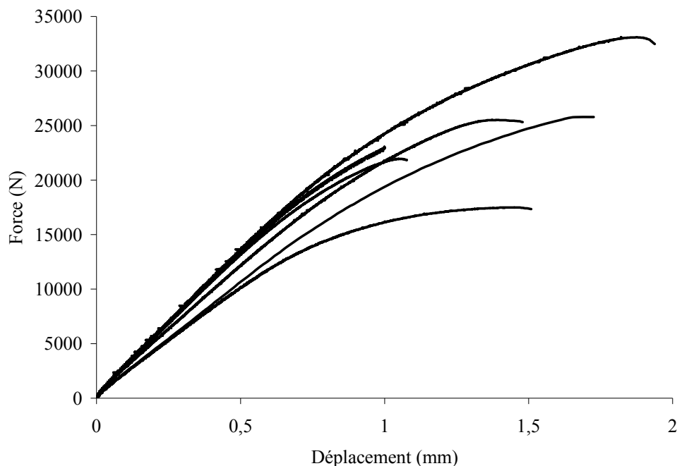
Figure 2.61 Courbe force-déplacement entre substrats centraux à 1 \text{ N}\cdot\text{s}^{-1} , 7 spécimens – colle XPU
