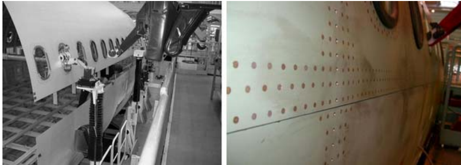
Figure 5.1 Assemblage des panneaux de fuselage d'un avion Airbus par trois lignes de fixation [Ramière, 2010]
