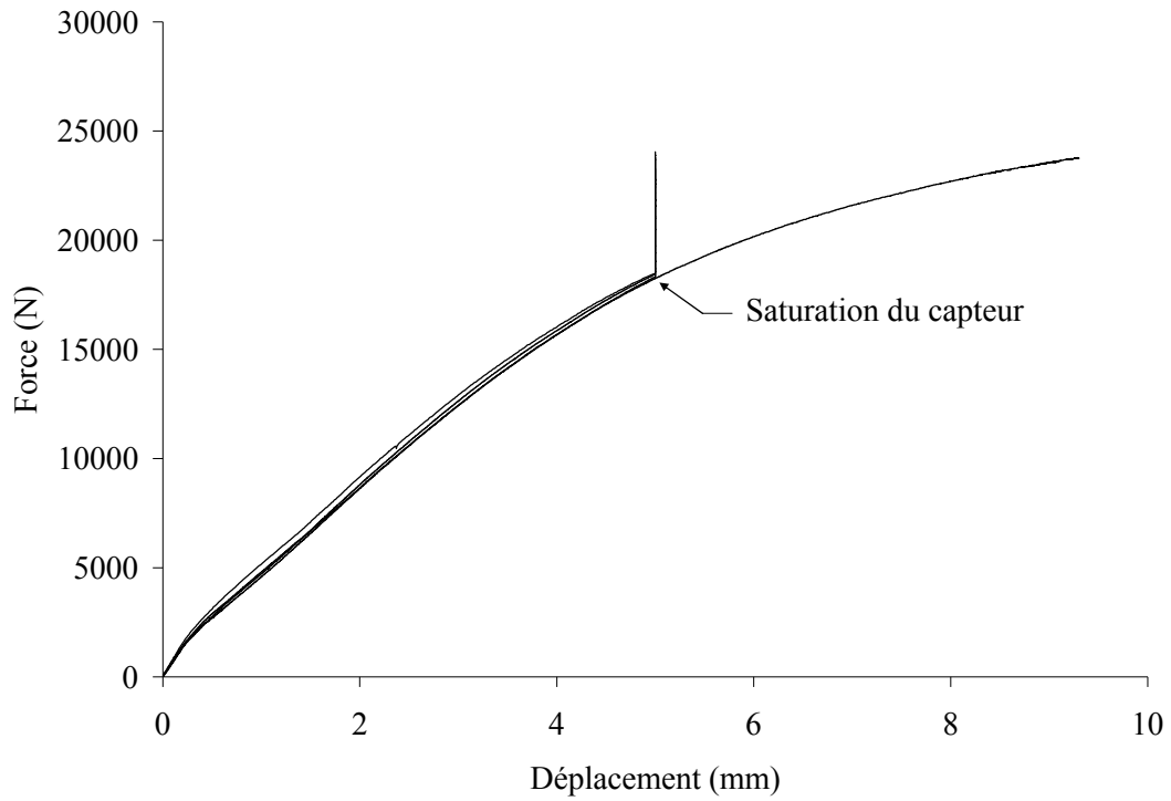
Figure 9.22 Eprouvettes boulonnées : courbe force-déplacement traverse à 71 N/s
