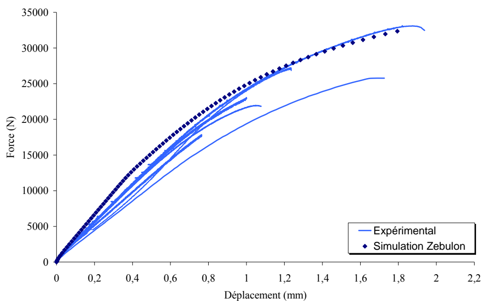
Figure 3.25 Essais et simulation des éprouvettes de quadruple cisaillement avec épaisseur nominale de colle
