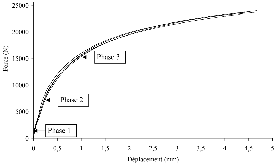
Figure 5.7 Eprouvettes boulonnées : courbe force-déplacement des fixations et phases de déformation
