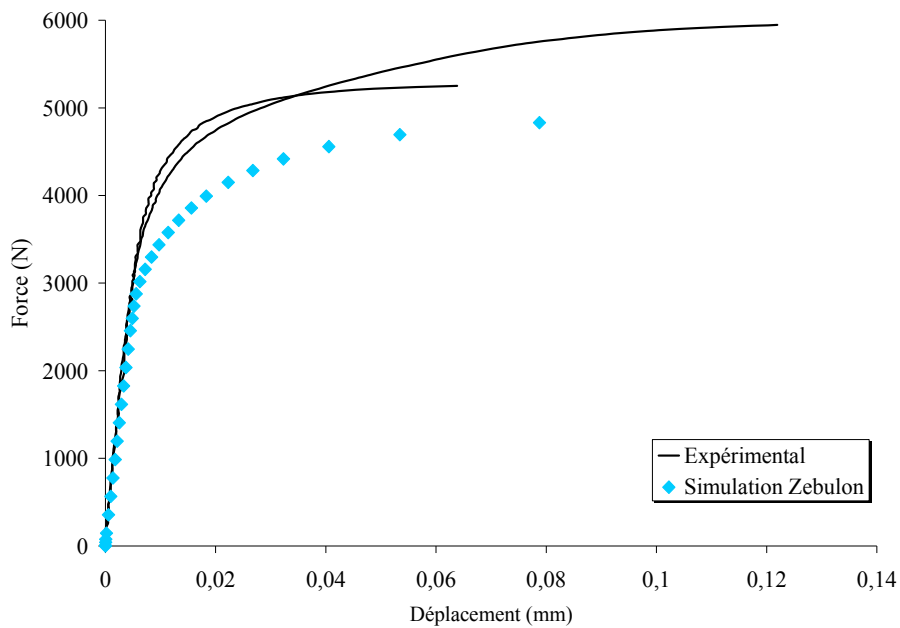
Figure 3.16 Simulation des essais Arcan-Mines à 0° - colle XPU
