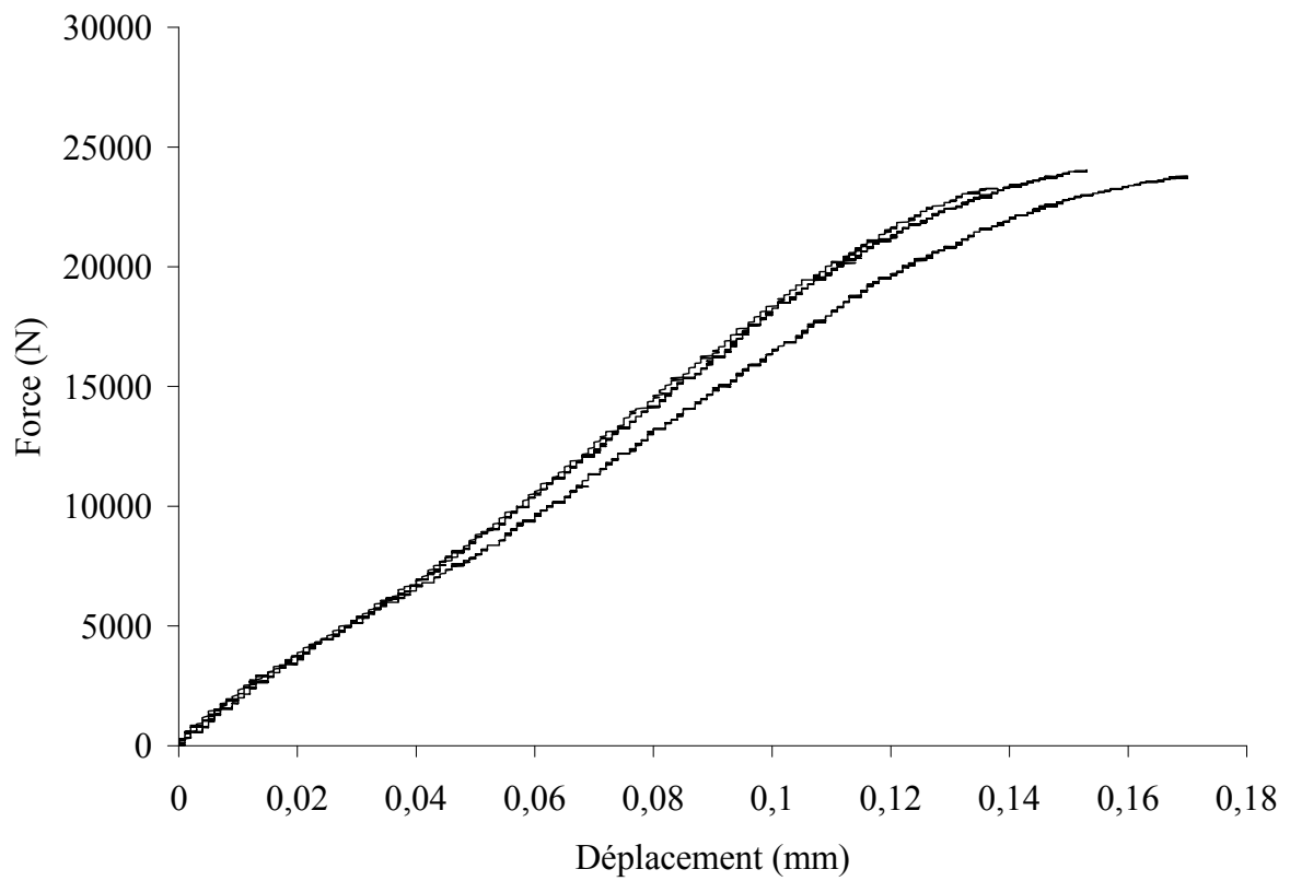
Figure 9.23 Eprouvettes boulonnées : courbes force-déplacement du substrat près du mors à 71 N/s
