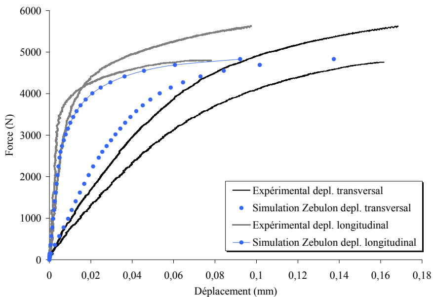
Figure 3.17 Simulation des essais Arcan-Mines à 30° - colle XPU
