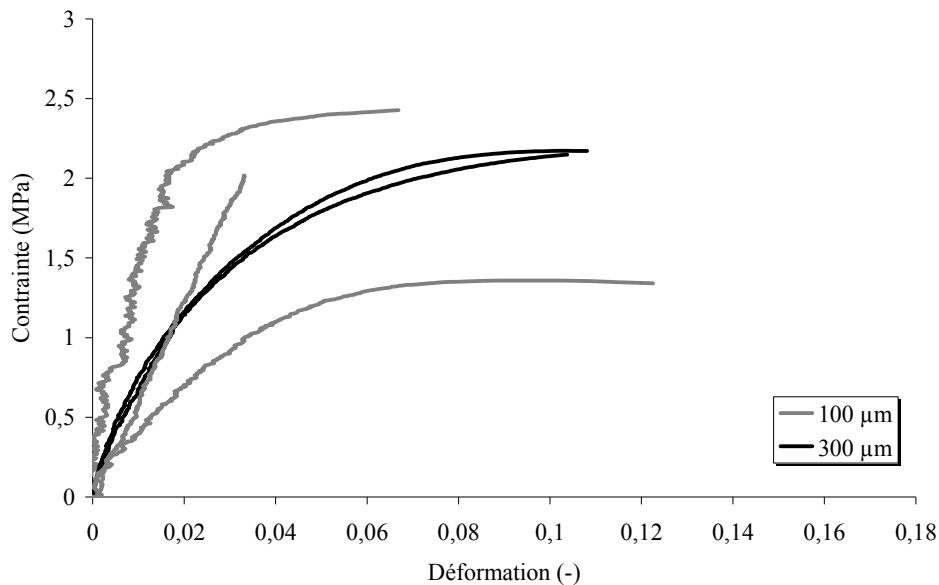
Figure 2.54 Comportement en traction (0°) à 7 N.s -1 , 3 spécimens à 100 µm, 2 spécimens à 300 µm - colle FMV
