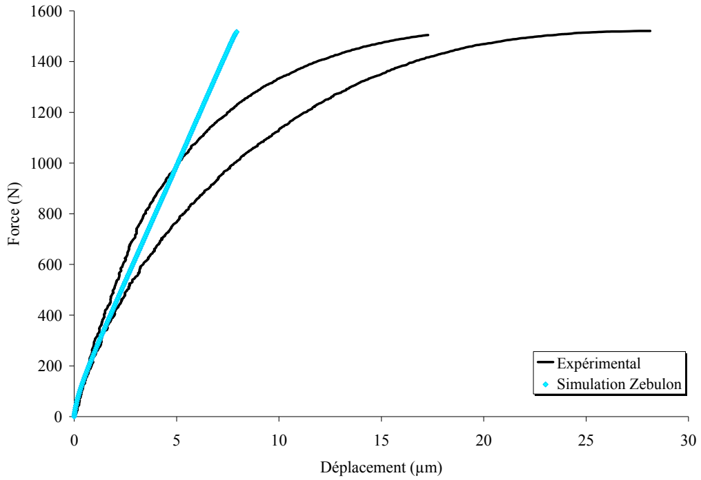
Figure 3.20 Simulation des essais Arcan-Mines à 0° à épaisseur nominale de 300 μm - colle FMV
