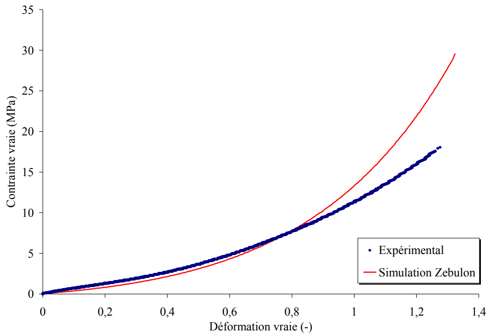
Figure 3.9 Optimisation des paramètres viscoélastiques sur un des essais d'écroutissage à 5 \cdot 10^{-3} \text{ s}^{-1} de déformation vraie
