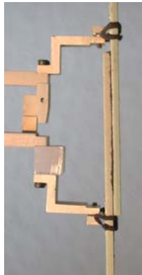
Figure 2.62 Mesure du déplacement relatif entre substrats
