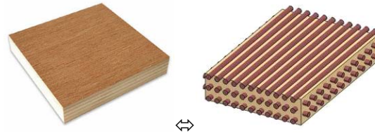
Figure 2.9 Le bois contreplaqué est un composite stratifié à plis orientés à 90°
