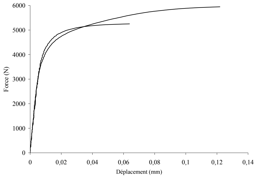
Figure 9.14 Essais Arcan-Mines à 0^\circ à 7 N.s^{-1} , 2 spécimens - colle XPU
