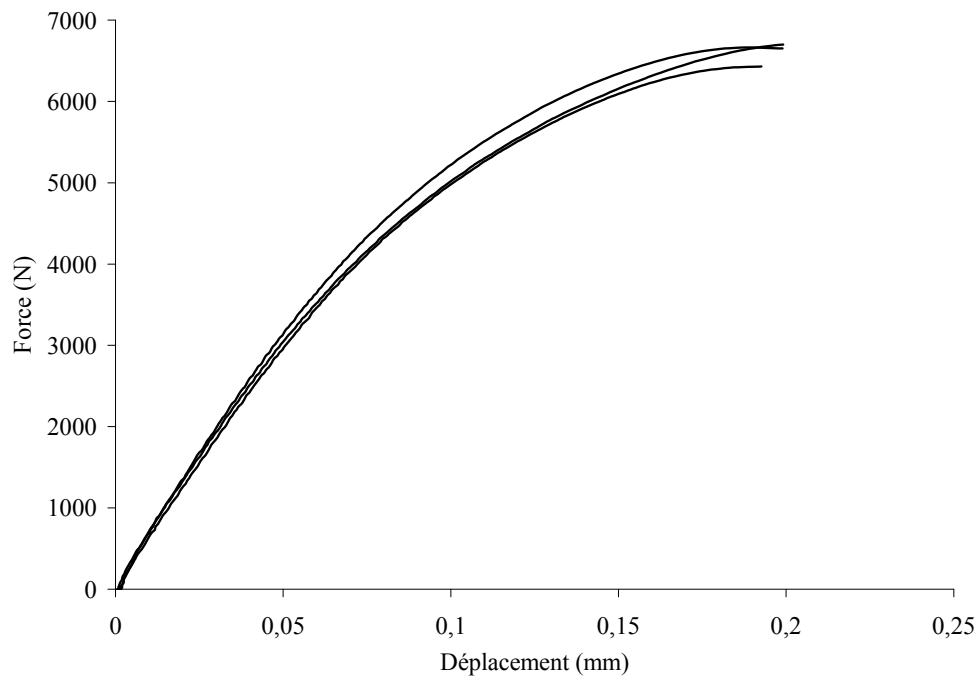
Figure 9.17 Essais Arcan-Mines à 90^\circ à 7 \text{ N.s}^{-1} , 3 spécimens - colle XPU
