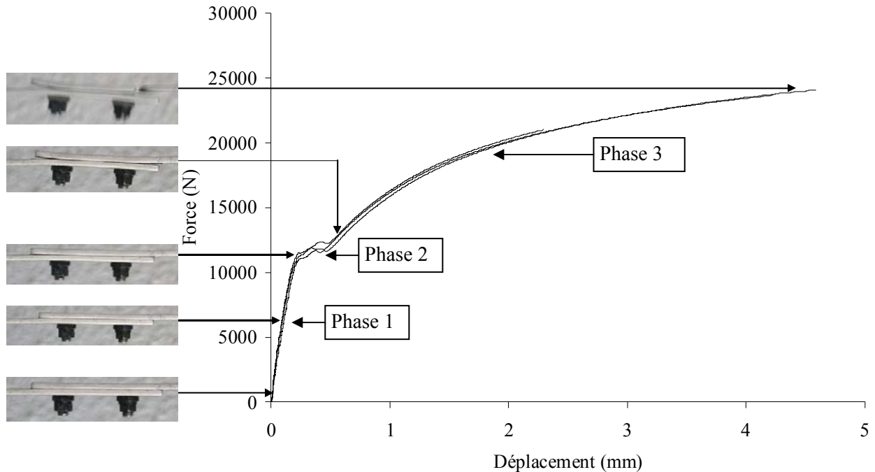
Figure 5.9 Eprouvettes hybrides : courbe force-déplacement des fixations et phases de déformation
