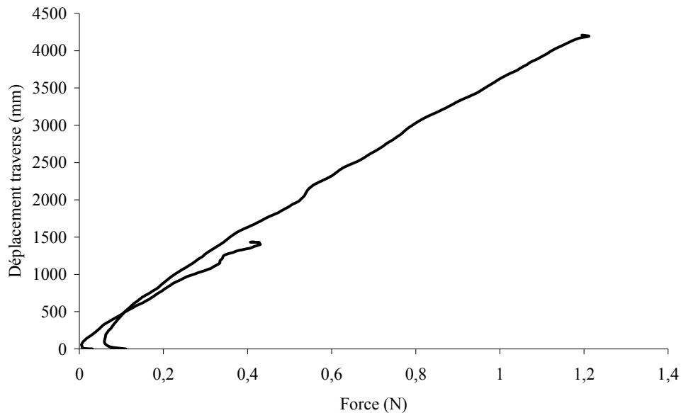
Figure 2.63 Courbe force-déplacement traverse des essais de simple recouvrement à 75 \text{ N}\cdot\text{s}^{-1} , 2 spécimens retenus sur les 6 testés
