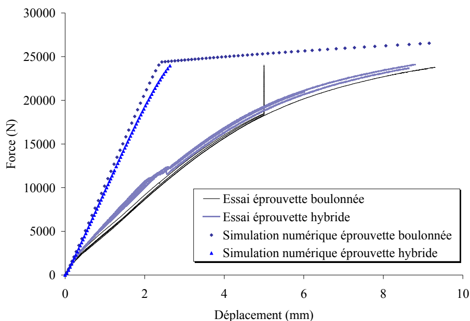
Figure 5.28 Comparaison des simulations : courbes force-déplacement traverse
