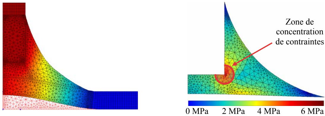
Figure 4.11 Déformée de la liaison en T : à gauche, isovalues de déplacement selon Ox ; à droite, isovalues par éléments de la contrainte de Von Mises dans la colle
