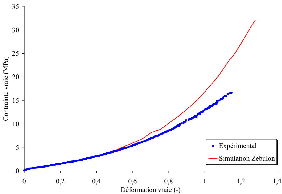
Figure 3.8 Optimisation des paramètres viscoélastiques sur un des essais d'écroutissage à 5.10^{-2} s^{-1} de déformation vraie
