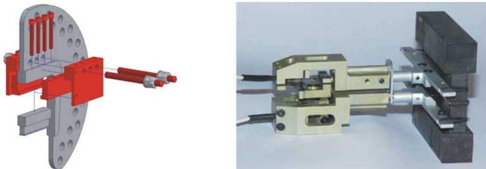
Figure 2.48 A gauche, ancrage des éprouvettes dans le système Arcan-Mines. A droite, extensomètre double utilisé pour les essais en état mixte. Images [Joannès, 2008]
