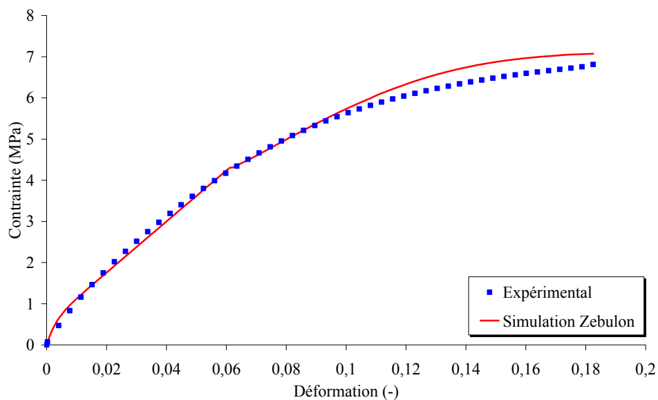
Figure 3.5 Optimisation des paramètres d'érouissage cinématique sur un des essais de traction à 10^{-3} \text{ s}^{-1}
