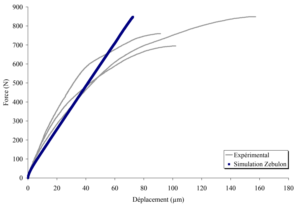
Figure 3.23 Simulation des essais Arcan-Mines à 90° à épaisseur nominale de 100 µm - colle FMV
