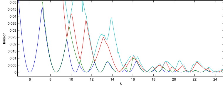
FIGURE 3.7 – Tension pour une plaque carrée encastree
