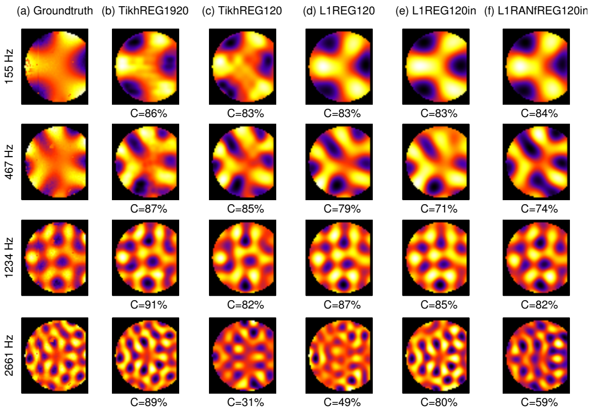
FIGURE 6.5 – Reconstruction de 4 déformées opérationnelles de la plaque circulaire avec diverses méthodes
