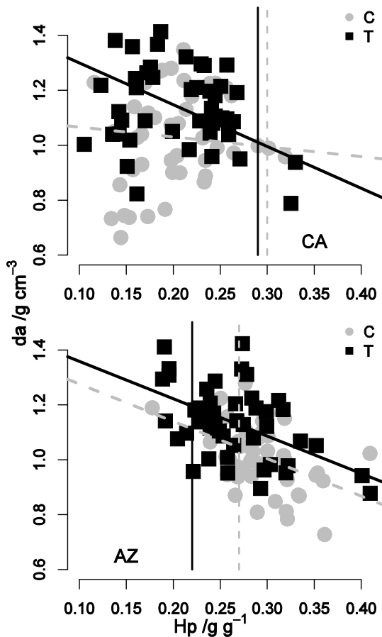
Figure 2 Analyse de l'effet du traitement (C, control/ témoin ; T, trafficked/ tassé) sur la densité du sol ( da ) de la couche de surface (0–10 cm) en prenant en compte l'effet de l'humidité pondérale du sol au moment du prélèvement ( Hp ), les points correspondent aux mesures et les lignes aux modèles expliquant da en fonction de Hp et du traitement (gris, témoin et noir, tassé). Les prélèvements ont eu lieu en même temps que les mesures de résistance à la pénétration des sols en juin 2011. Les barres verticales correspondent aux humidités lors des mesures de densité apparente sur fosses de mai 2011 (II).
