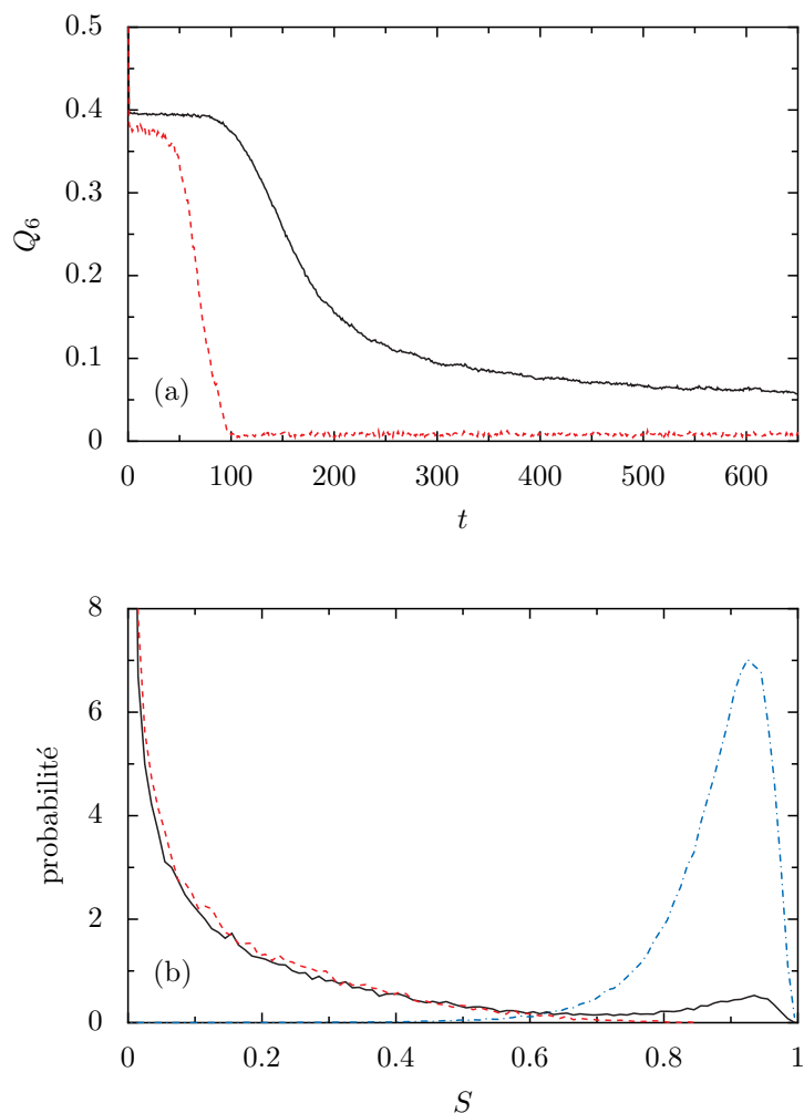
FIGURE 4.6 – Effets de taille finie sur la coexistence liquide-solide à l'équilibre en dynamique moléculaire. (a) Evolution temporelle du paramètre d'ordre global de liaison Q_6 , pour un nombre total de particules N = 110\,592 à la fraction volumique \phi = 0,504 (ligne continue) et pour N = 13\,824 à \phi = 0,499 (tirets). La dernière fraction volumique est choisie pour que les temps d'attente soient comparables et traçables aisément sur le même graphique, dans les deux cas. (b) Densité de probabilité de la variable S pour un système où solide et liquide coexistent à l'équilibre pour N = 110\,592 à \phi = 0,504 (ligne continue) ; un solide stable pour N = 110\,592 à \phi_f = 0,55 (ligne pointillée) et un liquide pur à l'équilibre pour N = 13\,824 à \phi = 0,504 (tirets).
