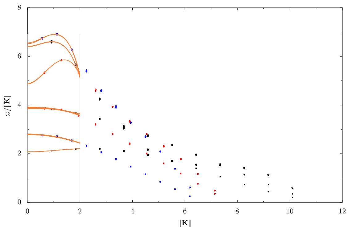
FIGURE 3.25 – Évolution de la variable \omega/K en fonction de la norme \|K\| du vecteur du réseau réciproque déduite de simulations de dynamique moléculaire après application de l’algorithme hongrois pour un système de N = 1\,728 particules à la fraction volumique \phi = 0,499 . Les symboles ont la même signification que dans la figure 2.5. Les courbes orange approchent les données de dynamique moléculaire par l’équation (2.112) pour des valeurs de \|K\| comprises entre 0 et 2. Ces deux valeurs limites sont signalées par deux lignes verticales grises.
