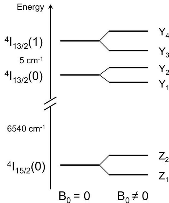
Figure 10 : éclatement des niveaux Zeeman fondamentaux et excités sous l'effet du champ magnétique externe.
