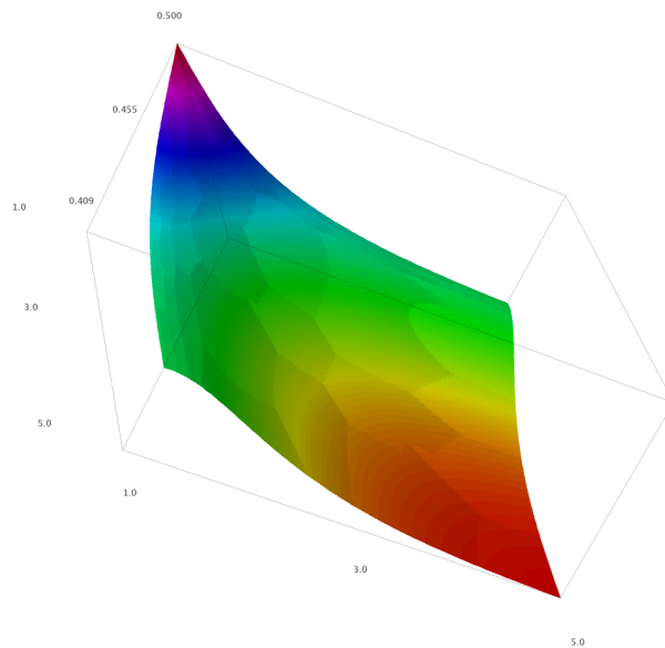
FIGURE 4 – Graphe de f_2(x, y) pour 1 \leq x, y \leq 5
