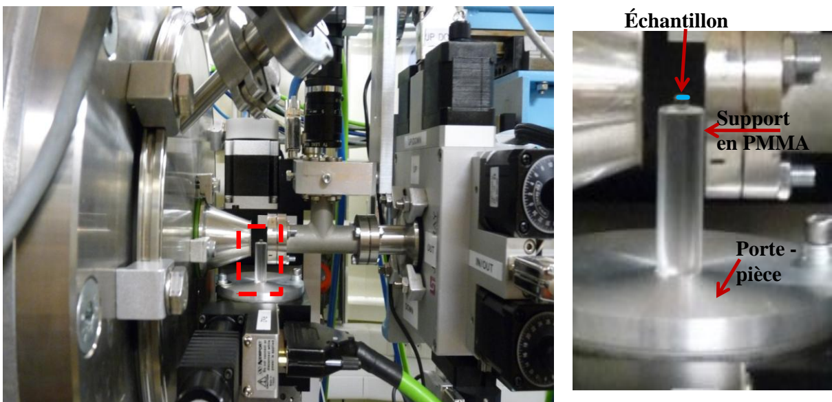
Figure 2.25 : Montage utilisé pour les mesures en SAXS et WAXS avec faisceau synchrotron.
