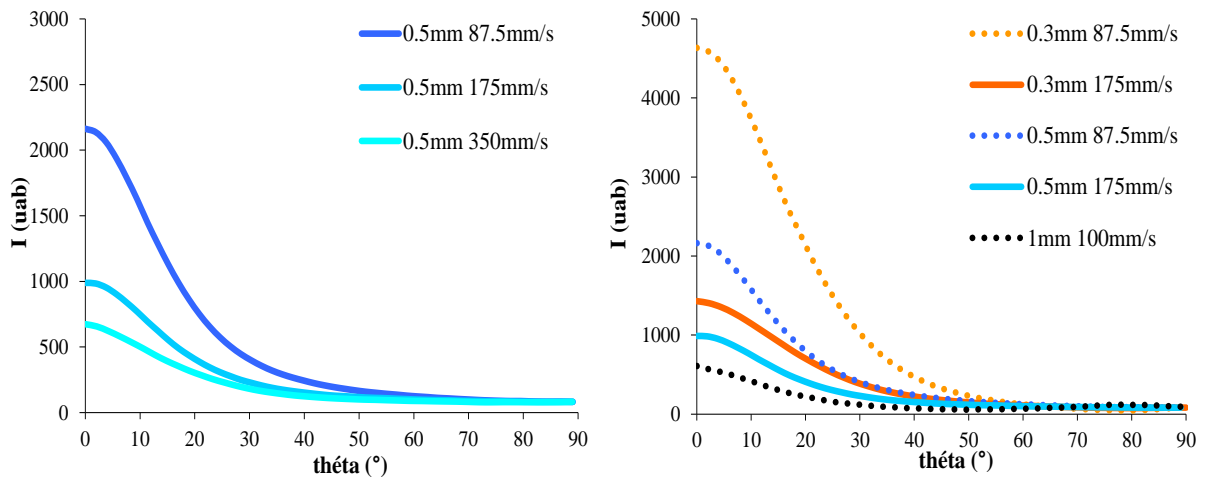
Figure 3.33 : Courbes d'intensités azimuthales diffusées pour des plaques de PEhd injectées à différentes épaisseurs (mm) et vitesses d'injection (mm/s) et une longueur d'écoulement de 15 mm.
