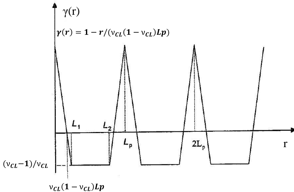
Figure 2.29 : Fonction d'autocorrélation monodimensionnelle d'une structure idéale [Etienne et David, 2002].
