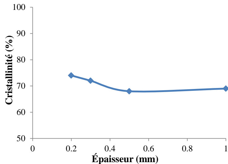
Figure 3.19 : Cristallinités mesurées par densimétrie des échantillons entiers en fonction de l'épaisseur injectée.
