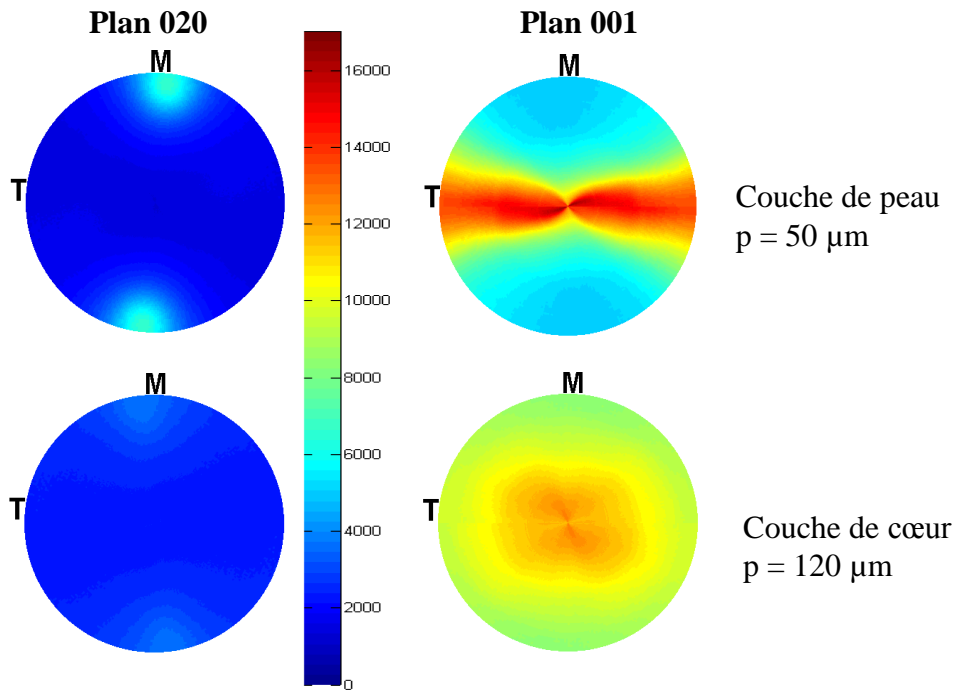
Figure 3.48 : Figures de pôle par WAXS avec faisceau synchrotron à différentes profondeurs d'une plaque de 0,2 mm d'épaisseur injectée en PA12. Temps d'injection = 0,04s, Température du moule = 105°C.
