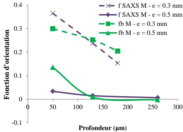
Figure 3.52 : Influence de l'épaisseur injectée sur les fonctions d'orientation de l'axe des chaînes b et des normales aux lamelles selon la direction d'injection M à travers l'épaisseur des plaques de 0,5 mm et de 0,3 mm injectées en PA12. Temps d'injection = 0,1 s. Température du moule = 105°C.
