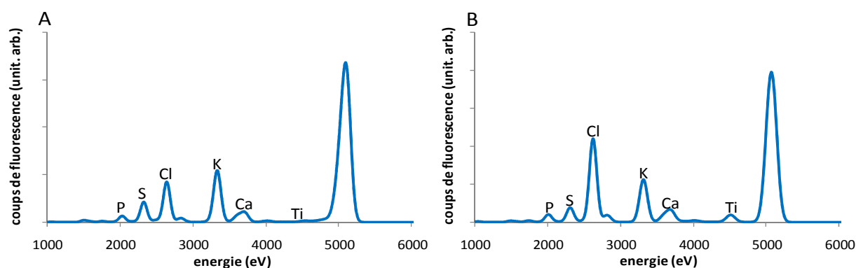
Figure 80 : Spectres XRF de coupes de racine de blé cultivé dans de l'eau ultrapure (A) ou exposé à 100 mg/L de NPs de TiO 2 A25 (B).
