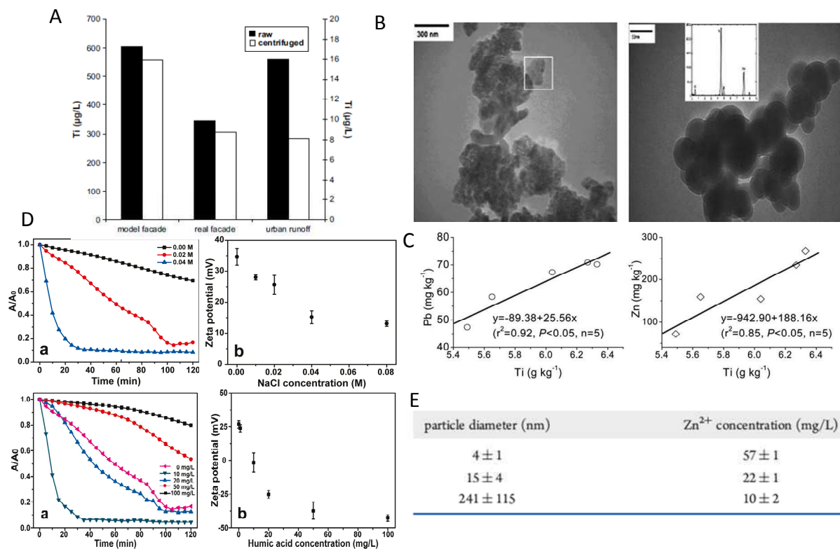
Figure 14 : A. Dosage du titane dans les eaux de lessivage directement après prélèvement ou après centrifugation (axe de gauche pour la façade modèle, axe de droite pour la façade réelle et pour les eaux de lessivage urbaines) [Kaegi et al., 2008]. B. Observations en microscopie électronique à transmission de l’aspect du titane dans les sédiments de la baie de Xiamen en Chine [Luo et al., 2011]. C. Corrélation du titane des sédiments avec le plomb et le zinc [Luo et al., 2011]. D. Influence de la force ionique et de la teneur en acides humiques sur le potentiel zeta et la sédimentation (A/A0) de NPs de ZnO [Bian et al., 2011]. E. Dissolution de 1000 mg/L de NPs de ZnO en suspension à pH 7,5 en fonction de leur diamètre nominal [Bian et al., 2011]
