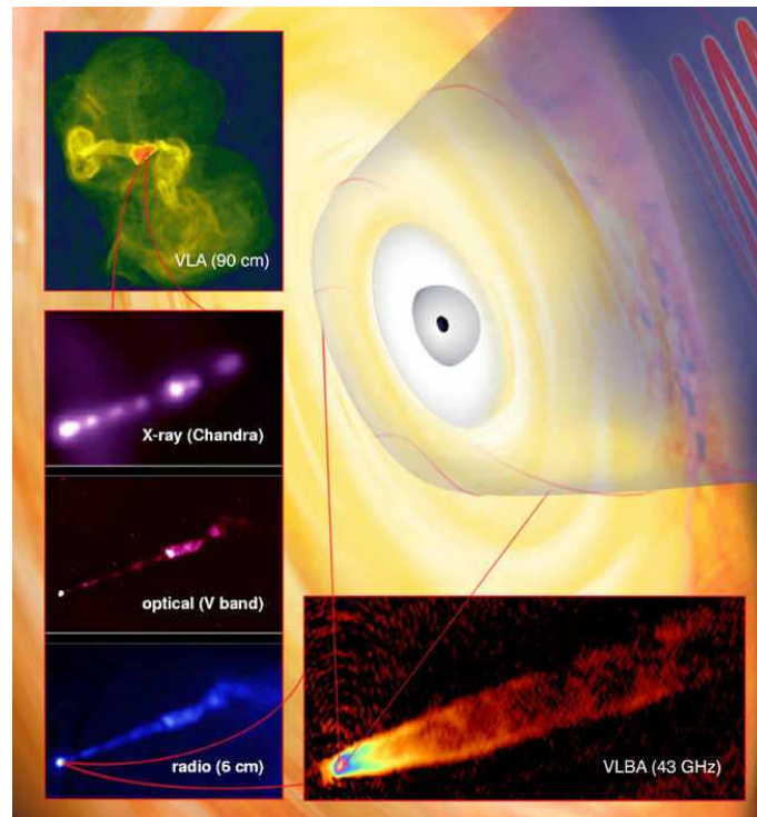
FIGURE 4.24 – Vue d'artiste de la base du jet (dans la région supposée responsable de l'émission au TeV à partir de contraintes sur la variabilité) et observations à différentes longueurs d'onde de la radiogalaxie M87.
