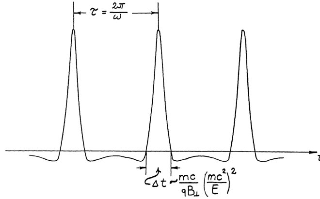
FIGURE 3.2 – Représentation de l'émission synchrotron d'un électron dans un champ magnétique B au cours du temps [Ginzburg 1965].
