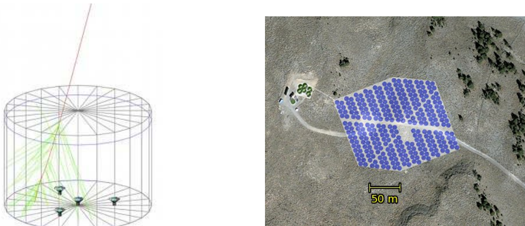
FIGURE 5.9 – Gauche : simulation d'une particule traversant une des cuves à eau de HAWC (en rouge) et émission Tcherenkov créée (en vert). Quatre PMTs sont disposés au fond de la cuve pour collecter la lumière Cherenkov. Droite : agencement prévu des 300 cuves à eau composant le détecteur HAWC. Le prototype VAMOS actuellement en cours de tests est visible sur la gauche. Crédit : http://hawc.umd.edu/ .
