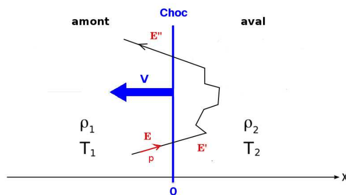
FIGURE 2.7 – Schématisation de l'accélération de Fermi du 1 er ordre.
