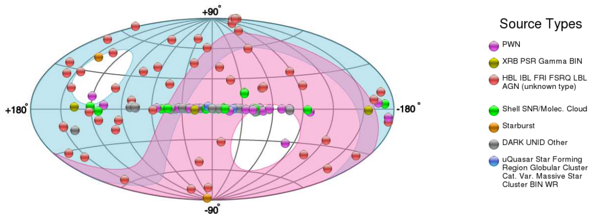
FIGURE 5.13 – Sources du catalogue TeV Cat en coordonnées galactiques et visibilité accessible par VERITAS/MAGIC (en bleu) ainsi que pour H.E.S.S. (en rose). Crédit : http://tevcats.uchicago.edu/ .
