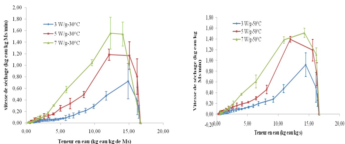
Figure 4.4- Effet des puissances spécifiques sur la vitesse de séchage à différentes conditions de séchage MOAC ( a- 3 W/g-30°C, 5 W/g-30°C et 7 W/g-30°C et b- 3 W/g-50°C, 5 W/g-50°C et 7 W/g-50°C à vitesse constante (1,5 m/s)) de la tomate, en régulation continue de la puissance spécifique.
