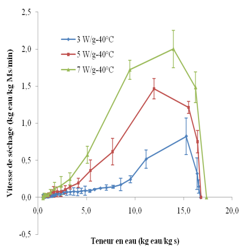
A.5.1d- Vitesse de séchage MOAC(40°C) avec pilotage de Ps par intermittence
