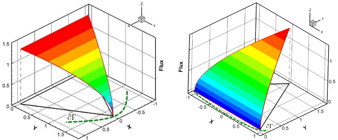
Fig 23. Interpolation du flux sur les éléments du type 1 et 2 [180]
