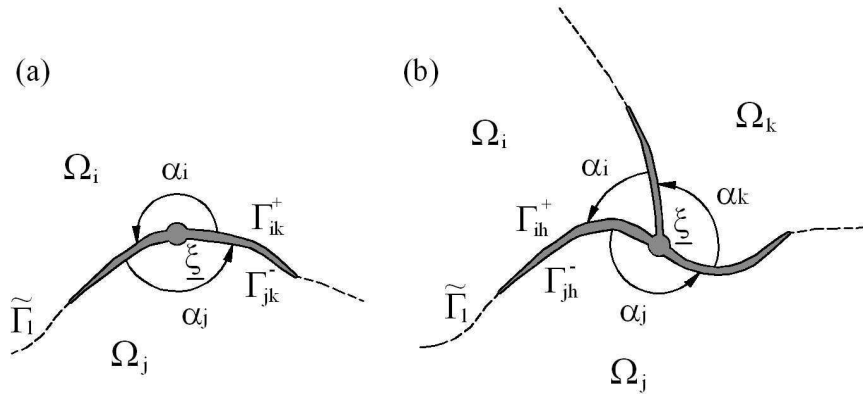
Fig 43. Point observé \underline{\xi} situé : (a) sur une fissure \alpha_i + \alpha_j = 2\pi ; en un point d'intersection entre fissures \alpha_i + \alpha_j + \alpha_k = 2\pi
